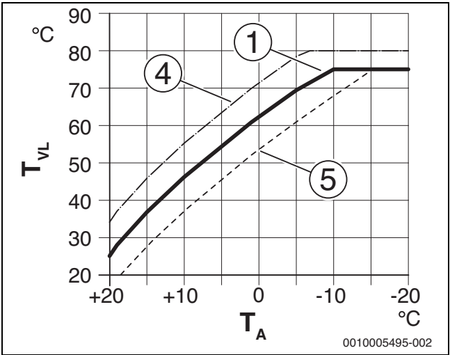
Bild 12 Einstellung der Heizkurve für Heizkörper Parallelverschiebung über Raumtemperatur-Offset oder gewünschte Raumtemperatur
