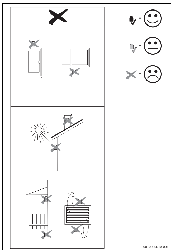
Bild 3 Ungeeigneter Installationsort des Außentemperaturfühlers
