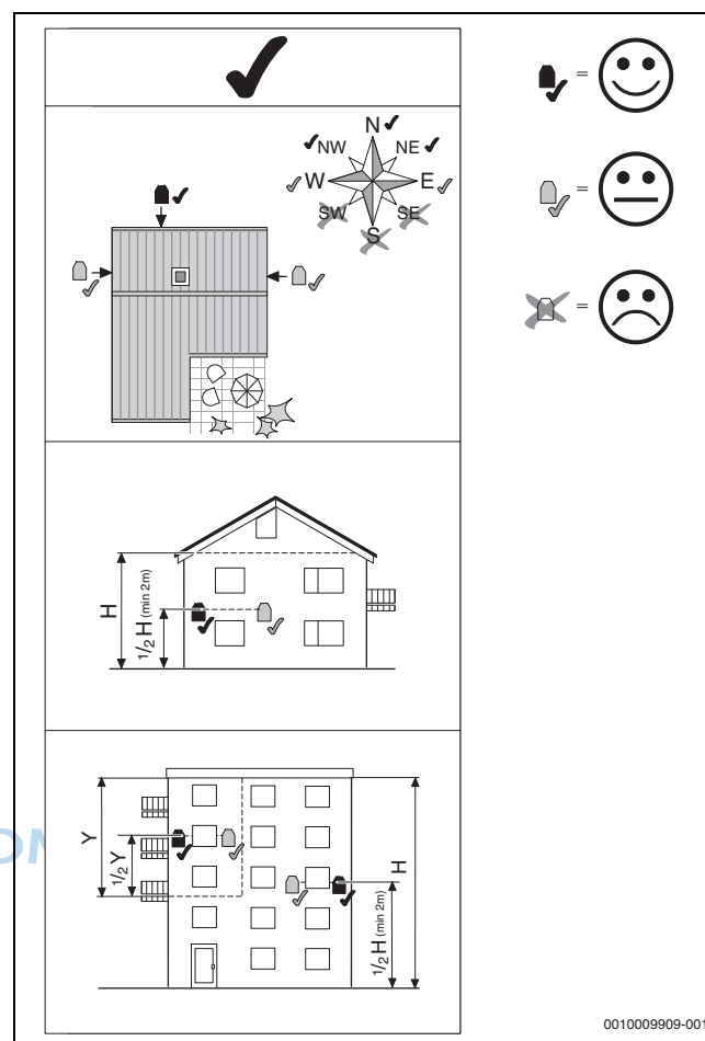
Bild 2 Geeigneter Installationsort des Außentemperaturfühlers
