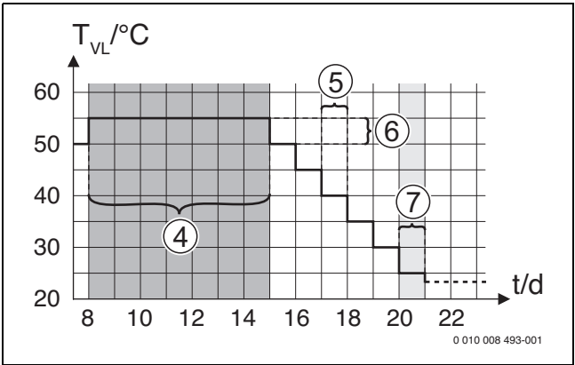
Bild 14 Ablauf der Estrichtrocknung mit den Grundeinstellungen in der Abkühlphase
