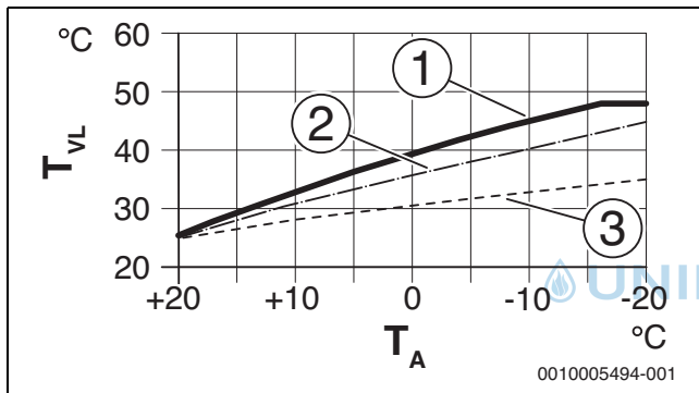
Bild 9 Einstellung der Heizkurve für Fußbodenheizung Steigung über Auslegungstemperatur T_{AL} und minimale Außentemperatur T_{A,min}
