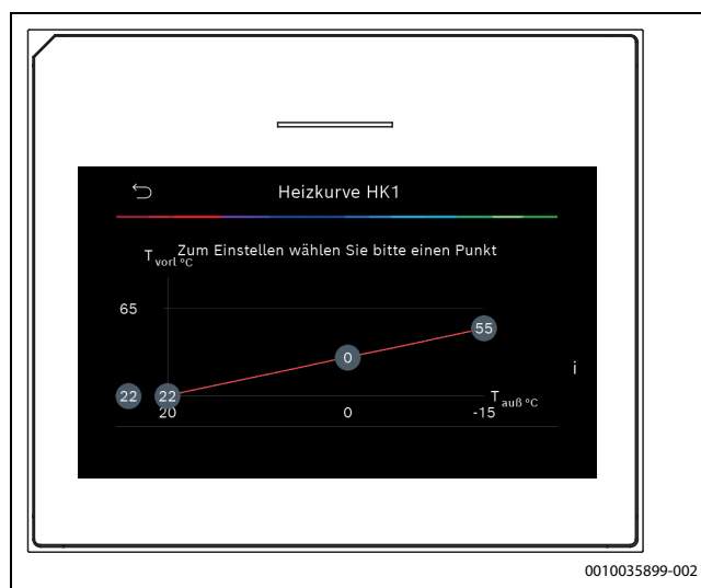
Bild 5 Startmenü Heizkurve
