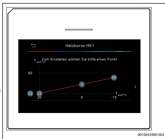
Bild 6 Endpunkt einstellen
