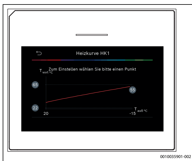
Bild 7 Fußpunkt einstellen
