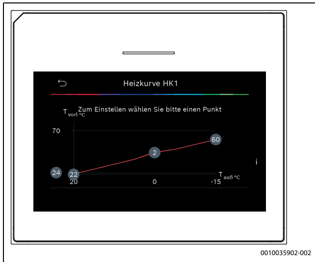
Bild 8 Komfortpunkt einstellen
