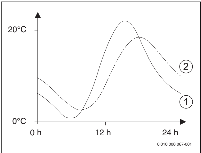
Bild 4 Beispiel für die gedämpfte Außentemperatur
