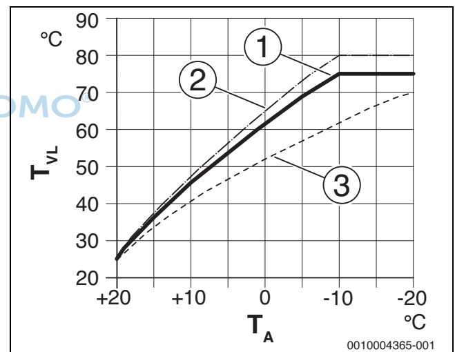
Bild 11 Einstellung der Heizkurve für Heizkörper Steigung über Auslegungstemperatur T_{AL} und minimale Außentemperatur T_{A,min}
