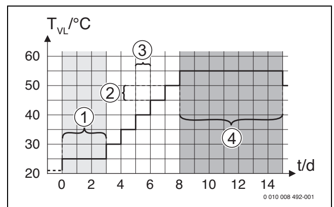
Bild 13 Ablauf der Estrichtrocknung mit den Grundeinstellungen in der Aufheizphase
