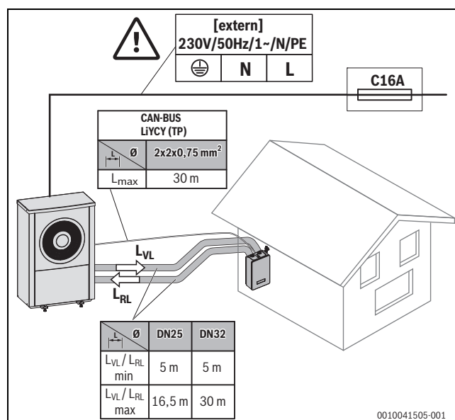
Bild 13 Maximale Längen der Leitungen
