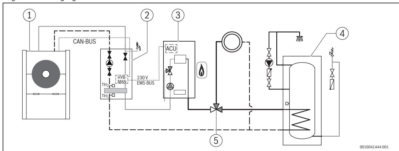
Bild 14 Hydraulisches Schema, Beispiel
