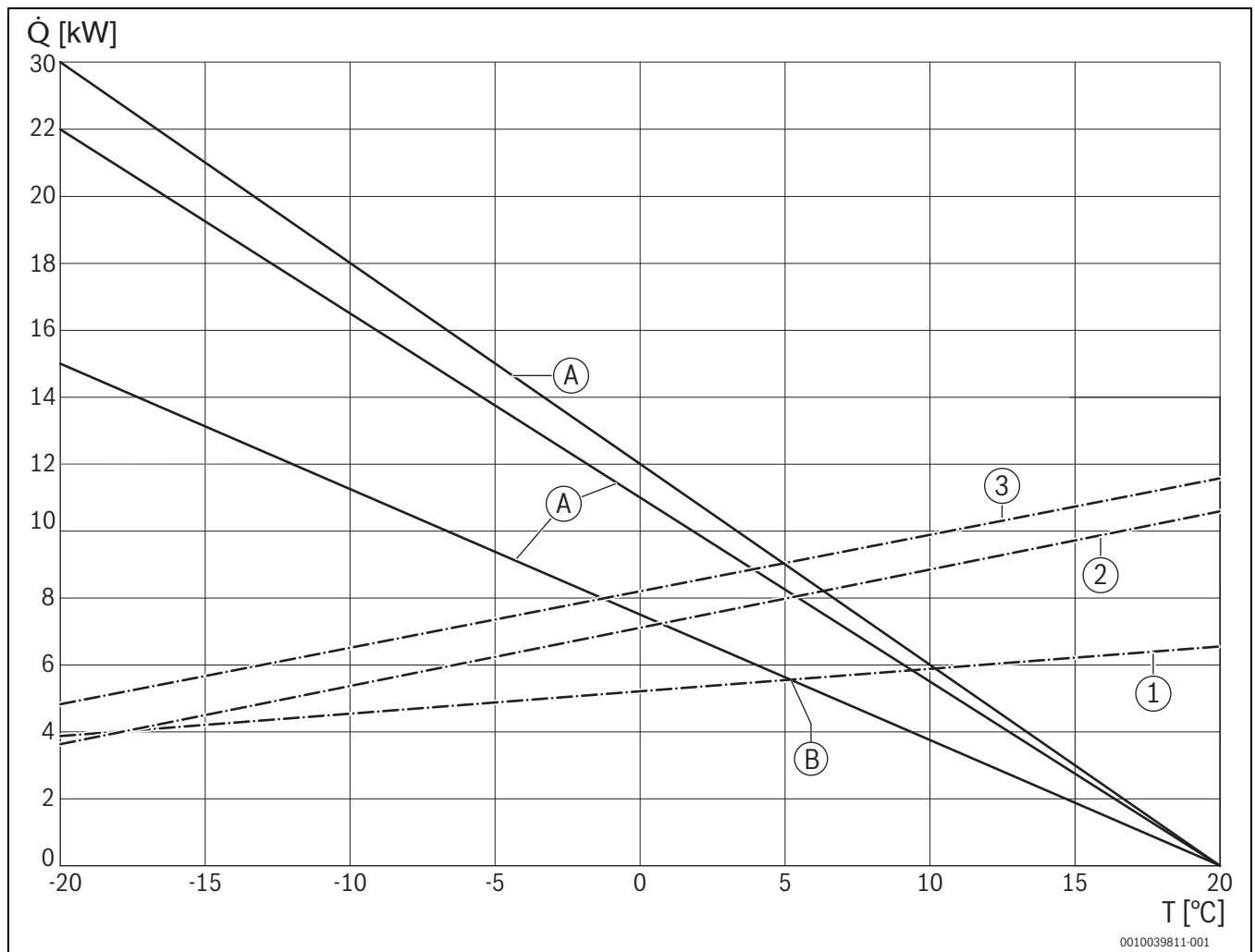
Bild 31 Diagramm zu Tab. 14; Zur Bestimmung der Bivalenzpunkte bei 55 °C Vorlauftemperatur
