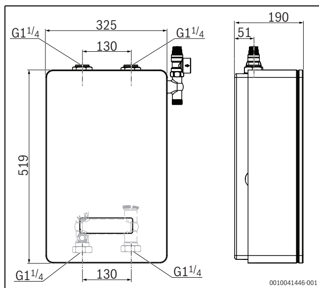
Bild 33 Abmessungen
