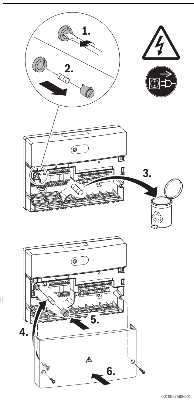
Bild 28 Sicherung tauschen
