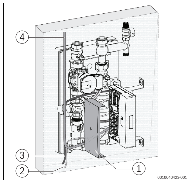
Bild 16 Elektrische Leitungen anschließen
