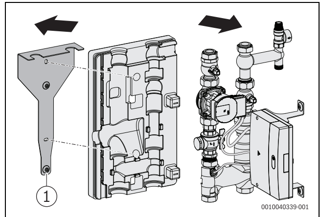
Bild 9 Wandhalterung entnehmen
