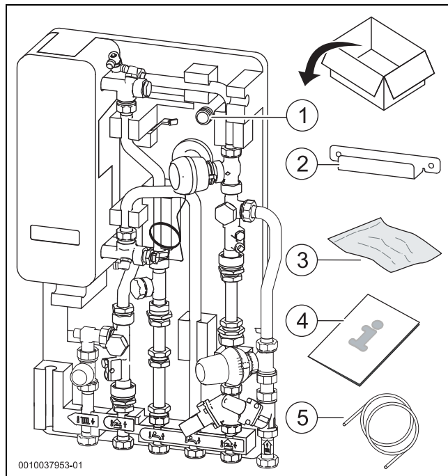
Bild 3 Lieferumfang Wohnungsstation
