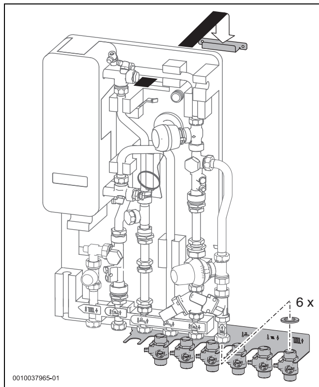
Bild 13 Station aufhängen
