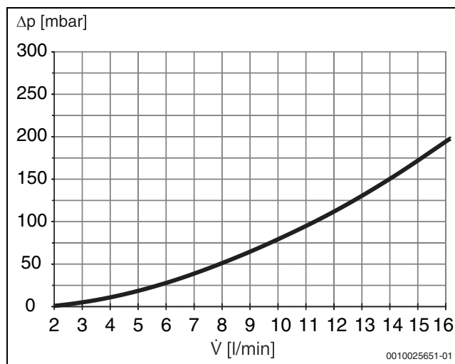
Bild 6 Druckverlust Trinkwasserseite
