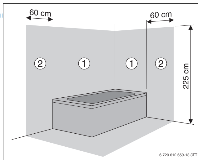
Bild 10 Schutzbereiche im Aufstellraum
