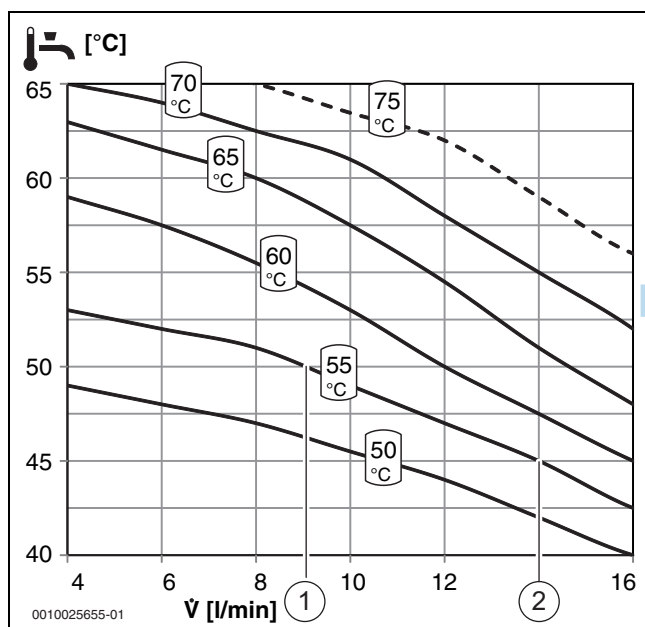
Bild 8 Temperaturverhalten bei entfernter Sperre des Warmwasserthermostats und Stellung 7 (max.)
