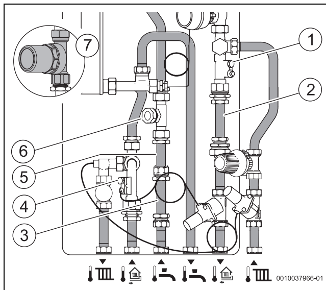
Bild 14 Adapterrohre ersetzen
