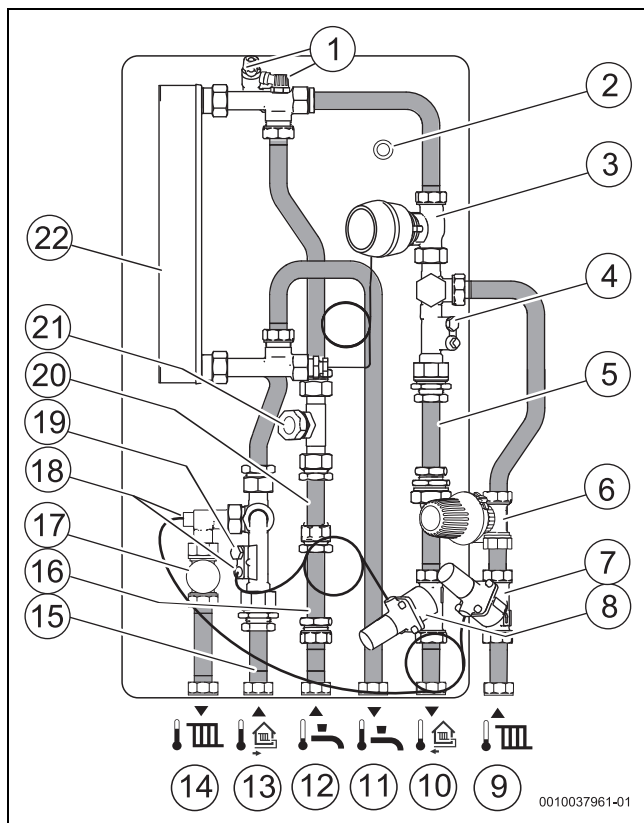
Bild 2 Station
