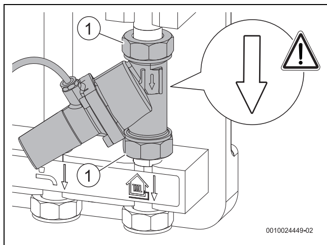
Bild 25 Differenzdruckregler
