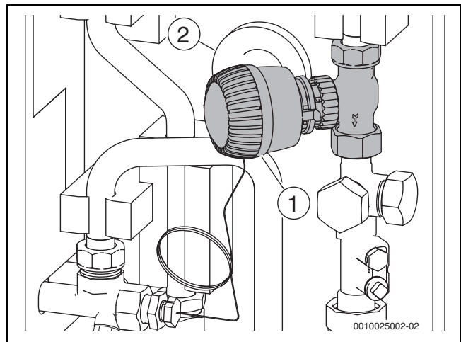
Bild 16 Warmwassertemperatur einstellen
