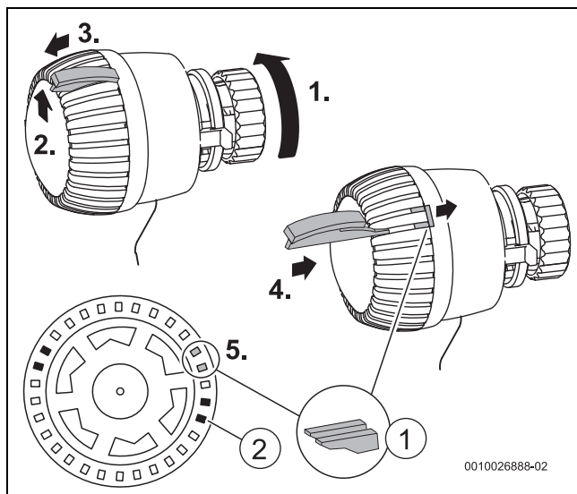
Bild 17 Sperre umsetzen
