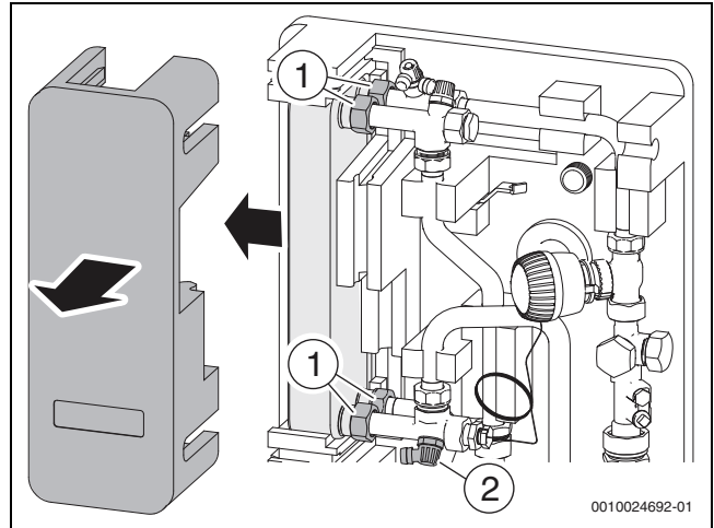
Bild 23 Wärmetauscher demonieren
