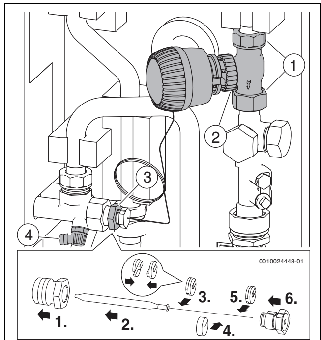
Bild 24 Warmwasserthermostat und Temperaturfühler
