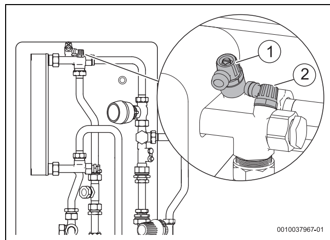
Bild 15 Warmwasser- und Heizkreis entlüften
