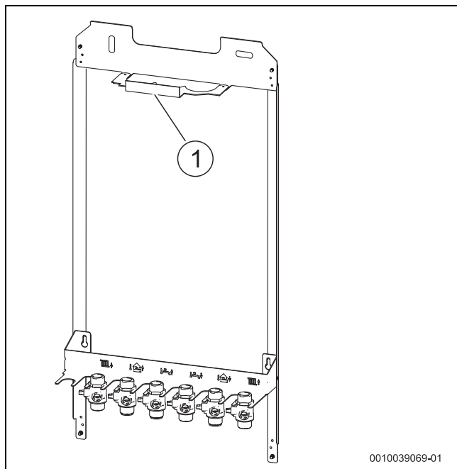
Bild 11 Beispiel Montagerahmen
