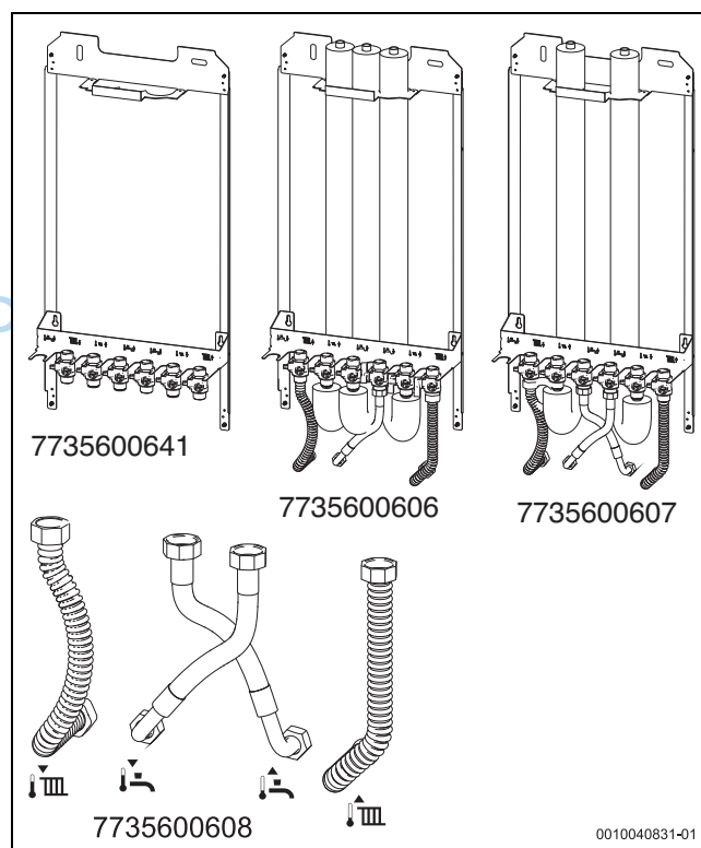
Bild 9 Montagerahmen und Anschluss-Set unten (Installationsanleitungen liegen bei)
