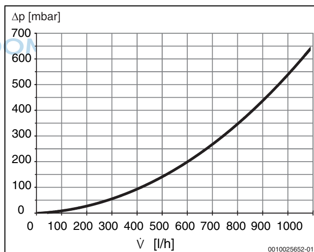
Bild 7 Druckverlust Primärseite
