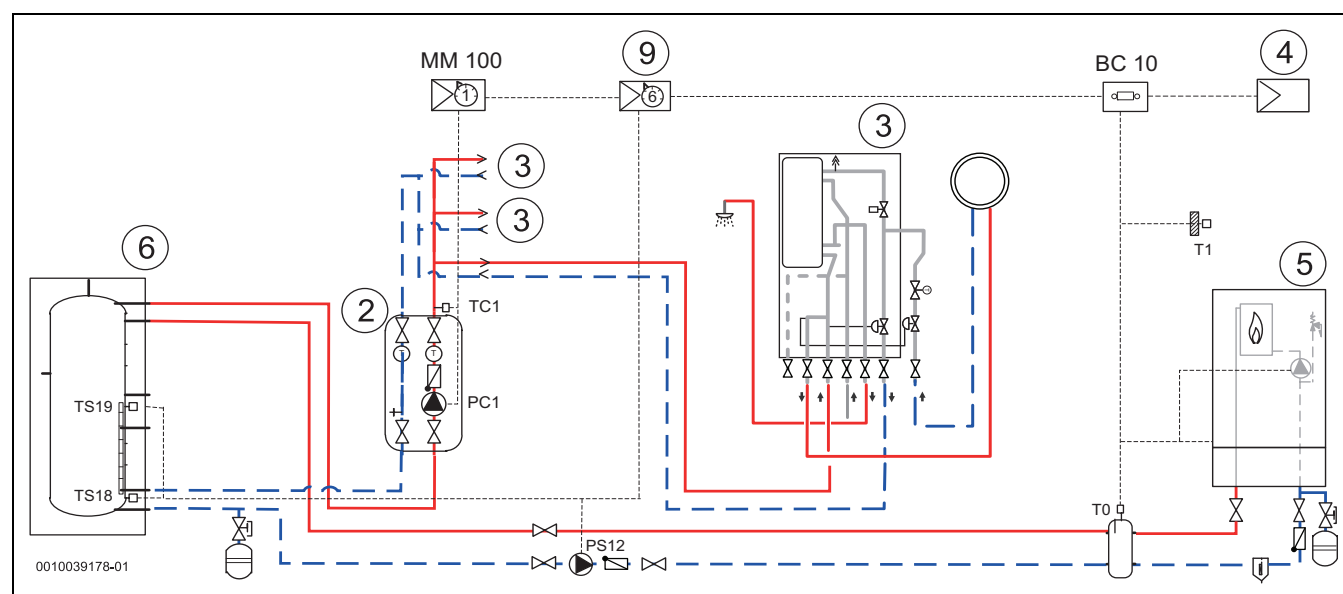
Bild 20 Beispiel 2: Heizgerät mit intelligenter Speicherladung, Wohnungsstation für ungemischte Heizkreisversorgung (Heizkörper)
