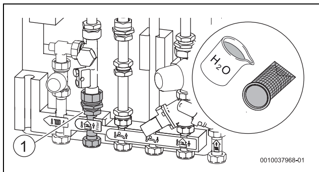
Bild 22 Filter reinigen
