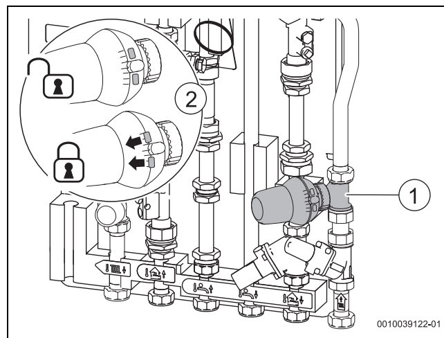
Bild 18 Rücklauftemperaturbegrenzer
