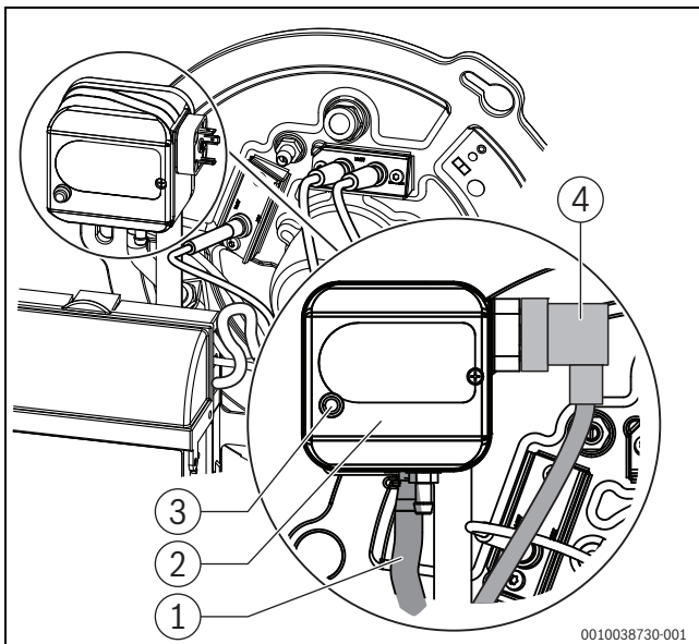
Bild 51 Feuerraum-Druckwächter
