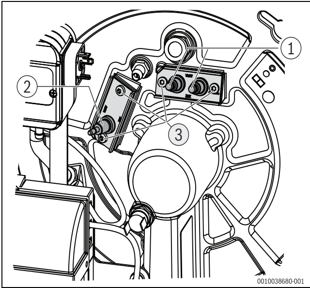
Bild 46 Elektrodenposition
