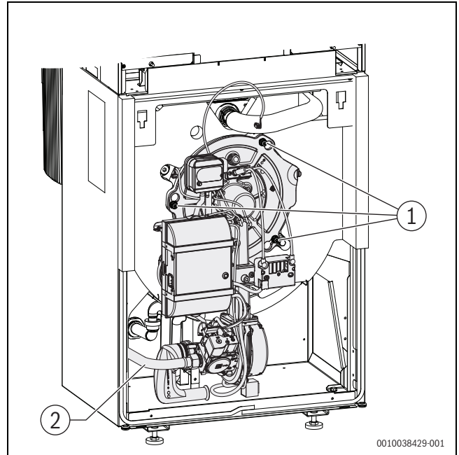
Bild 41 Befestigungsmuttern lösen
