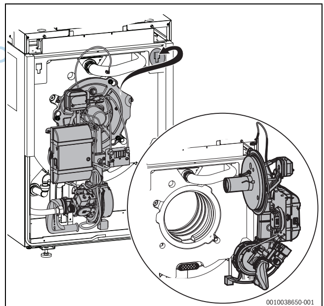
Bild 42 Brenner in Wartungsposition
