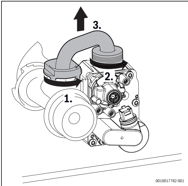
Bild 75 Gasrohr ausbauen
