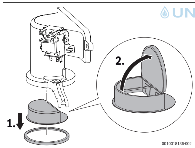
Bild 65 Rückschlagklappe in der Mischeinrichtung
