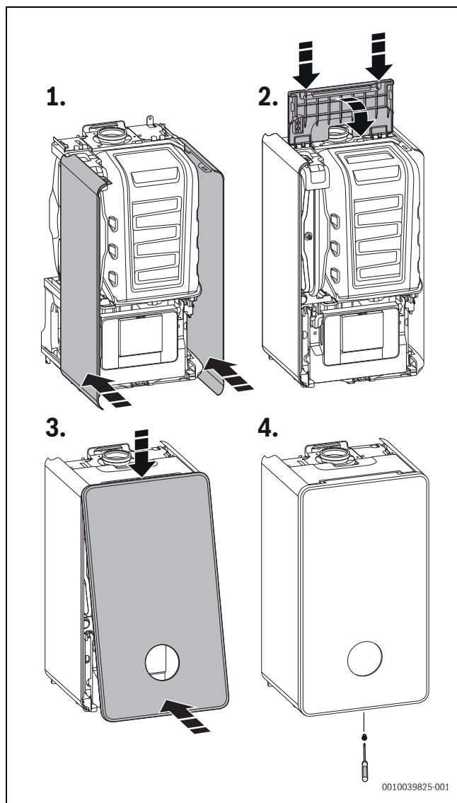
Bild 50 Verkleidung montieren
