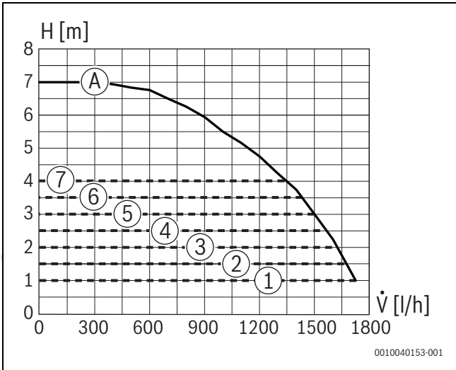
Bild 87 Pumpenkennfelder und Pumpenkennlinien
