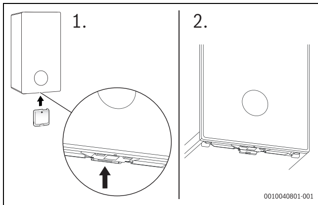
Bild 48 Lage des Steckplatzes
