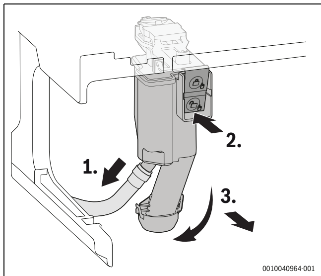
Bild 71 Kondensatsiphon ausbauen
