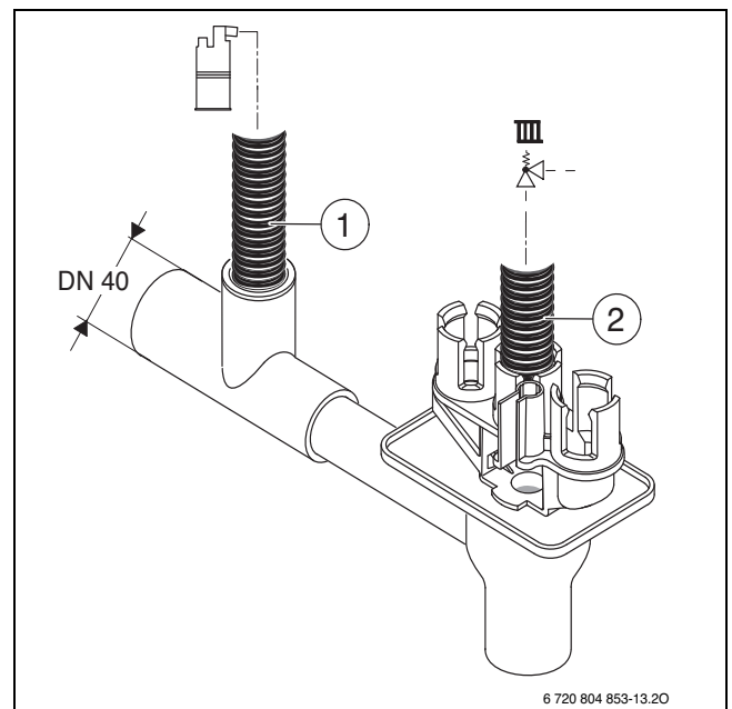
Bild 40 Kondensatschlauch und Schlauch vom Sicherheitsventil am Siphon montieren
