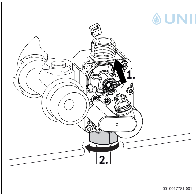
Bild 76 Stecker abziehen und Überwurfmutter lösen
