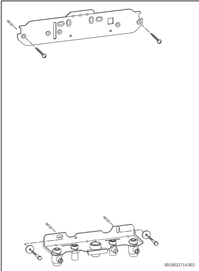
Bild 34 Aufhängeschiene (Zubehör) montieren
