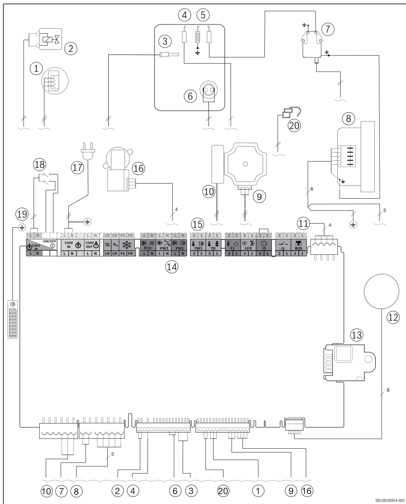
Bild 88 Elektrische Verdrahtung
