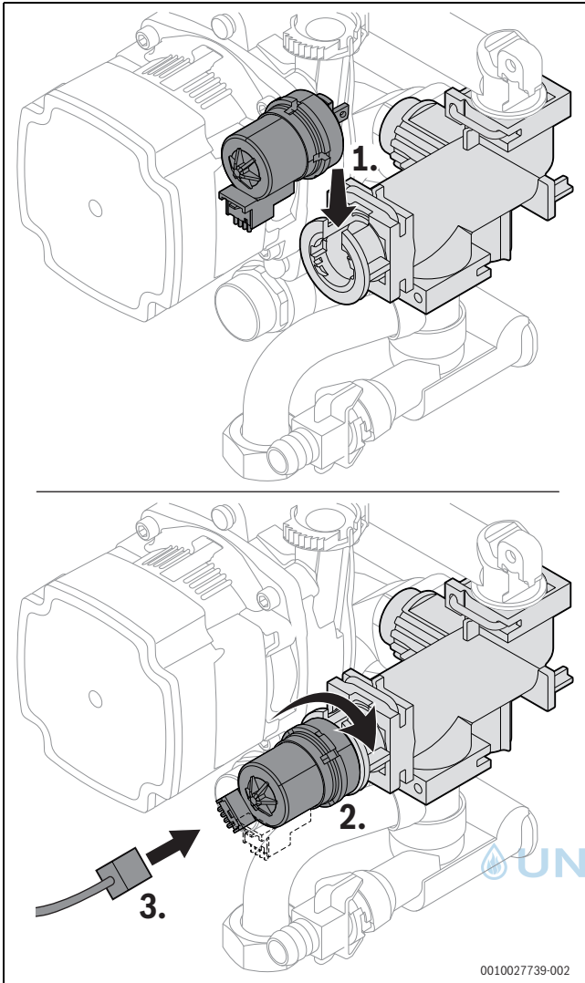
Bild 83 Motor am 3-Wege-Ventil einbauen (Variante ohne Schrauben)
