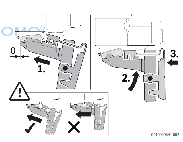
Bild 74 Kondensatsiphon einbauen
