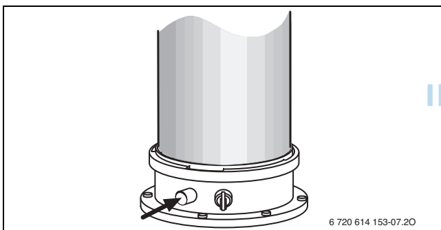
Bild 56 Abgasmessstutzen
