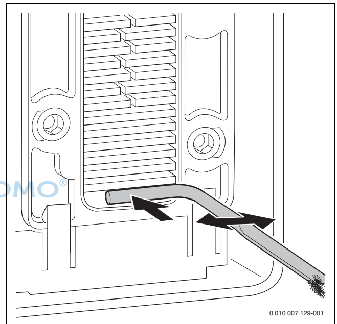
Bild 70 Kondensatwanne reinigen
