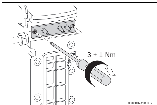
Bild 59 Elektroden-Set montieren
