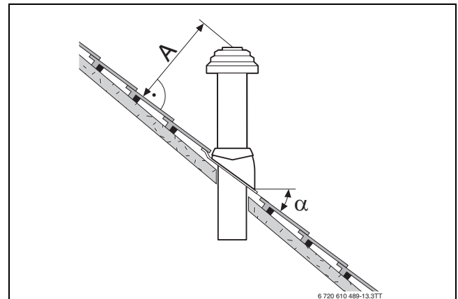
Bild 9 Abstandsmaße und Dachneigungen bei Schrägdach
