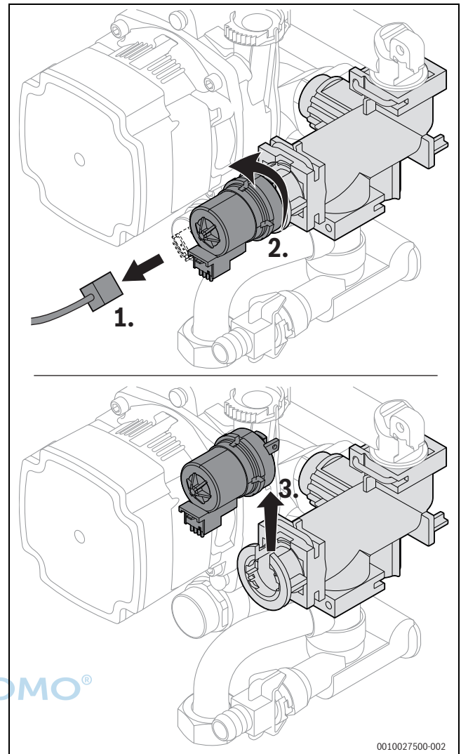
Bild 82 Motor am 3-Wege-Ventil ausbauen (Variante ohne Schrauben)
