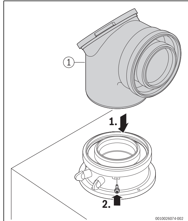
Bild 43 Abgaszubehör einsetzen und mit Schraube sichern
