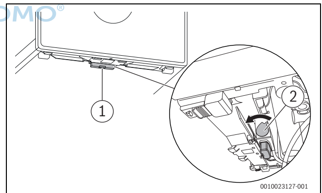
Bild 49 Connect-Key sichern
