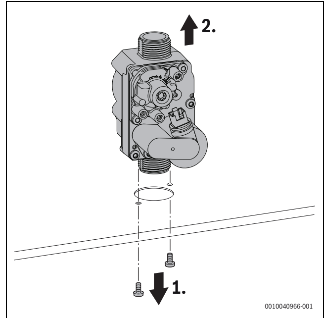
Bild 77 Gasarmatur ausbauen
