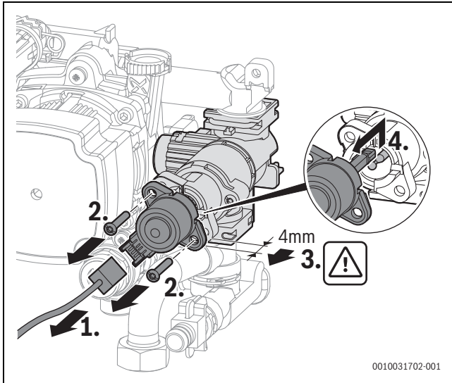
Bild 80 Motor am 3-Wege-Ventil ausbauen (Variante mit Schrauben)
