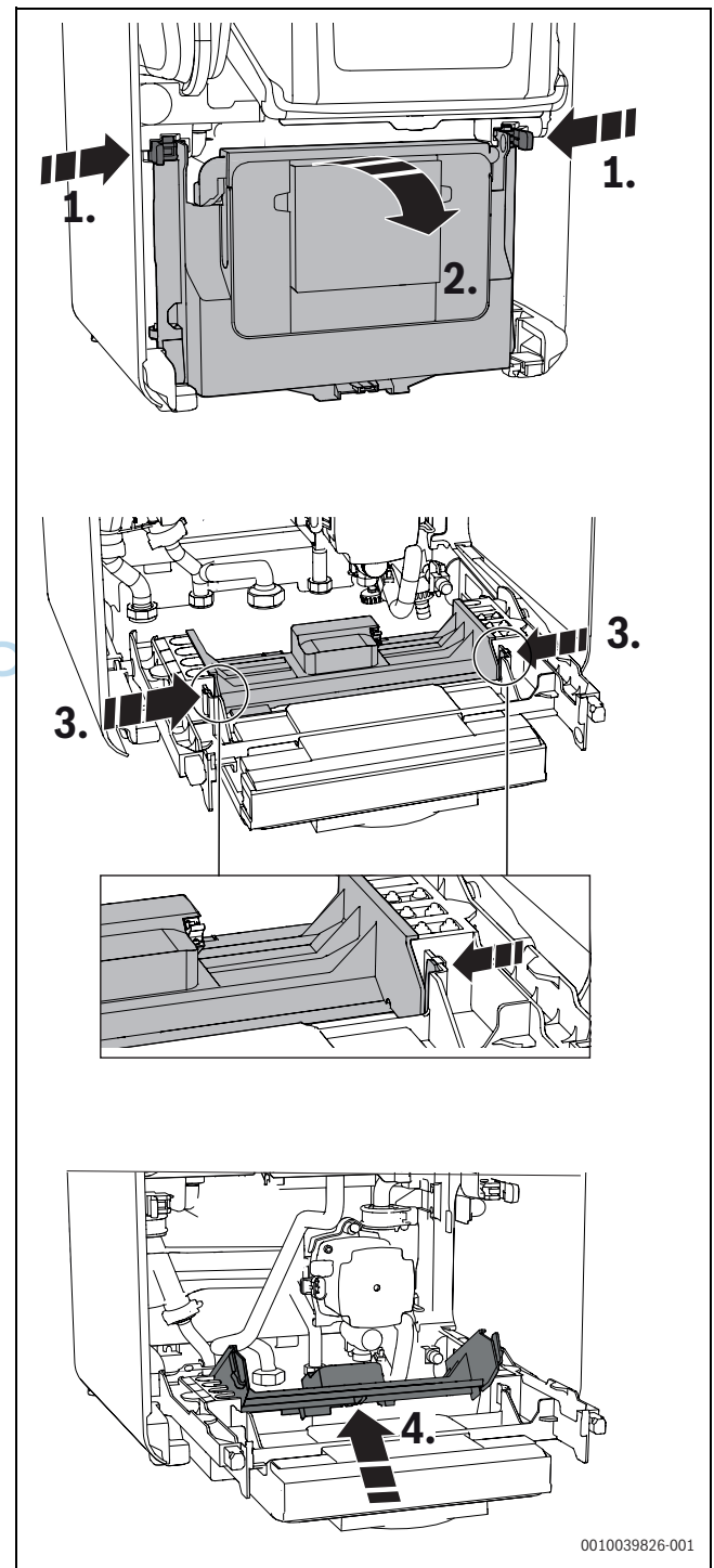
Bild 45 Steuergerät öffnen
