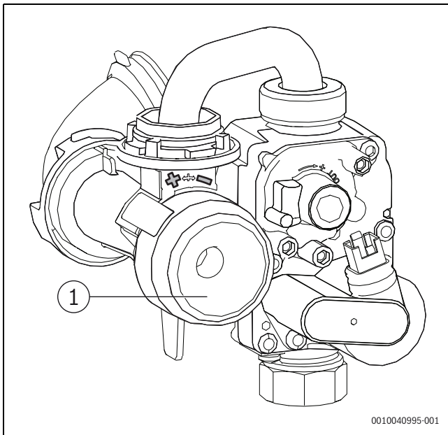
Bild 55 Gas-Luft-Verhältnis einstellen
