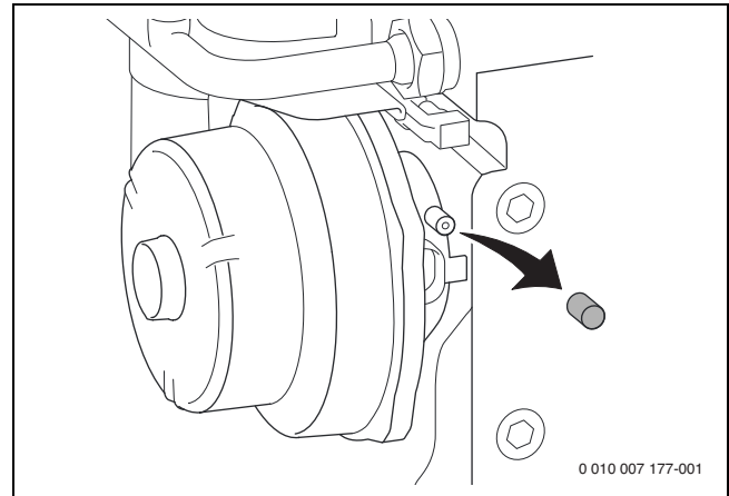
Bild 66 Messstutzen an der Mischeinrichtung
