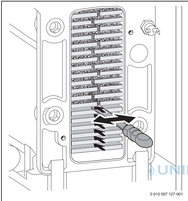
Bild 67 Reinigungsmesser
