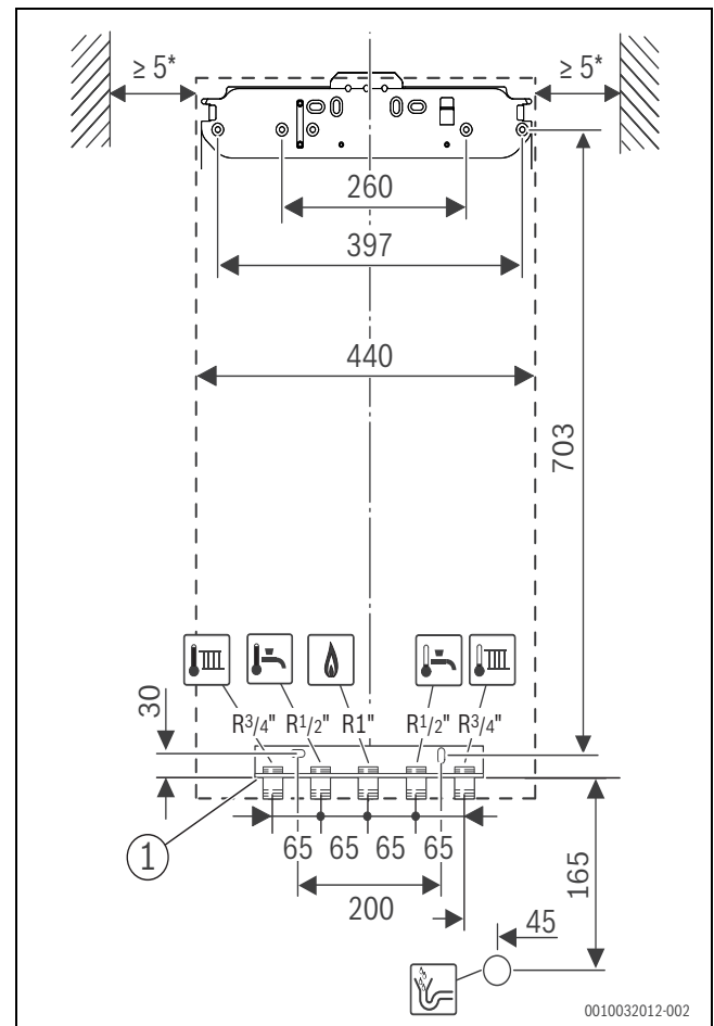
Bild 3 Frontansicht (mm)
