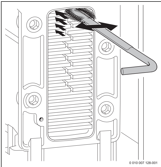
Bild 68 Wärmeblock mit Bürste reinigen
