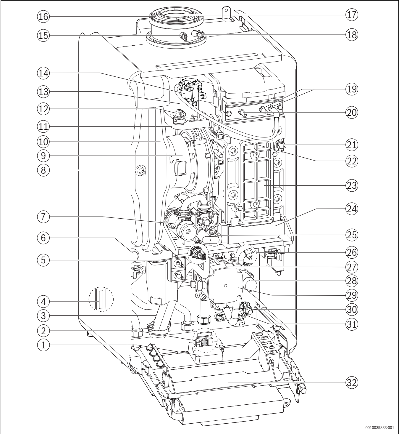
Bild 4 Produktübersicht
