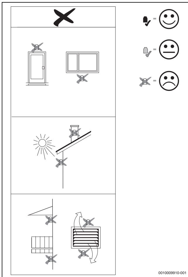
Bild 37 Ungeeigneter Installationsort des Außentemperaturfühlers
