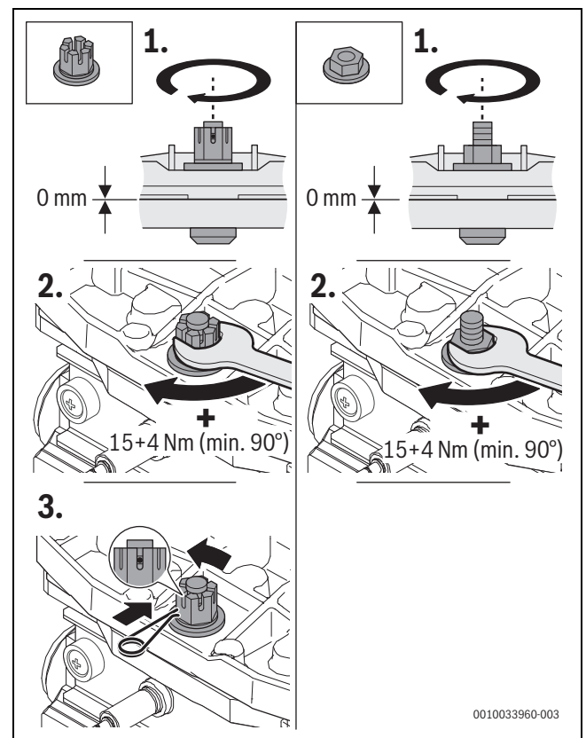
Bild 63 Mutter am Brennerdeckel festziehen
