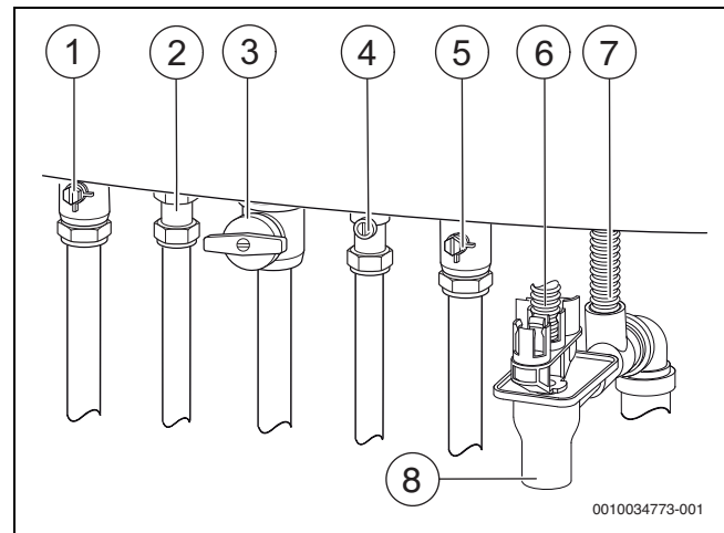
Bild 44 Gas- und wasserseitige Anschlüsse (Zubehör)
