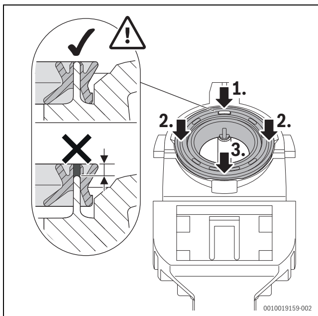
Bild 73 Dichtung andrücken
