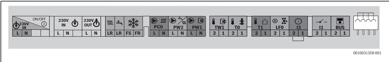
Bild 47 Klemmleiste für externes Zubehör
