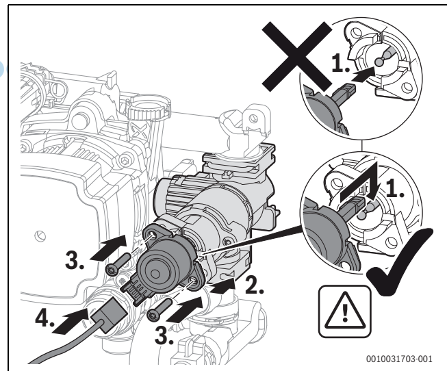
Bild 85 Motor am 3-Wege-Ventil einbauen (Variante mit Schrauben)
