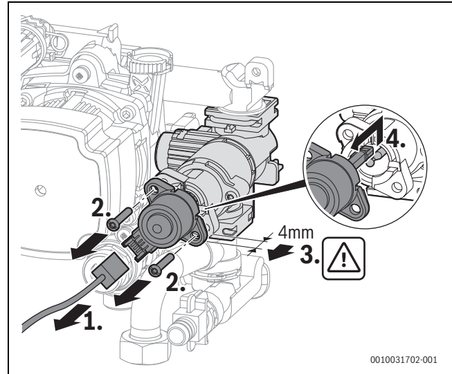
Bild 84 Motor am 3-Wege-Ventil ausbauen (Variante mit Schrauben)
