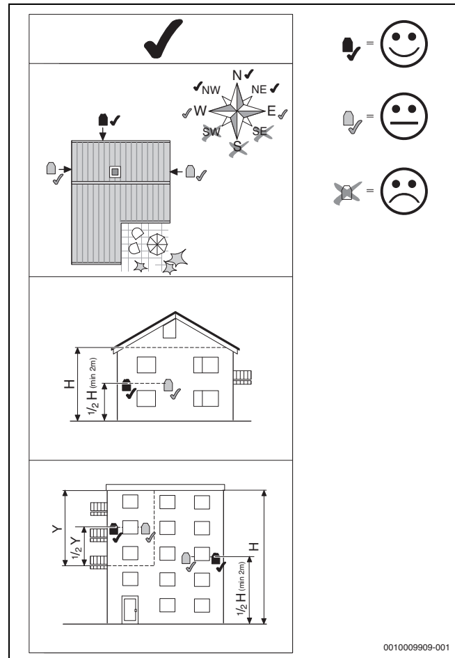
Bild 36 Geeigneter Installationsort des Außentemperaturfühlers
