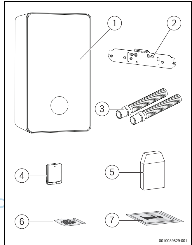
Bild 1 Lieferumfang
