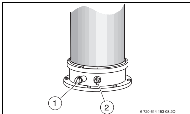
Bild 58 Abgassensstutzen und Verbrennungsluft-Messstutzen
