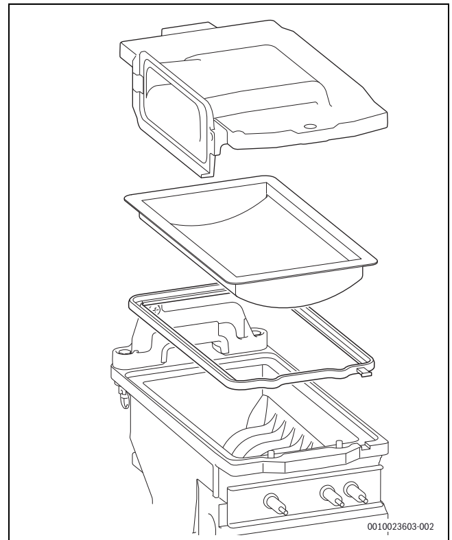
Bild 62 Brenner
