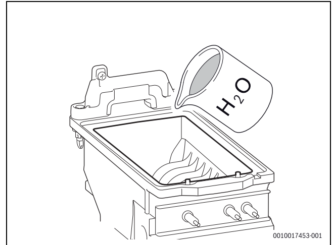
Bild 69 Wärmeblock spülen
