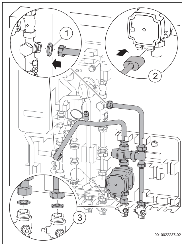
Bild 21 Heizkreismodul montieren
