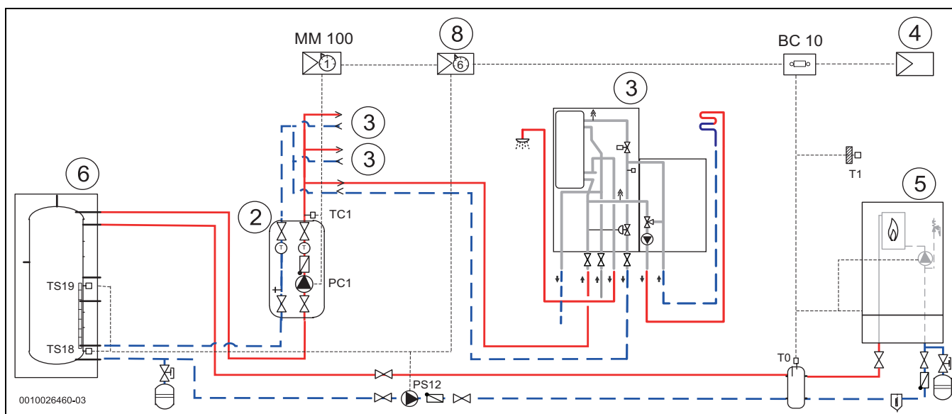
Bild 37 Beispiel 2: Heizgerät mit intelligenter Speicherladung, Wohnstation für gemischte Heizkreisversorgung (Fußbodenheizung)
