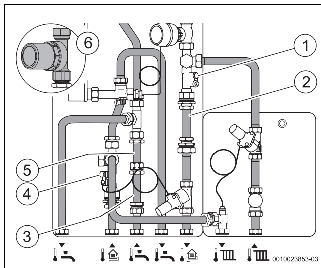
Bild 26 Adapterrohre ersetzen
