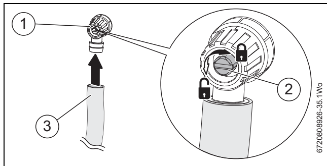
Bild 38 Entleerungsanschluss
