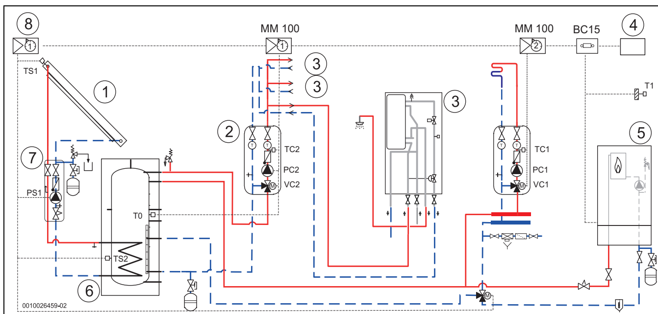
Bild 36 Beispiel 1: Heizgerät mit Solaranlage, Wohnstation als dezentrale Frischwasserstation
