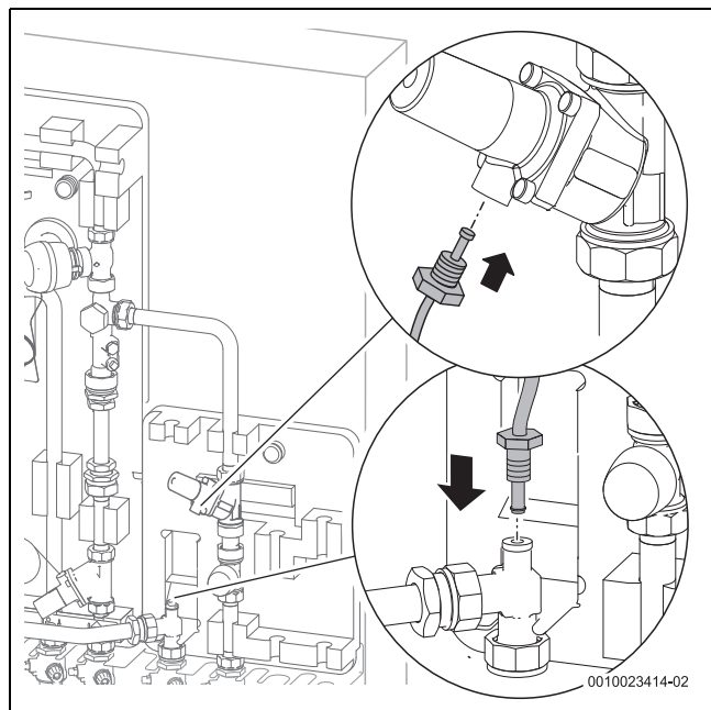
Bild 24 Kapillarleitung montieren
