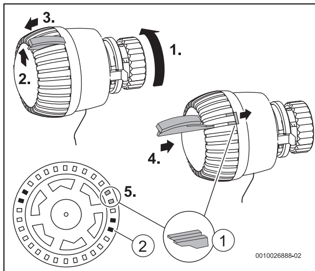
Bild 29 Sperre umsetzen
