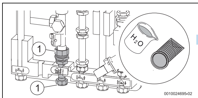
Bild 39 Filter reinigen
