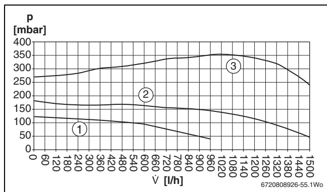
Bild 34 Restförderhöhe
