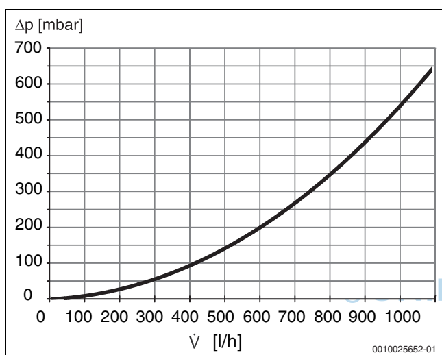
Bild 7 Druckverlust Primärseite
