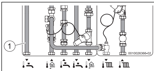
Bild 15 Kaltwasserabgang anschließen oder demontieren
