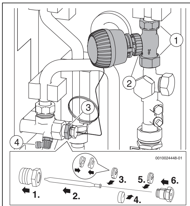
Bild 41 Warmwasserthermostat und Temperaturfühler
