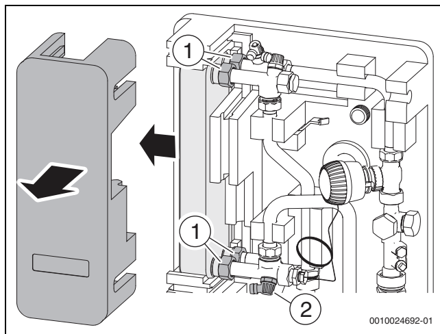
Bild 40 Wärmetauscher demontieren
