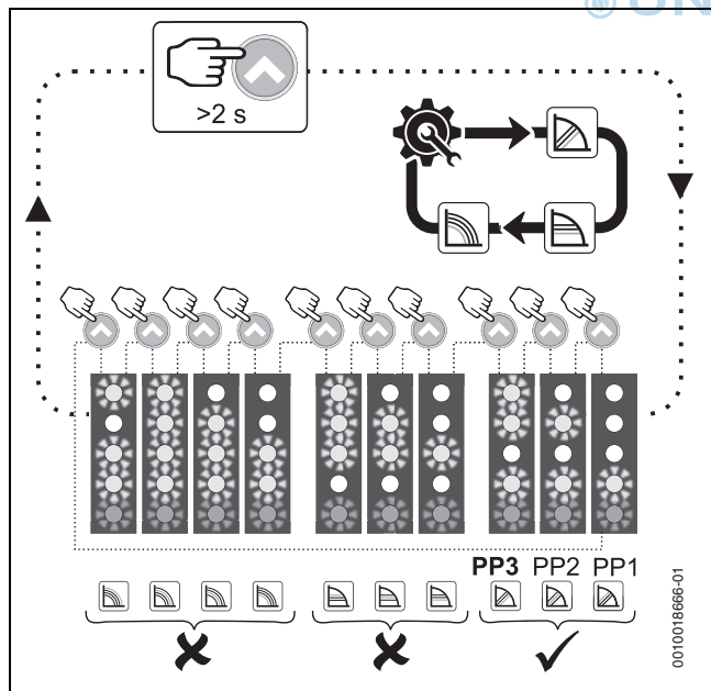
Bild 35 Einstellung der Pumpenkennlinie
