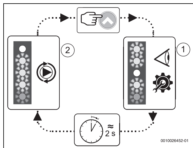
Bild 33 Betriebs- und Anzeige Pumpenkennlinie
