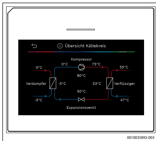
Bild 10 Übersicht Kältekreis
