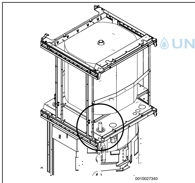
Fig. 35 Démontage des tubes
