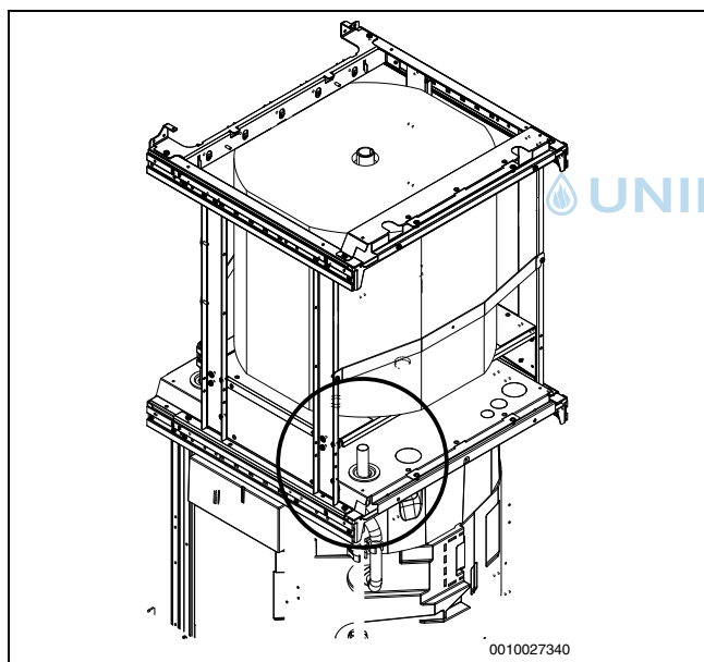
Bild 8 Demontage von Rohren
