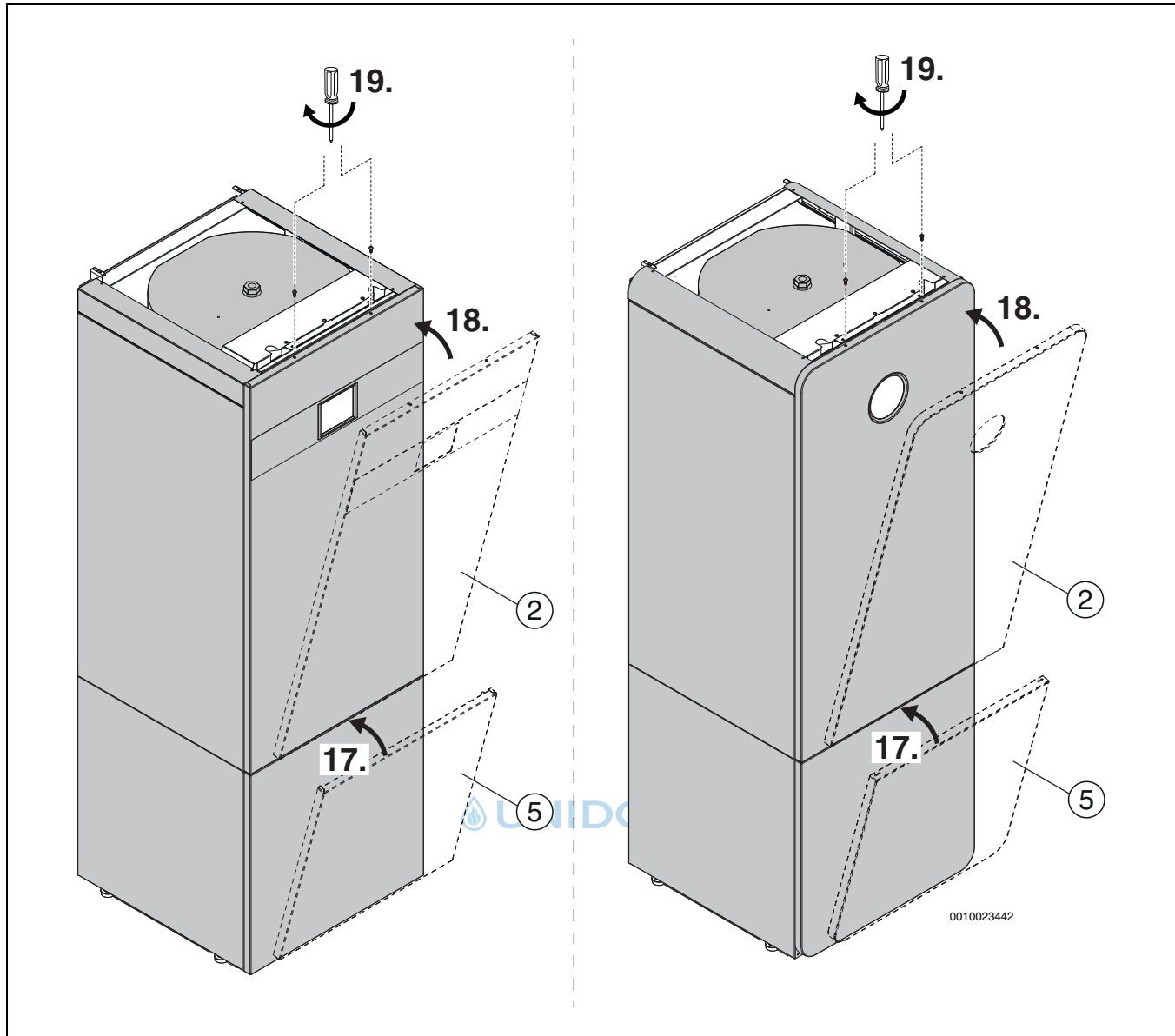
Fig. 53 Montage des panneaux avant avec cache carré ou rond
