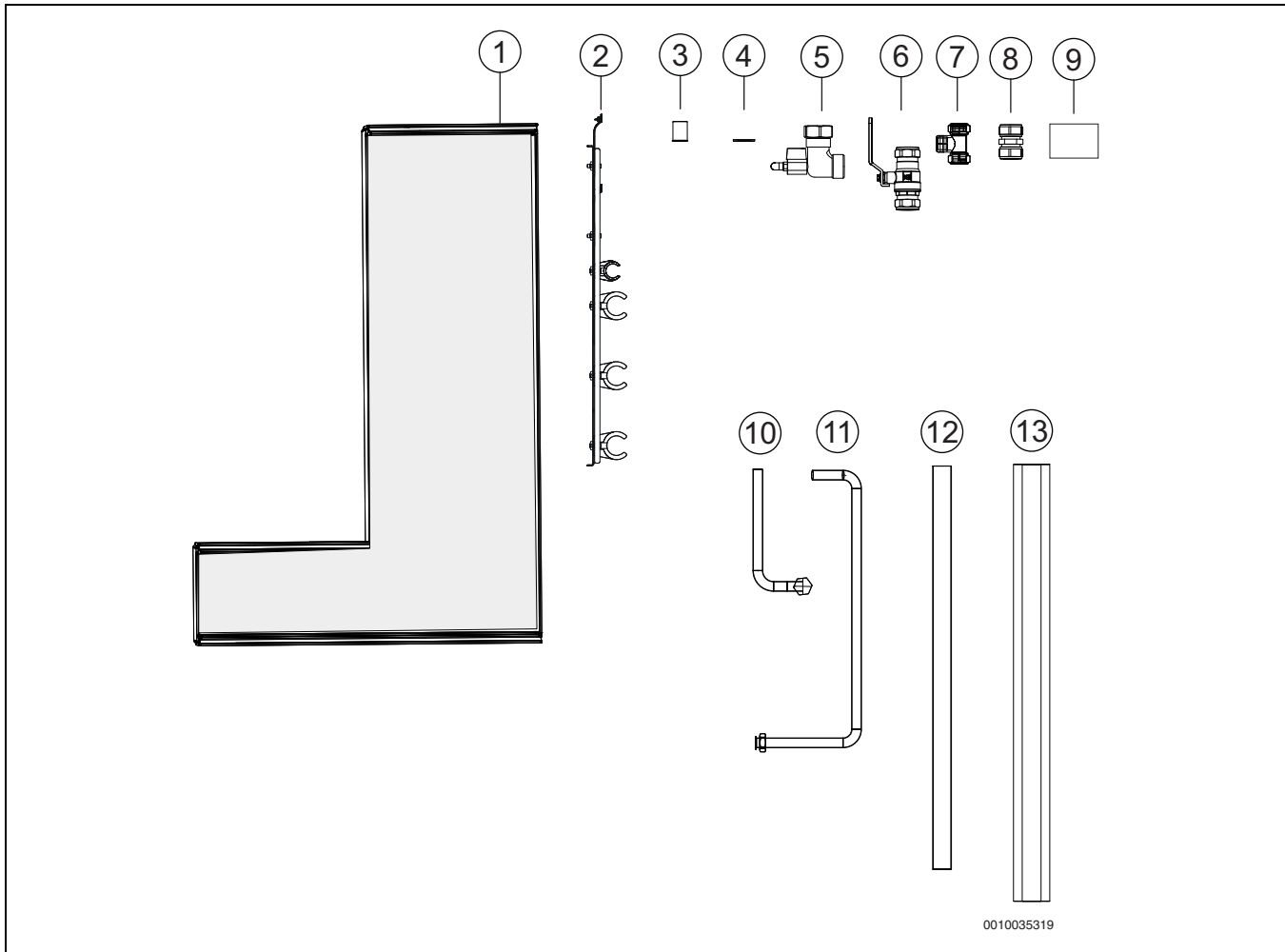
Bild 3 Anschlusssatz Pufferspeicher – Wärmepumpe
