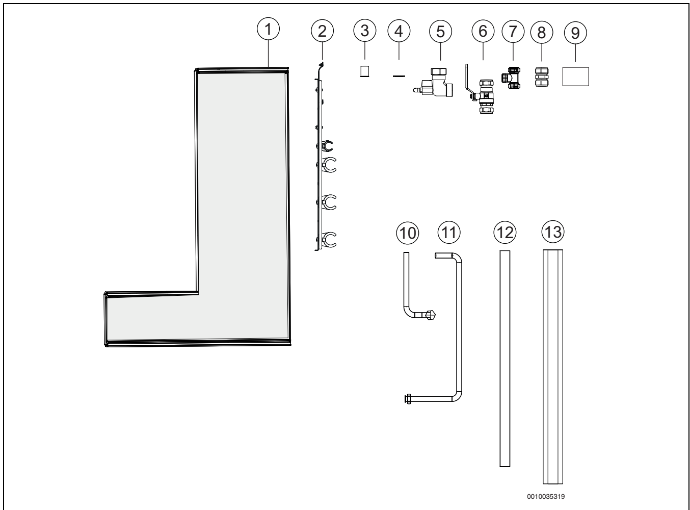
Afb. 84 Aansluitset buffervat – warmtepomp
