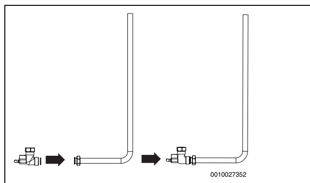
Bild 11 Ablaufrohr (Nr. 12)
