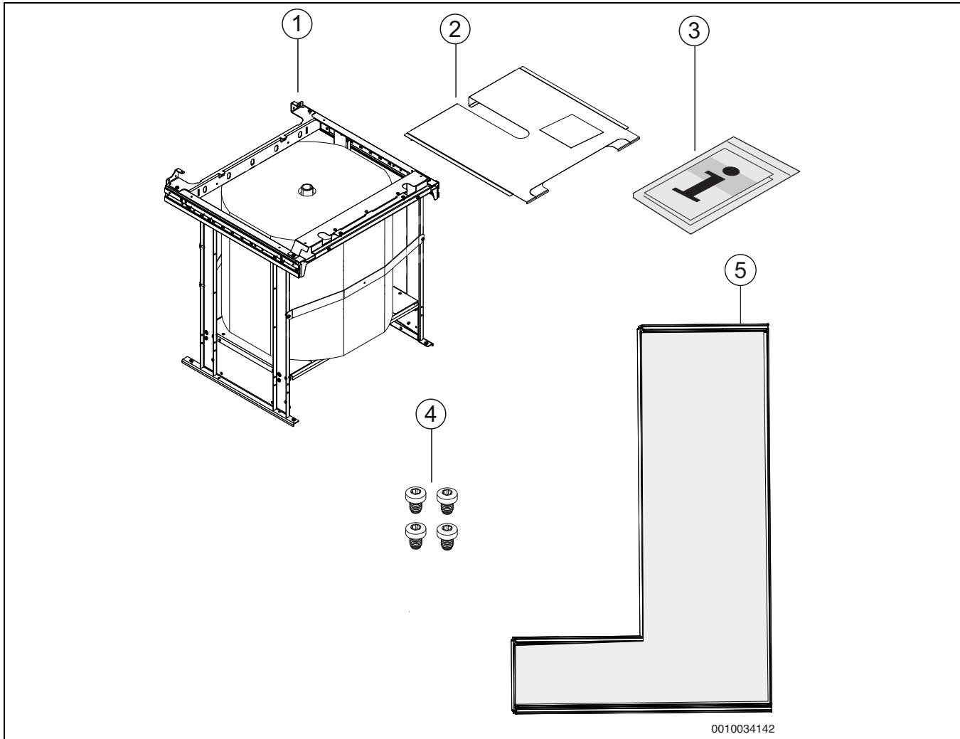
Bild 1 Lieferumfang
