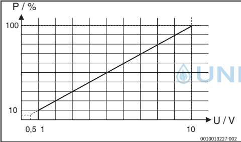
Fig. 1 Relación lineal entre la señal 0-10 V (U en V) y la potencia solicitada (P en porcentaje)
