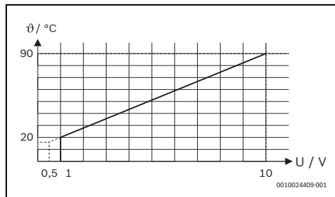
Afb. 2 Lineaire relatie tussen 0-10 V-sigitaal (U in V) en gevraagde aanvoertemperatuur (θ in °C)
