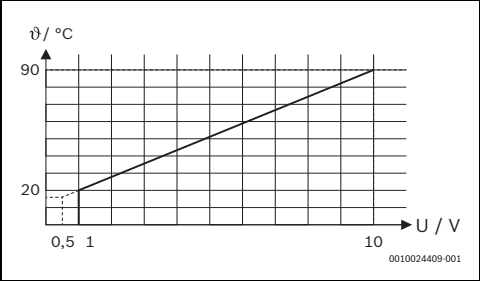
Fig. 2 Relación lineal entre la señal 0-10 V (U en V) y la temperatura de impulsión requerida (9 en °C)
