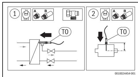
Rys. 4 Optimalny montaż czujnika
