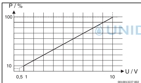
Afb. 1 Lineaire relatie tussen 0-10 V-sigitaal (U in V) en gevraagde vermogen (P in %)
