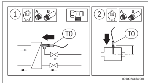
Bild 4 Optimierte Fühlermontage
