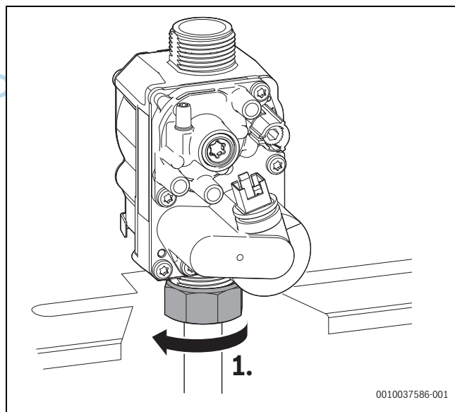
Bild 41 Überwurfmutter lösen
