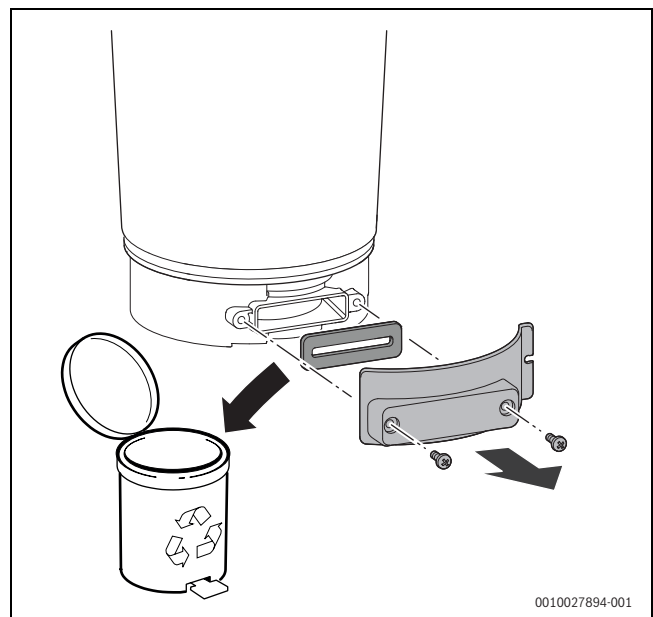
Bild 30 Prüfföffnung öffnen
