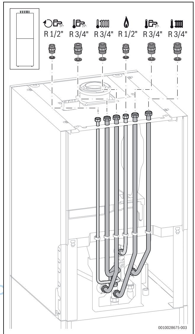
Bild 93 Zubehör CS 33 nach Abschluss der Installation
