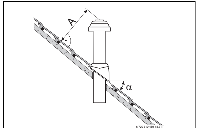
Bild 25 Abstandsmaße und Dachneigungen bei Schrägdach
