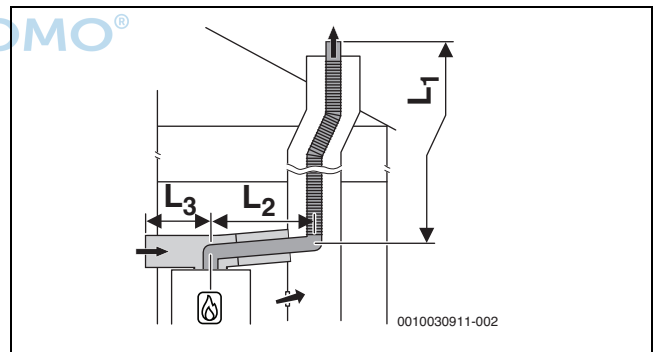
Bild 32 Flexible Abgasführung nach C 53x im Schacht und Luft-Abgas-Führung mit separater Luftzufuhr und konzentrischer Abgasableitung im Aufstellraum
