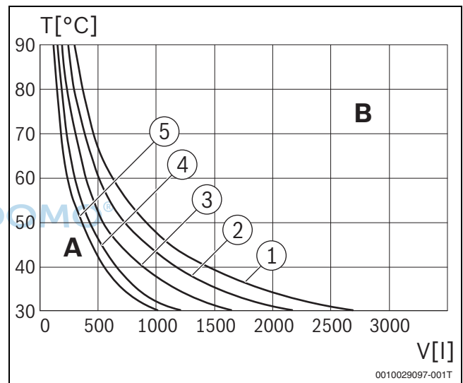
Bild 50 Kennlinien für Ausdehnungsgefäß (29 l)
