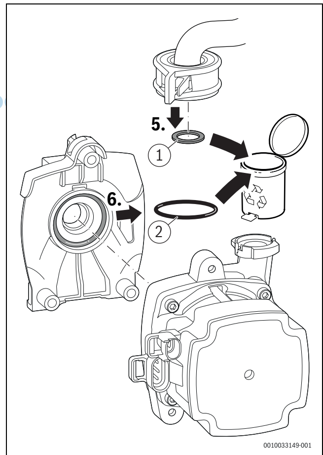
Bild 38 Dichtungen entsorgen
