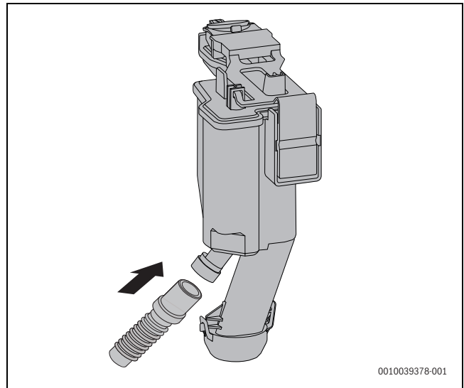
Bild 78 Schlauch am Kondensatsiphon anschließen
