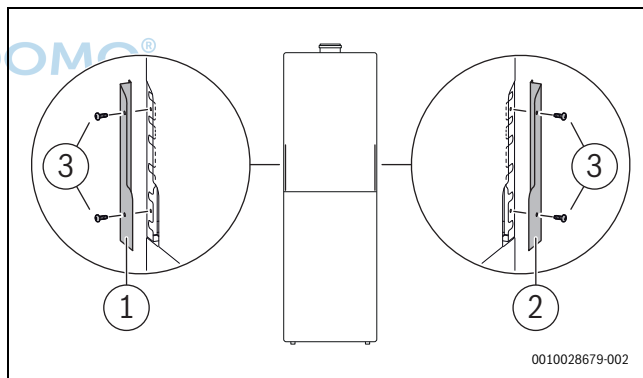
Bild 97 Zubehör SF 11 befestigen
