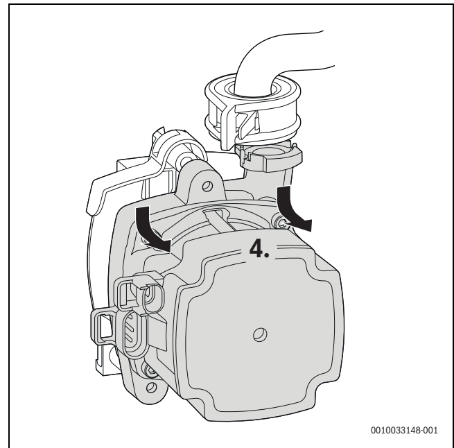
Bild 37 Heizungspumpe abnehmen
