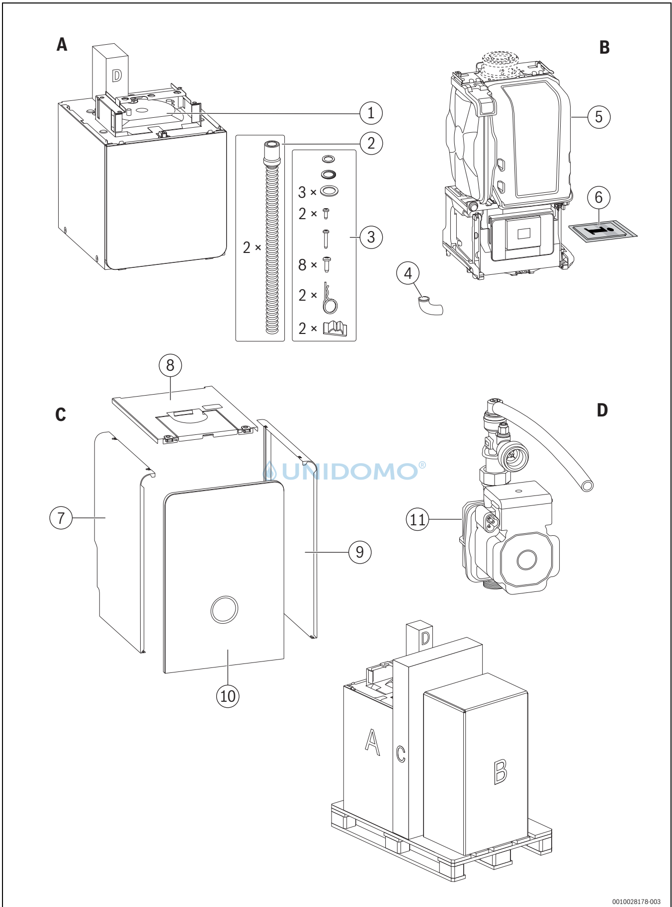
Bild 4 Lieferumfang
