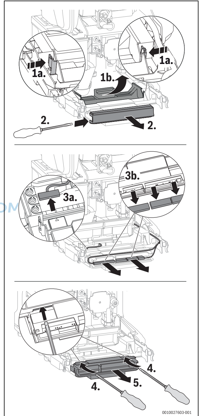
Bild 47 Steuergerät herausnehmen
