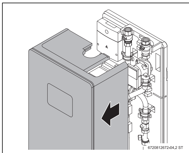
Bild 3 Vorderen Wärmeschutz entfernen
