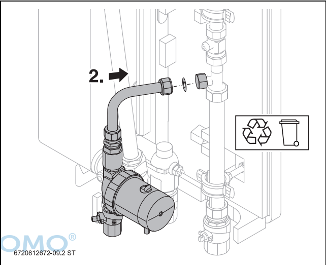
Bild 21 Zirkulationsstrang montieren
