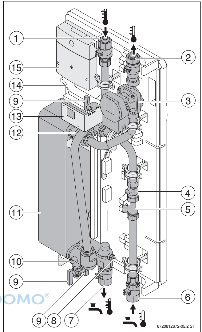
Bild 2 Frischwasserstation ohne vorderen Wärmeschutz
