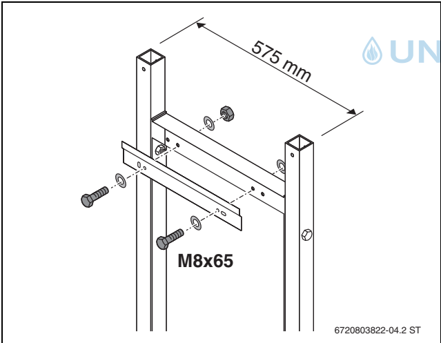
Bild 20 Wandhalter montieren
