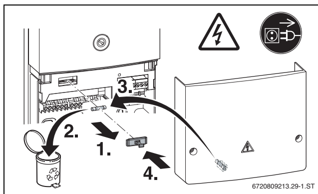
Bild 59 Sicherung tauschen
