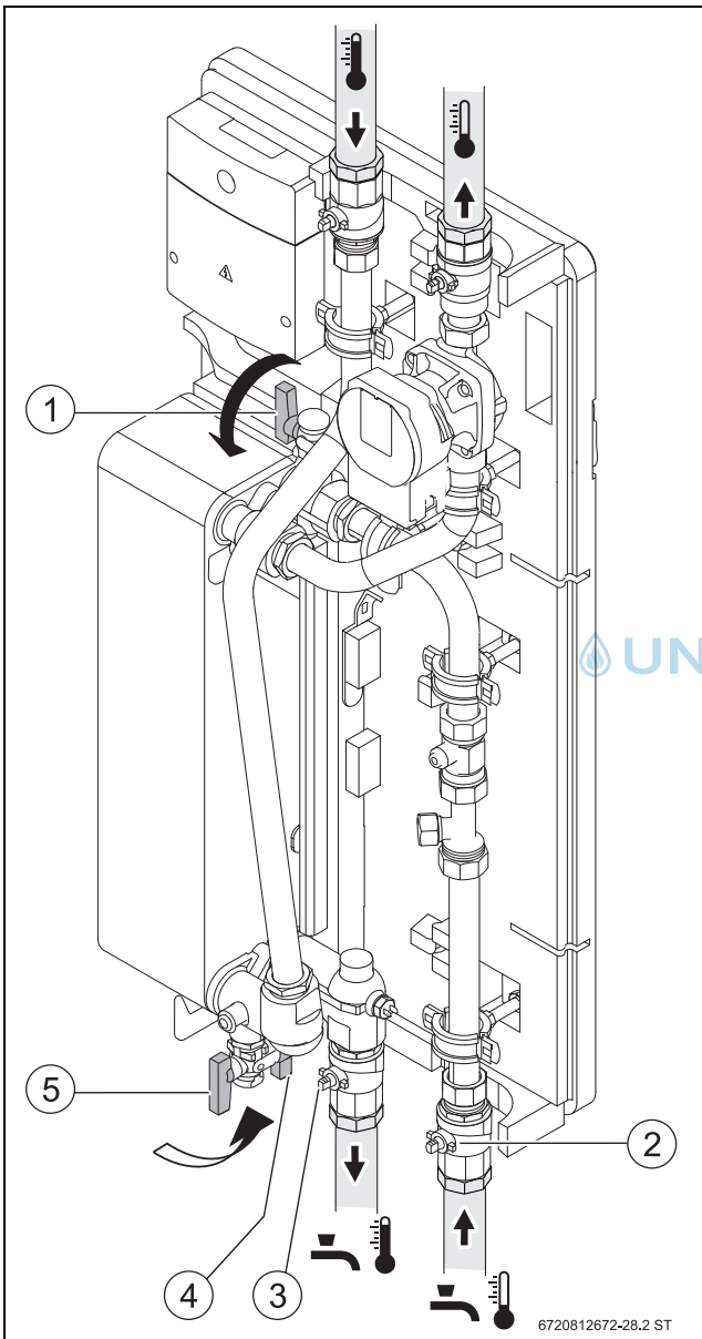
Bild 49 Spül-/Befüllanlagen an der Einzelstation
