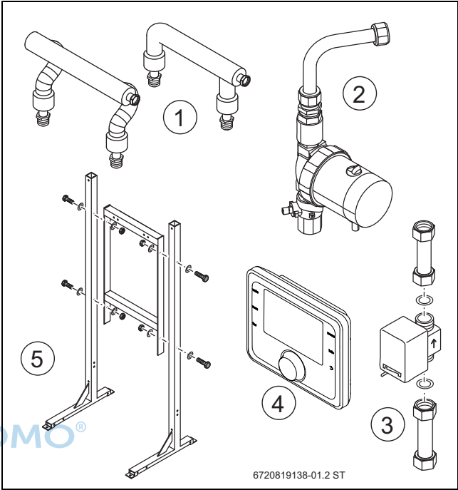
Bild 15 Zubehör für die Frischwasserstationen
