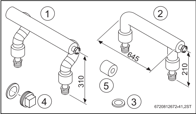
Bild 29 Lieferumfang Verrohrungssatz
