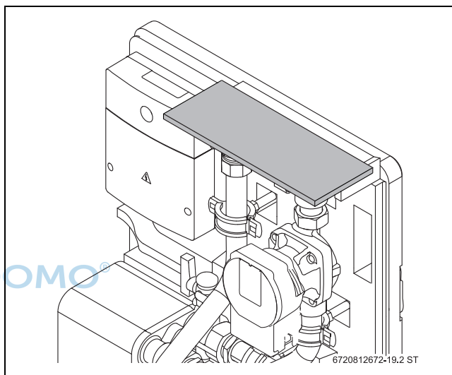
Bild 16 Anschlüsse oben während der Montagearbeiten abdecken
