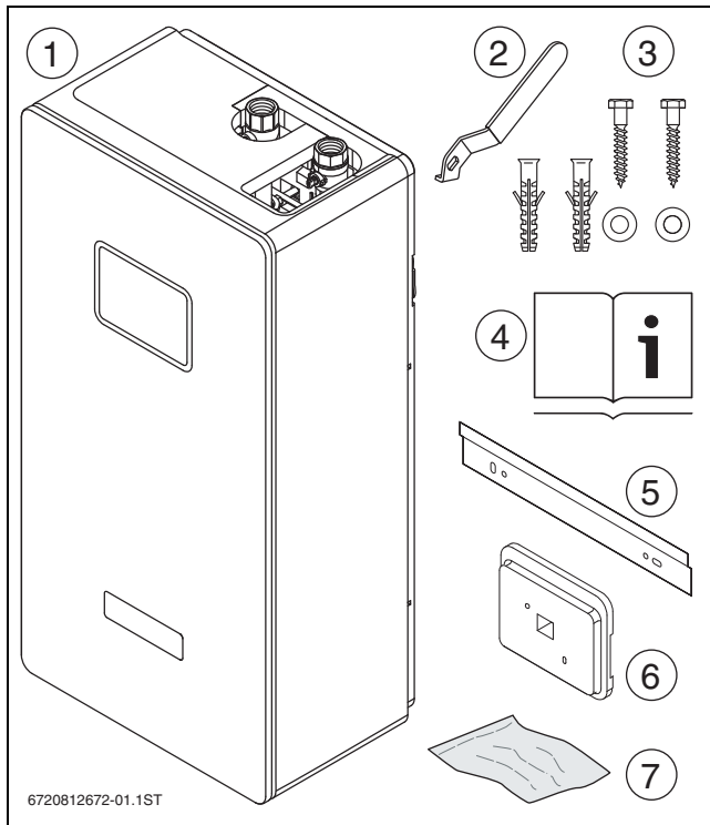
Bild 1 Lieferumfang Einzelstation
