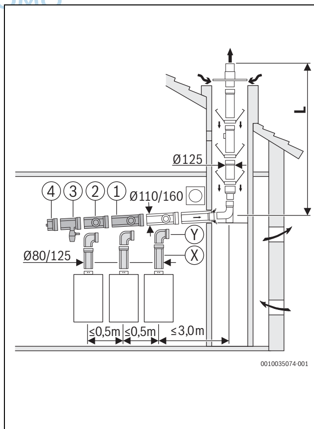
6 V2: DN110/160 - DN125
