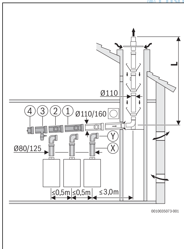
5 V2: DN110/160 - DN110
