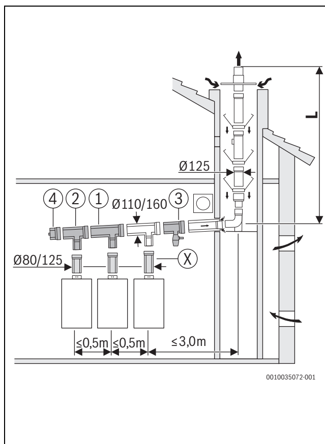
4 V1: DN110/160 - DN125
