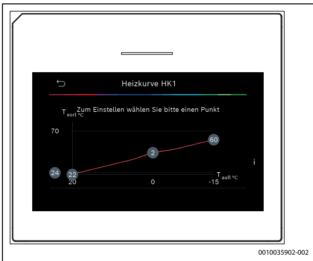
Bild 4 Komfortpunkt einstellen (Krümmung der Heizkurve)
