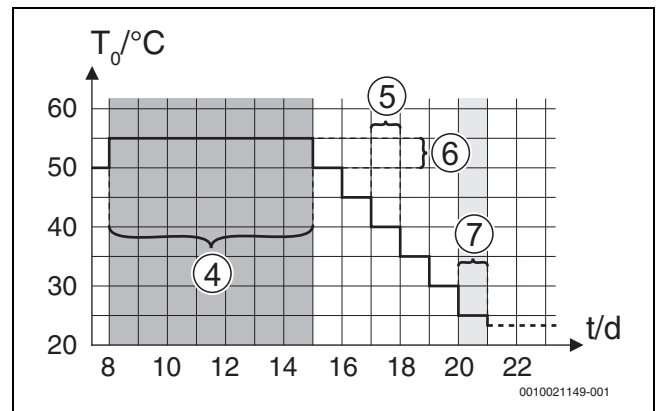
Bild 6 Ablauf der Estrichtrocknung mit den Grundeinstellungen in der Abkühlphase
