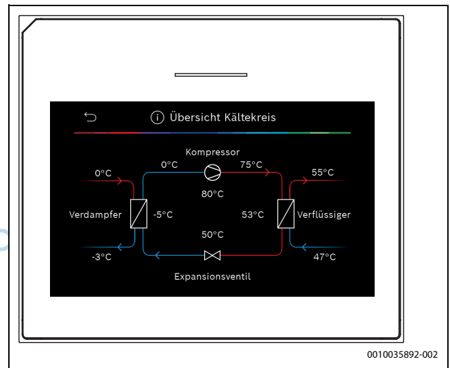
Bild 8 Übersicht Kältekreis
