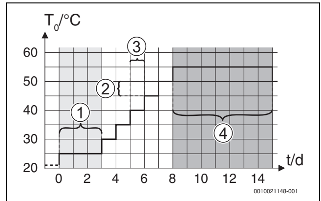
Bild 5 Ablauf der Estrichtrocknung mit den Grundeinstellungen in der Aufheizphase
