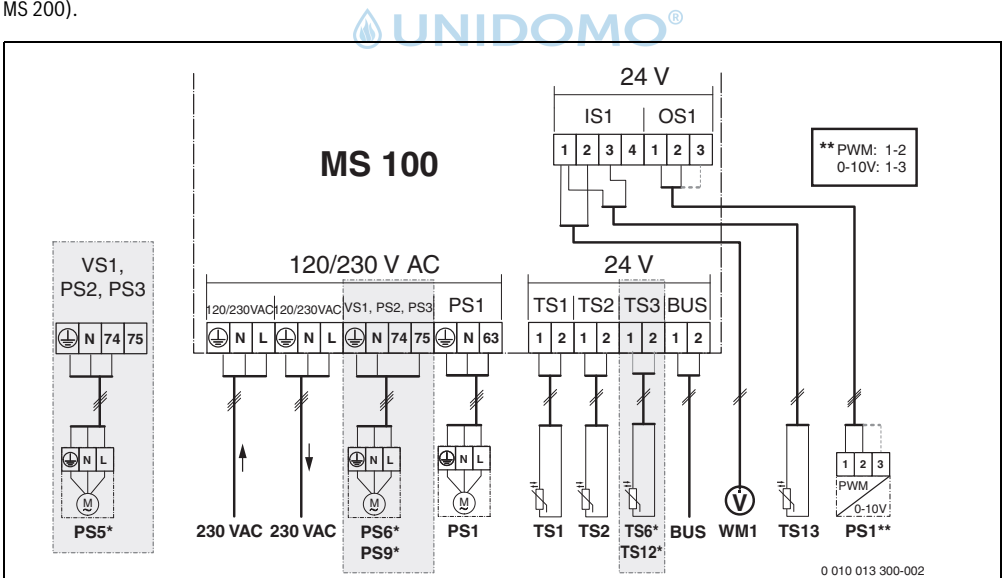
Bild 1 Anschlussklemmenbelegung für Solaranlage
