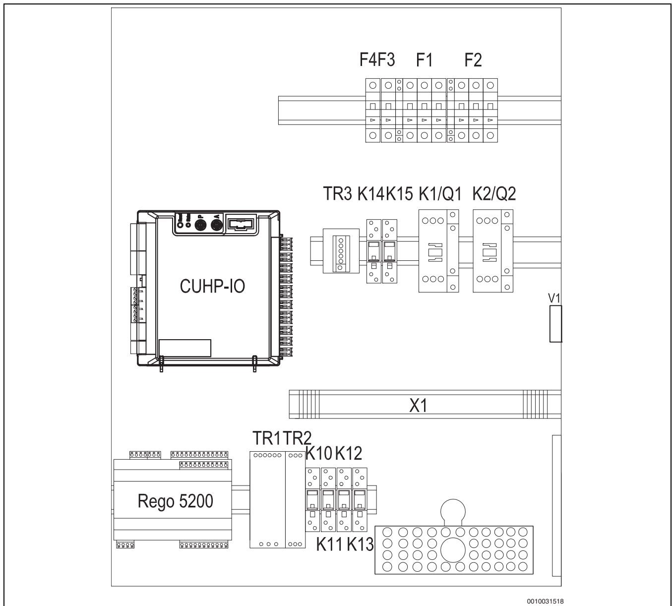
Bild 36 Übersicht Klemmenkasten 38–48 kW
