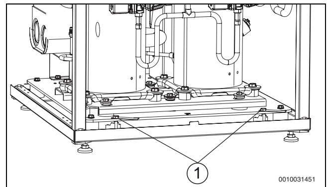
Bild 8 Transportsicherungen
