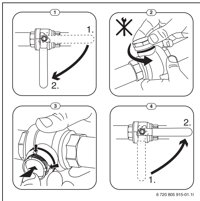
Bild 22 Siebreinigung
