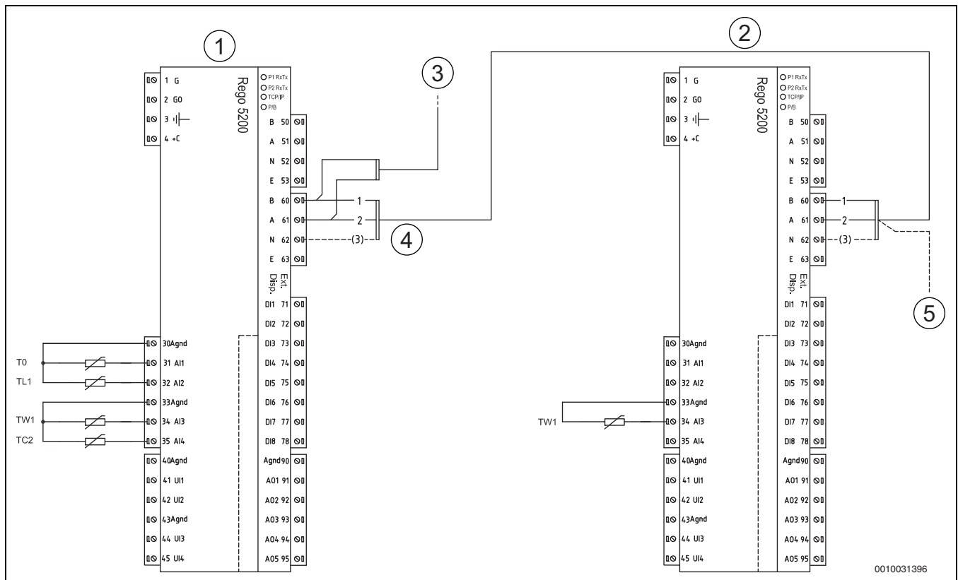
Bild 49 Schaltplan Kaskadenschaltung
