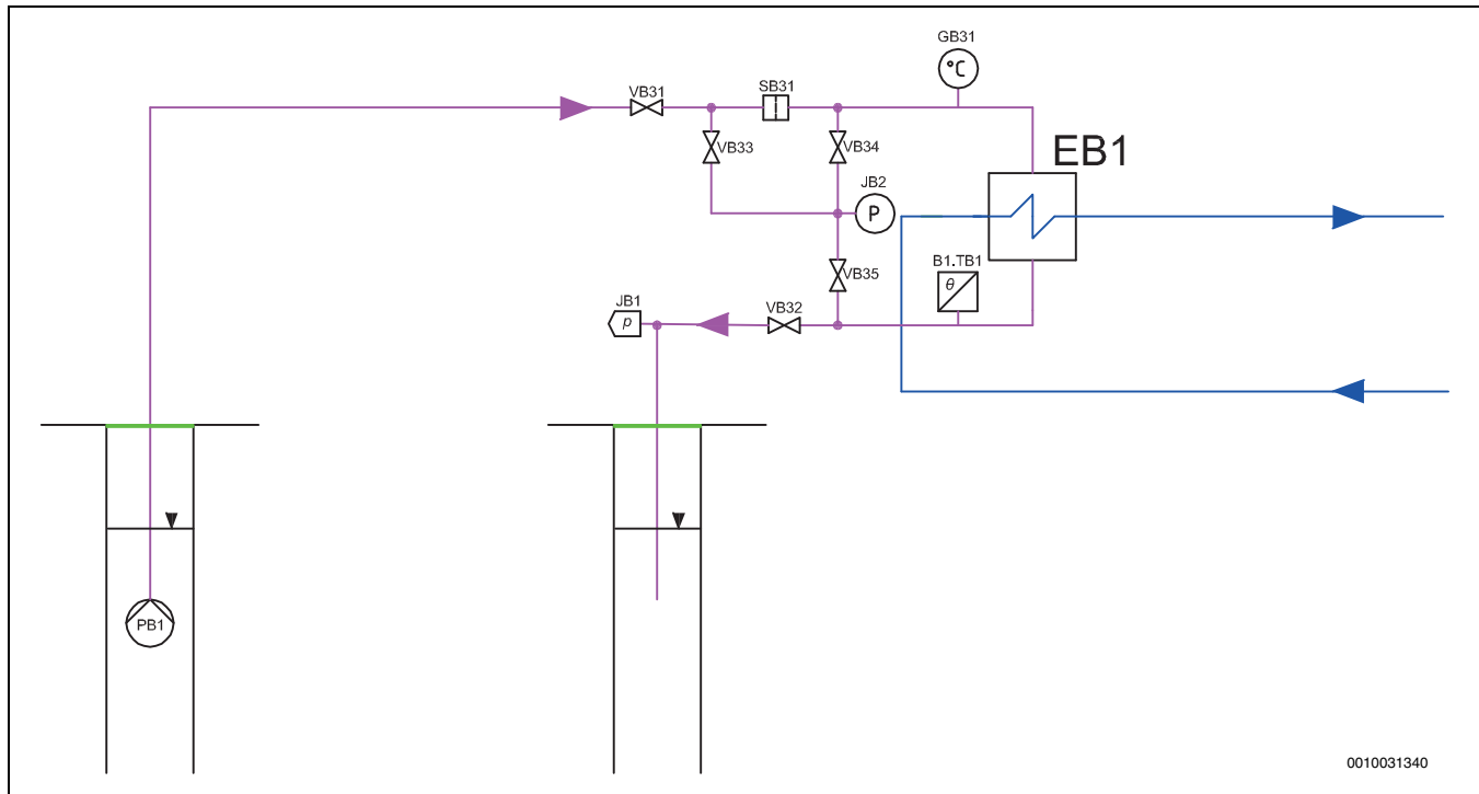
Bild 54 Grundwassersystem
