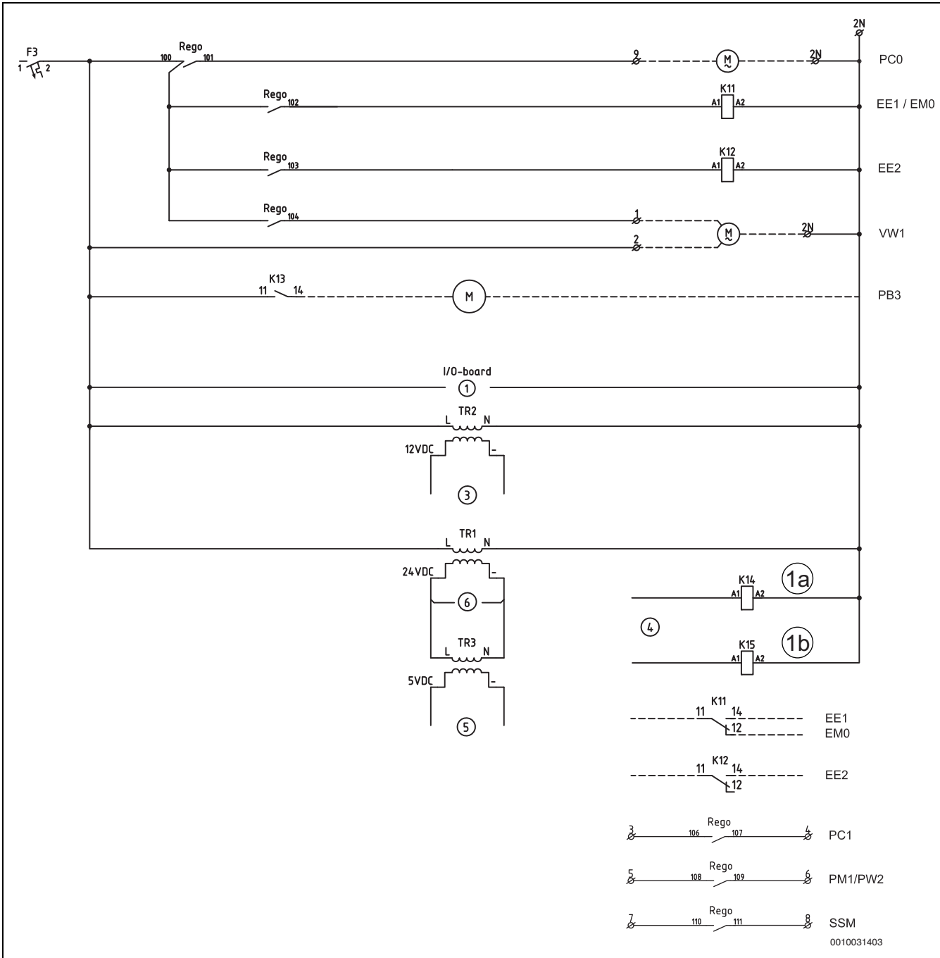
Bild 30 Schaltplan Wärmepumpe
