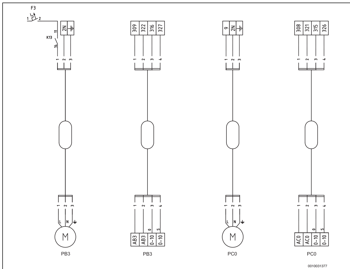
Bild 32 Anschluss Solekreispumpe/Heizkreispumpe
