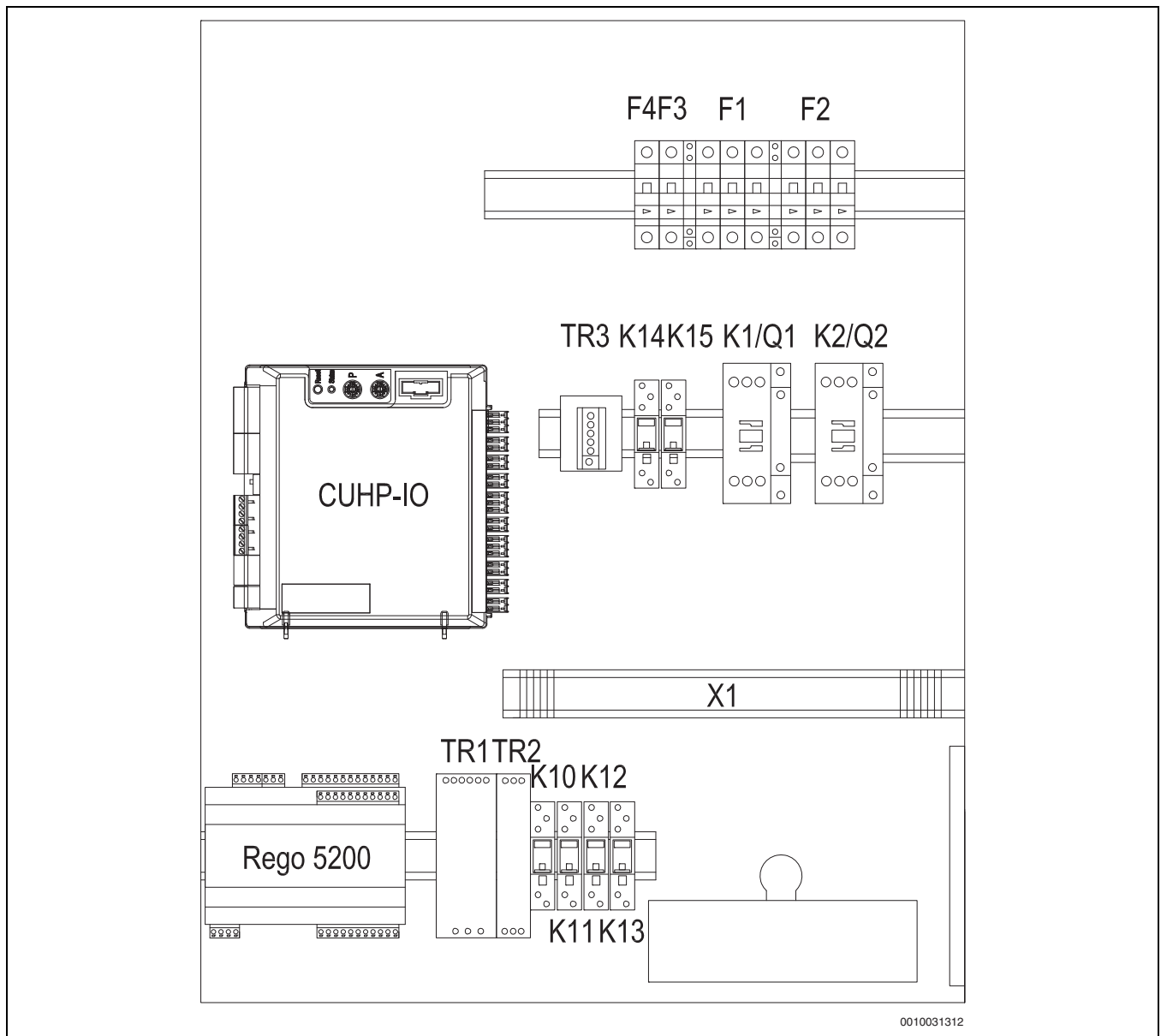
Bild 18 Überblick Klemmenkasten
