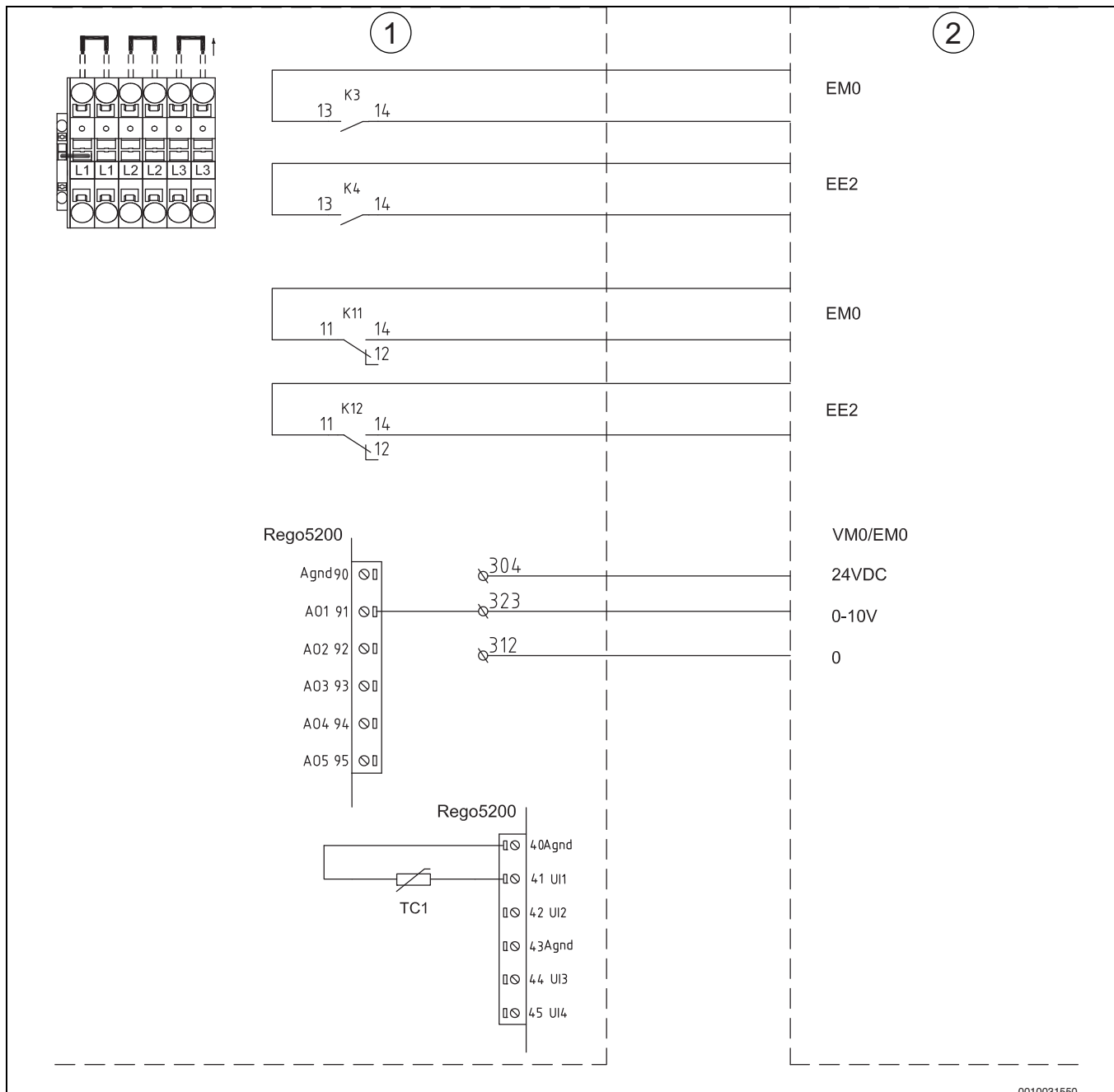
Bild 31 Anschluss des externen Zuheizers mit Mischer (22–80 kW)
