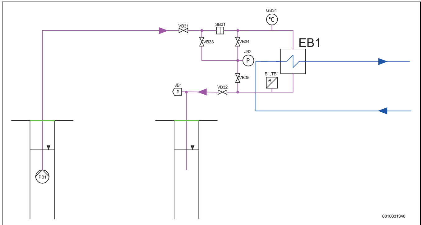
Bild 38 Grundwassersystem
