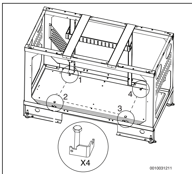
Bild 6 Transportsicherungen, Wärmepumpe
