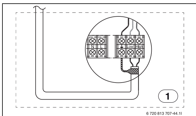
Bild 25 CAN-BUS-Verbindung
