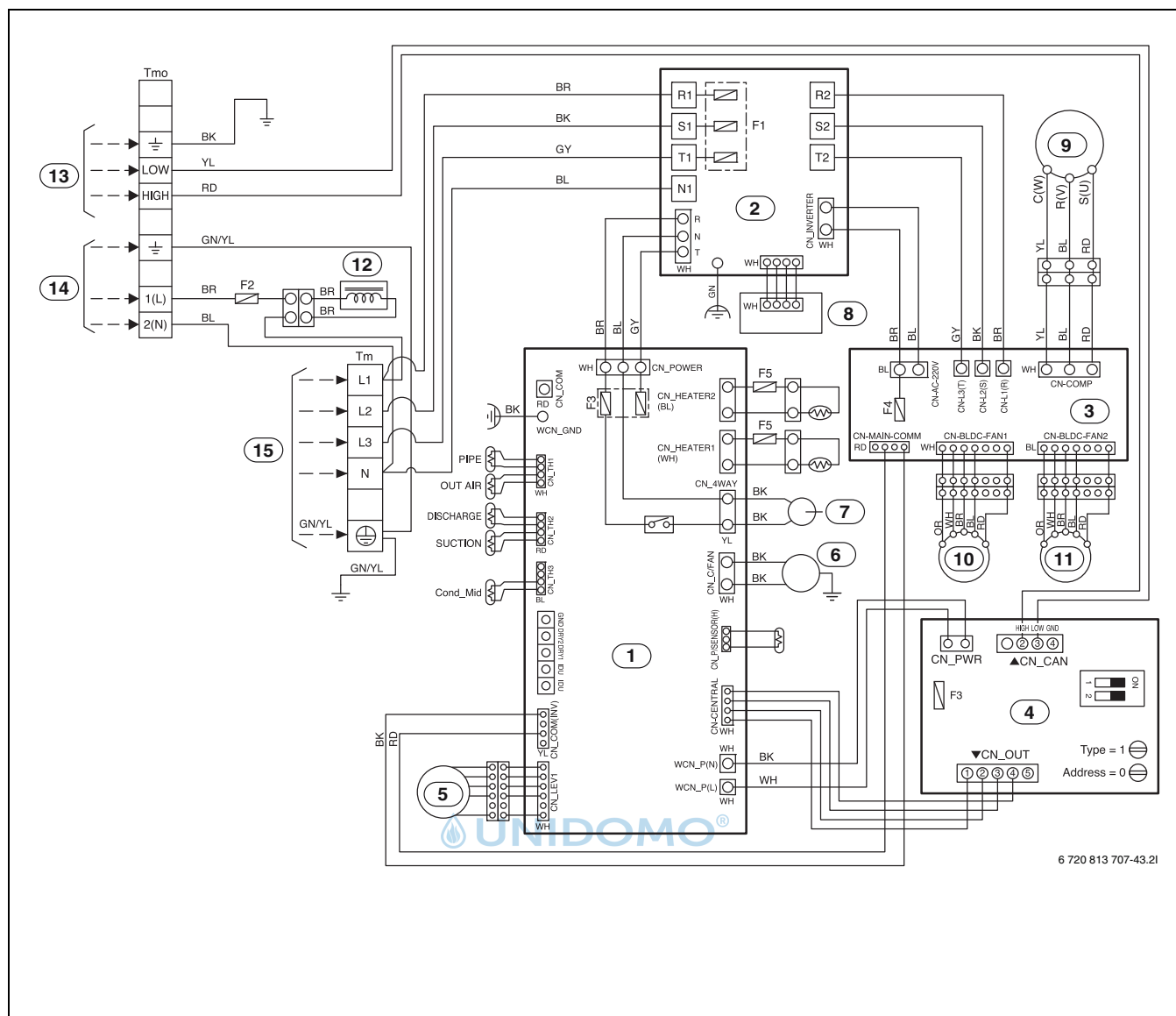
Bild 32 Split 11t-15t
