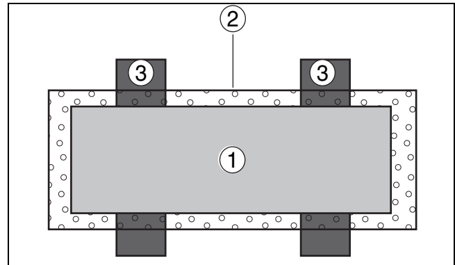
Bild 9 Außeneinheit auf der Bodenkonsole (Draufsicht)
