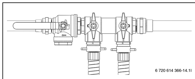
Bild 22 Befüllstation STE 60-1 - 100-1, STM 60-1 - 100-1
