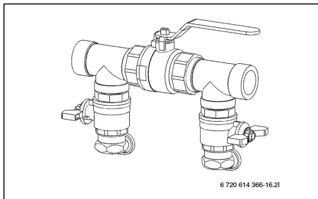
Bild 22 Befüllvorrichtung STE 130-1 - 170-1
