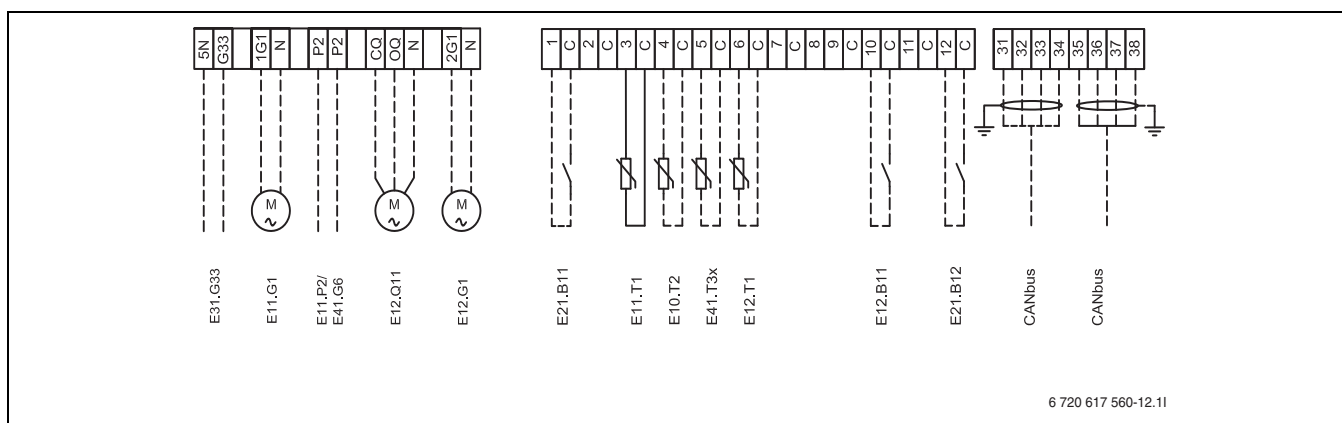
Bild 43 Externe Anschlüsse
