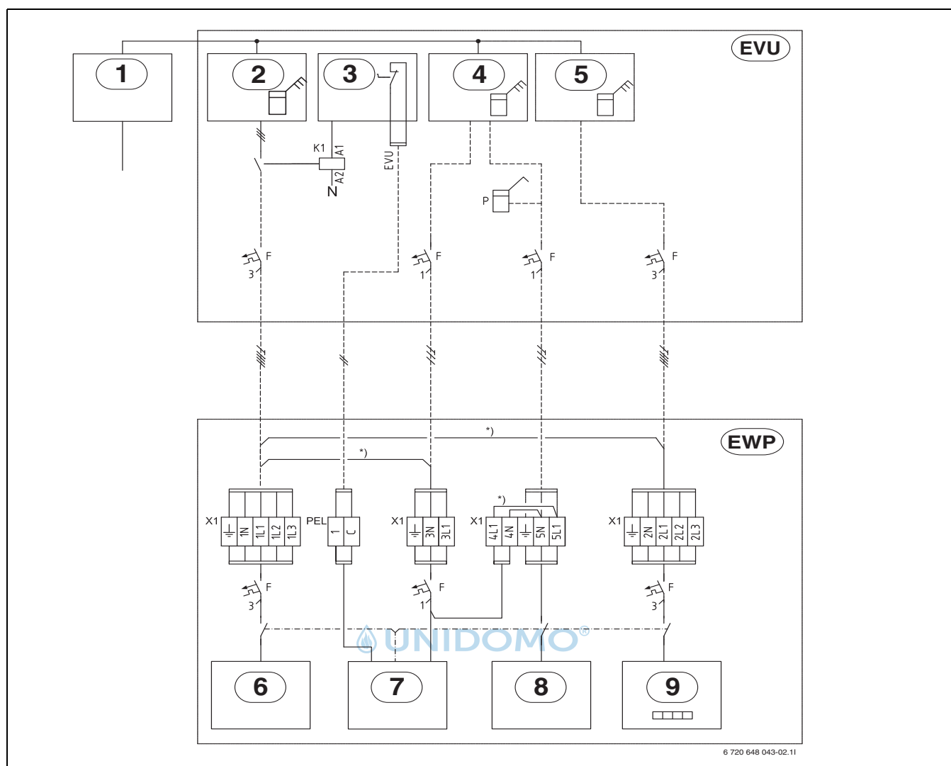
Bild 29 Anschlussübersicht Elektroschaltschrank - Wärmepumpe
