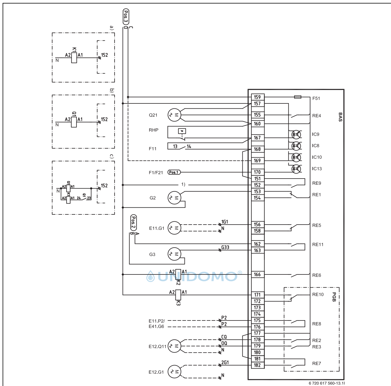
Bild 46 Kompletter Anschlussschaltplan (230 V)
