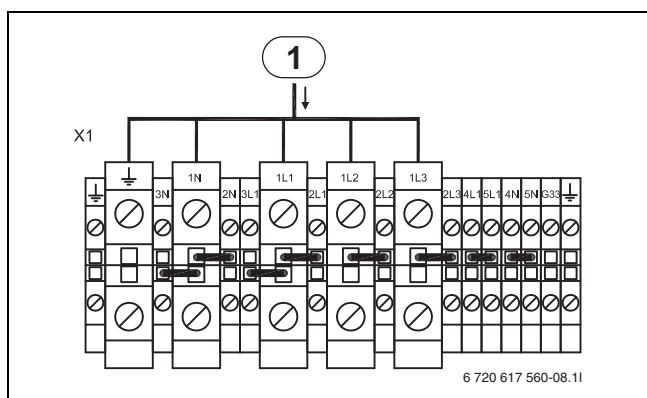
Bild 39 Standardausführung, STE 130-1 - 170-1
