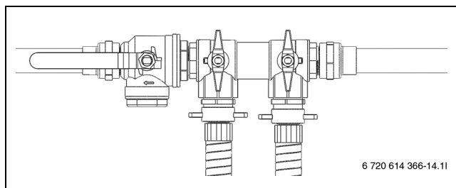
Bild 21 Befüllvorrichtung STE 60-1 - 100-1, STM 60-1 - 100-1
