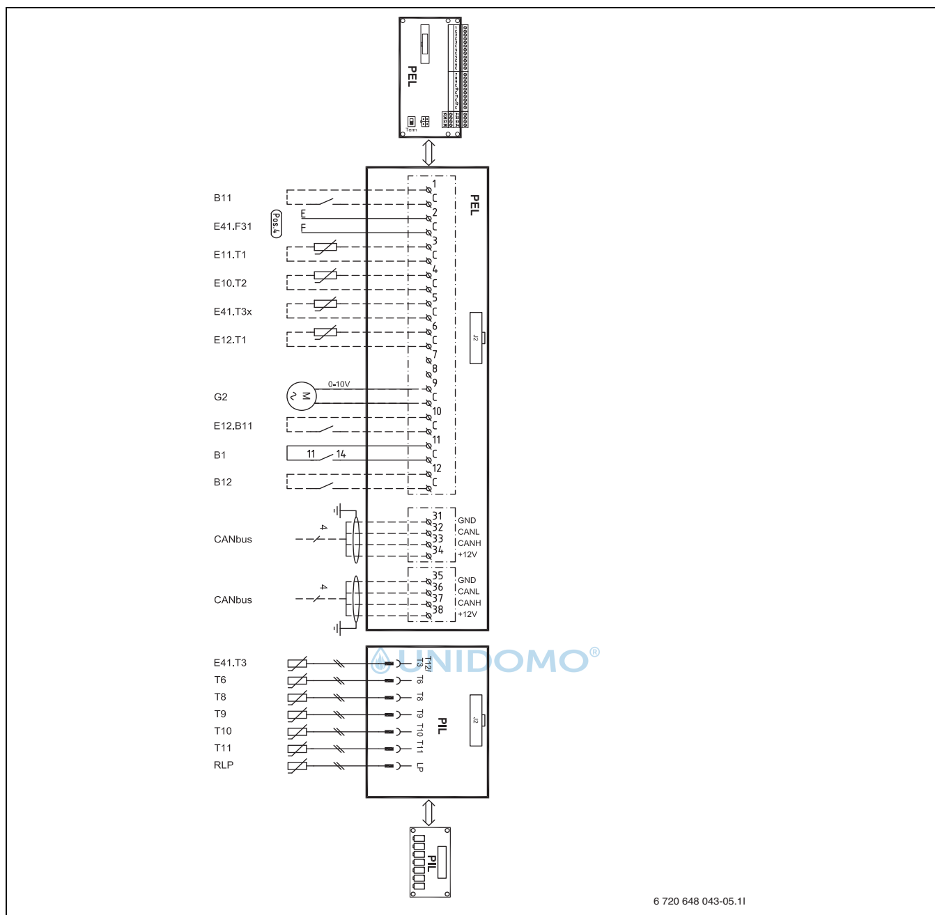
Bild 47 Kompletter Anschlussschaltplan (Niederspannung)
