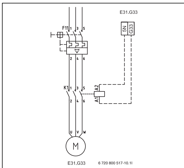
Bild 44 Anschluss Grundwasserpumpe
