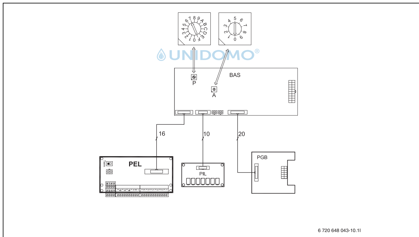
Bild 32 Leiterplattenverbindungen
