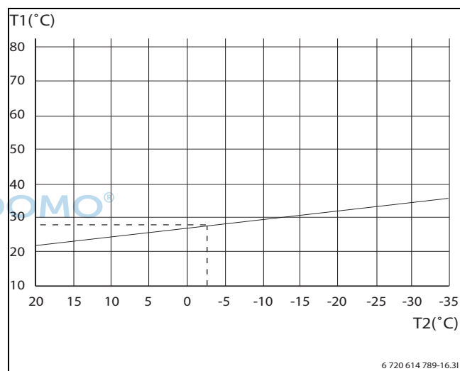
Bild 51 Fußbodenheizung
