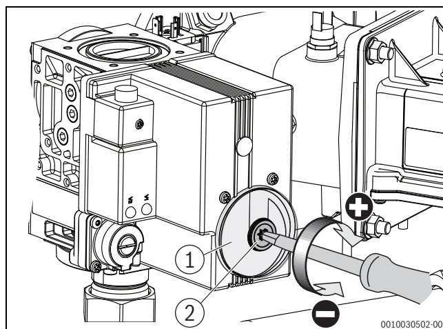
Bild 14 O 2 -Gehalt bei Volllast einstellen (Kesselgröße 150 kW [bis V03] – 300 kW)
