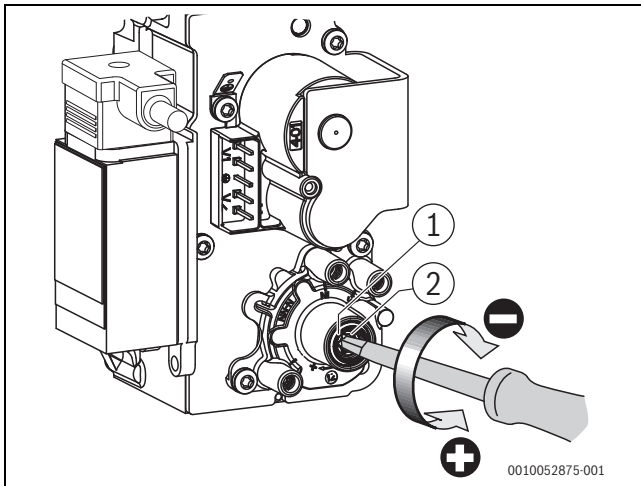
Bild 16 O 2 -Gehalt bei Teillast einstellen (Kesselgröße 150 kW [V04])
