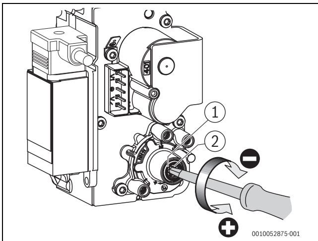
Bild 12 O 2 -Gehalt bei Teillast einstellen (Kesselgröße 150 kW [V04])
