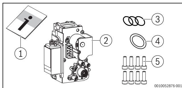
Bild 3 Lieferumfang Ersatz-Gasarmatur 150 kW [V04] 2)
