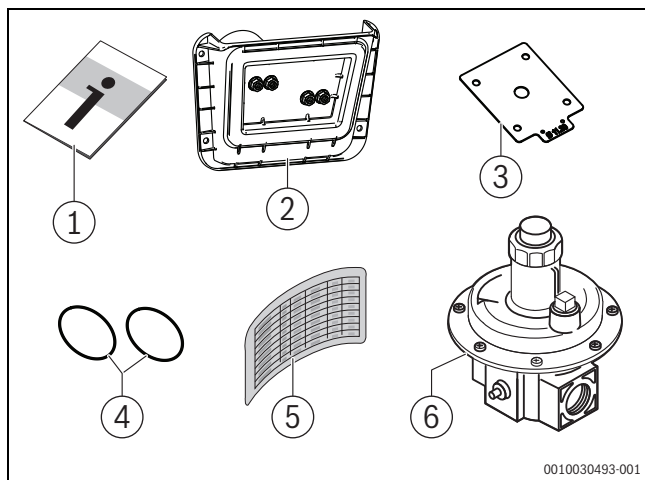
Bild 4 Lieferumfang Umstell-Set Flüssiggas
