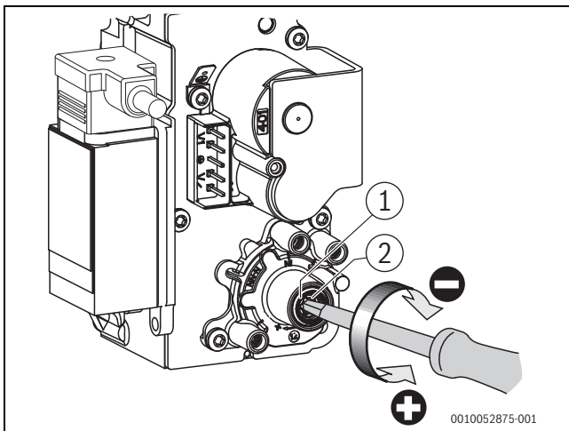
Bild 7 O 2 -Gehalt bei Teillast einstellen (Kesselgröße 150 kW [V04])
