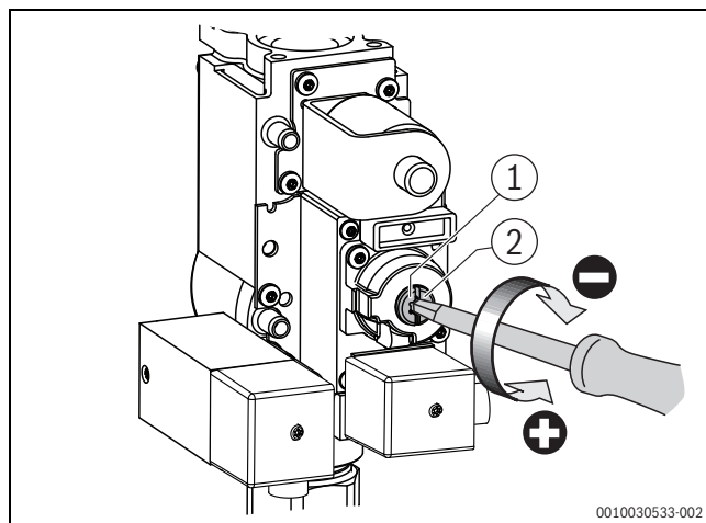
Bild 15 O 2 -Gehalt bei Teillast einstellen (Kesselgröße 75 – 100 kW)
