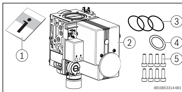
Bild 2 Lieferumfang Ersatz-Gasarmatur 150 kW [bis V03] 1) – 300 kW
