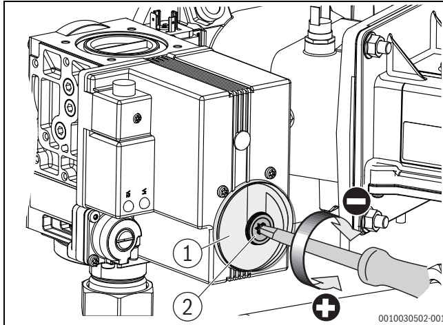
Bild 5 CO 2 -Gehalt bei Volllast einstellen (Kesselgröße 150 – 300 kW)
