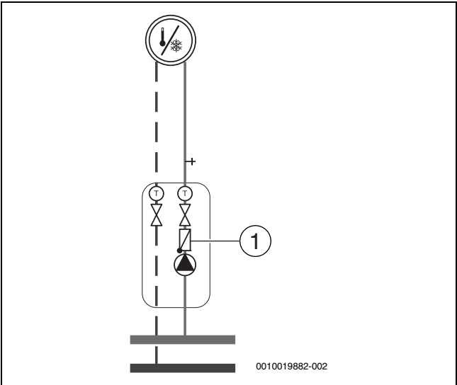
Bild 25 Heizkreis
