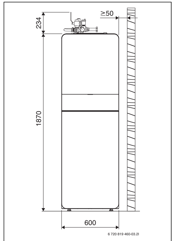
Bild 4 Abmessungen (mm)
