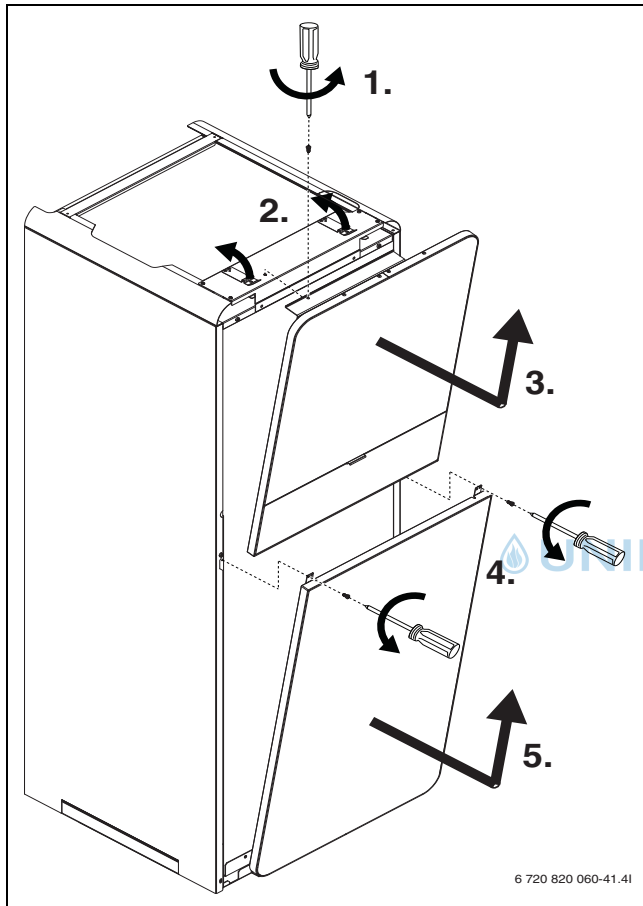
Bild 6 Frontplatten abnehmen
