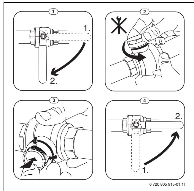
Bild 18 Siebreinigung
