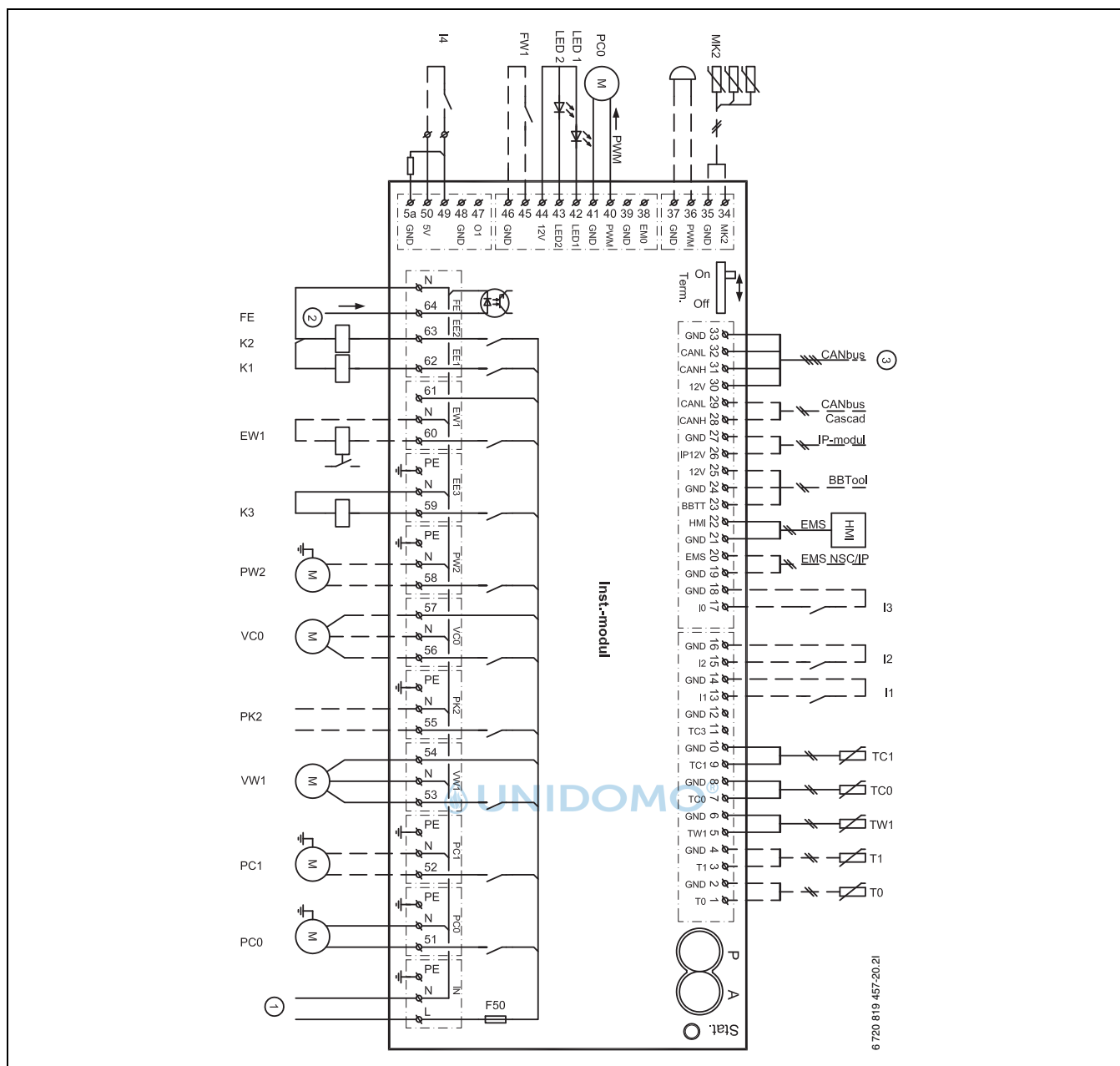
Bild 29 Schaltplan, Installationsmodul
