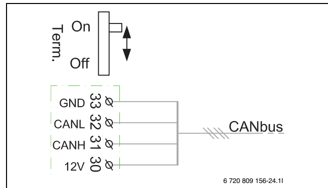
Bild 12 CAN-BUS-Terminierung
