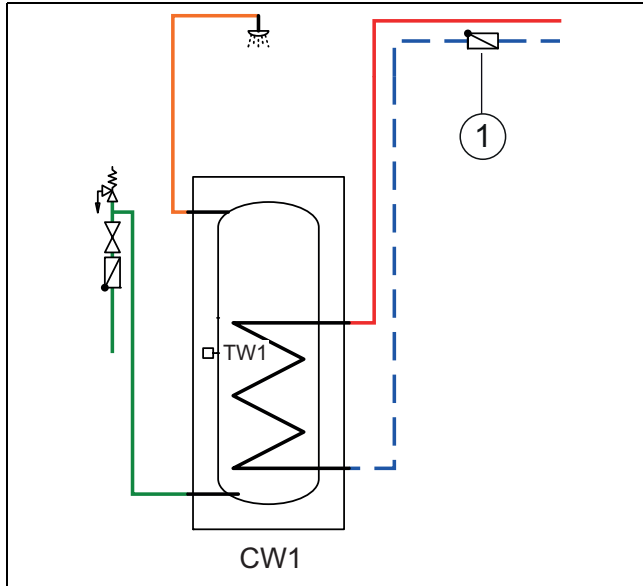
Bild 17 Warmwasserspeicher
