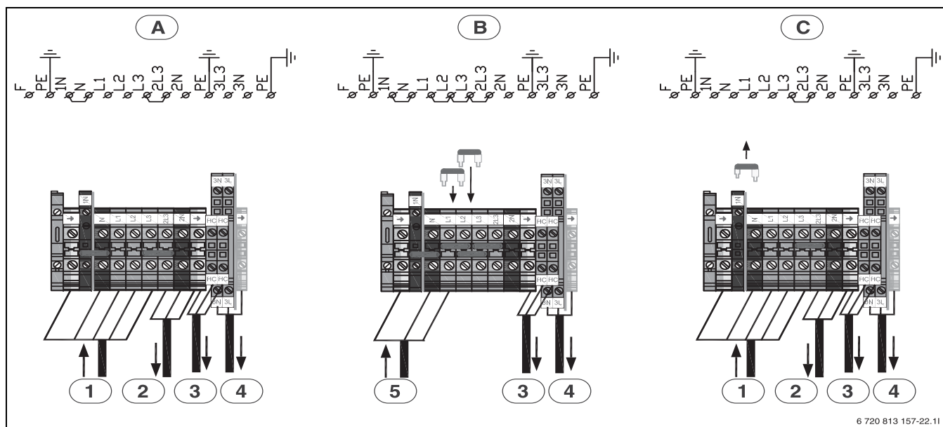
Bild 31 Anschlussklemmen
