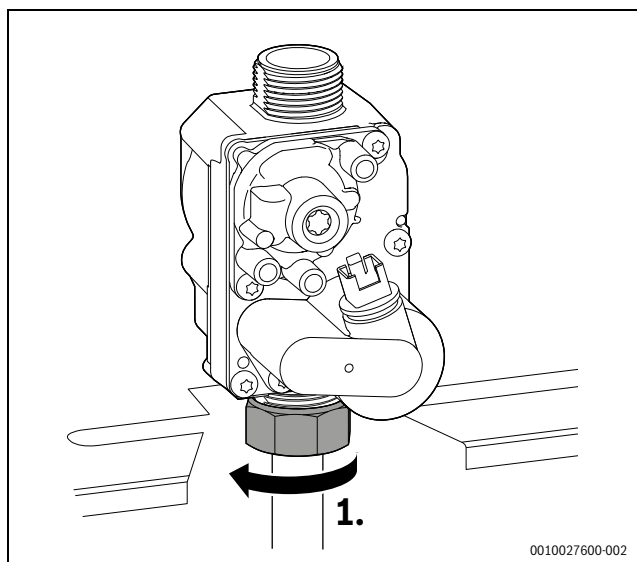
Bild 79 Überwurfmutter lösen
