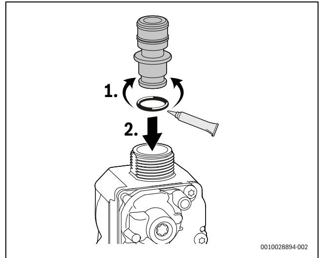
Bild 83 Gasdrossel einsetzen
