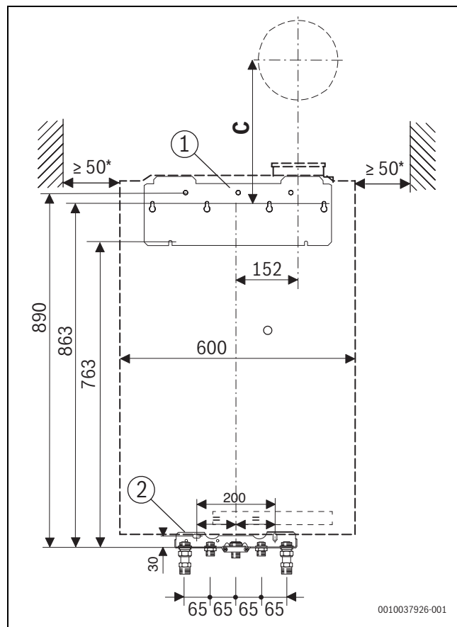
Bild 4 Frontansicht, vertikaler hydraulischer Anschluss(mm)
