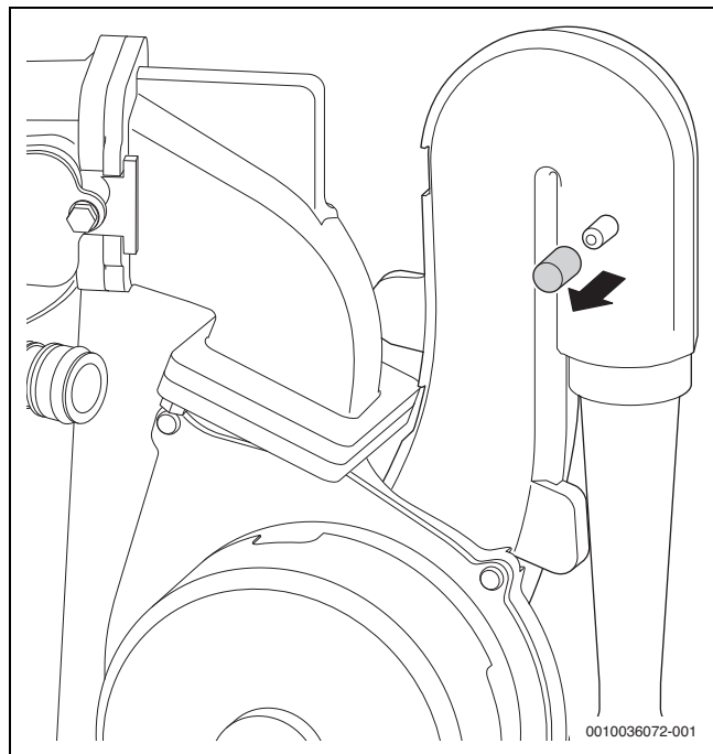
Bild 55 Messstutzen an der Mischeinrichtung
