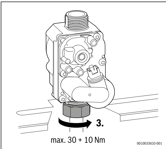
Bild 82 Anzugsdrehmoment beachten
