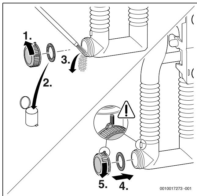
Bild 70 Kondensatsiphon reinigen
