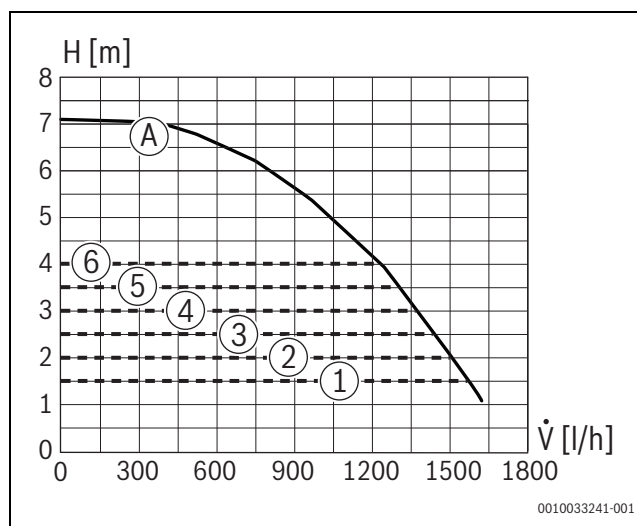
Bild 89 Pumpenkennfelder und Pumpenkennlinien
