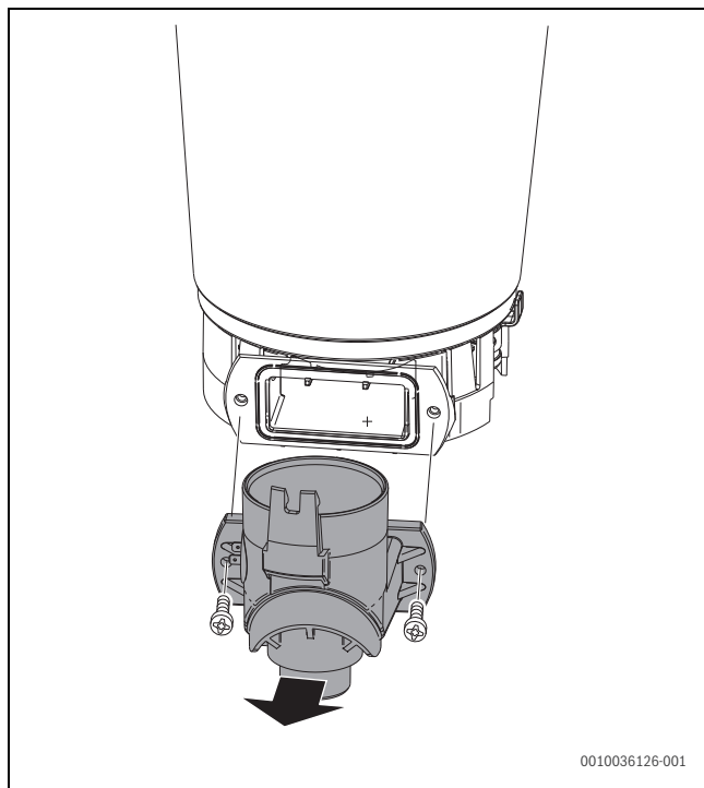
Bild 67 Prüfoffnung öffnen
