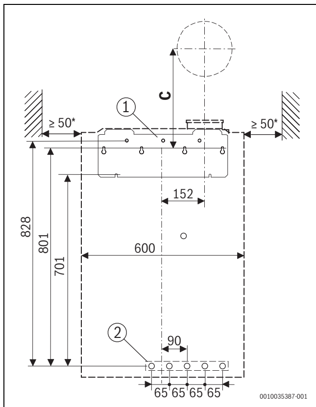
Bild 3 Frontansicht, horizontaler hydraulischer Anschluss(mm)
