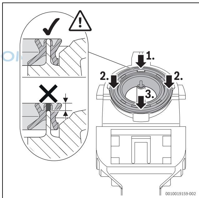
Bild 73 Dichtung andrücken
