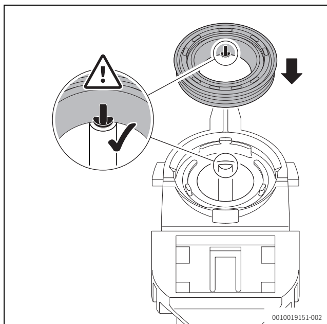
Bild 72 Neue Dichtung am Kondensatsiphon ausrichten
