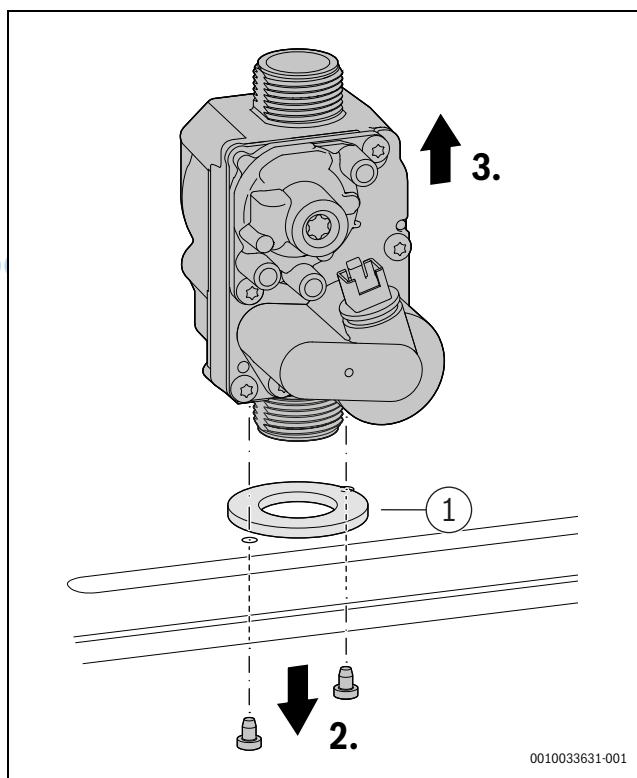
Bild 80 Gasarmatur ausbauen
