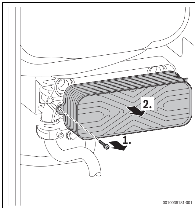
Bild 56 Plattenwärmetauscher ausbauen
