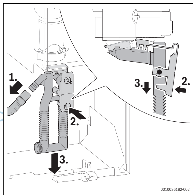
Bild 69 Kondensatsiphon ausbauen
