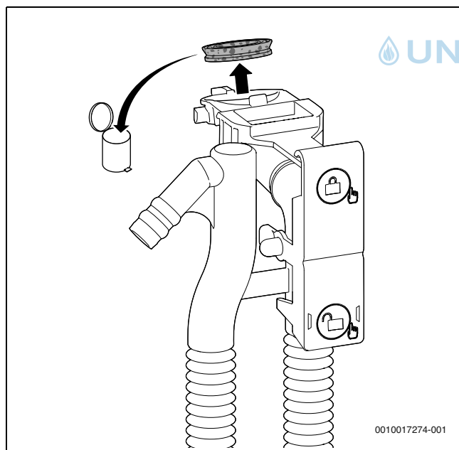
Bild 71 Dichtung oben am Kondensatsiphon entfernen
