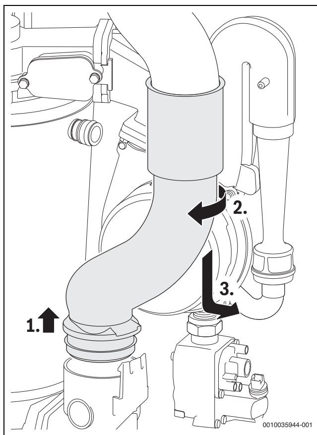
Bild 57 Abgasrohr ausbauen
