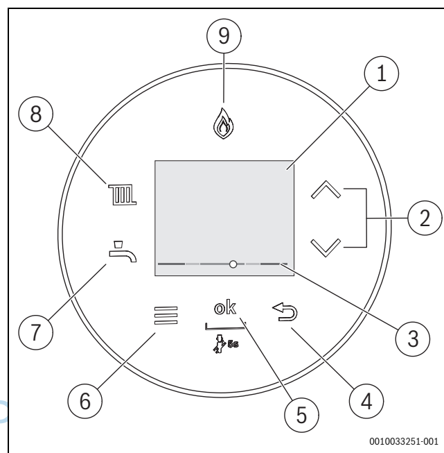
Bild 48 Bedienfeld
