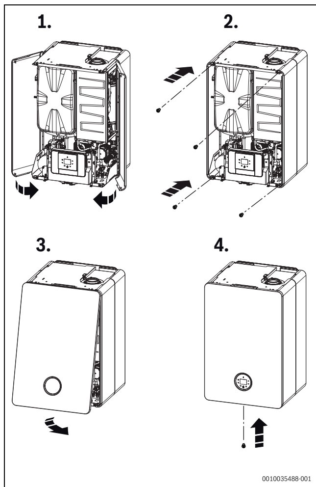
Bild 47 Verkleidung montieren
