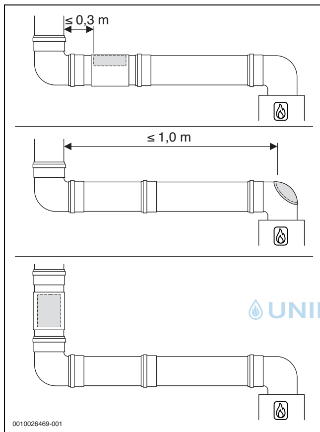
Bild 7 Anordnung der unteren Prüfföffnung
