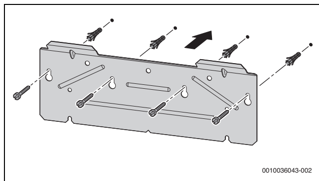
Bild 33 Aufhängeschiene montieren
