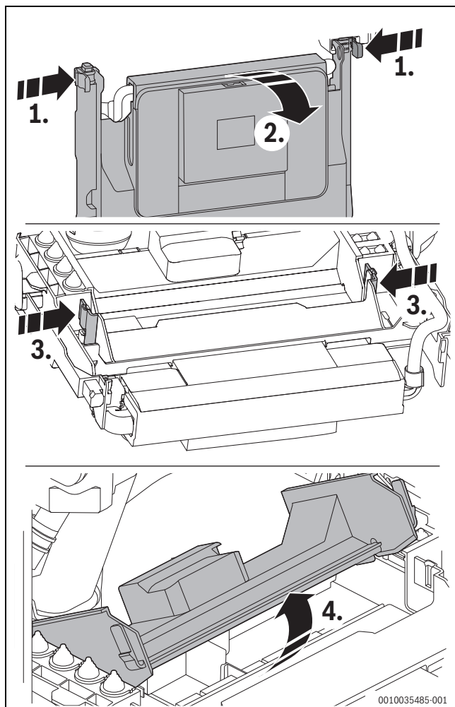
Bild 44 Steuergerät öffnen
