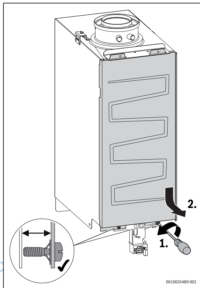
Bild 49 Brennerhaube abnehmen
