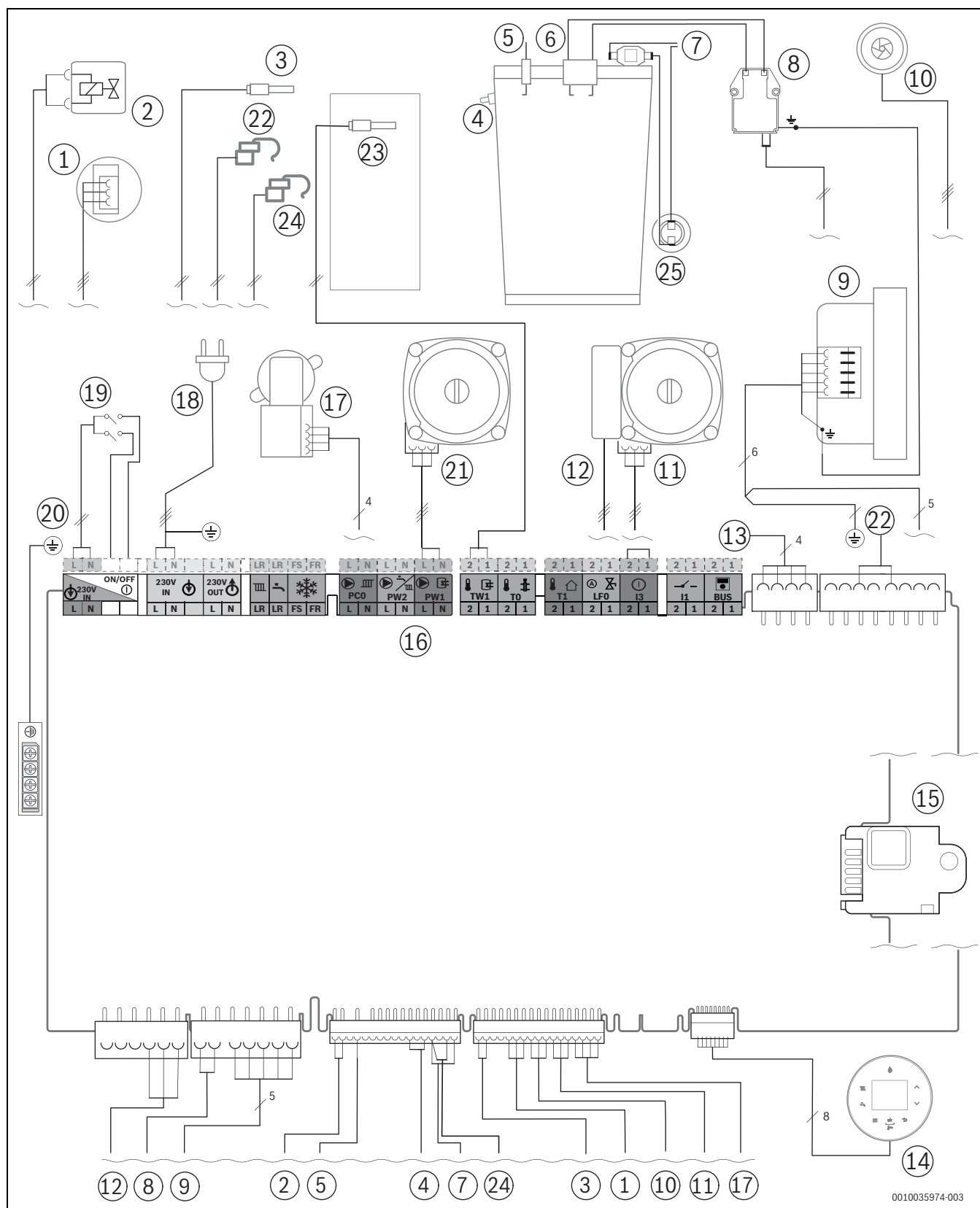
Bild 90 Elektrische Verdrahtung
