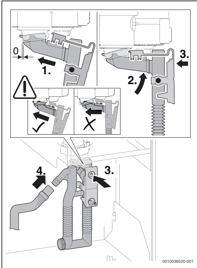
Bild 74 Kondensatsiphon einsetzen
