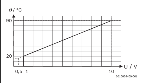
Afb. 2 Lineaire relatie tussen 0-10 V-sigitaal (U in Volt) en gevraagd vermogen van de aanvoertemperatuur (θ in °C)
