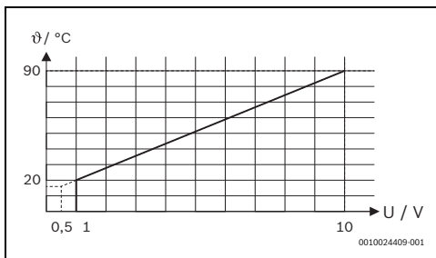
Obr. 2 Lineární závislost mezi signálem 0-10 V (U ve V) a požadovanou teplotou na výstupu (9 ve °C)
