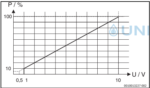
Afb. 1 Lineaire relatie tussen 0-10 V-sigitaal (U in Volt) en gevraagd vermogen (P in procenten)
