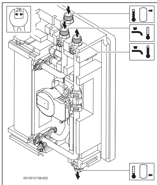
Bild 25 Anschlüsse Frischwasserstation
