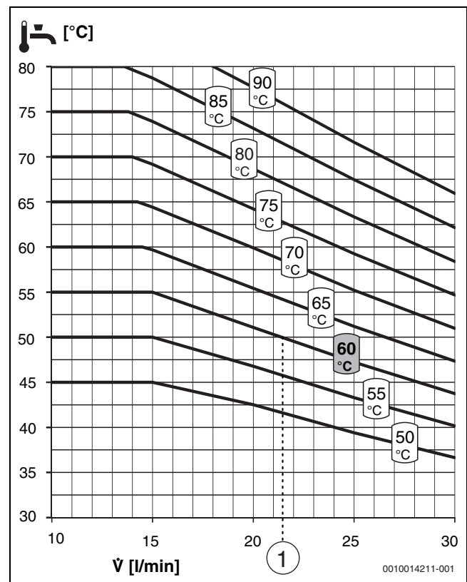
Bild 40 Temperaturverhalten FF20
