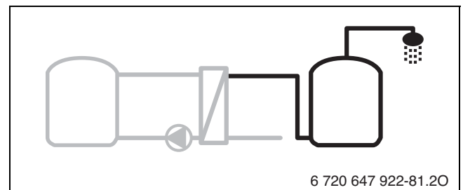
Bild 31 Display: Vorwärmen des Warmwassers mit der Frischwasserstation
