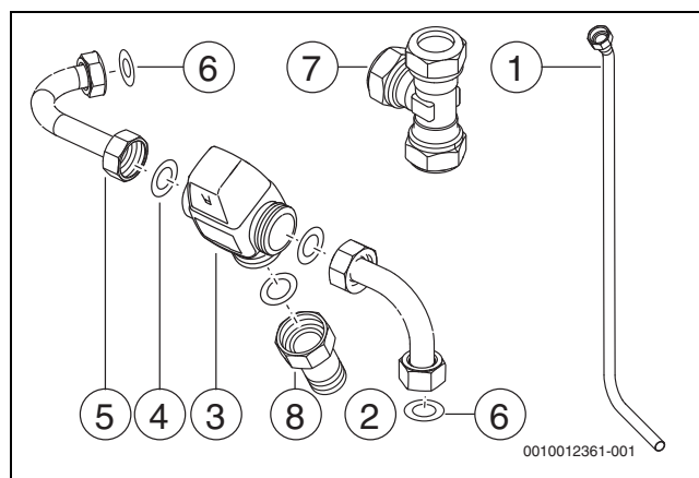
Bild 18 Lieferumfang Mischventil-Set
