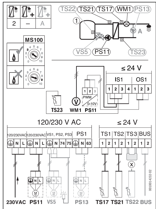
Bild 34 Anschlussklemmen bei Frischwasserstation
