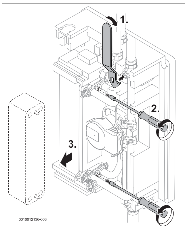
Bild 43 Wärmetauscher demontieren
