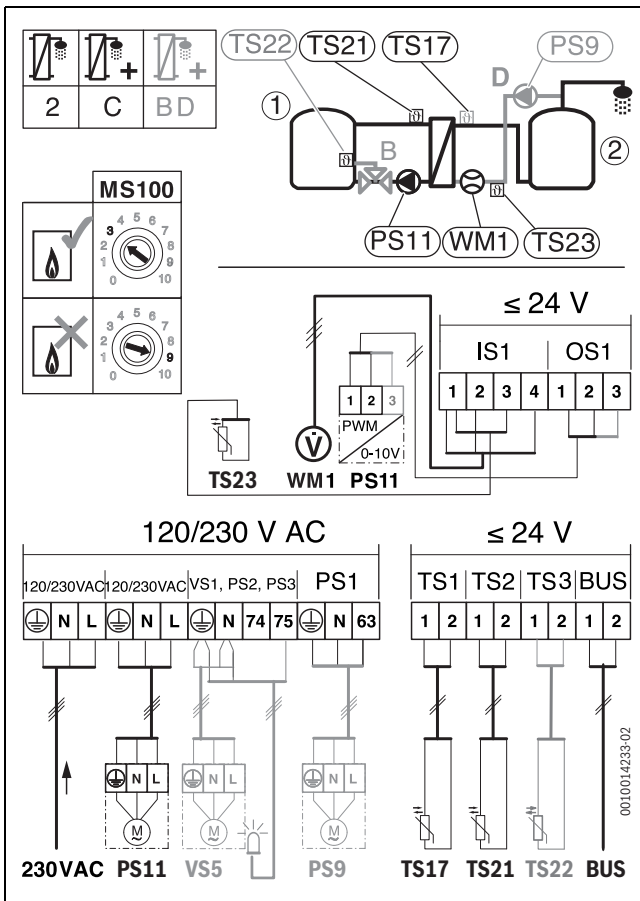
Bild 35 Anschlussklemmen bei Vorwärm-Frischwasserstation
