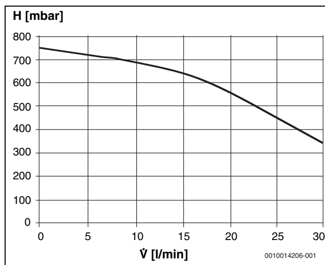
Bild 6 Restförderhöhe Primärkreispumpe
