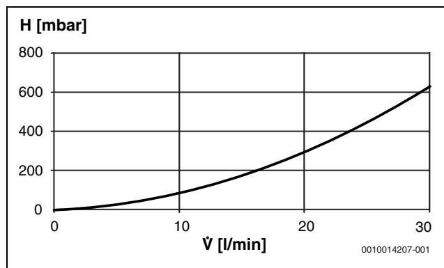
Bild 7 Druckverlust Sekundärseite
