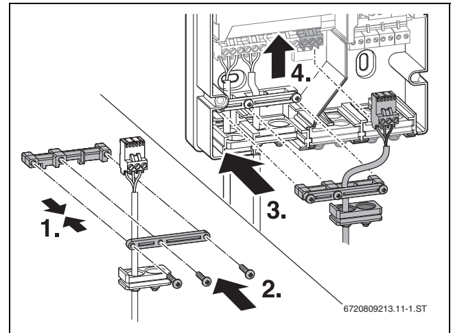
Bild 37 Zugentlastungen montieren und Stecker einstecken
