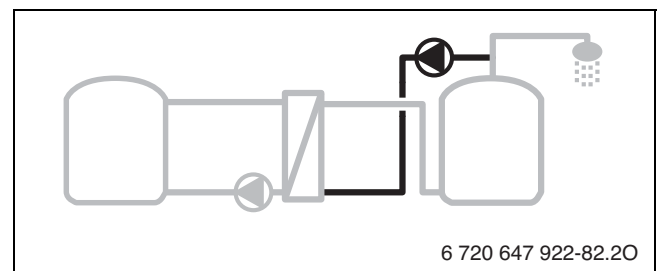
Bild 32 Display: Tägliche Aufheizung zur Vermeidung von Legionellen
