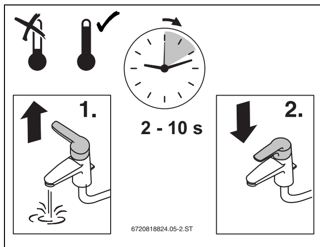
Bild 39 Zirkulation über Impuls aktivieren
