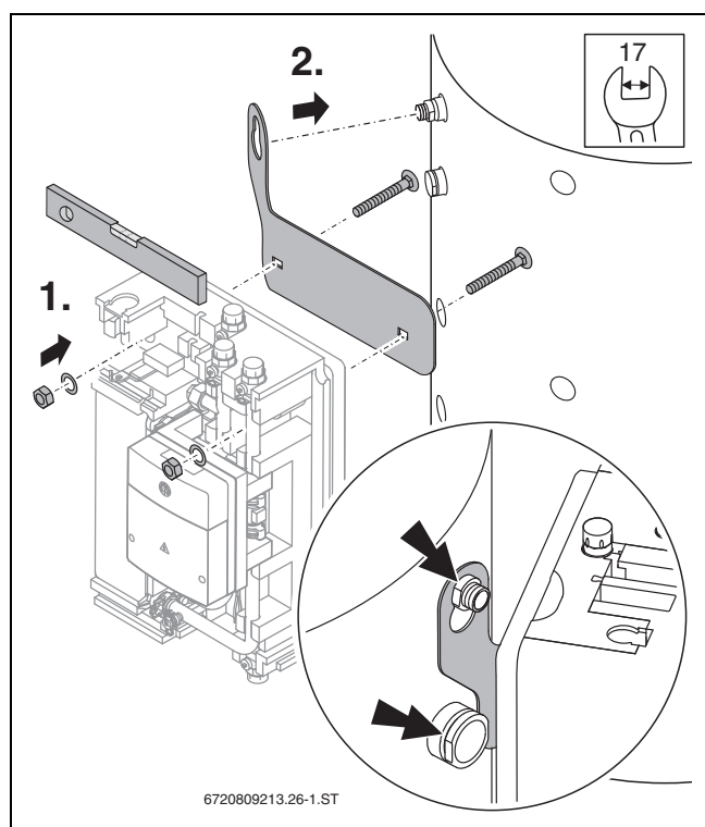
Bild 14 Halteblech montieren
