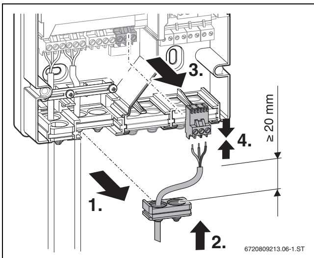
Bild 36 Pumpe anschließen (Zirkulation oder tägliche Aufheizung)
