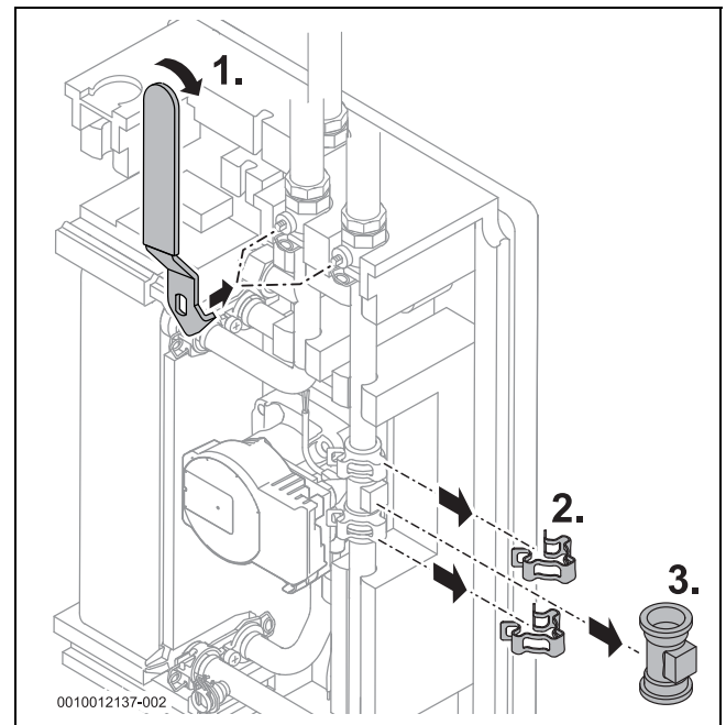
Bild 44 Volumenstromfühler demontieren
