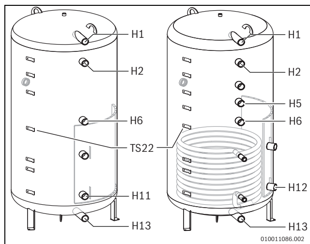
Bild 26 Pufferspeicher ohne Trennbleche
