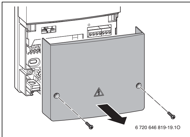
Bild 33 Modul öffnen
