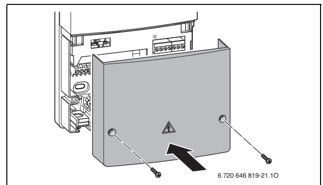
Bild 38 Abdeckung montieren
