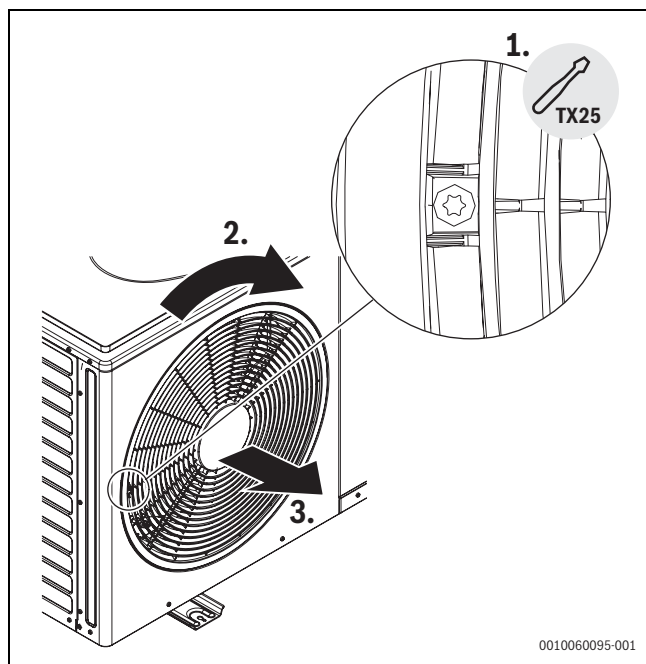
Bild 38 Anleitung für die Demontage der Ventilatorblende
