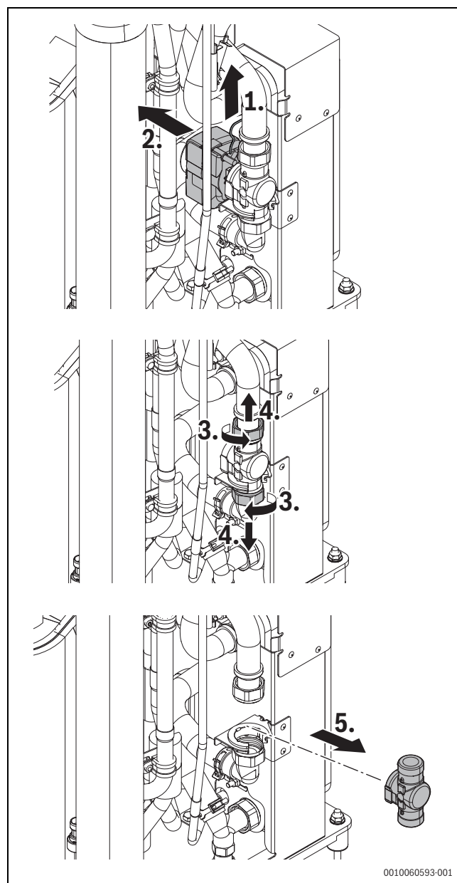
Bild 45 Ausbau des normalerweise geschlossenen Ventils
