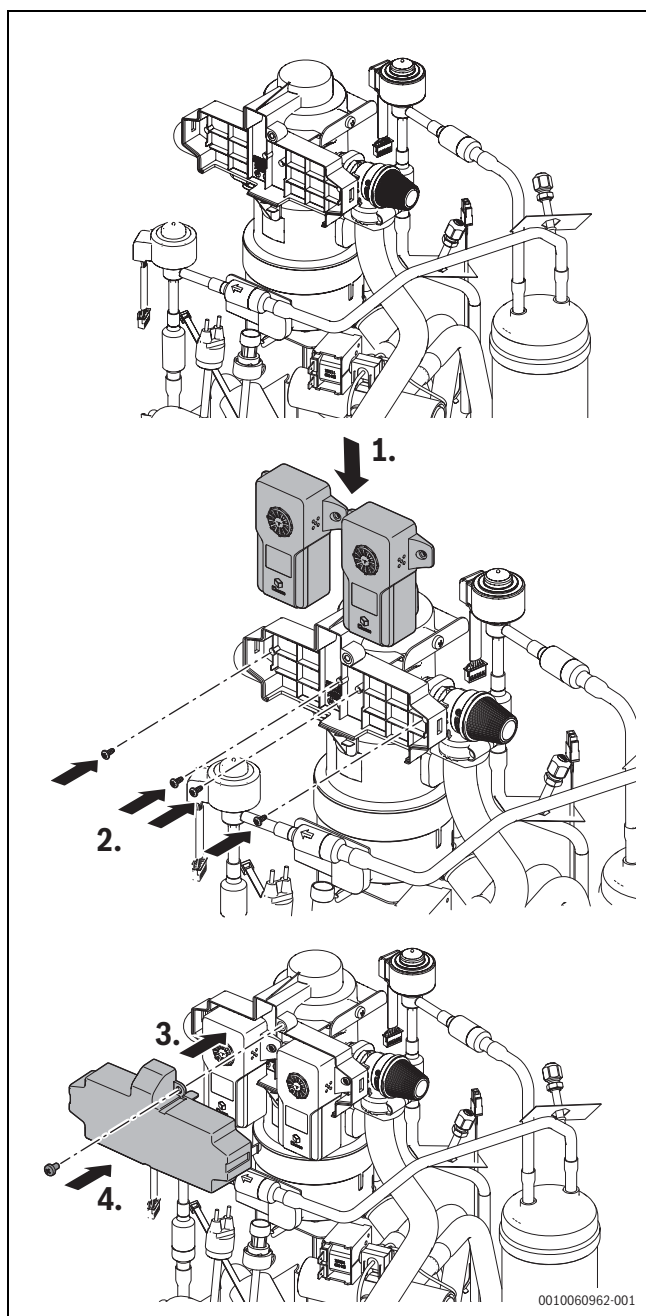
Bild 44 R290-Fühler austauschen
