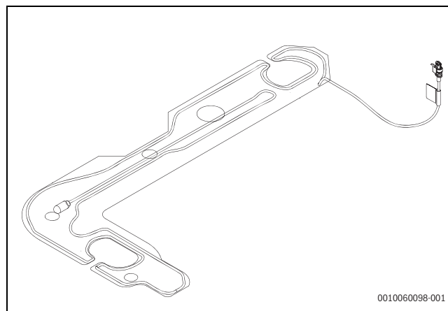
Bild 41 Kondensatwannenheizung
