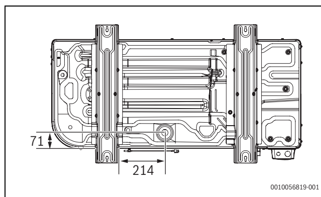
Bild 7 Abmessungen der Wärmepumpe, Ansicht Unterseite
