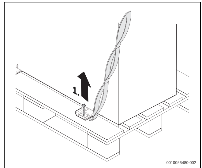
Bild 16 Schrauben entfernen.
