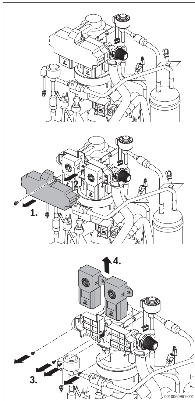
Bild 43 R290-Fühler austauschen
