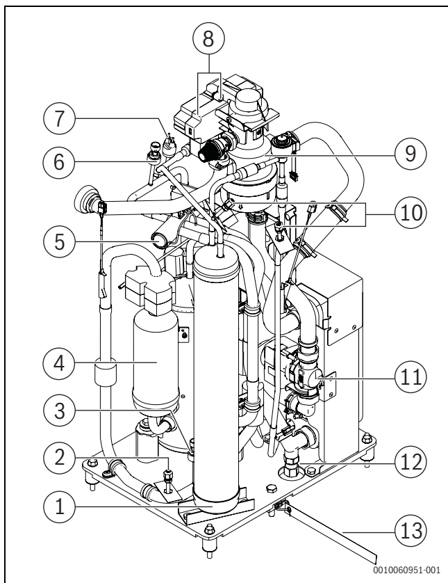
Bild 2 Kältekreis-Übersicht
