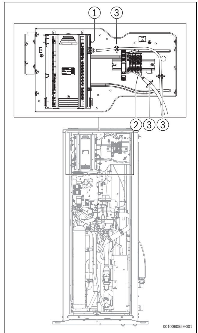
Bild 37 Anschlussklemmen im Anschlussbereich bei Installation (O-T)
