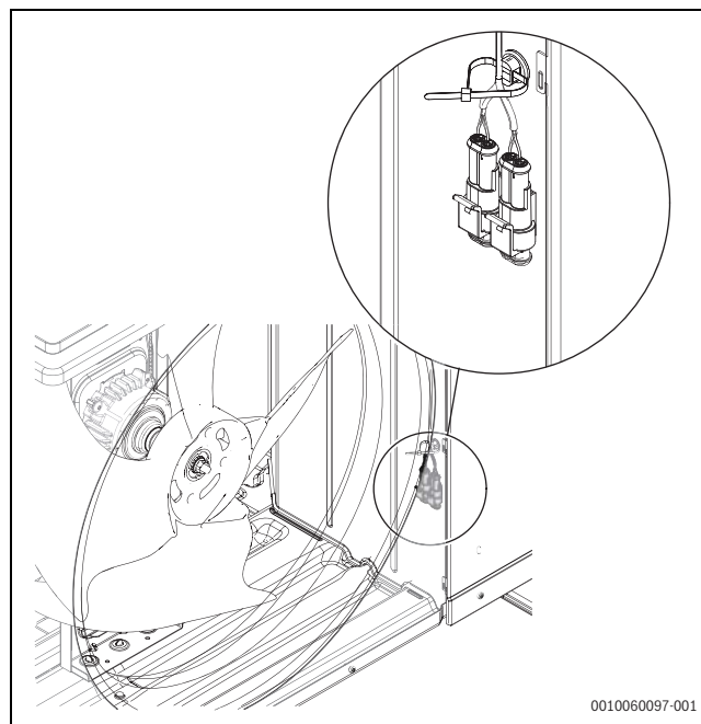
Bild 40 Kondensatwannenheizung und Heizkabelanschluss
