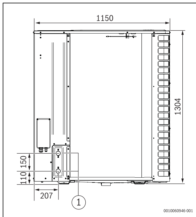
Bild 4 Abmessungen und Hydraulik Anschlüsse der Wärmepumpe, Rückansicht
