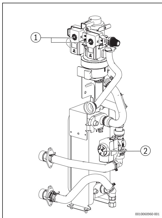
Bild 42 Propan-Sicherheitskit
