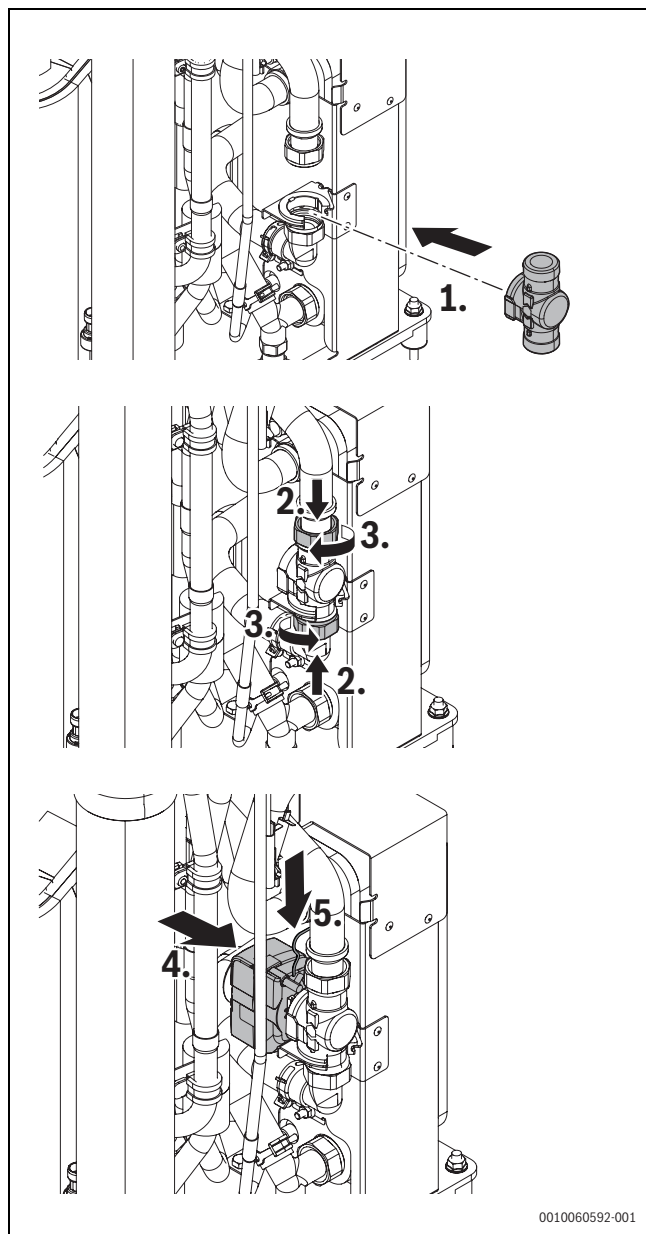
Bild 46 Anwendung des normalerweise geschlossenen Ventils
