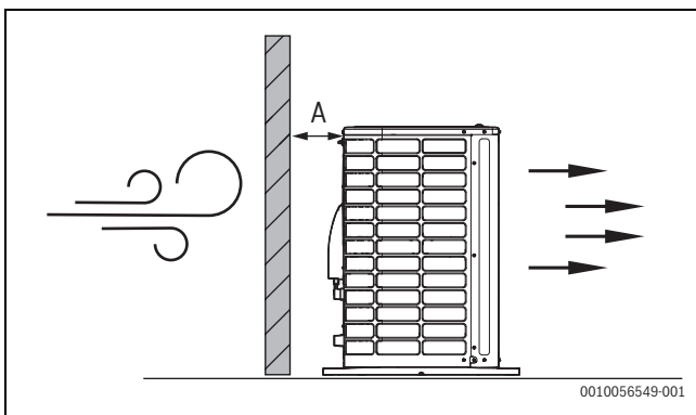
Bild 19 Freistehende Wärmepumpe
