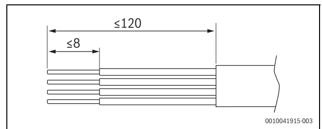
Bild 32 Abisolierung CAN-BUS (mm)
