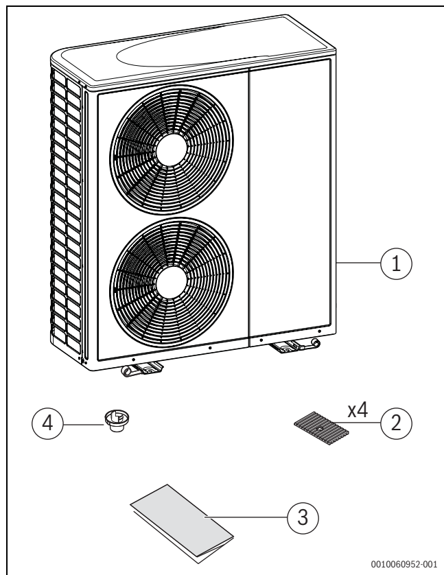
Bild 1 Gerät und Teile aus dem Zubehörkarton
