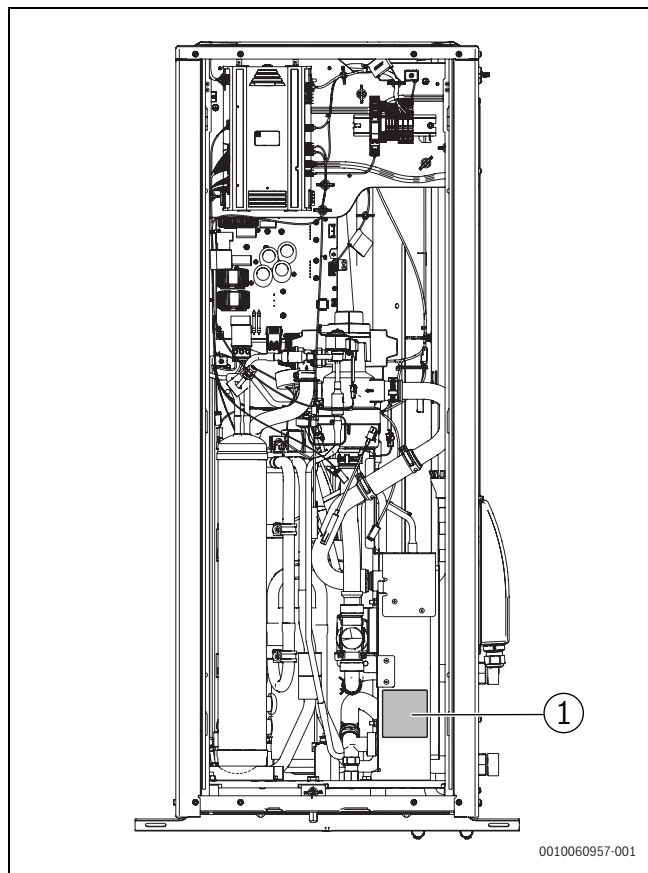
Bild 5 Platz für Typschild auf Halterung des Plattenwärmetauschers (PHE)
