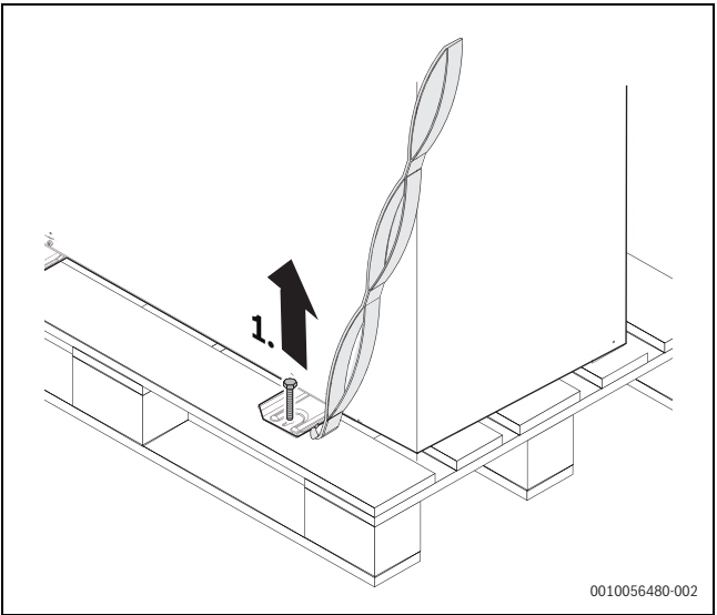
Bild 16 Schrauben herausdrehen.
