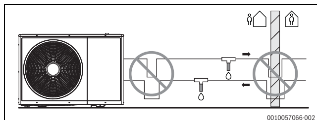
Bild 22 Installation des Frostschutzventils
