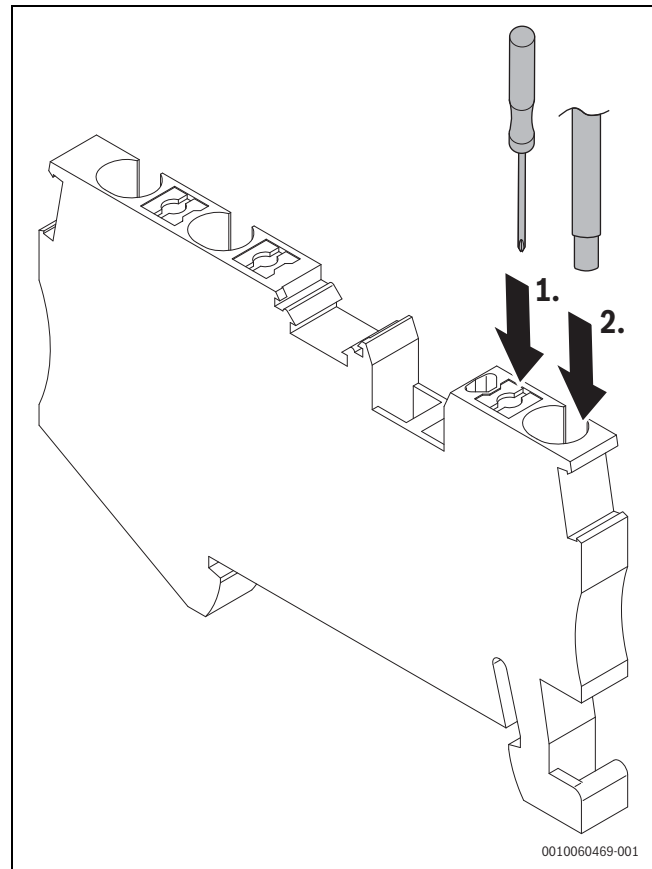
Bild 35 Netzkabelanschluss
