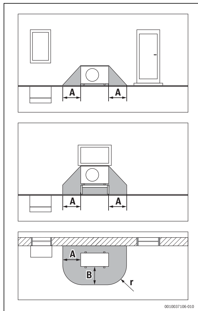
Bild 8 Schutzbereich bei bodenstehender Aufstellung
