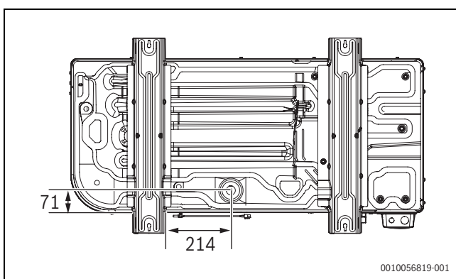
Bild 7 Abmessungen der Wärmepumpe, Ansicht von unten
