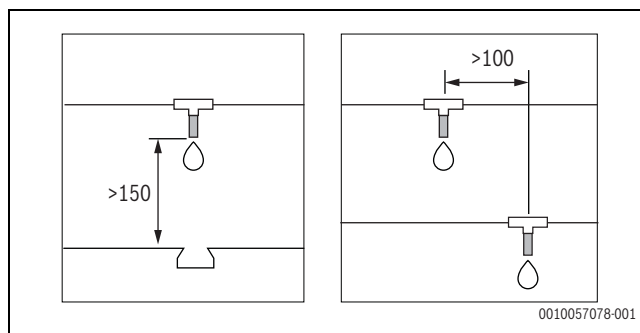
Bild 23 Montageabstände für Frostschutzventile in mm
