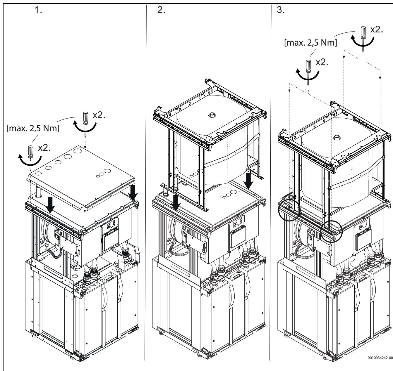
Fig. 73 Installazione dell'accumulatore inerziale sulla pompa di calore
