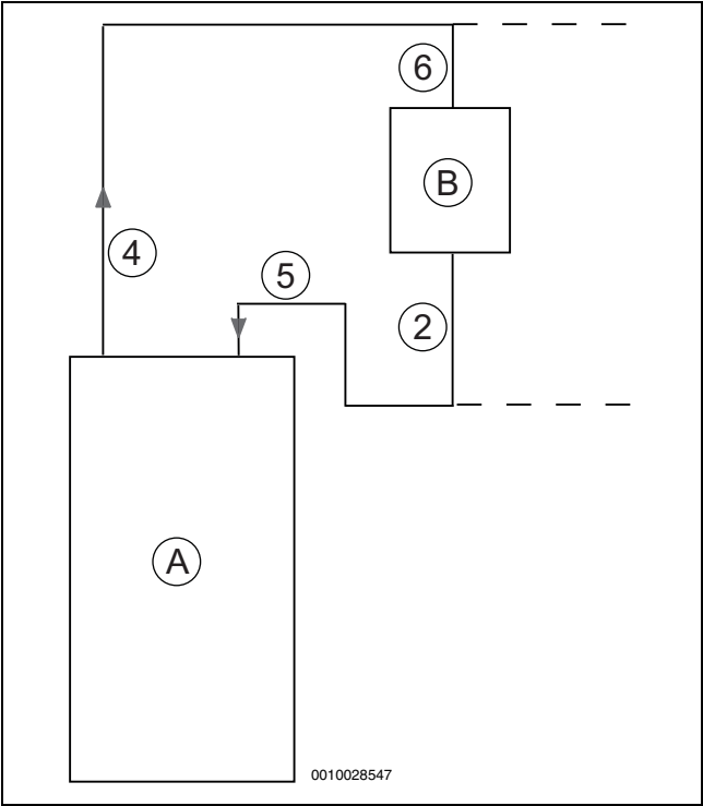
Fig. 79 Schema di principio – accumulatore inerziale con pompa di calore
