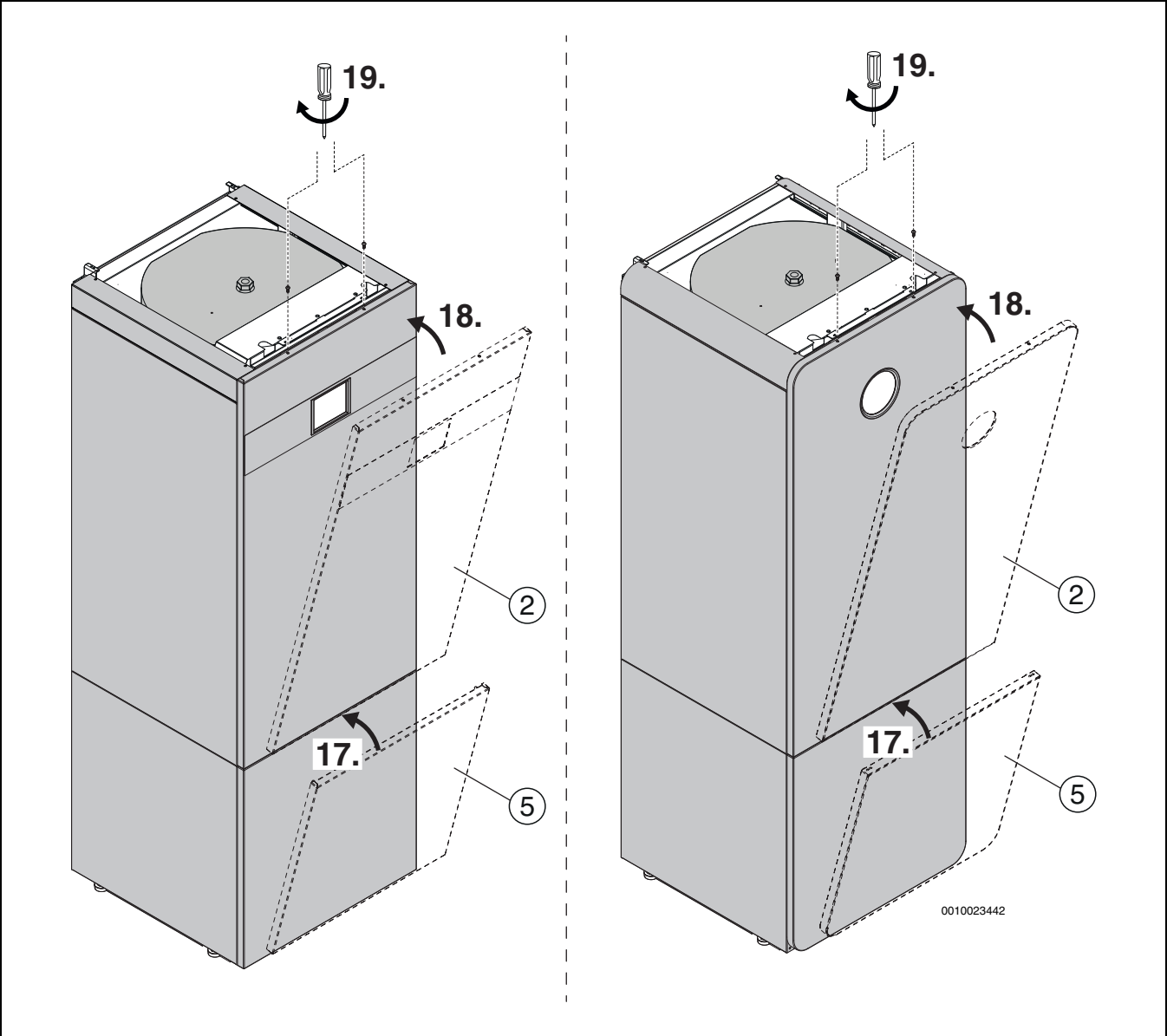
Afb. 115 Montage van de voorwanden met hoekige of ronde afdekking
