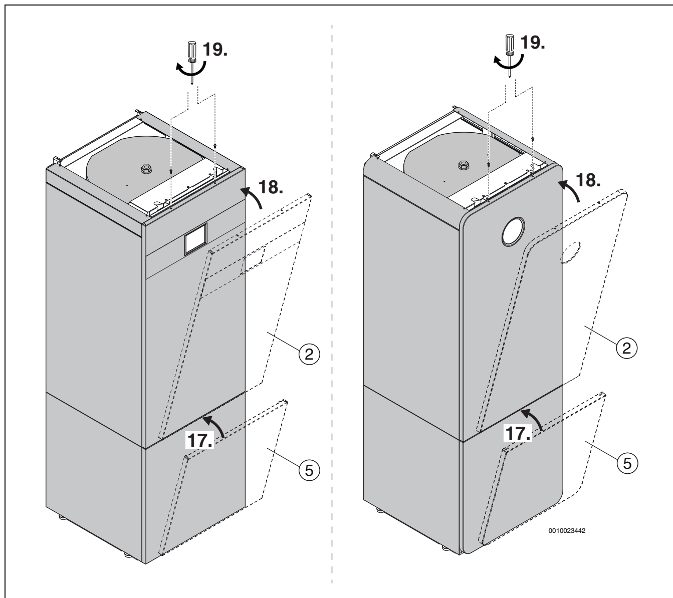
Fig. 86 Montaggio dei pannelli laterali con pannello protettivo rettangolare o circolare
