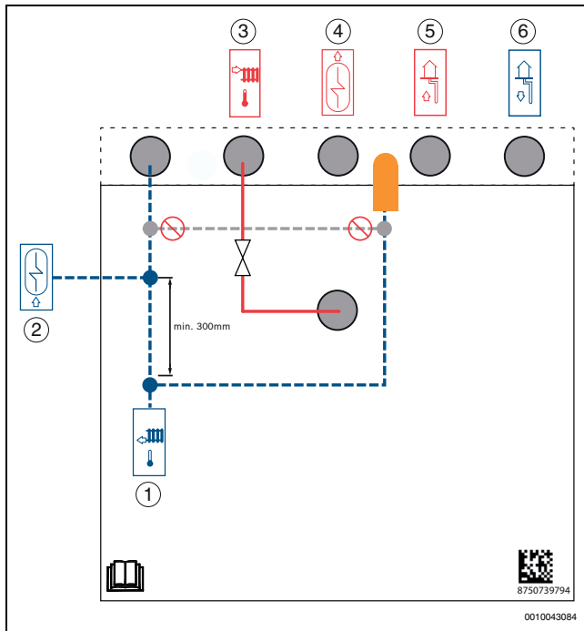
Bild 22 Anschluss Pufferspeicher
