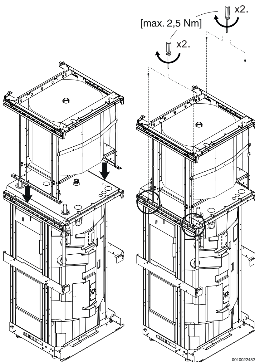
Fig. 65 Installazione dell'accumulatore inerziale sul bollitore di acqua calda sanitaria
