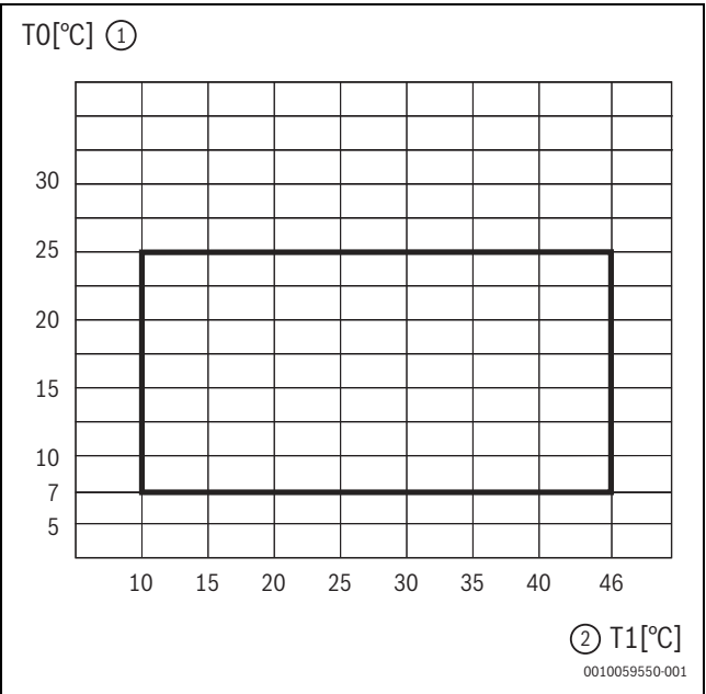
Fig. 8 Pompa di calore in modo raffreddamento
