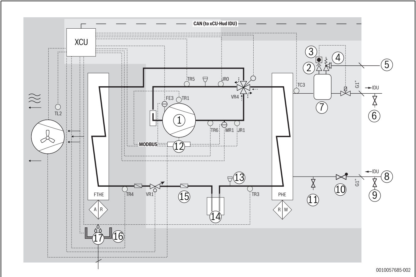
Afb. 9 koudemiddelcircuit
