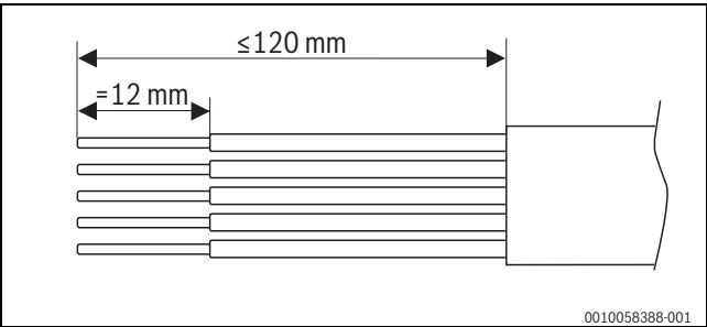
Rys. 4 Usuwanie izolacji z przewodu zasilania sieciowego
