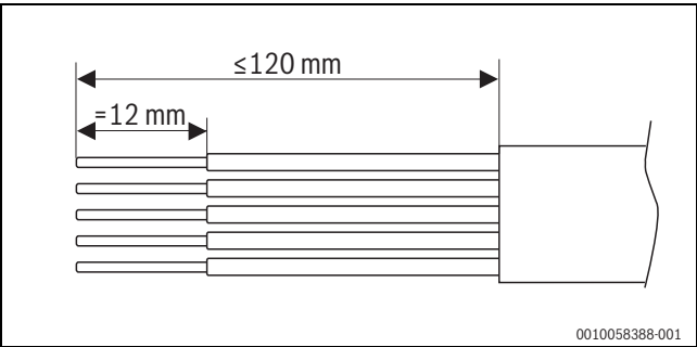
Afb. 4 Striplengte ader voedingsaansluiting
