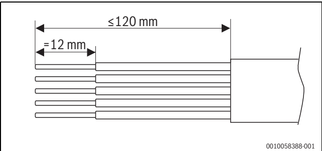
Fig. 4 Raccordement à l'alimentation secteur avec dénudage des fils
