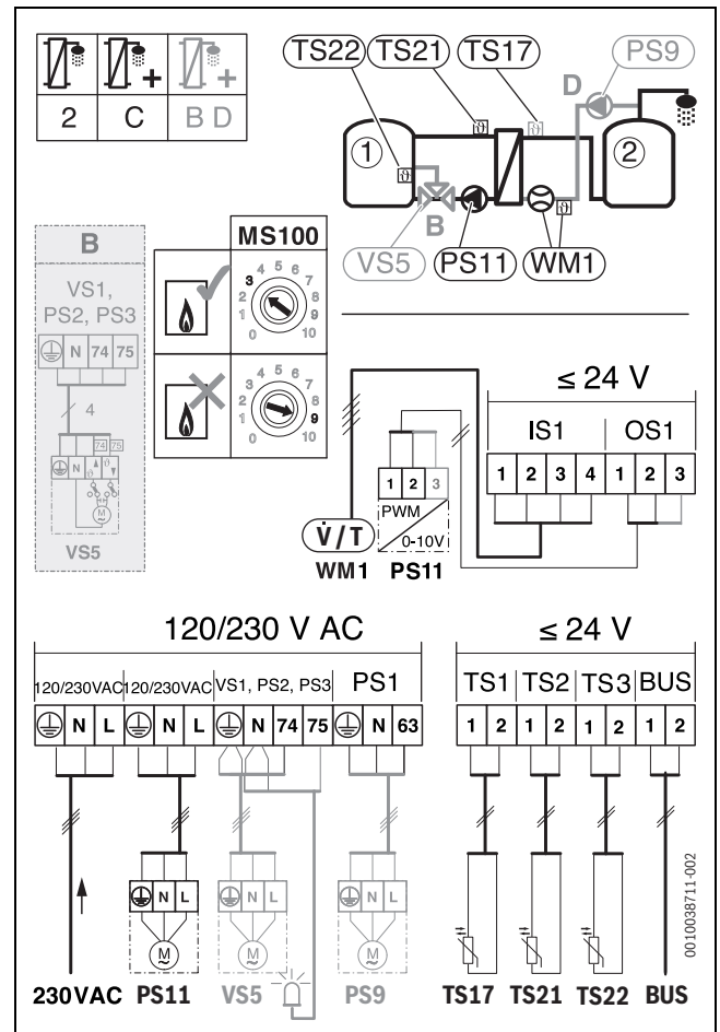
Bild 48 Anschlussklemmen bei Vorwärm-Frischwasserstation
