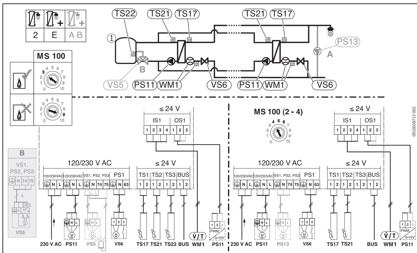
Bild 49 Anschlussklemmen bei Frischwasserstation Kaskade
