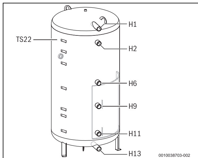
Bild 36 Pufferspeicher als Solarspeicher (getrenntes Volumen), Hydraulik (→ Bild 6, Seite 7)
