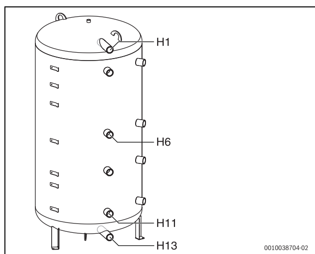
Bild 37 Pufferspeicher als Solarspeicher für Vorwärmesystem (auch mit internem Wärmetauscher möglich), Hydraulik (→ Bild 7, Seite 8)
