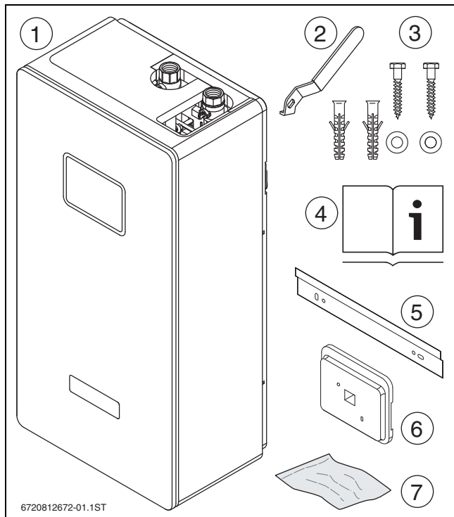
Bild 2 Lieferumfang Einzelstation
