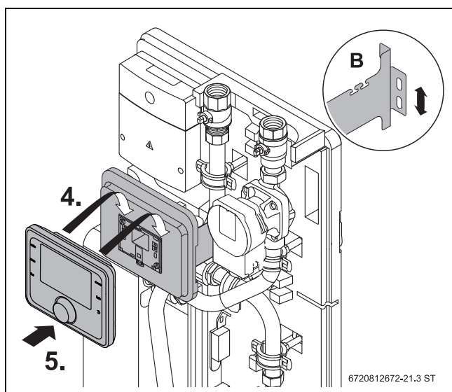
Bild 39 Bedieneinheit montieren
