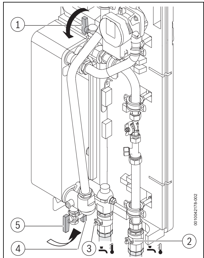
Bild 56 Spül- / Befüllleinrichtungen an der Einzelstation
