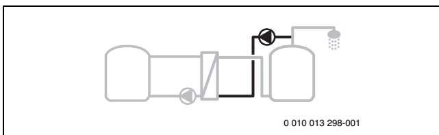
Bild 44 Tägliche Aufheizung
