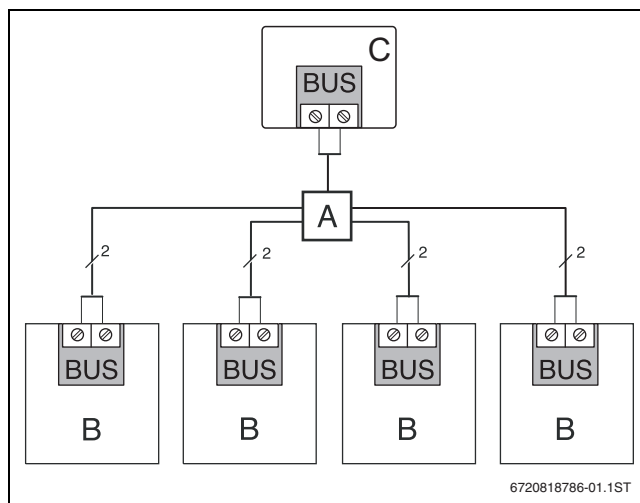
Bild 54 BUS-Leitungen anschließen
