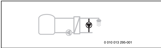
Bild 41 Zirkulation
