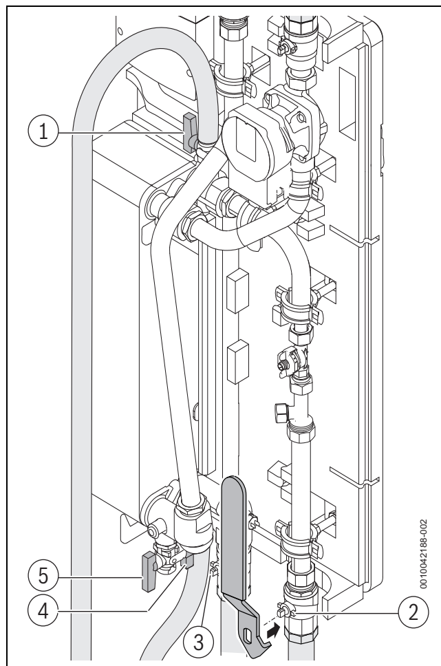
Bild 64 Wartung Frischwasserstation
