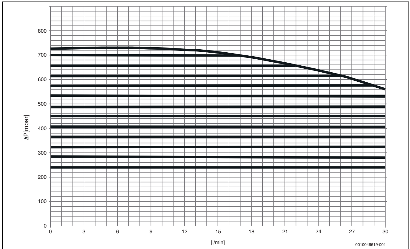
Bild 50 Leistungsdiagramm für Pumpe PC0
