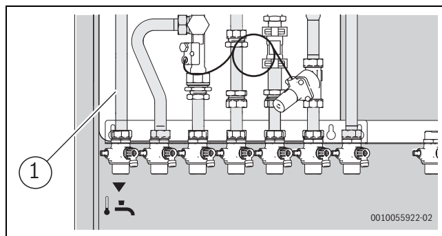
Bild 21 Kaltwasserabgang anschließen oder demontieren
