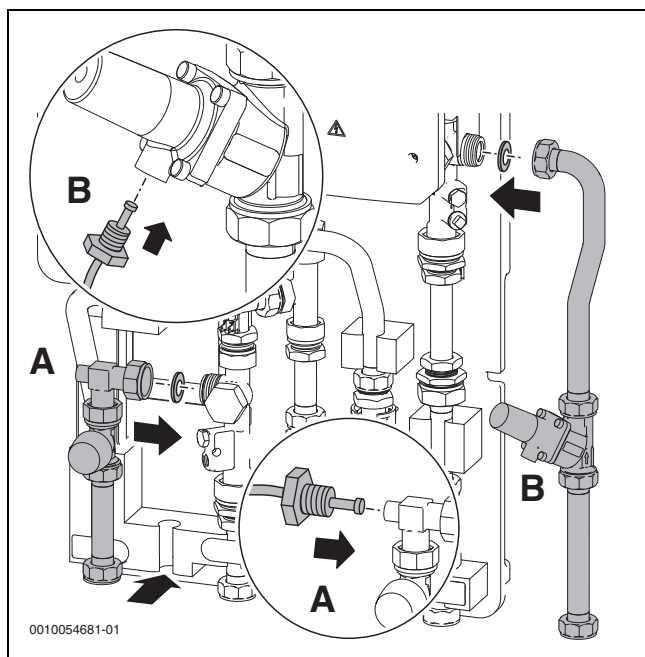
Bild 24 Vor- und Rücklaufrohr montieren
