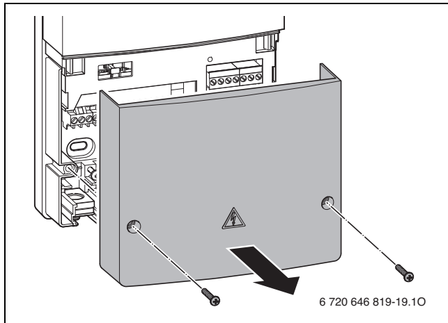
Bild 35 Modul öffnen
