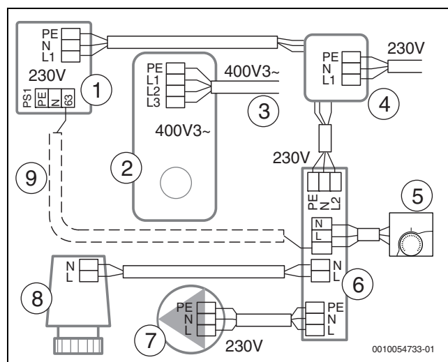
Bild 34 Übersicht Baugruppen und elektrische Verdrahtung
