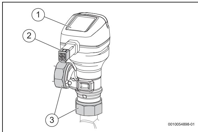
Bild 63 Regelventil
