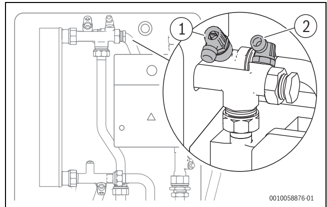
Bild 43 Warmwasser- und Heizkreis/Primärkreis entlüften
