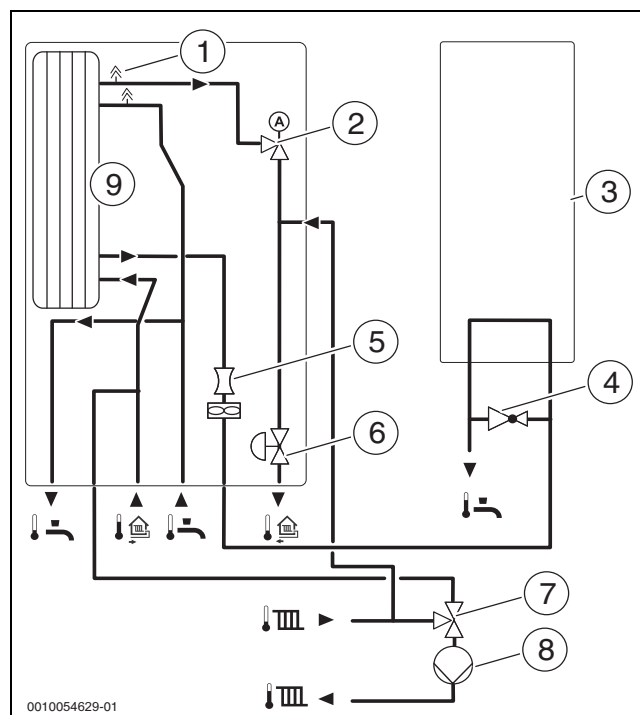
Bild 8 Gemischter Heizkreis
