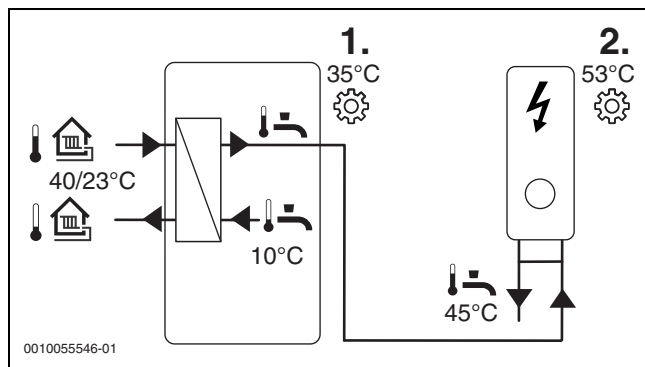
Bild 50 Schematische Darstellung der Wassererwärmer
