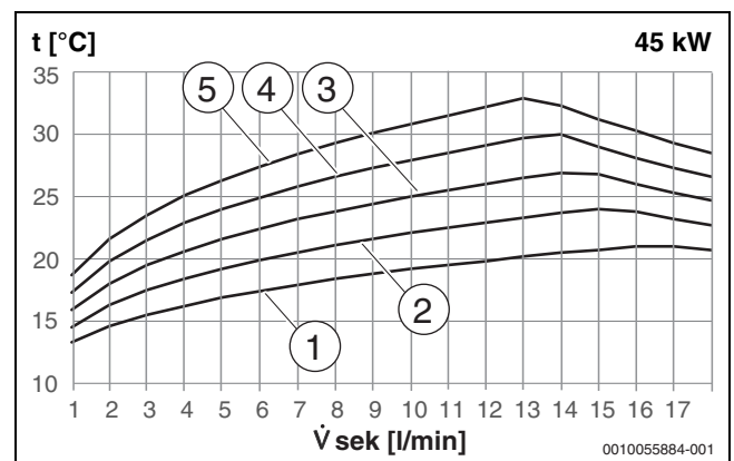
Bild 14 45 kW - Primäre Rücklauftemperatur in Abhängigkeit der primären Vorlauftemperatur und Zapfrate (l/min)
