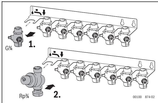
Bild 22 Druckminderer montieren
