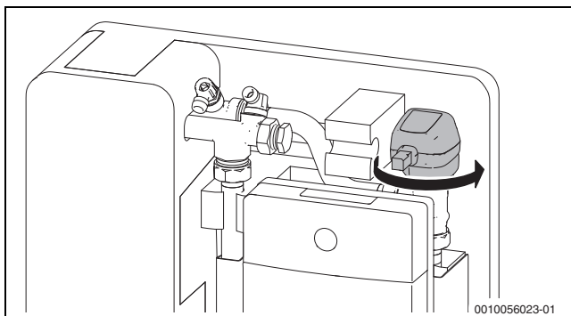
Bild 52 Regelventil vorsichtig nach rechts drehen
