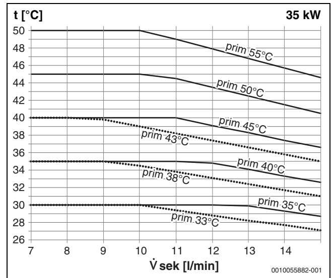
Bild 12 35 kW - Warmwassertemperatur in Abhängigkeit der primären Vorlauftemperatur und Zapfrate (l/min)
