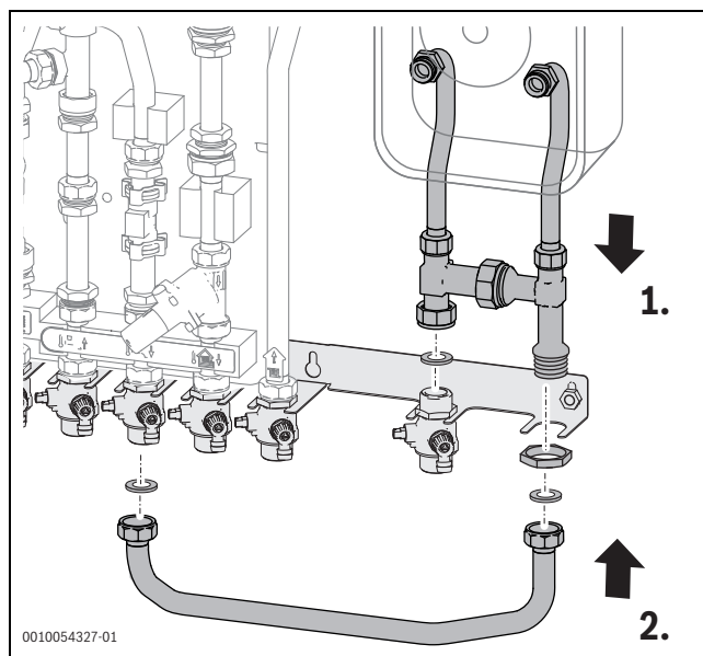
Bild 27 Verbindungsmodul montieren
