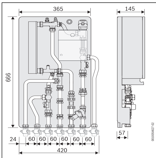
Bild 4 Abmessungen der Station
