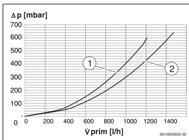
Bild 7 Druckverlust Primärseite
