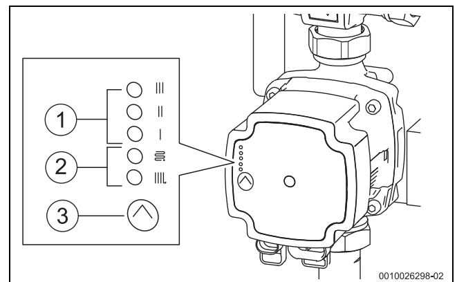
Bild 54 Statusanzeigen der integrierten Heizungspumpe
