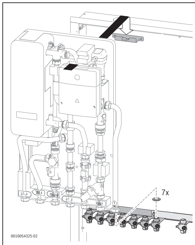
Bild 26 Basismodul aufhängen
