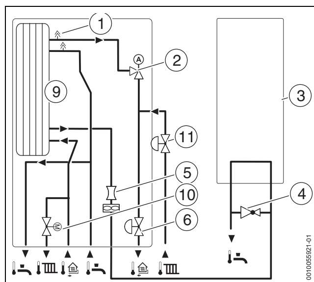
Bild 9 Ungemischter Heizkreis
