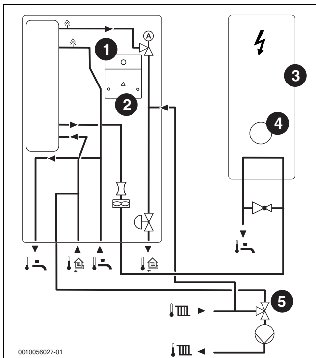
Bild 44 Übersicht der Komponenten mit Einstellungsmöglichkeiten
