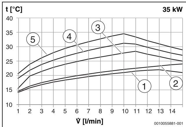
Bild 11 35 kW - Primäre Rücklauftemperatur in Abhängigkeit der primären Vorlauftemperatur und Zapfrate (l/min)
