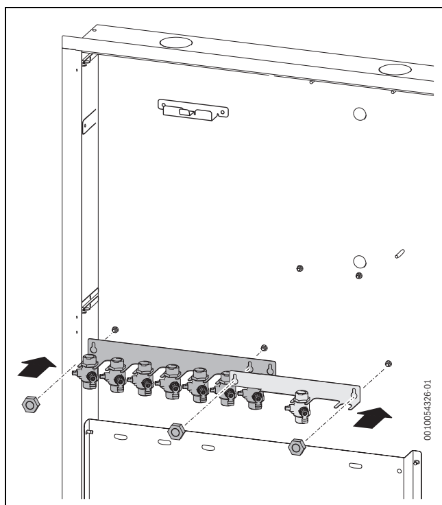
Bild 25 Montageanschlussplatten montieren
