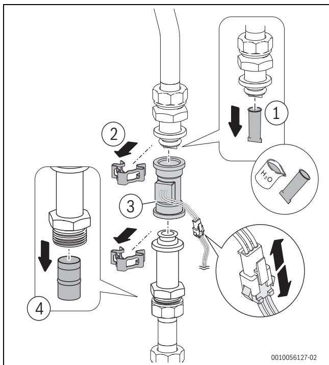
Bild 62 Durchflussbegrenzer und Durchflussturbine (Durchfluss 35 kW: 15 l/min, unten lila / 45 kW: 18 l/min, unten rot)
