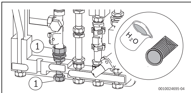
Bild 58 Filter Primärseite reinigen
