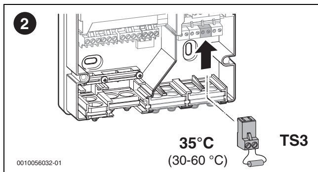
Bild 46 Option: Warmhaltefunktion mittels Widerstand aktivieren
