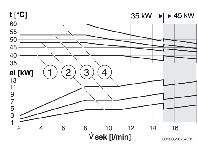
Bild 18 45 °C Vorlauf Primärkreis / 40 °C am Modul eingestellt
