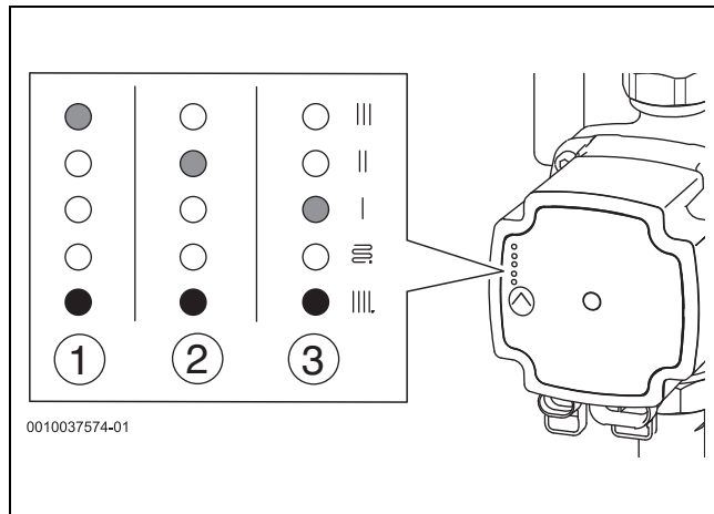
Bild 65 Störungsanzeigen der integrierten Heizungspumpe
