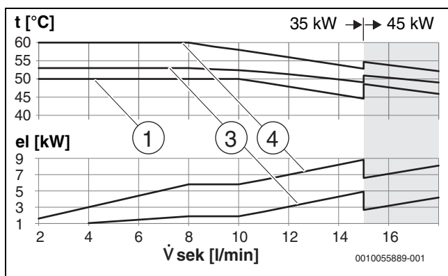
Bild 20 55 °C Vorlauf Primärkreis / 50 °C am Modul eingestellt
