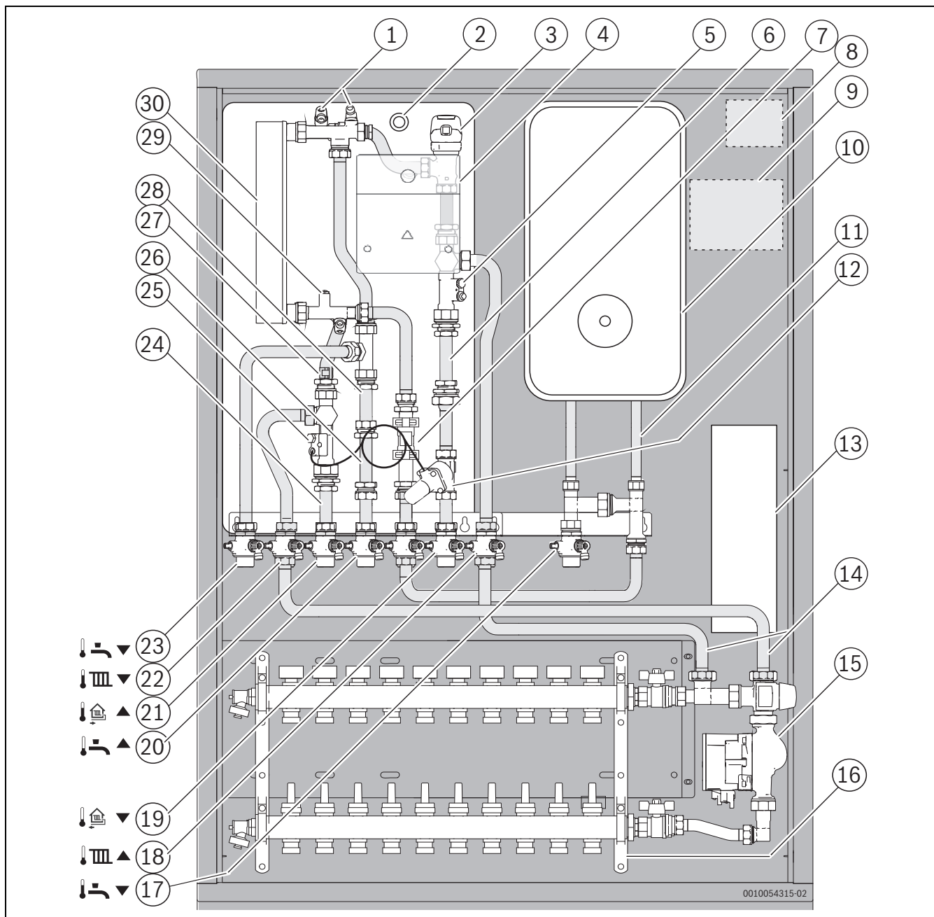
Bild 2 Beispiel: Station mit elektrischen Durchlauferhitzer und gemischter Heizkreis im Unterputzschrank
