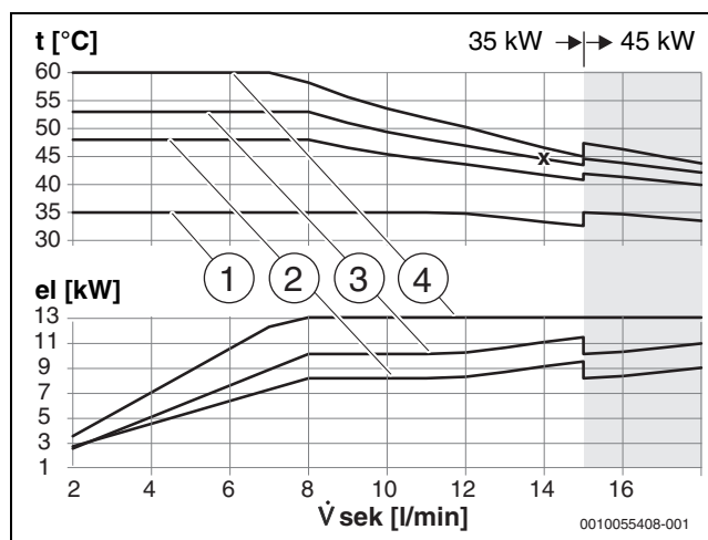
Bild 17 40 °C Vorlauf Primärkreis / 35 °C am Modul eingestellt
