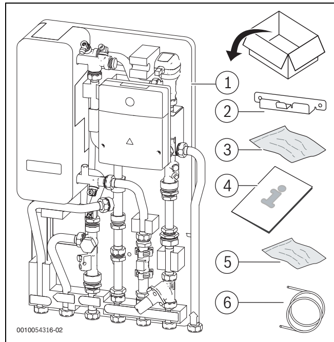
Bild 1 Lieferumfang Wohnungsstation
