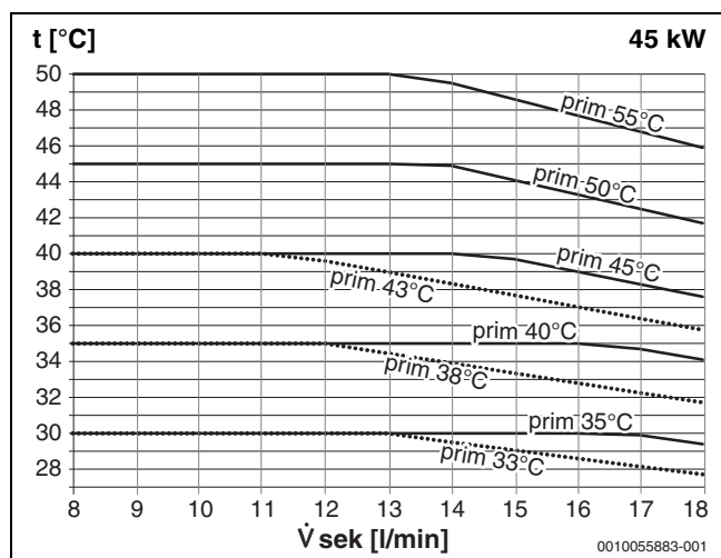
Bild 15 45 kW - Warmwassertemperatur in Abhängigkeit der primären Vorlauftemperatur und Zapfrate (l/min)
