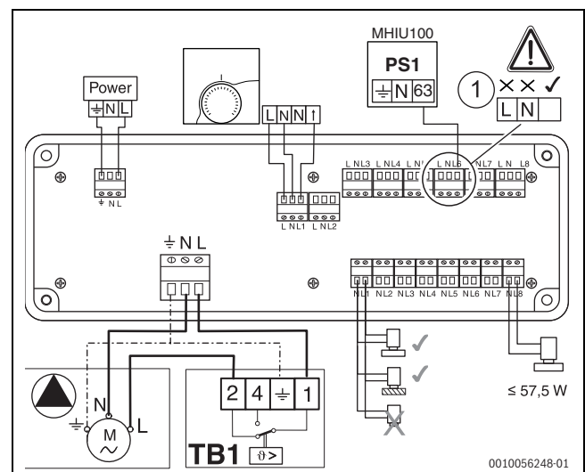
Bild 38 Elektrischer Anschluss Pumpenkick-Funktion (Option)
