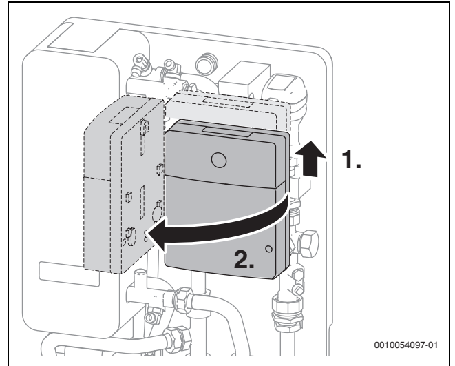
Bild 59 Modul in Wartungsstellung umsetzen
