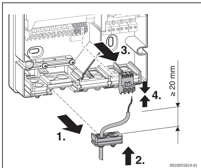
Bild 39 Kabel vom Heizkreisverteiler anschließen
