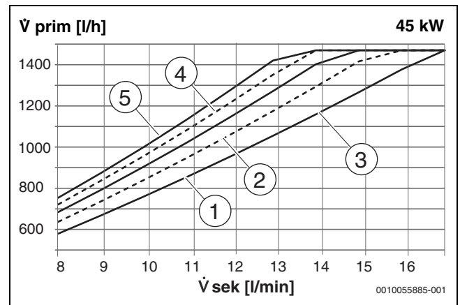
Bild 13 45 kW - Primärer Volumenstrom in Abhängigkeit der Primärtemperatur und Zapfrate (l/min)
