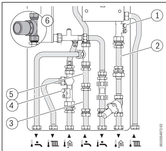
Bild 33 Adapterrohre ersetzen
