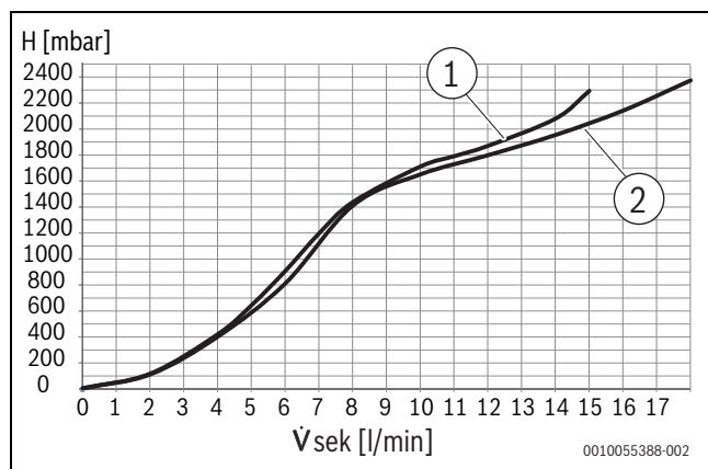
Bild 6 Druckverlust Trinkwasserseite Wohnungsstation mit Durchlauferhitzer
