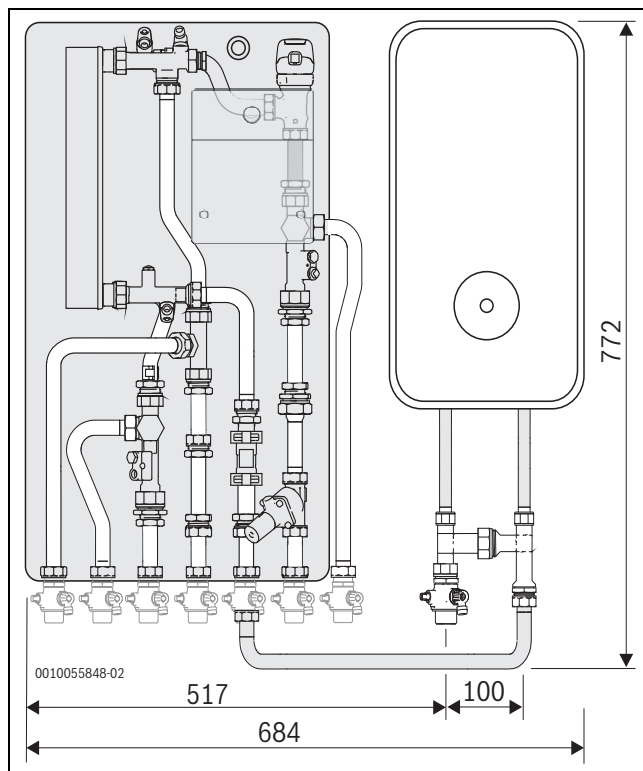
Bild 5 Abstände Station und elektrischer Durchlauferhitzer
