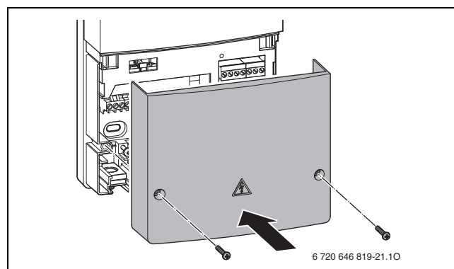
Bild 42 Abdeckung montieren
