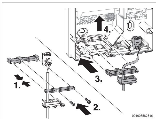
Bild 40 Zugentlastungen montieren und Stecker einstecken
