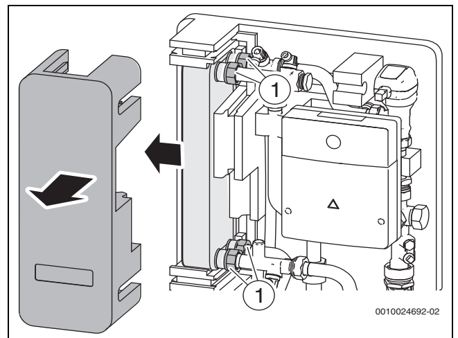
Bild 60 Wärmetauscher demontieren
