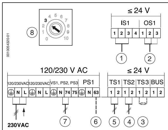
Bild 36 Anschlussklemmen am Modul MHIU100
