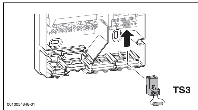
Bild 41 Stecker mit Widerstand montieren
