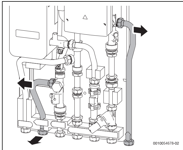
Bild 23 Vor- und Rücklaufrohr demontieren
