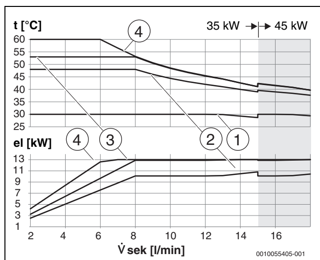
Bild 16 35 °C Vorlauf Primärkreis / 30 °C am Modul eingestellt
