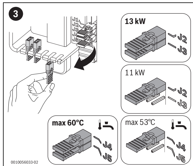
Bild 47 Leistung des Durchlauferhitzers und max. Warmwassertemperatur mittels Brücke einstellen (ab Werk: 13 kW, max 60°C)
