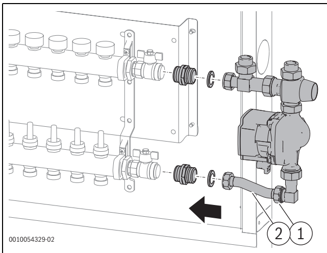
Bild 29 Rückwand des Heizkreismoduls aufhängen
