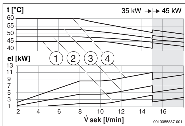
Bild 19 50 °C Vorlauf Primärkreis / 45 °C am Modul eingestellt
