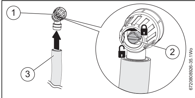
Bild 57 Entleerungsanschluss
