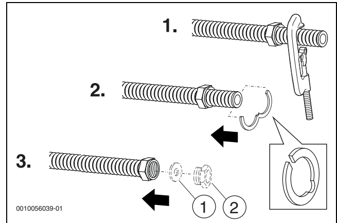
Bild 30 Edelstahlwellrohre bei Bedarf einkürzen
