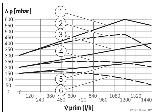
Bild 55 Proportionaldruck-Kennlinien
