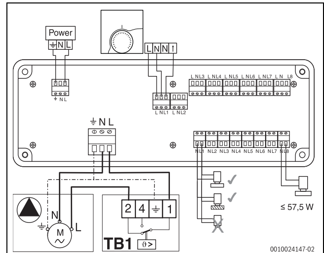
Bild 37 Elektrischer Anschluss an die Klemmleiste Fußbodenheizung (Zubehör)
