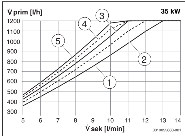
Bild 10 35 kW - Primärer Volumenstrom in Abhängigkeit der Primärtemperatur und Zapfrate (l/min)
