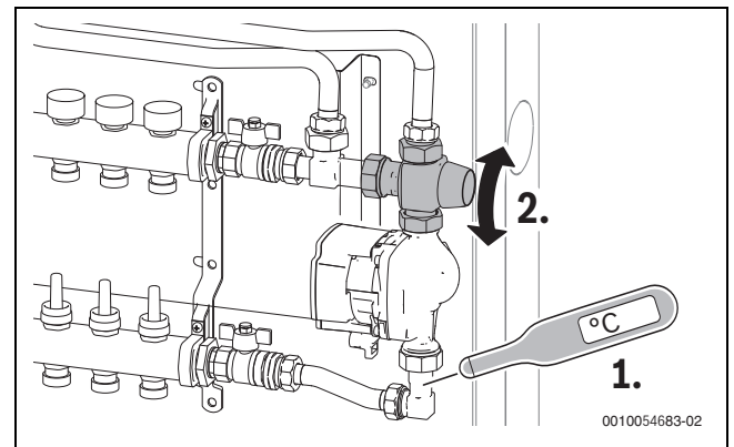
Bild 53 Maximale Vorlauftemperatur einstellen
