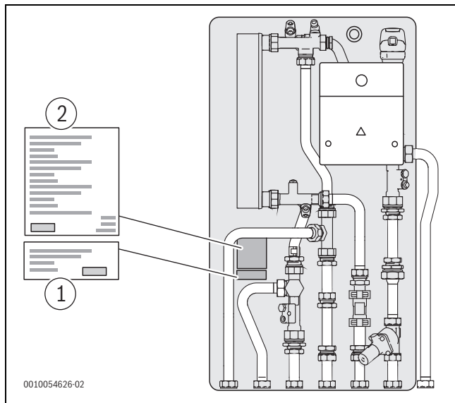
Bild 3 Typschild und Datenschild
