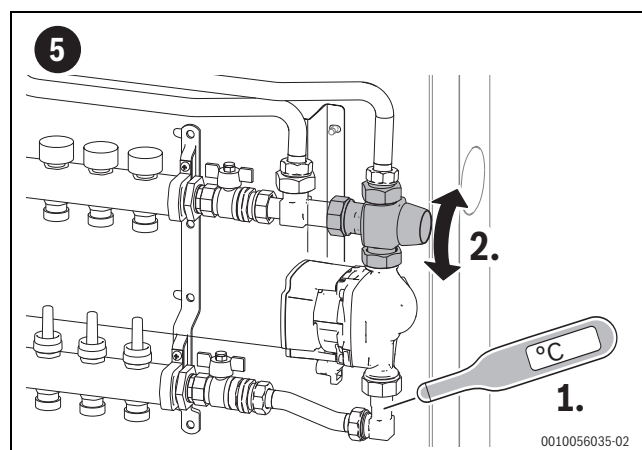
Bild 49 Gewünschte max. Vorlauftemperatur einstellen
