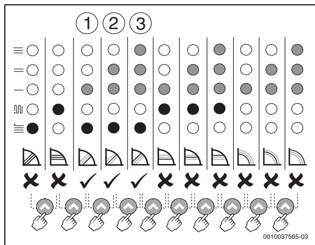
Bild 56 Einstellung der Pumpenkennlinie
