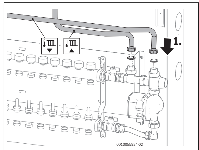
Bild 31 Verbindungsrohre mit Dichtung an Heizkreispumpe schrauben
