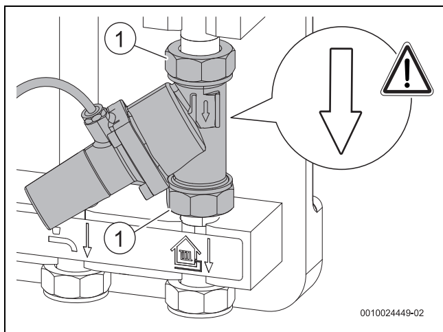
Bild 61 Differenzdruckregler
