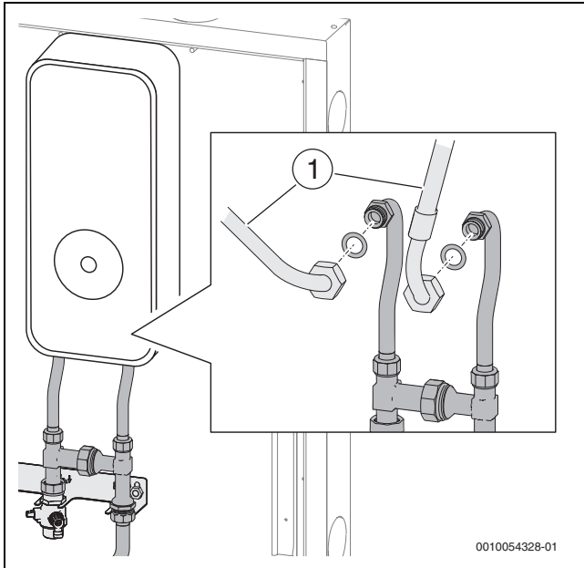
Bild 28 Anschlüsse verschrauben
