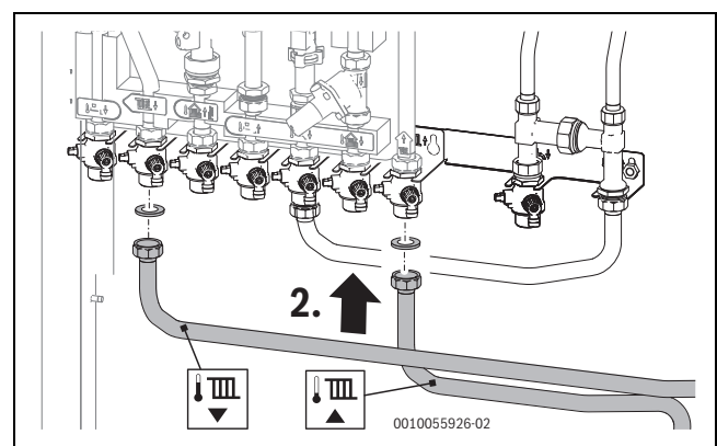
Bild 32 Verbindungsrohre mit Dichtung an Station schrauben
