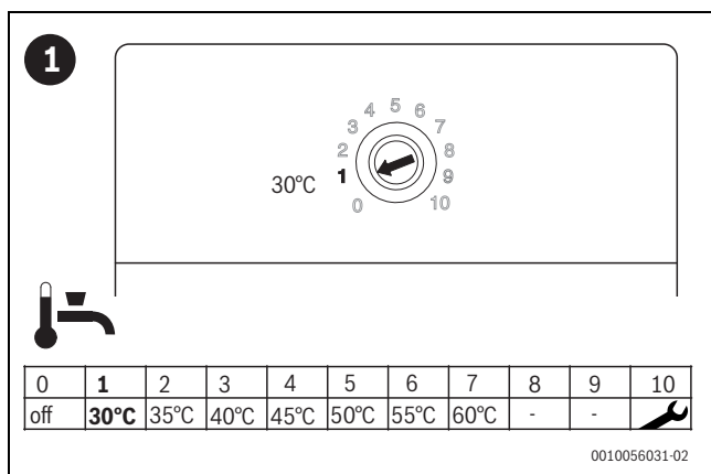
Bild 45 Warmwassertemperatur am Modul (ab Werk: 30 °C)
