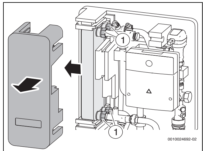
Bild 53 Wärmetauscher demontieren
