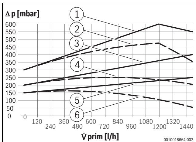
Bild 46 Proportionaldruck-Kennlinien
