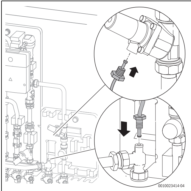
Bild 30 Kapillarleitung montieren
