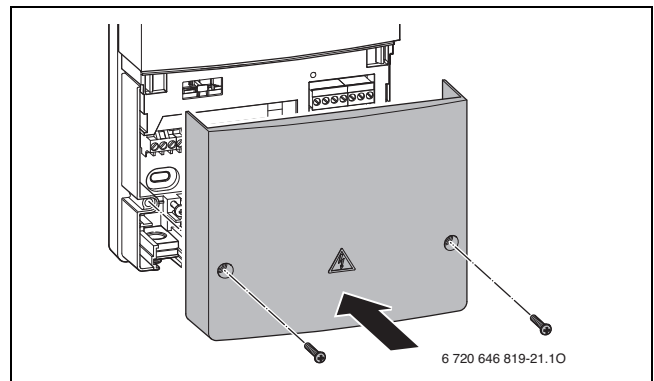
Bild 40 Abdeckung montieren
