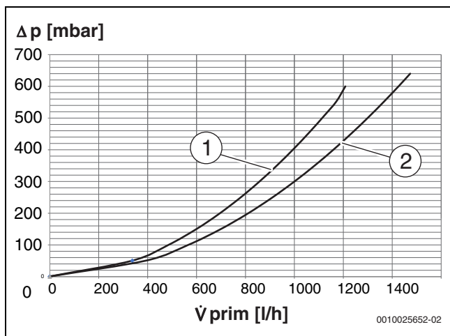
Bild 7 Druckverlust Primärseite
