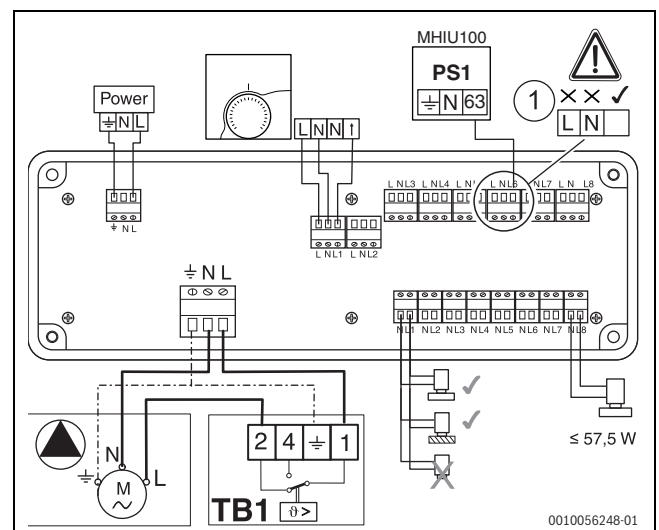
Bild 36 Elektrischer Anschluss Pumpenkick-Funktion (Option)
