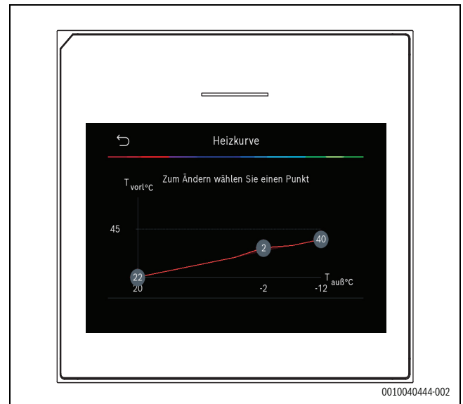
Bild 1 Startbildschirm für die Einstellung der Heizkurve für die Regelungsart Außentemperatur mit Fußpunkt (und Komfortpunkt)
