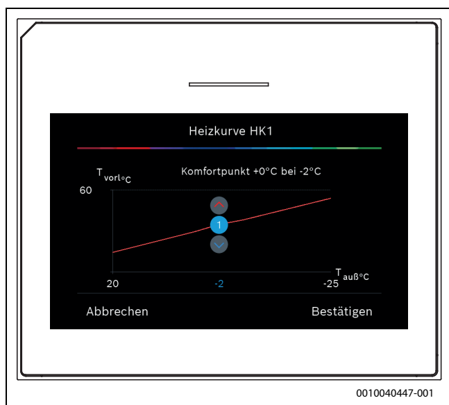
Bild 4 Komfortpunkt einstellen (nur wenn der Regelungstyp auf Außenlufttemperaturführung mit Fußpunkt eingestellt ist)
