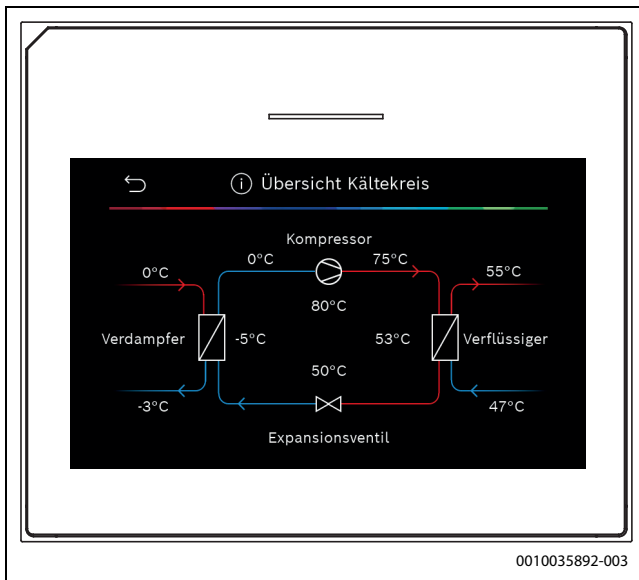
Bild 10 Übersicht Kühlkreis
