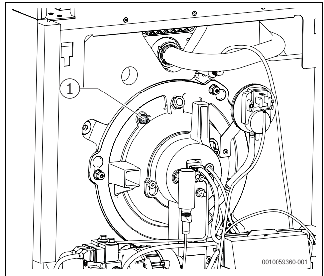
Bild 81 Druckmessstelle am Brenner
