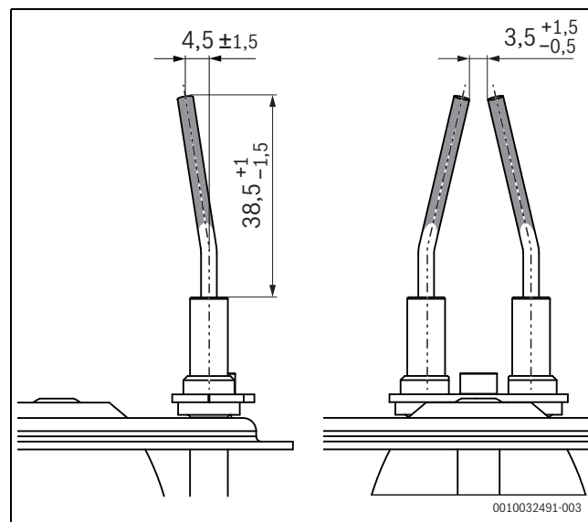
Bild 103 Zündelectrode, Maße in mm
