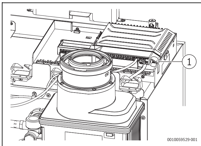
Bild 42 Netzanschluss herstellen
