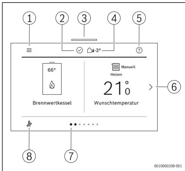
Bild 49 Bedienfeld
