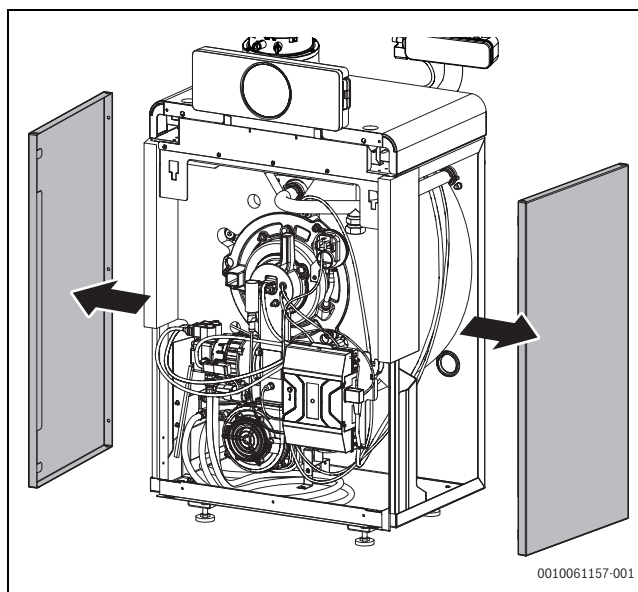
Bild 12 Seitenwände abnehmen
