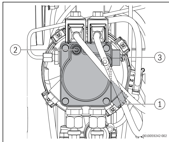
Bild 59 Druck einstellen - Ölpumpe Suntec
