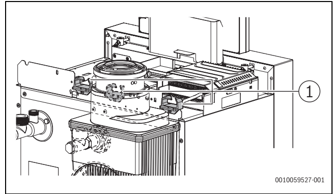
Bild 39 Kabel verlegen
