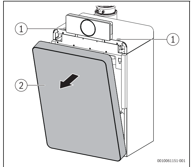
Bild 8 Kesselvorderwand demontieren
