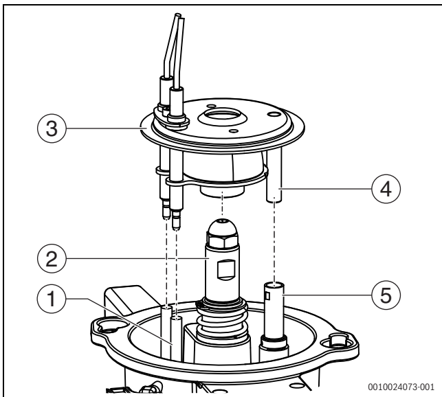
Bild 72 Mischsystem montieren
