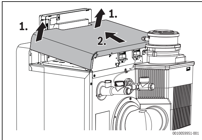
Bild 37 Kesselhaube abnehmen
