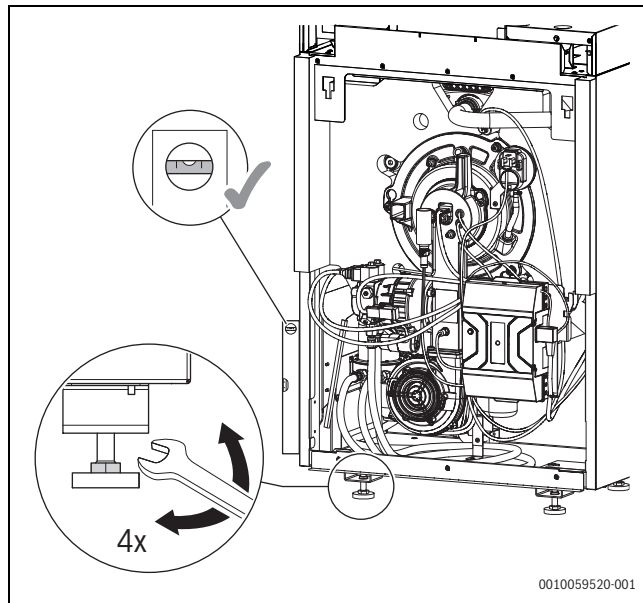
Bild 19 Heizkessel ausrichten
