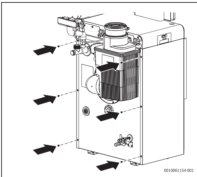
Bild 15 Seitenwände befestigen
