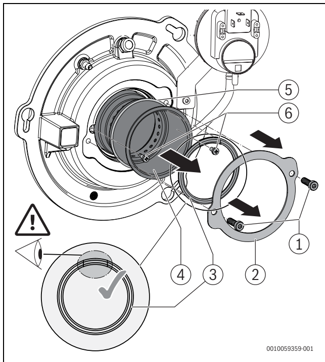
Bild 77 Brennerrohr austauschen
