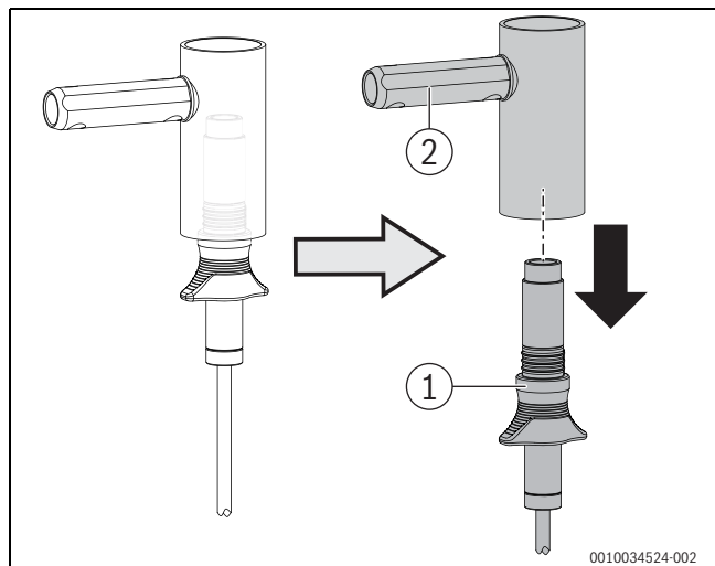
Bild 88 Flammpfeifenreiniger demontieren
