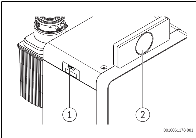
Bild 100 Geräteversicherung am Regelgerät IMX 45 mit Bedienfeld UI 800
