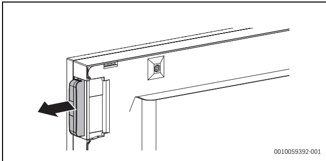
Bild 47 Kommunikationsmodul demontieren
