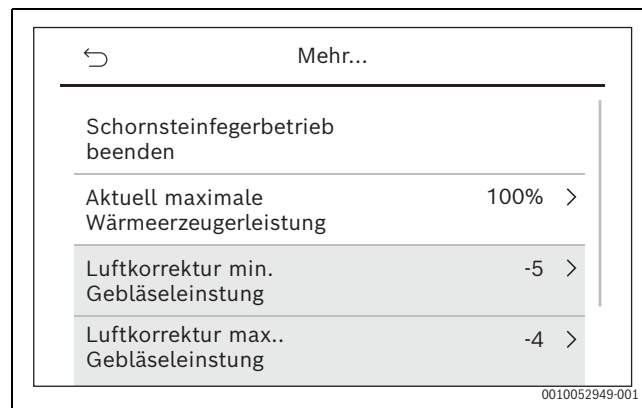
Bild 58 Luftkorrektur/Gebläsedrehzahl einstellen
