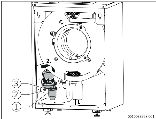
Bild 79 Ölfilter demontieren
