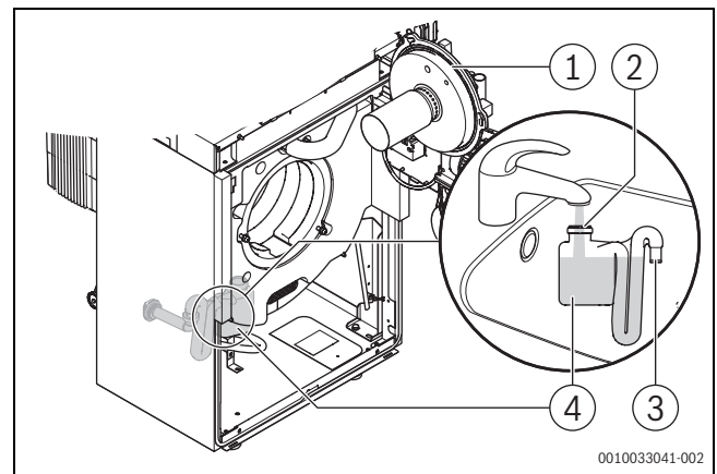
Bild 85 Siphon reinigen
