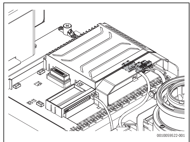
Bild 25 Gehäuseklemmenabdeckung abnehmen
