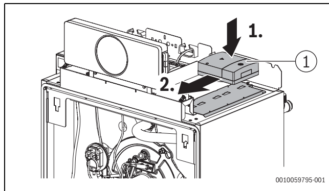
Bild 43 Funktionsmodule einstecken
