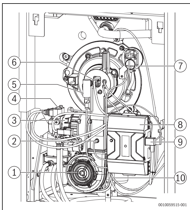
Bild 96 Ölbrenner
