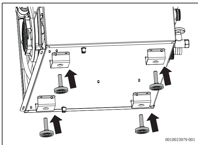
Bild 18 Stellfüße montieren
