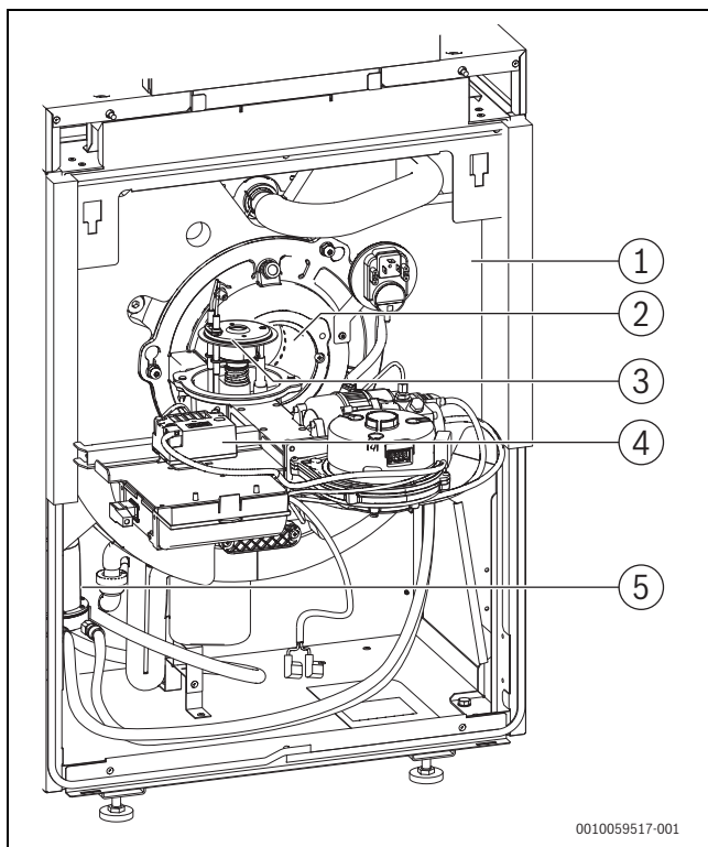
Bild 98 Ölbrenner in Serviceposition 2
