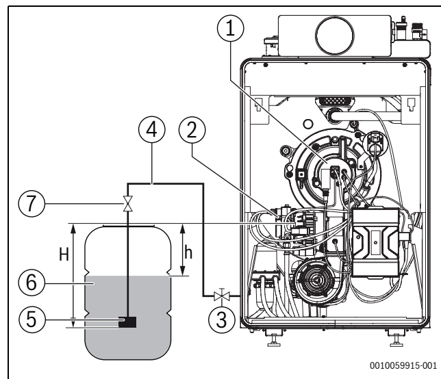
Bild 31 Ölversorgungseinrichtung, Öltank unterhalb der Ölpumpe
