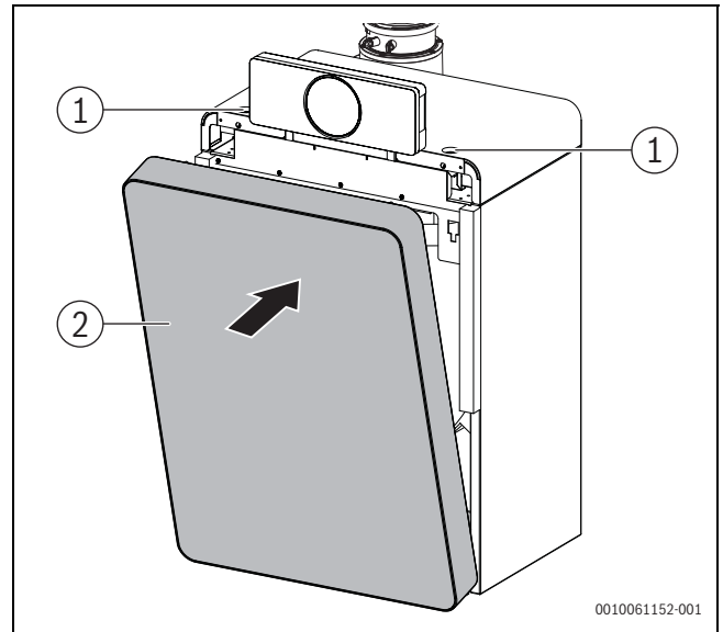
Bild 16 Kesselvorderwand montieren
