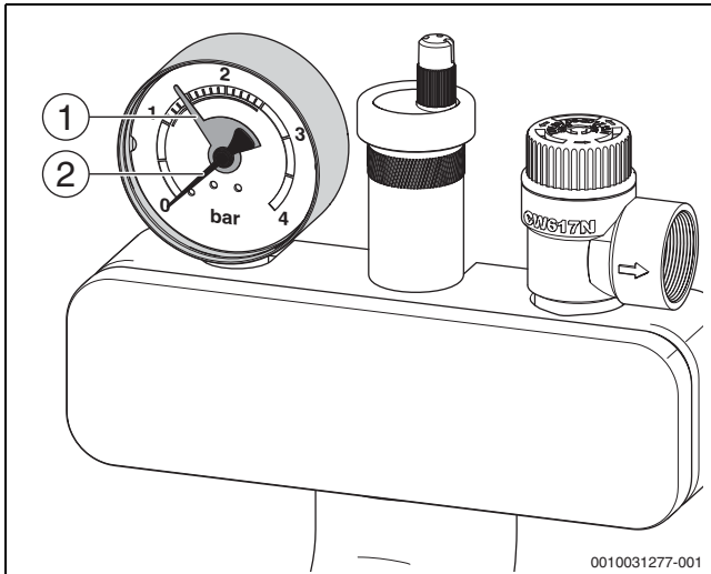
Bild 86 Manometer
