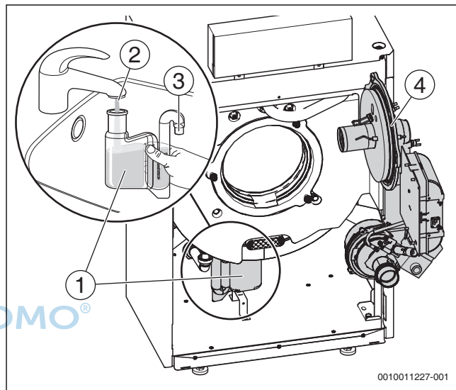
Bild 76 Siphon reinigen
