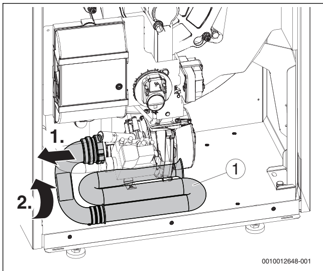
Bild 66 Ausbau Verbrennungsluft-Ansaugrohr
