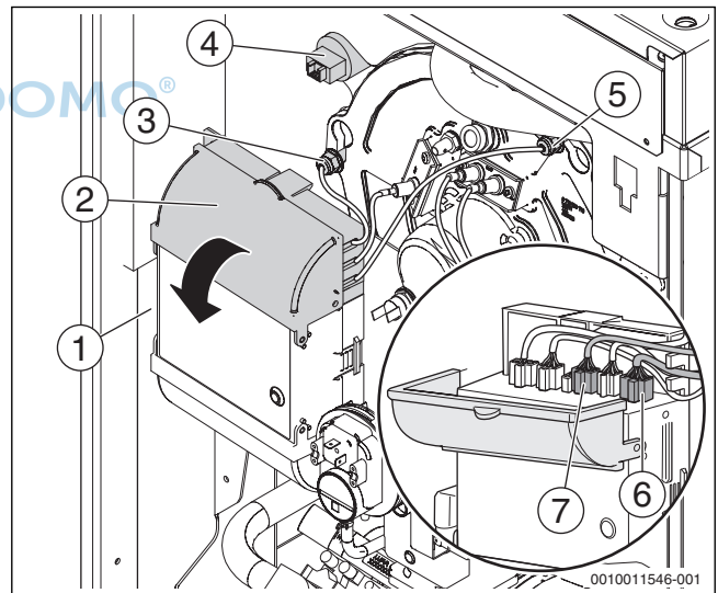
Bild 65 Steckverbinder lösen
