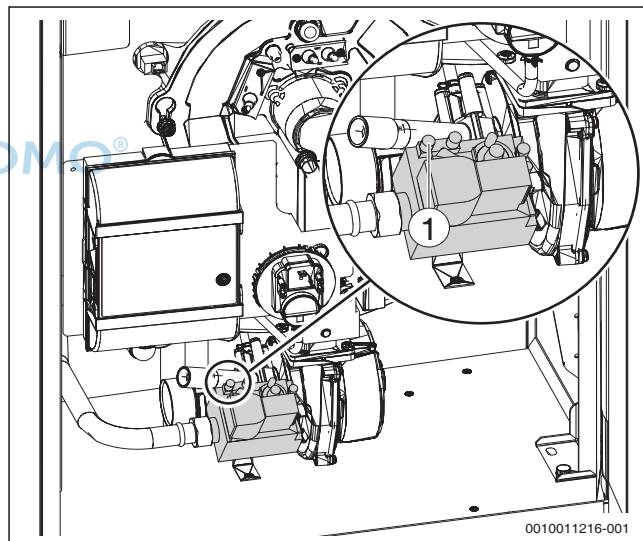
Bild 37 Gasleitung entlüften
