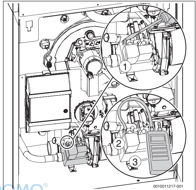
Bild 54 Gas-Anschlussdruck messen
