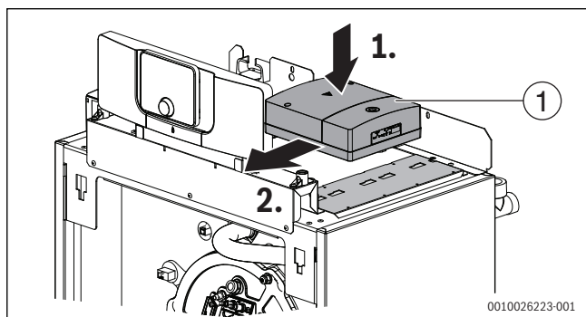
Bild 27 Funktionsmodule einstecken
