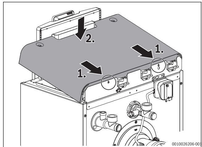
Bild 25 Kesselhaube montieren
