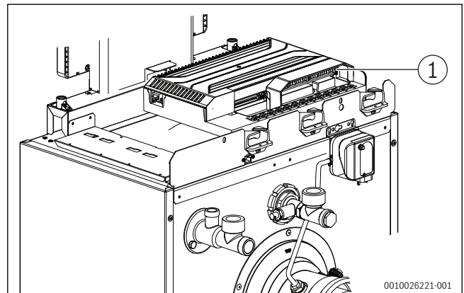
Bild 26 Netzanschluss herstellen
