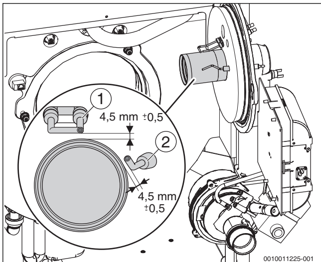
Bild 75 Abstände Elektroden
