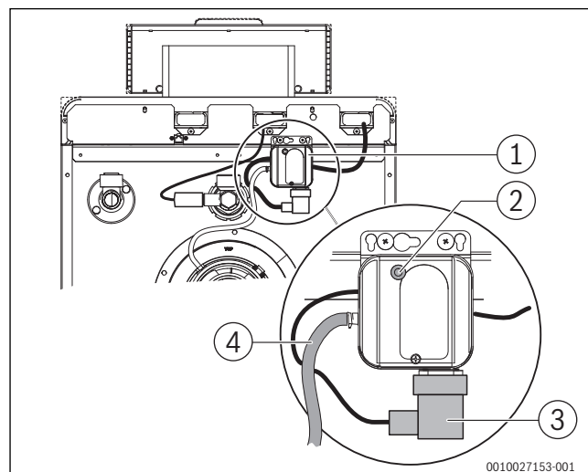
Bild 86 Abgas-Druckwächter
