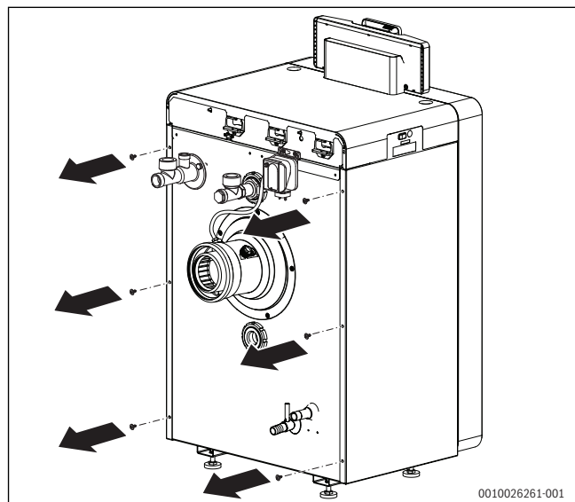
Bild 77 Befestigungsschrauben lösen
