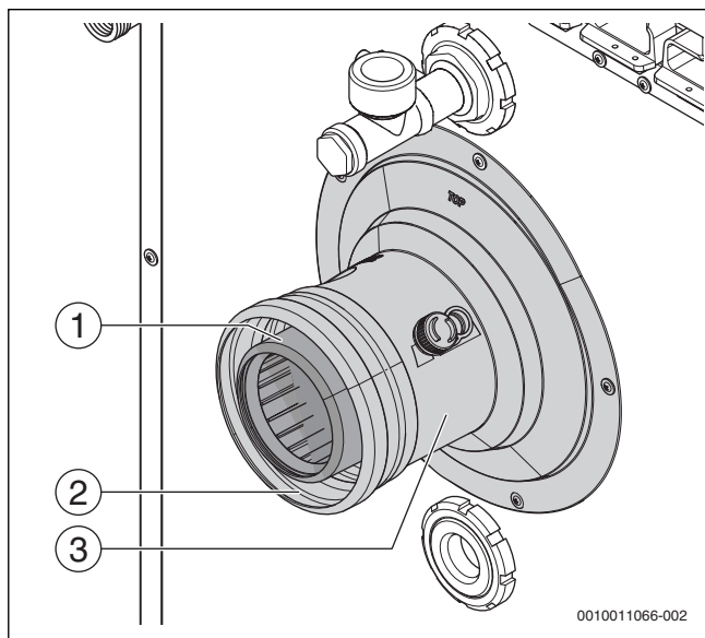
Bild 11 Abgasanschluss montieren
