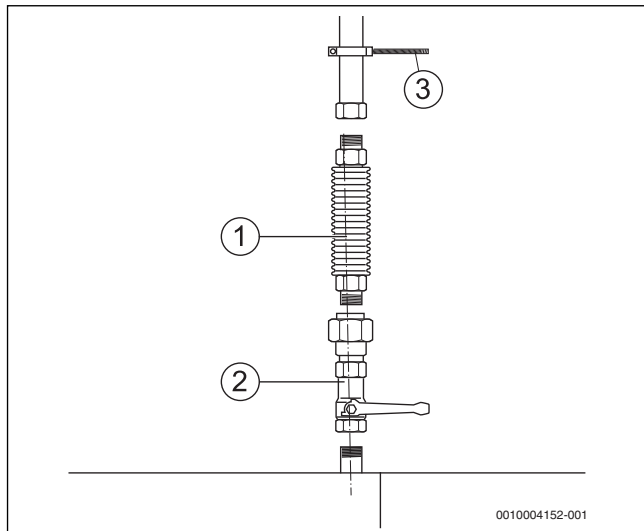
Bild 18 Gasanschluss herstellen
