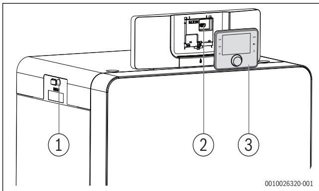
Bild 92 Gerätesicherung
