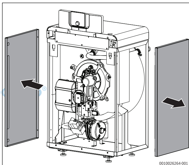
Bild 80 Seitenwände abnehmen
