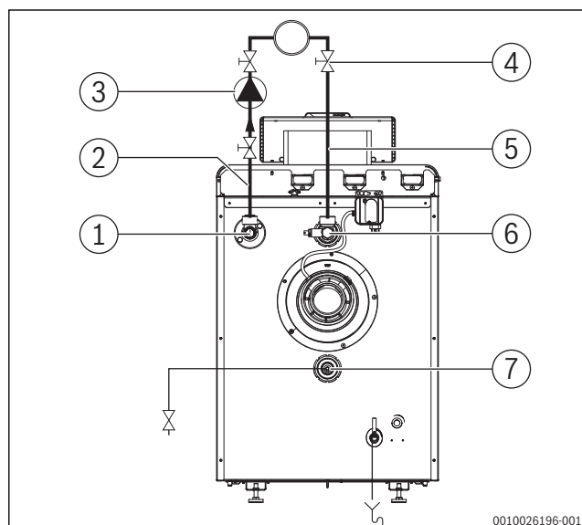
Bild 15 Anschlussschema Hydraulik
