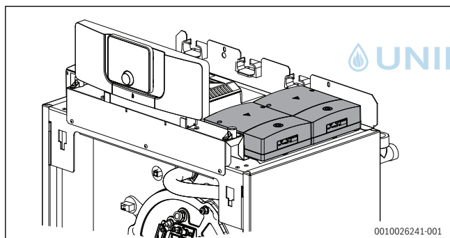
Bild 28 Standard-Funktionsmodule montiert
