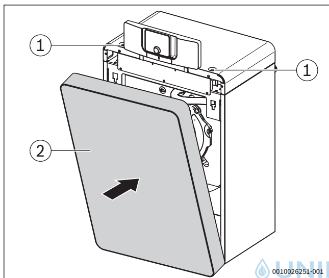
Bild 60 Kesselvorderwand montieren
