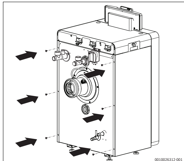
Bild 83 Seitenwände befestigen
