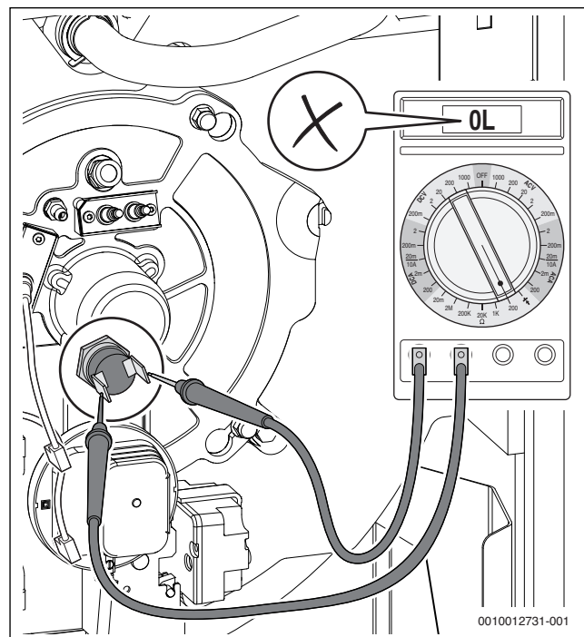
Bild 90 Elektrischen Widerstand an den Kontakten des Temperaturwächters messen (Temperaturwächter nicht in Ordnung)
