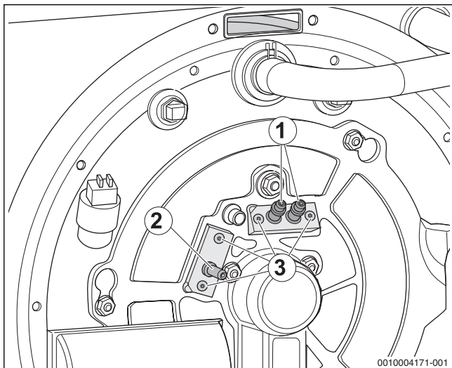
Bild 74 Elektrodenposition
