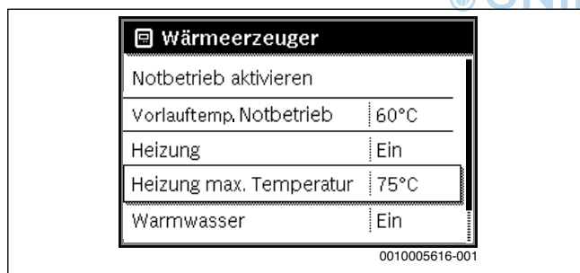
Bild 45 Maximale Vorlauftemperatur
