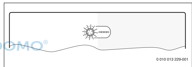
Fig. 18 interruptor codificador con visualización de estado del módulo y visualización de estado de los módulos o generadores de calor conectados
