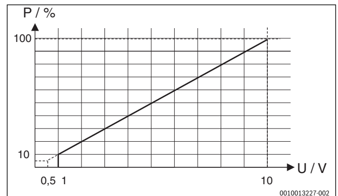
Afb. 22 Lineaire relatie tussen 0-10 V-sigtaal (U in Volt) en gevraagde vermogen P (in procenten gerelateerd aan het maximale vermogen van de installatie)
