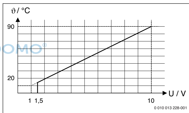
图 58 0-10V 信号 (U 单位为 V) 和要求的出水温度 \theta (单位为 °C, 以最低出水温度至最高出水温度的范围为 [基本设置 20 °C 至 90 °C]) 之间的线性关系
