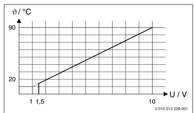
Afb. 44 Lineaire relatie tussen 0-10 V-sigitaal (U in Volt) en gevraagde aanvoertemperatuur ϑ (in °C gerelateerd aan het bereik minimale aanvoertemperatuur tot maximale aanvoertemperatuur [basisinstelling 20 °C tot 90 °C])
