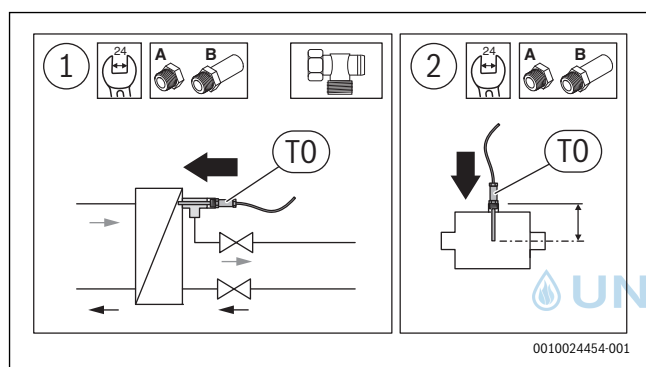
Afb. 45 Geoptimaliseerde sensormontage
