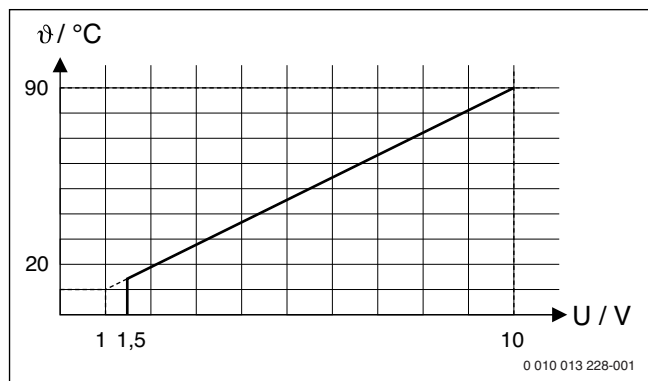
Fig. 30 Relation linéaire entre le signal 0-10 V (U en Volt) et la température de départ demandée \theta (en °C par rapport à la plage température de départ minimale à maximale [réglage de base 20 °C à 90 °C])
