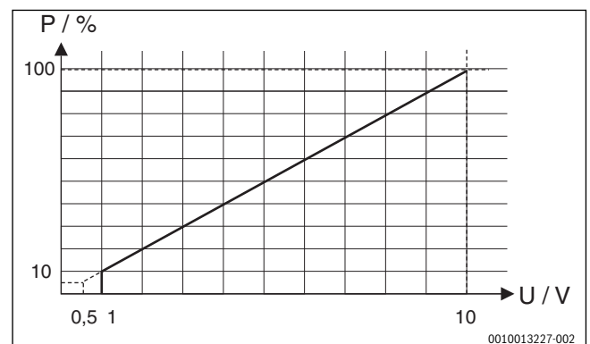
Afb. 43 Lineaire relatie tussen 0-10 V-sigitaal (U in Volt) en gevraagde vermogen P (in procenten gerelateerd aan het maximale vermogen van de installatie)
