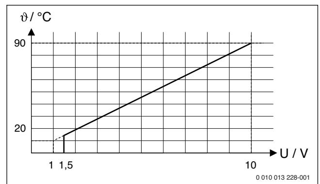
Afb. 23 Lineaire relatie tussen 0-10 V-sigtaal (U in Volt) en gevraagde aanvoertemperatuur ϑ (in °C gerelateerd aan het bereik minimale aanvoertemperatuur tot maximale aanvoertemperatuur [basisinstelling 20 °C tot 90 °C])
