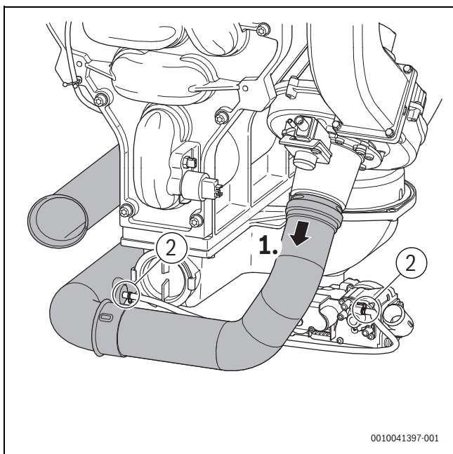
Bild 34 Entfernen des Luftsammlers
