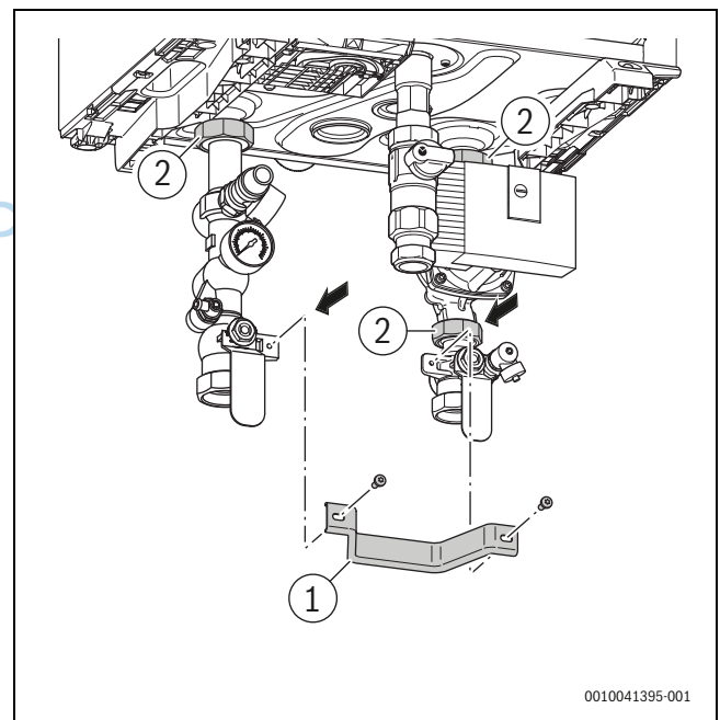
Bild 15 Bügel montieren
