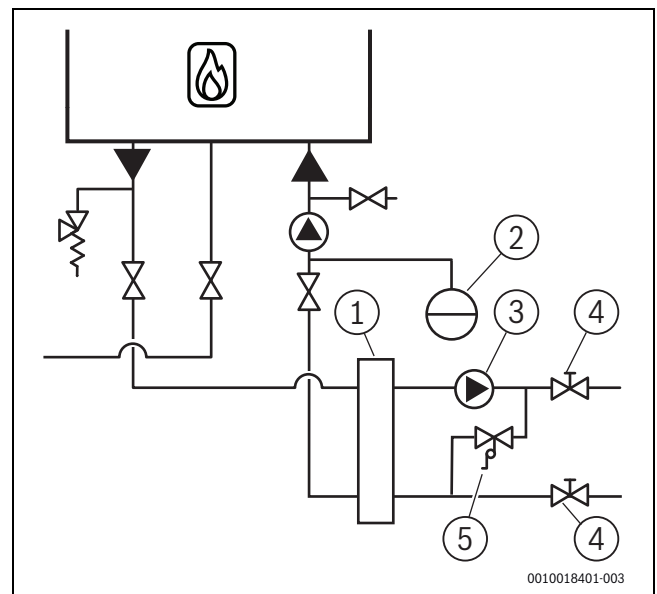
Bild 19 Aufstellung mit hydraulischer Weiche
