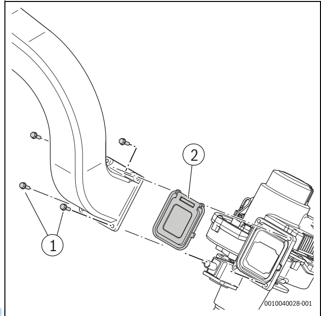
Bild 45 Ersetzen des Abgasrückschlagventils
