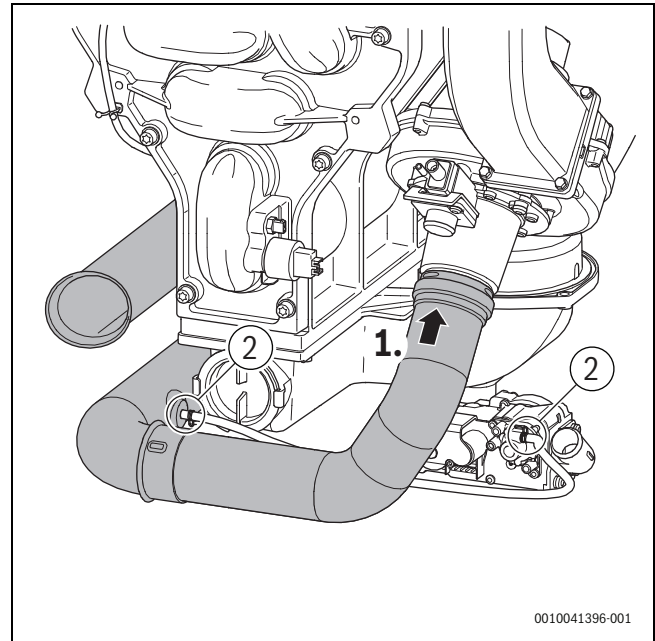
Bild 42 Kontrollieren der Anschlüsse des Druckausgleichsschlauchs
