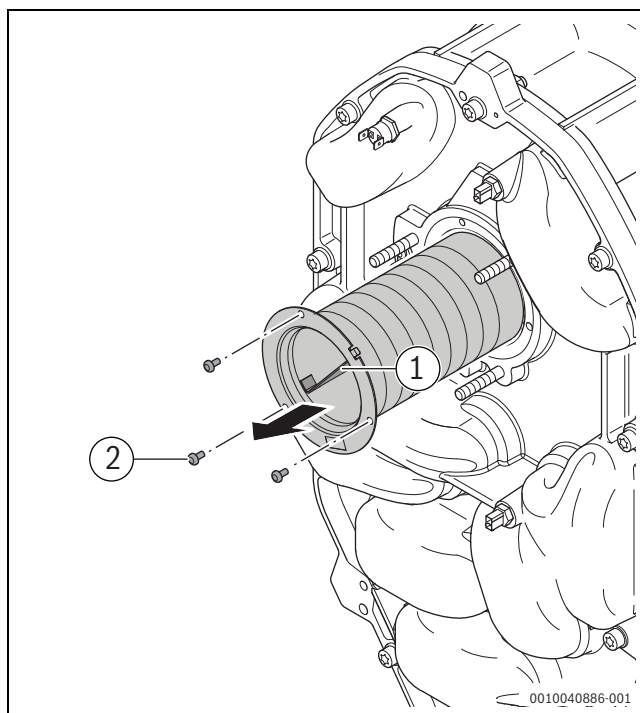
Bild 36 Demontieren des Brenners
