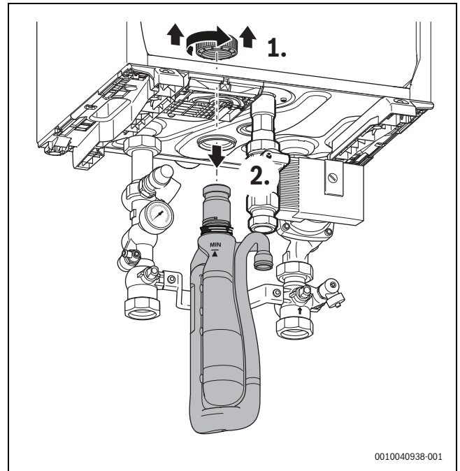
Bild 39 Kesselsiphon entfernen
