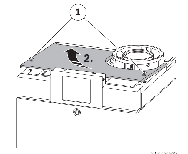
Bild 22 Öffnen der oberen Abdeckung
