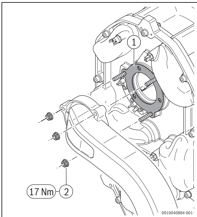
Bild 41 Montieren des Gas-Luft-Mischrohrs
