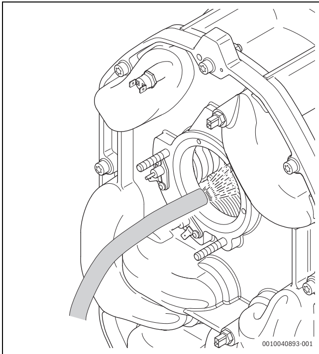
Bild 37 Spülen des Wärmetauschers
