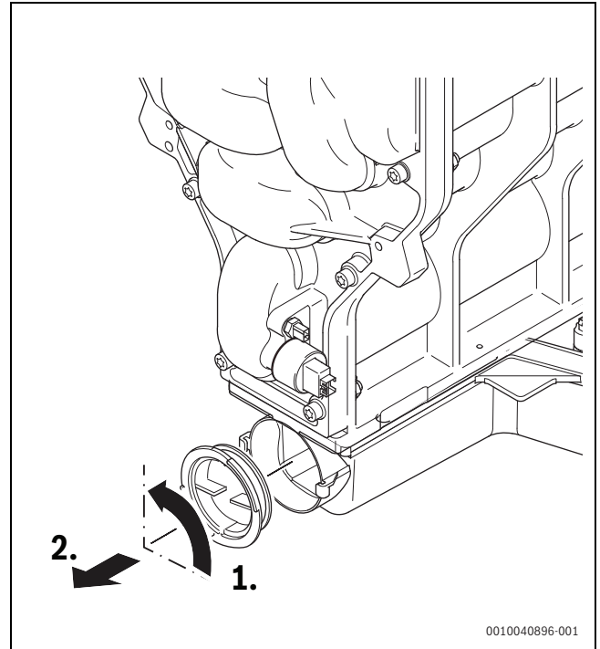
Bild 38 Den Deckel der Kondensatwanne öffnen.
