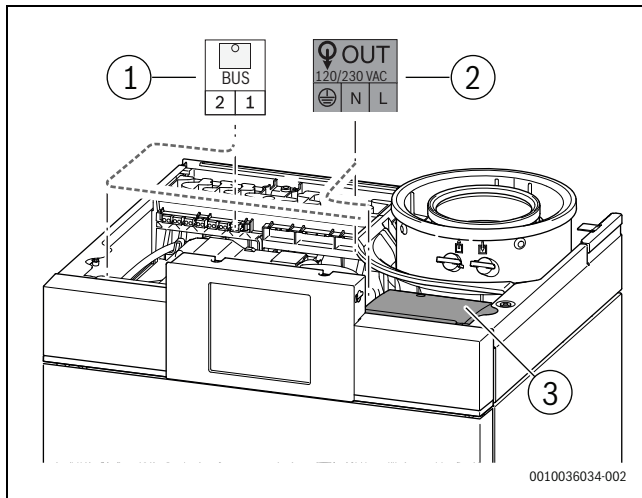
Bild 27 Montieren des Funktionsmoduls
