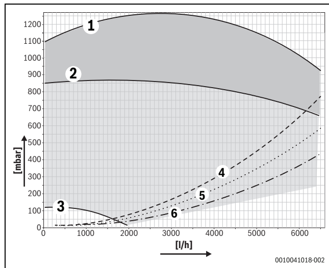
Bild 48 Restförderhöhe der Pumpe GC7000WP 125, GC7000WP 150
