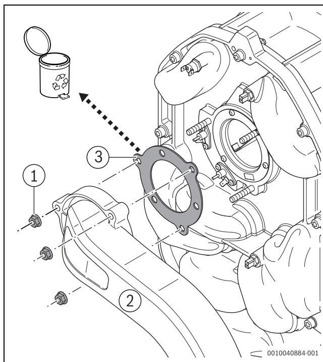
Bild 35 Gas-Luft-Mischrohr demontieren
