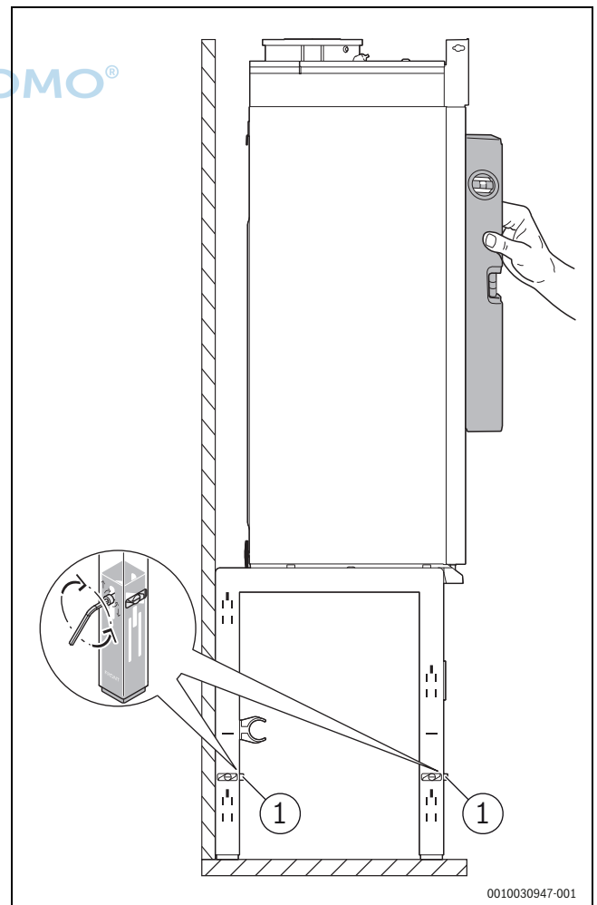
Bild 10 Ausrichten des Heizkessels auf dem Rahmen
