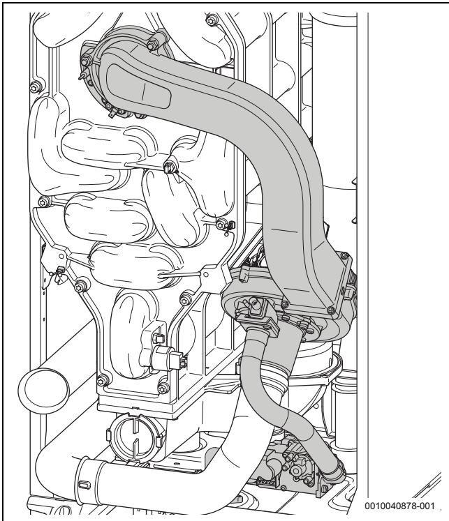
Bild 31 Prüfung des Gaswegs
