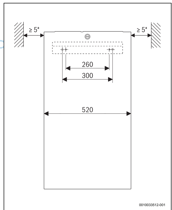
Bild 5 Vorderansicht [mm]
