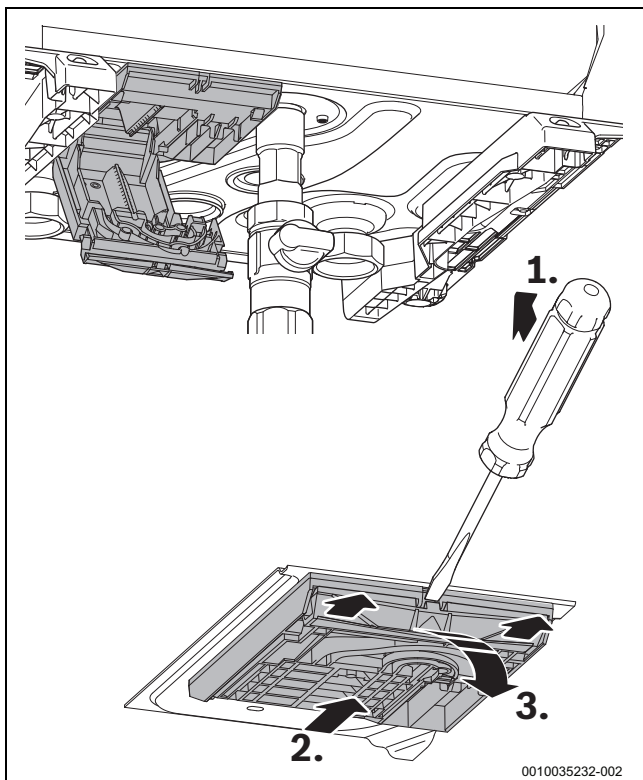
Bild 25 Pumpenanschluss-Einheit öffnen
