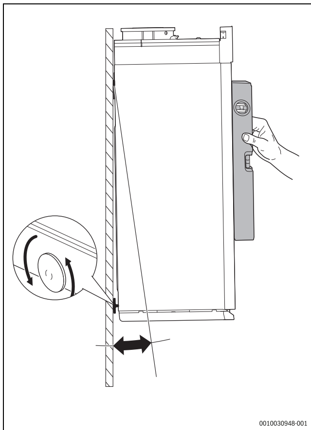
Bild 12 Ausrichten des Heizkessels an der Wand
