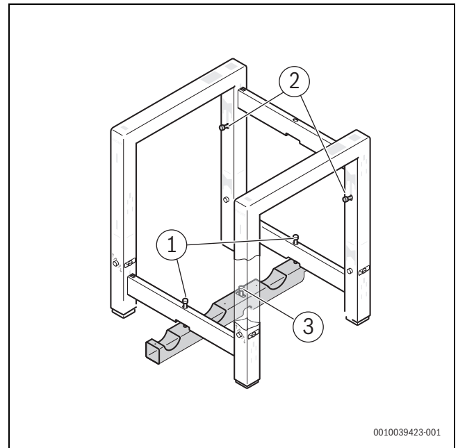
Bild 9 Sichern des Rahmens an der Wand oder am Boden
