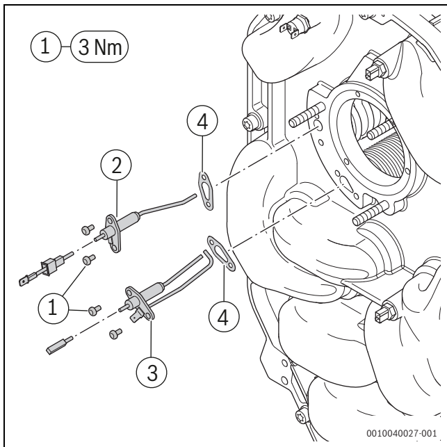
Bild 44 Ersetzen des Ionisations- und Zündstifts
