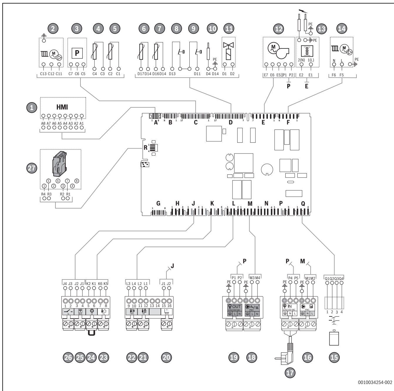
Bild 47 Schaltplan
