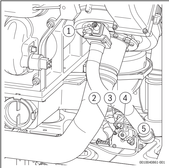
Bild 29 Übersicht Messstutzen und Justierschrauben
