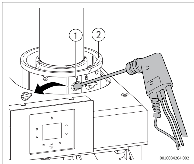
Bild 30 Entfernen des Dübels an am Abgasaustritt
