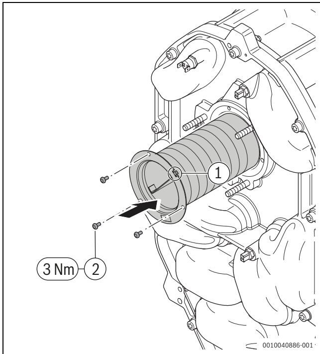
Bild 40 Montieren des Brenners
