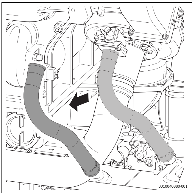
Bild 33 Gasschlauch entfernen
