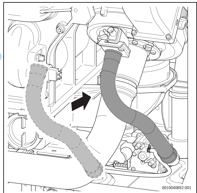
Bild 43 Montieren des Gasschlauchs
