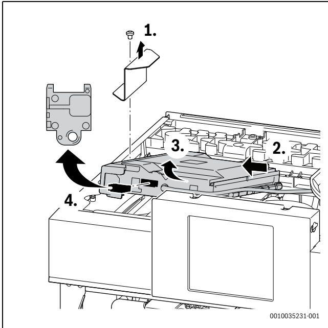
Bild 46 Ersetzen des Kodiersteckers
