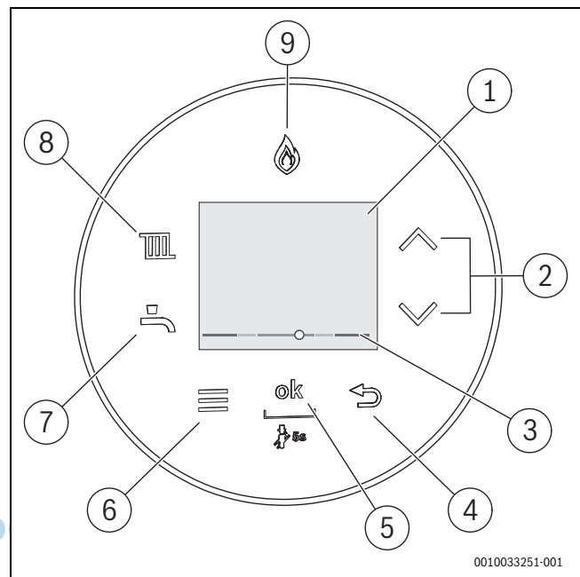
Bild 32 Bedienfeld
