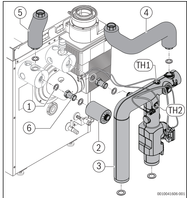
Bild 7 Montage Rohrgruppe HF-Set HYC25
