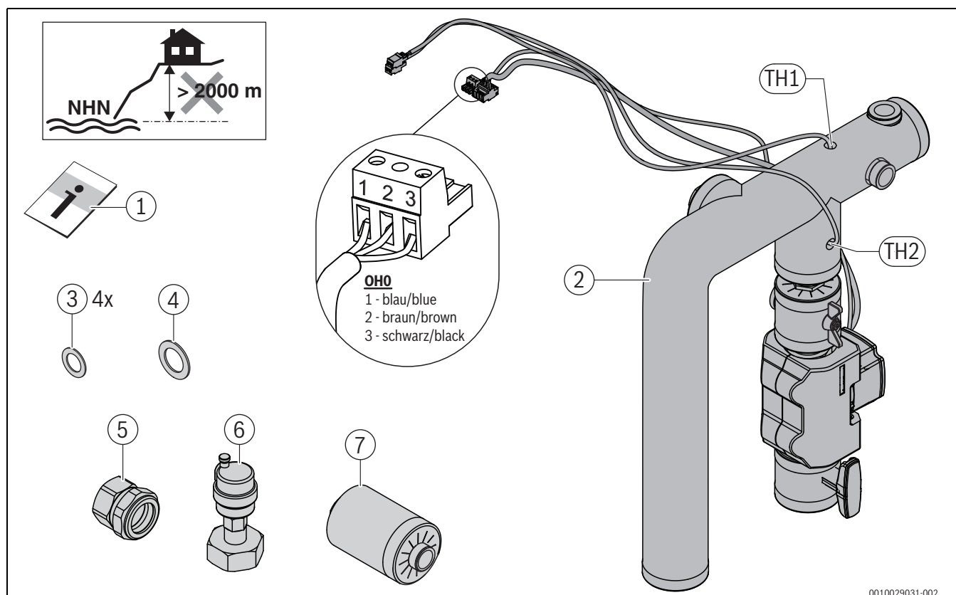
Bild 1 Lieferumfang HF-Set HYC25
