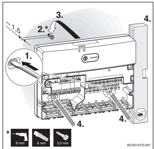
Bild 19 Wandbefestigung anzeichnen
