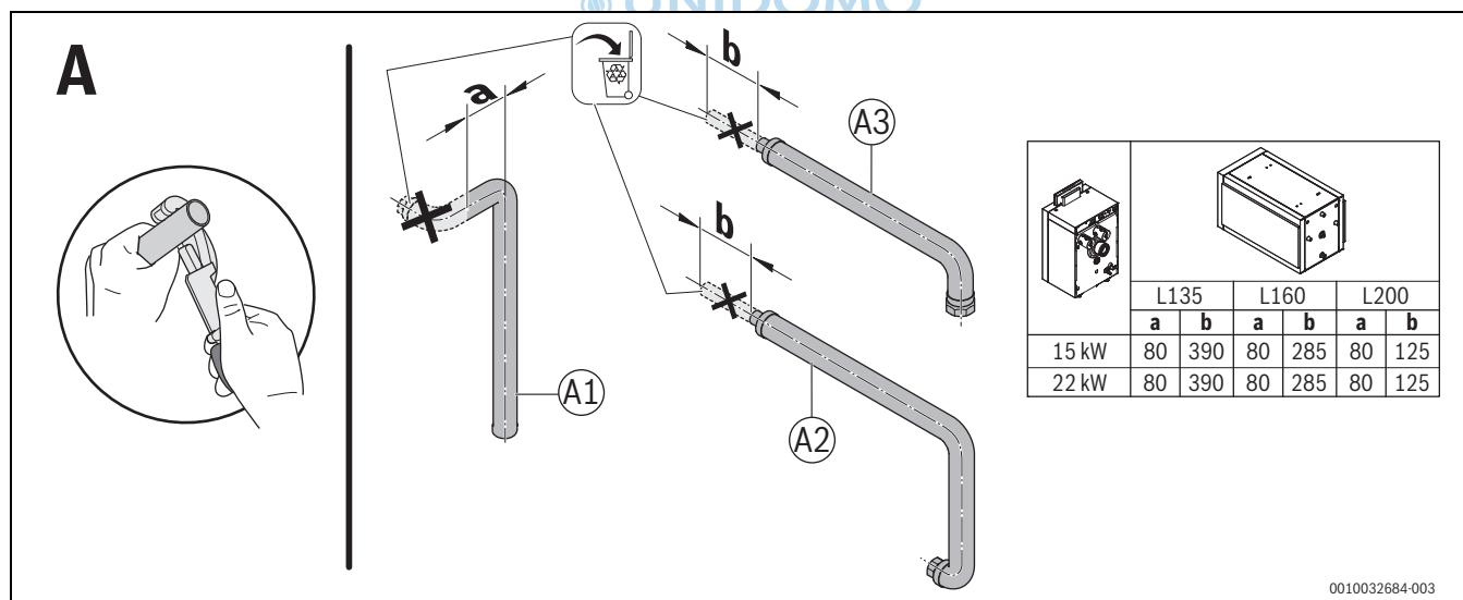
Bild 8 Kürzen der Rohre, Variante A
