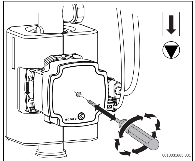
Bild 25 Pumpenblockierung lösen
