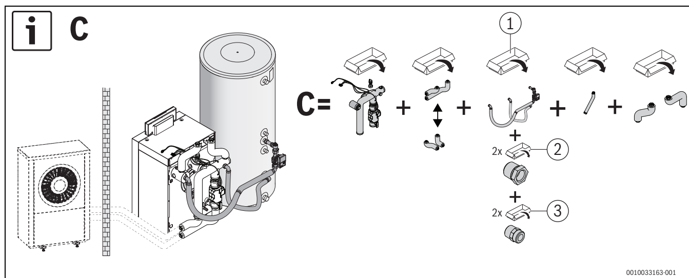
Bild 11 Speicherverbindung stehender Speicher links, Variante C
