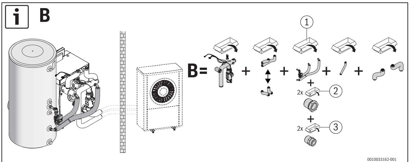
Bild 10 Speicherverbindung stehender Speicher rechts, Variante B
