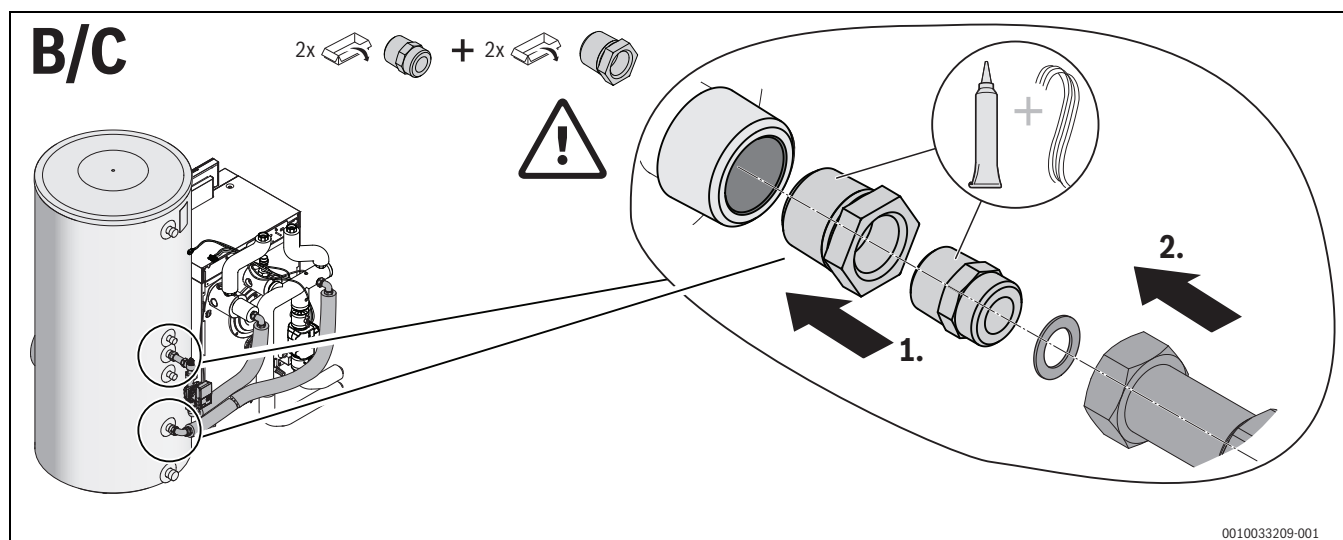
Bild 12 Montage Speicherverbindung stehender Speicher, Varianten B und C
