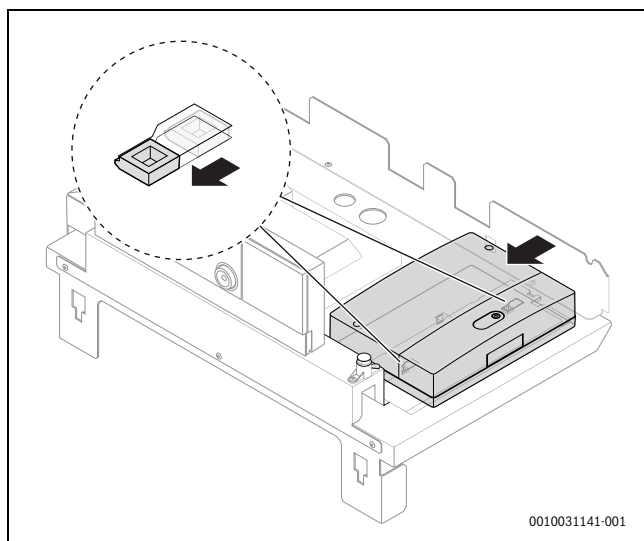
Bild 16 Montage des Elektronik-Moduls unter der Kesselhaube (Beispiel)
