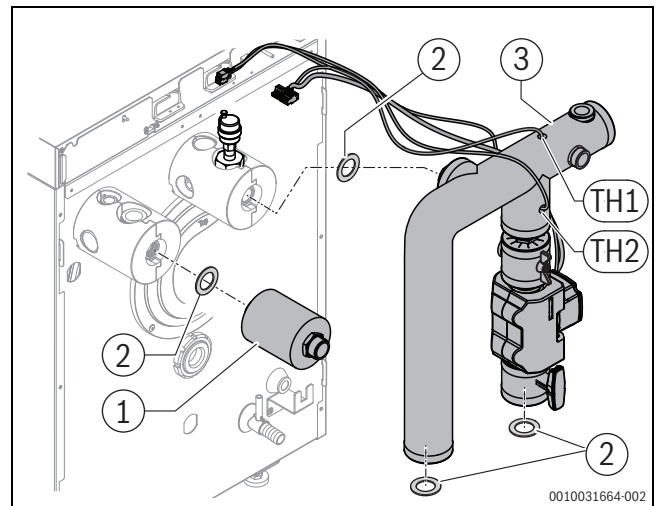
Bild 5 Montage Rohrgruppe HF-Set HYC25
