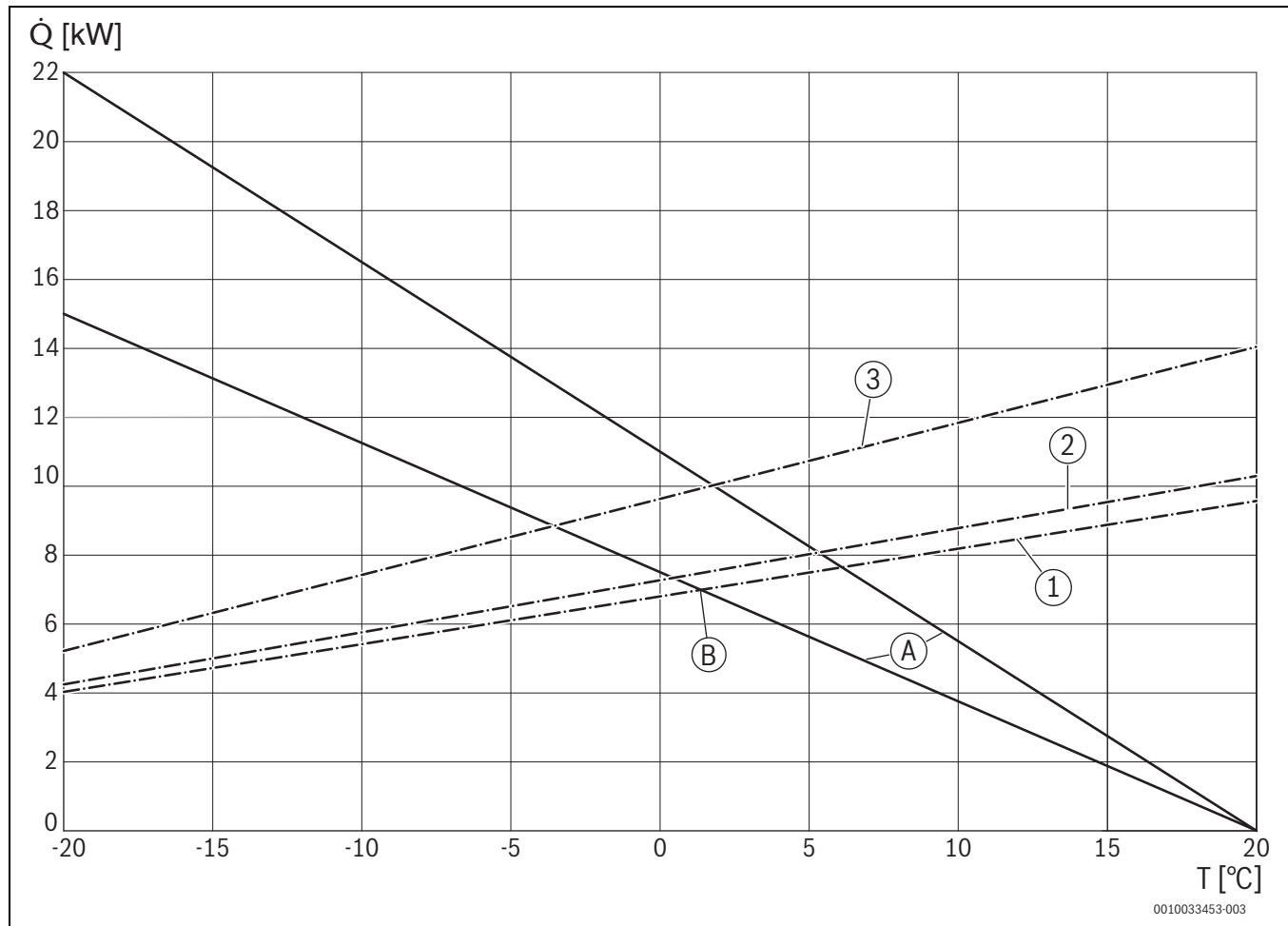
Bild 23 Diagramm zu Tab. 3; Bivalentenpunkte, Heizleistungskurven der Wärmepumpen bei 35 °C Vorlauftemperatur
