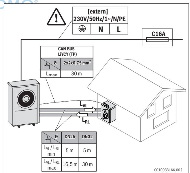
Bild 6 Maximale Längen der Leitungen
