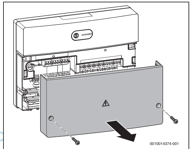
Bild 18 Deckel des Elektronik-Moduls abnehmen
