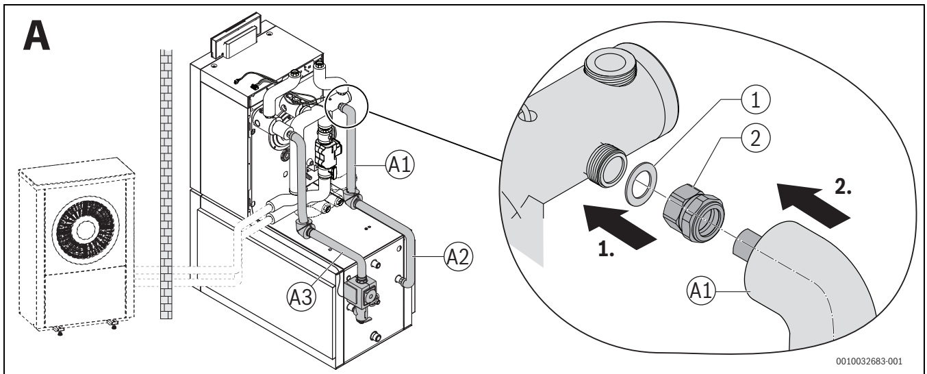
Bild 9 Montage Speicherverbindung liegender Speicher, Variante A
