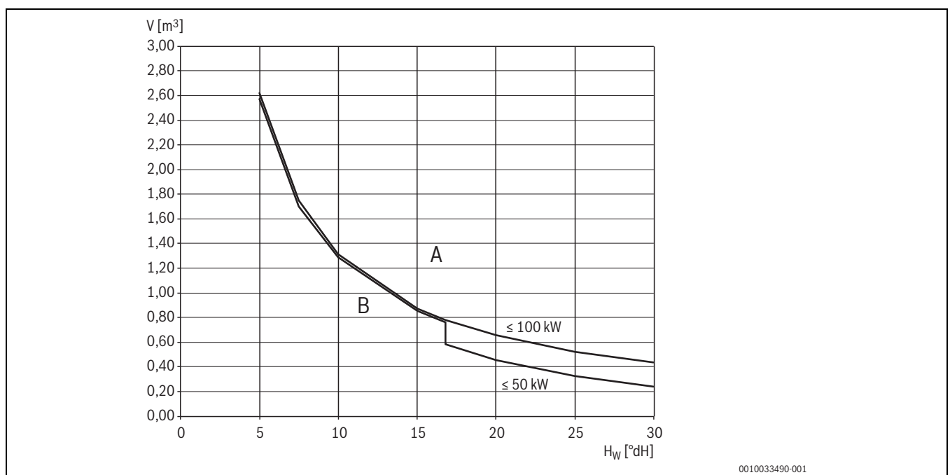
Bild 22 Grenzen zur Wasserbehandlung bei Wärmepumpen ≤ 50 kW und ≤ 100 kW
