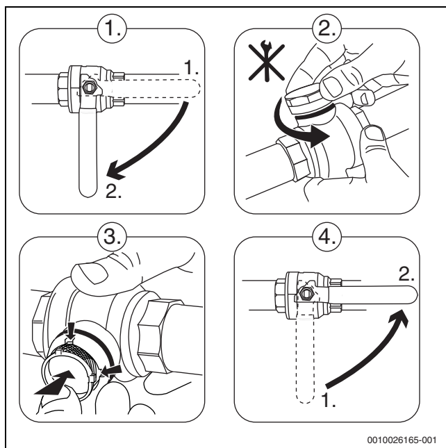
Bild 24 Aus- und Einbau des Partikelfilters (Beispiel)
