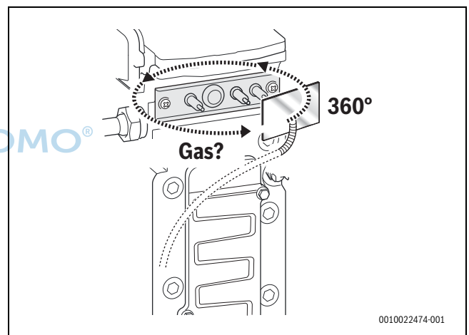
Bild 67 Dichtheitsprüfung
