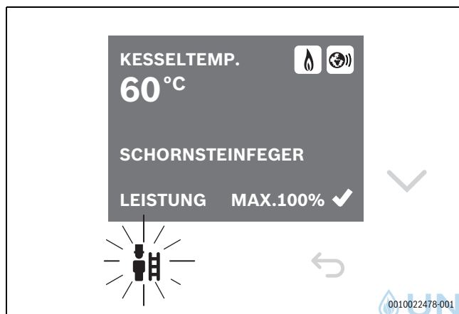
Bild 61 Menü Schornsteinfegerbetrieb
