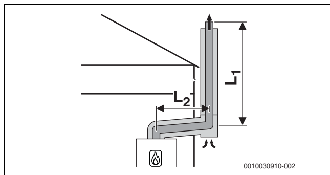
Bild 35 Konzentrische Luft-Abgas-Führung nach C 53x an der Außenwand
