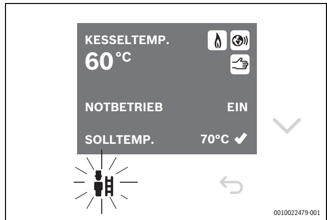
Bild 62 Menü Notbetrieb
