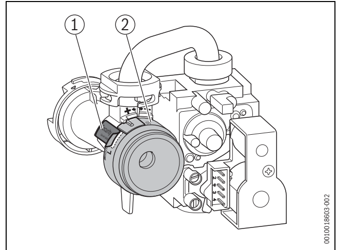
Bild 55 Aufkleber lösen
