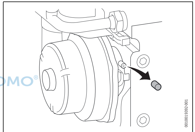
Bild 73 Messstutzen an der Mischereinrichtung
