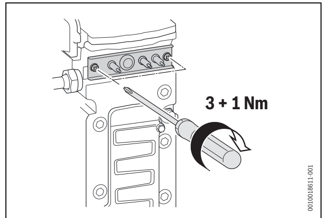
Bild 66 Elektroden-Set montieren
