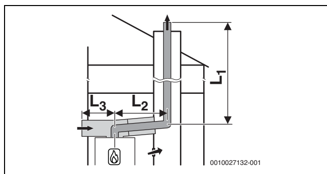
Bild 33 Starre Abgasführung nach C 53x im Schacht und Luft-Abgas-Führung mit separater Luftzufuhr und konzentrischer Abgasableitung im Aufstellraum
