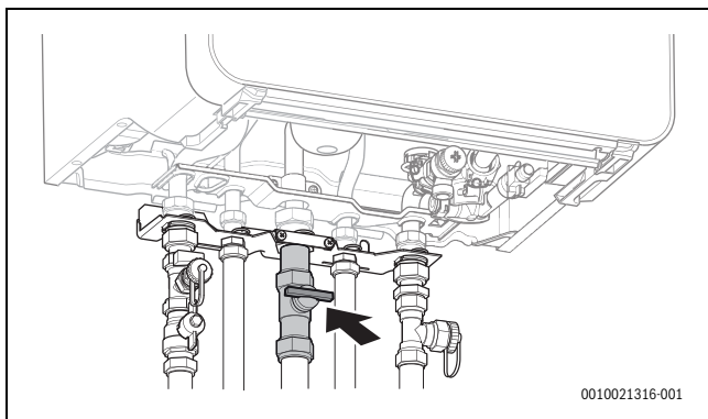
Bild 64 Gashahn geschlossen
