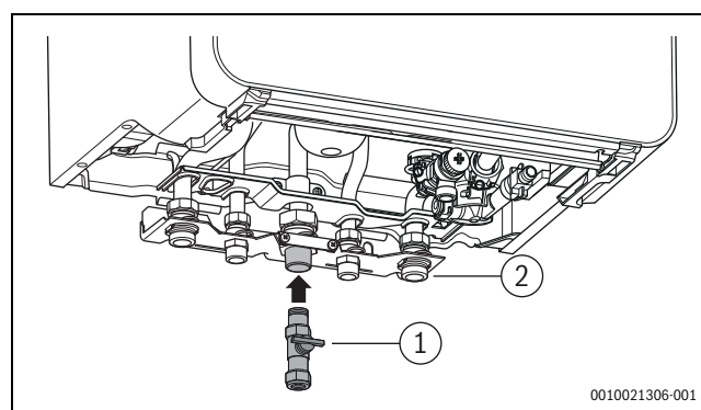
Bild 16 Gasanschluss herstellen
