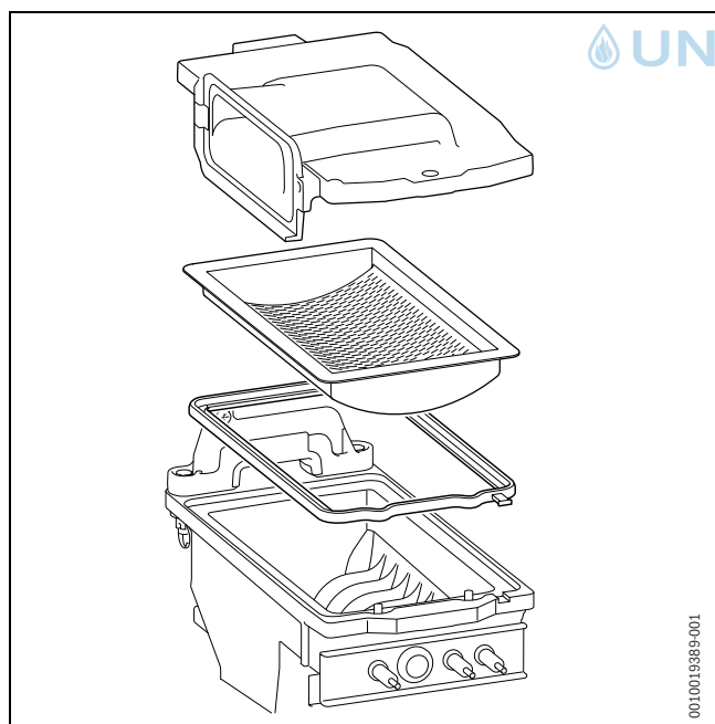
Bild 69 Brenner herausnehmen
