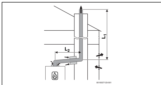
Bild 38 Starre Abgasführung im Schacht nach B 23p /B 53p mit raumluftabhängiger Luftzufuhr am Gerät und konzentrischem Verbindungsstück zwischen Aufstellraum und Schacht
