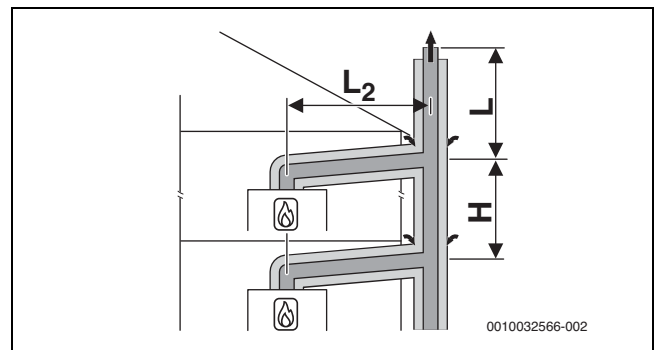
Bild 44 Mehrfachbelegung nach C_{(13)3x} mit konzentrischer Luft-Abgas-Führung an der Außenwand und im Aufstellraum
