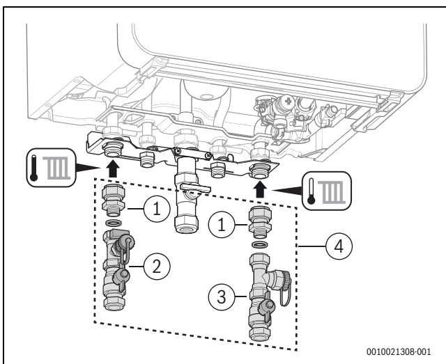
Bild 18 Anschluss der Heizwasserrohre am Gerät
