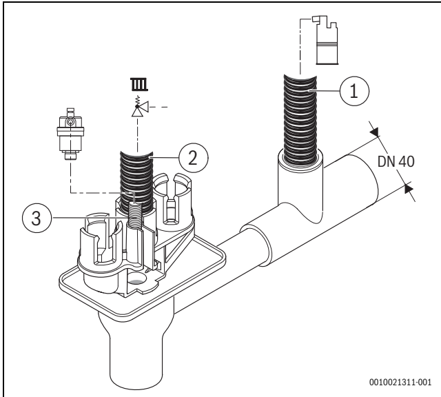
Bild 22 Kondensatschlauch und Schlauch vom Sicherheitsventil und Entlüfter montieren
