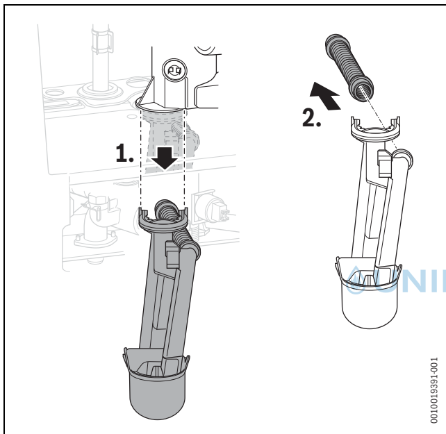
Bild 72 Kondensatsiphon
