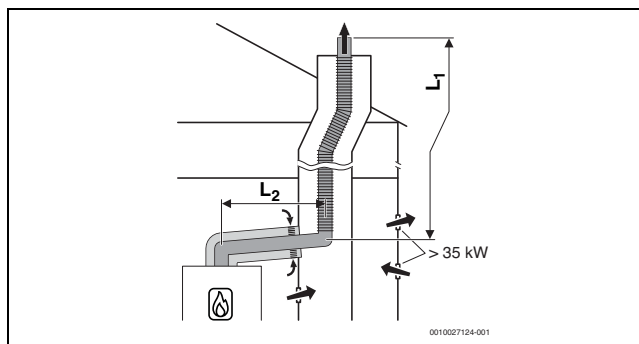
Bild 41 Flexible Abgasführung im Schacht nach B 33 mit raumluftabhängiger Luftzufuhr über die konzentrische Luft-Abgas-Führung im Aufstellraum
