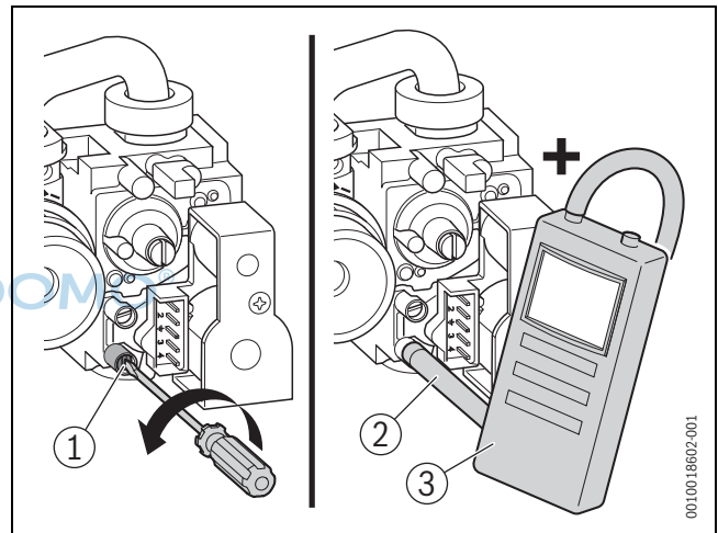
Bild 54 Gas-Anschlussdruck messen
