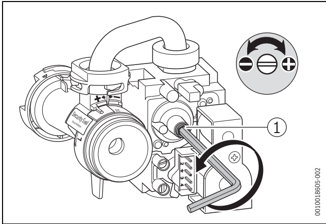
Bild 57 Plombe entfernen
