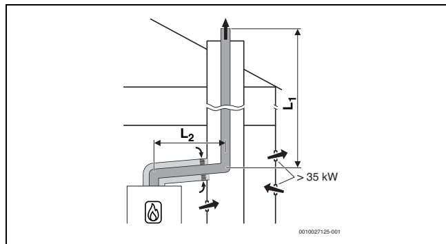
Bild 40 Starre Abgasführung im Schacht nach B 33 mit raumluftabhängiger Luftzufuhr über die konzentrische Luft-Abgas-Führung im Aufstellraum
