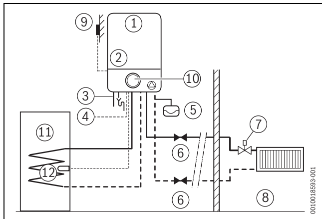
Bild 20 Anwendungsbeispiel mit außentemperaturgeführter Regelung und Warmwasserspeicher
