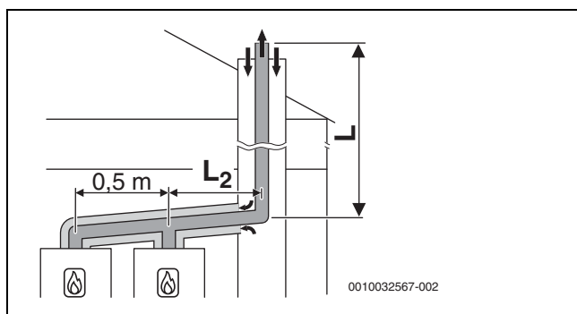
Bild 48 Starre Abgasführung nach C 93x im Schacht und konzentrische Luft-Abgas-Führung im Aufstellraum
