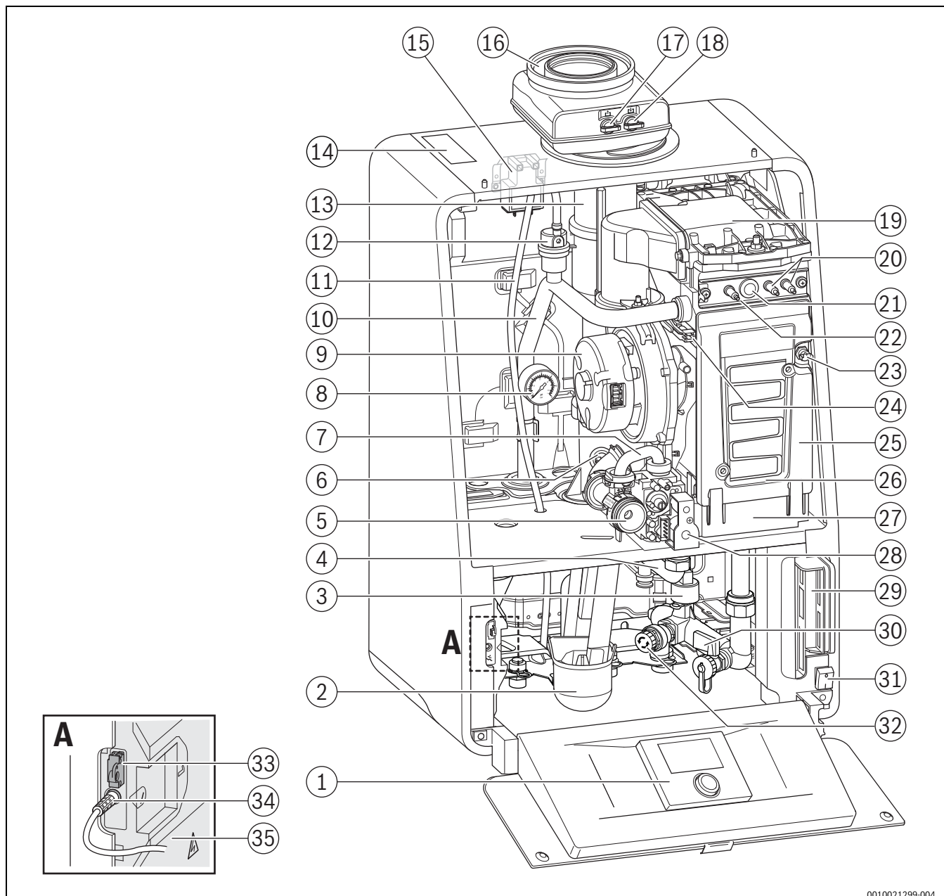
Bild 3 GC9000iW 20H, 30H, 40H, 50H
