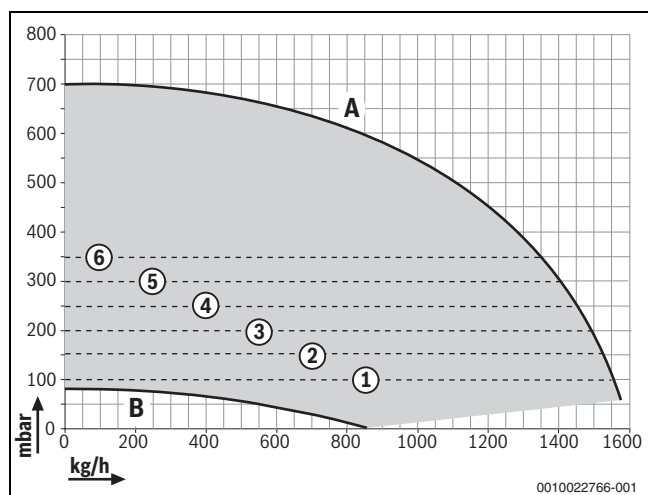
Bild 8 20 bis 40 kW: Restförderhöhe bei Einstellung 1-6
