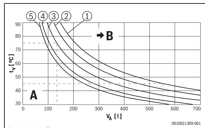
Bild 19 Kennlinien des Ausdehnungsgefäßes, Heizungsausdehnungsgefäß 14 l
