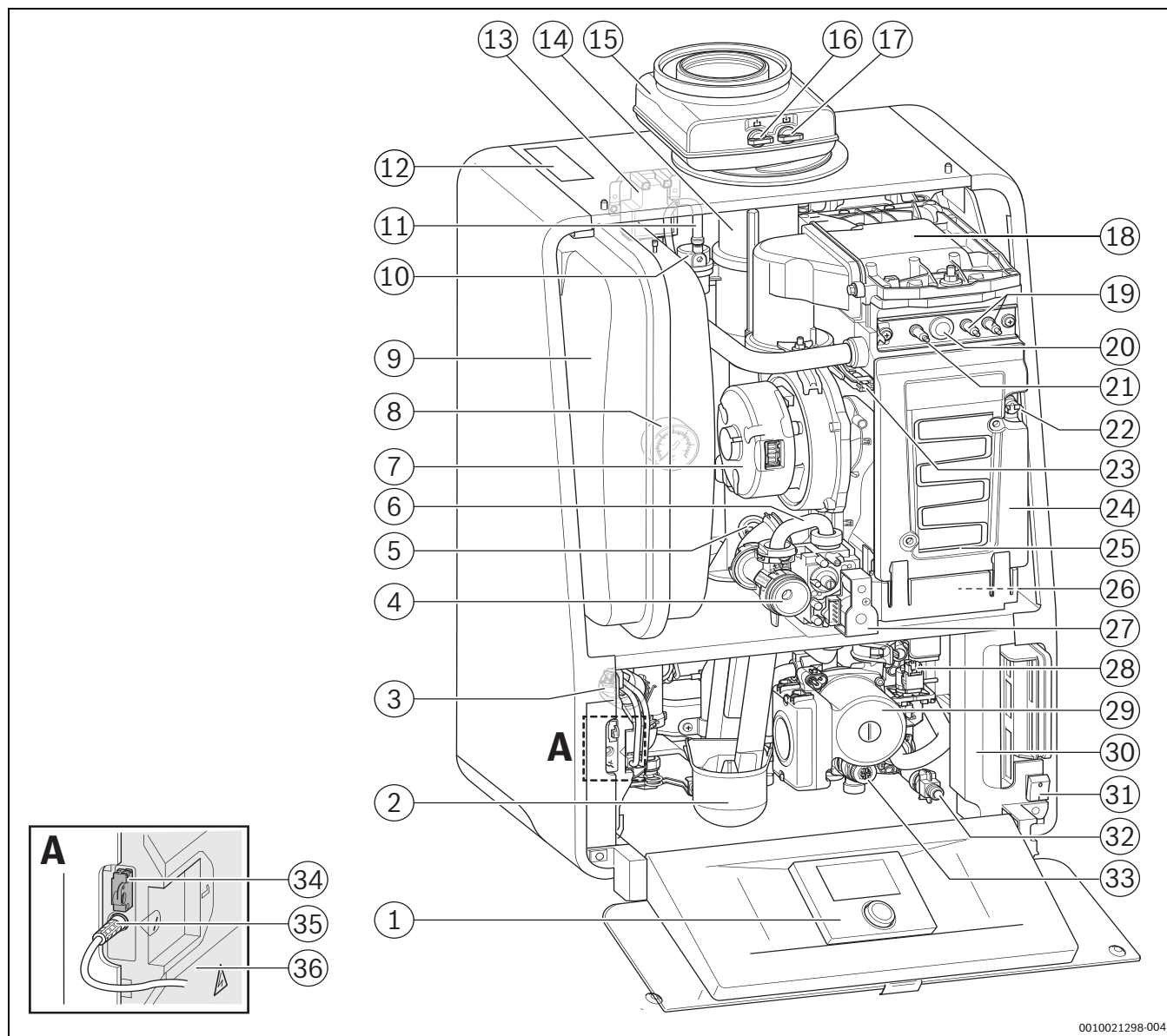
Bild 2 GC9000iW 20/30 E(B)
