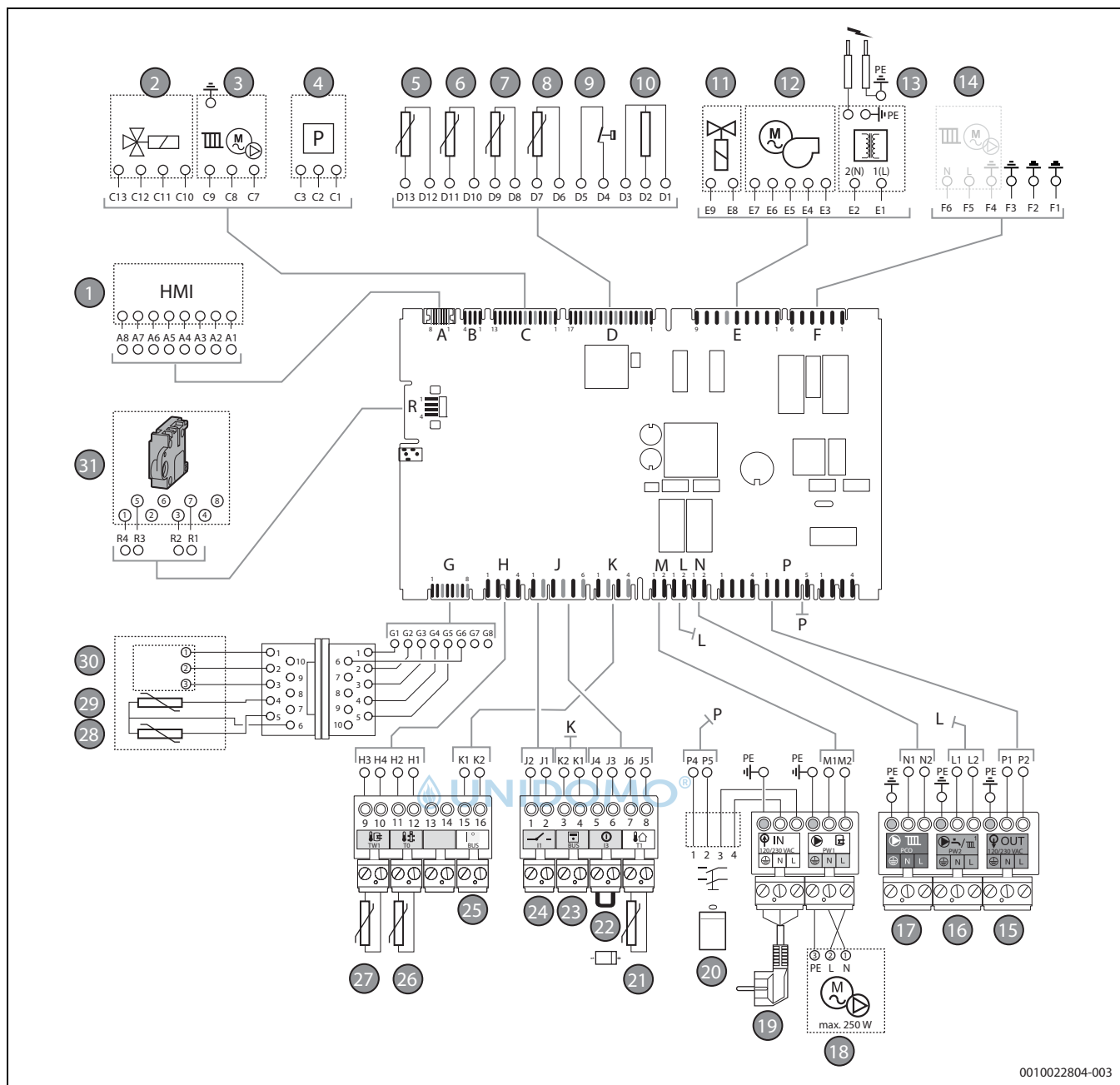
Bild 6 Leiterplatte
