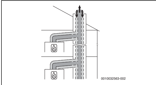
Bild 42 Mehrfachbelegung nach C_{(10)3x} mit konzentrischer Luft-Abgas-Führung im Aufstellraum
