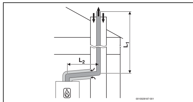
Bild 36 Starre Abgasführung nach C 93x im Schacht und konzentrische Luft-Abgas-Führung im Aufstellraum
