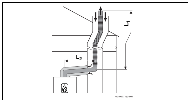
Bild 37 Flexible Abgasführung nach C 93x im Schacht und konzentrische Luft-Abgas-Führung im Aufstellraum
