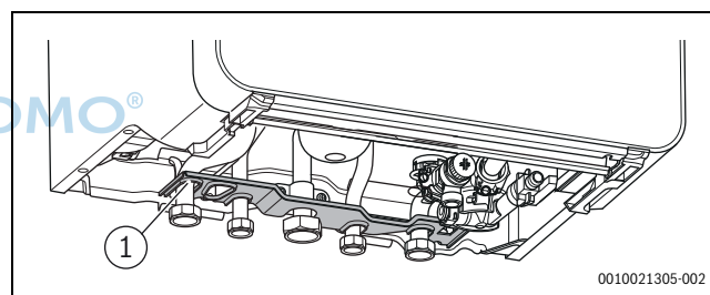
Bild 15 Entfernen Transporthalterung
