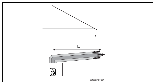
Bild 30 Horizontale konzentrische Luft-Abgas-Führung nach C 13x durch die Außenwand
