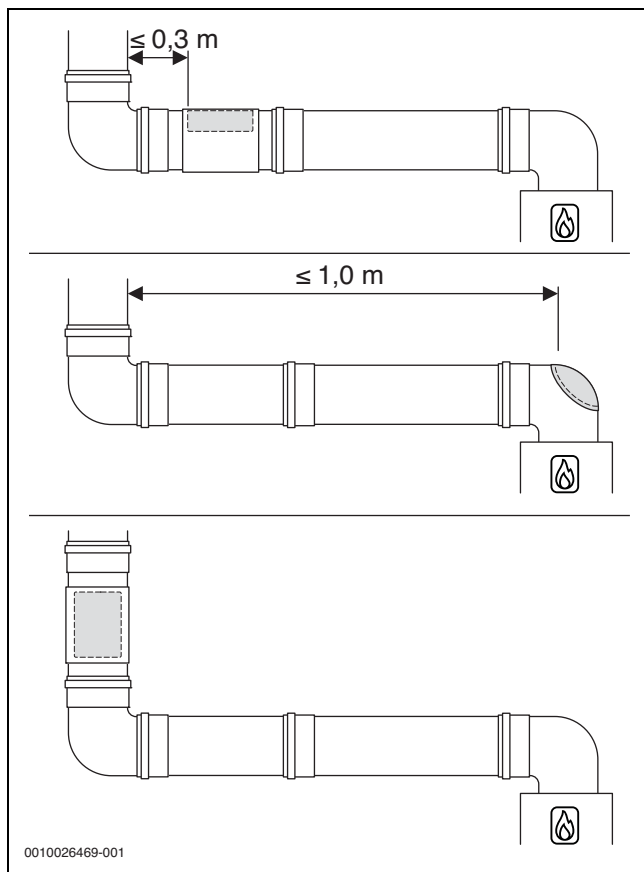
Bild 24 Anordnung der unteren Prüfföffnung
