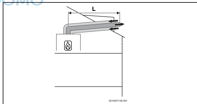
Bild 29 Horizontale konzentrische Luft-Abgas-Führung nach C 13x über das Dach
