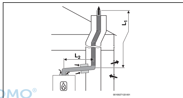
Bild 39 Flexible Abgasführung im Schacht nach B 23p /B 53p mit raumluftabhängiger Luftzufuhr am Gerät und konzentrischem Verbindungsstück zwischen Aufstellraum und Schacht
