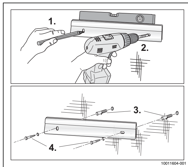
Bild 14 Aufhängeschiene montieren
