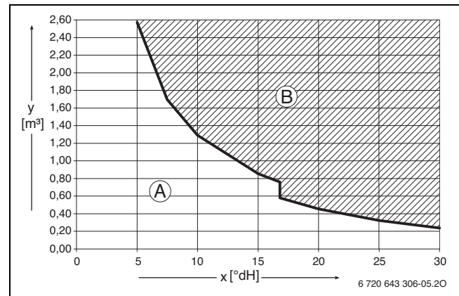
Bild 13 Anforderungen an Füll- und Ergänzungswasser Geräte < 50 kW
