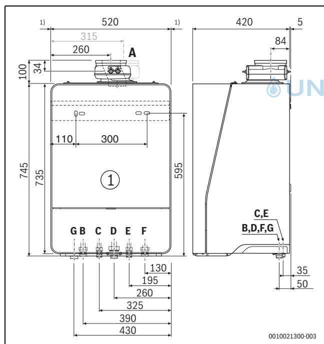
Bild 4 Typ E - Abmessungen und Anschlüsse [mm]
