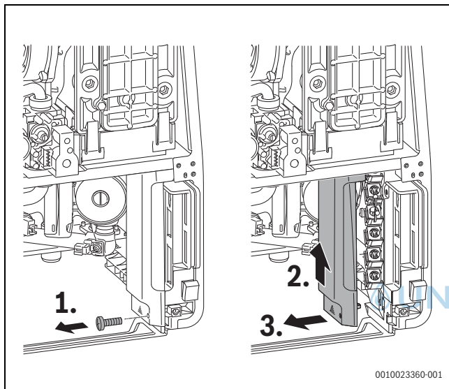
Bild 50 Abdeckung der Anschlussklemmen
