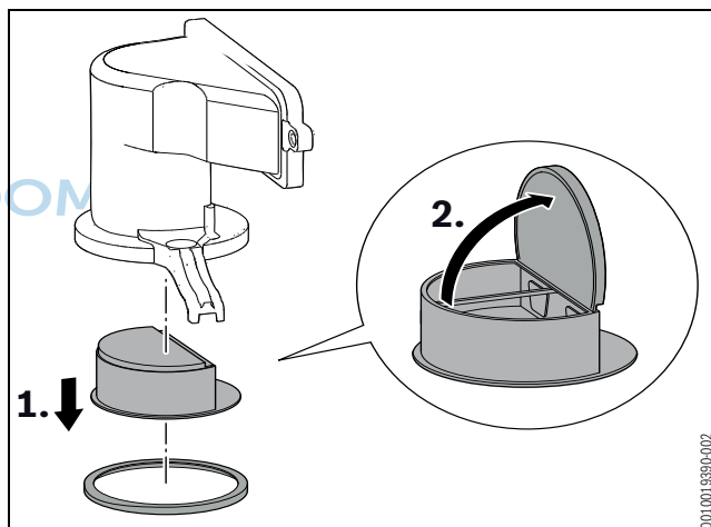
Bild 71 Rückschlagklappe in der Mischeinrichtung
