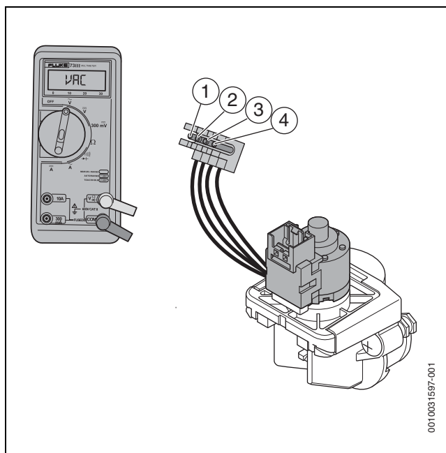
Bild 77 3-Wege-Ventil
