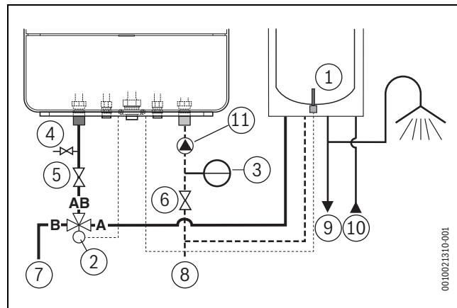
Bild 21 Externes 3-Wege-Ventil montieren (230 V)
