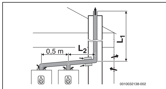
Bild 47 Kaskade mit 2 Geräten:
