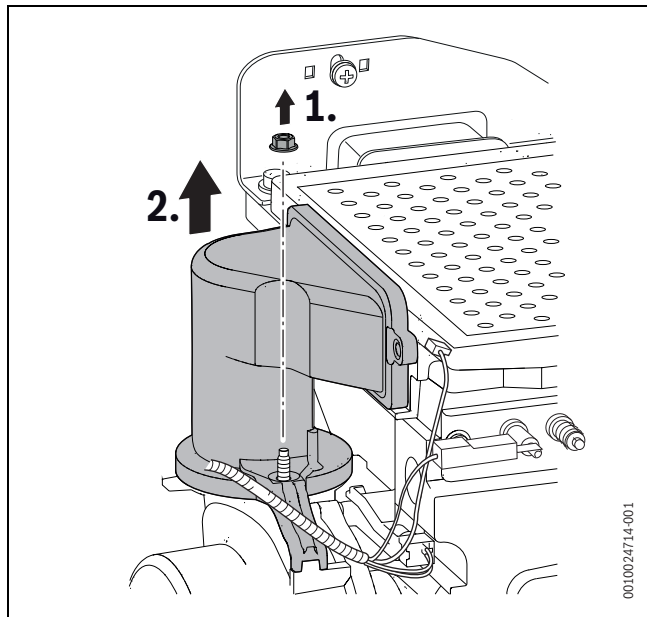
Bild 71 Mischeinrichtung ausbauen
