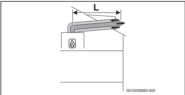
Bild 27 Horizontale konzentrische Luft-Abgas-Führung nach C 13x über das Dach
