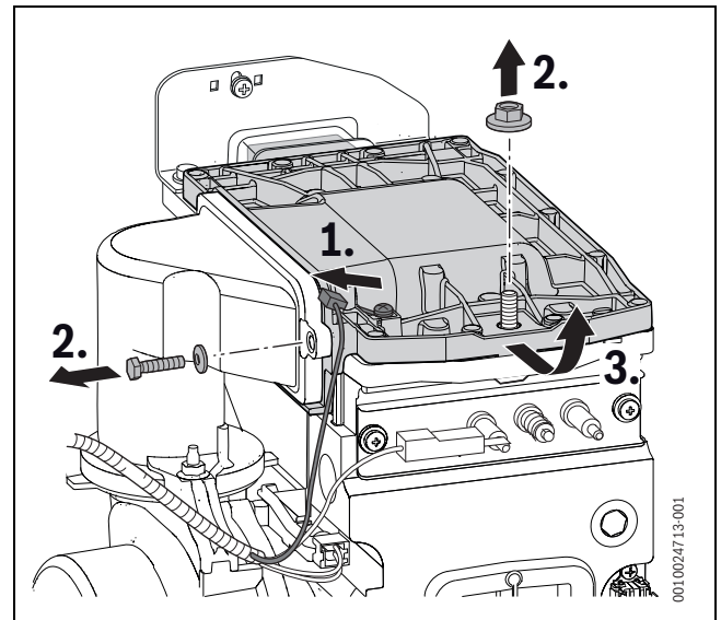
Bild 69 Brennerdeckel ausbauen
