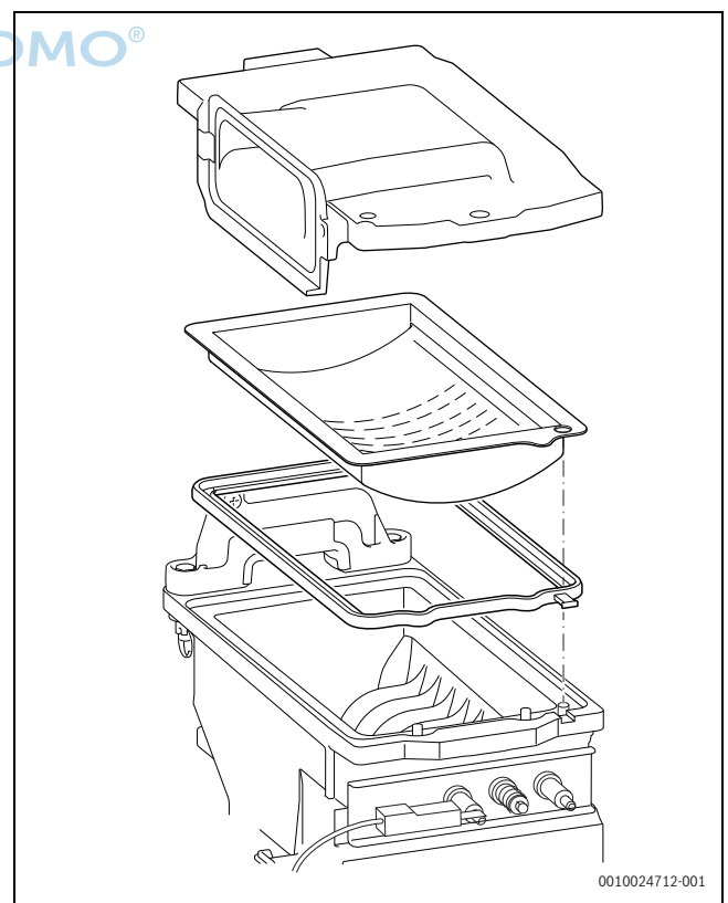
Bild 70 Brenner herausnehmen
