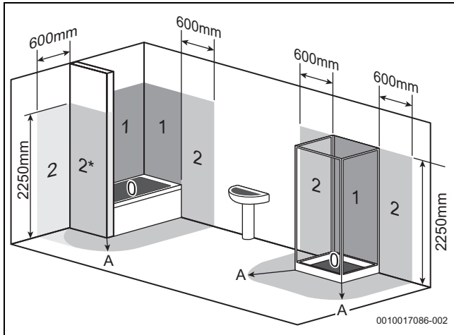
Bild 49 Schutzbereiche (Beispieldarstellung)
