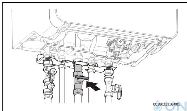
Bild 65 Gashahn geschlossen
