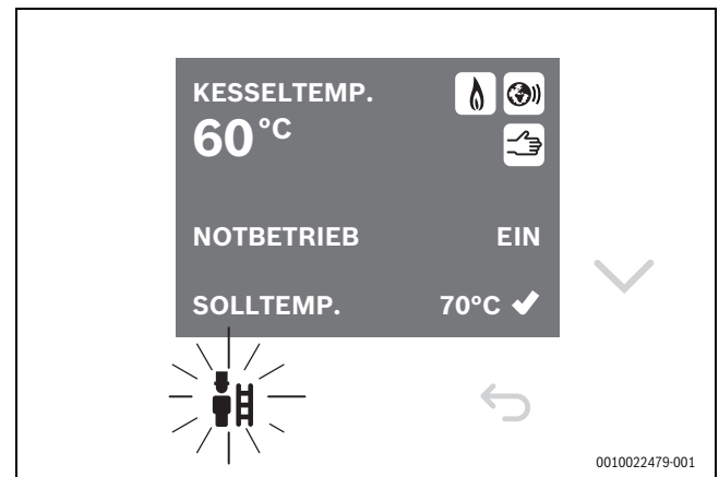
Bild 63 Menü Notbetrieb
