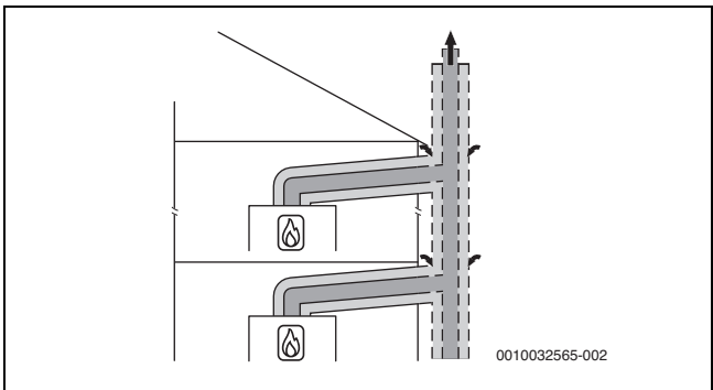
Bild 43 Mehrfachbelegung nach C (12)3x mit konzentrischer Luft-Abgas-Führung im Aufstellraum
