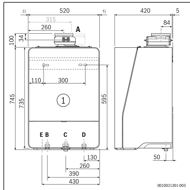
Bild 5 Typ H - Abmessungen und Anschlüsse [mm]
