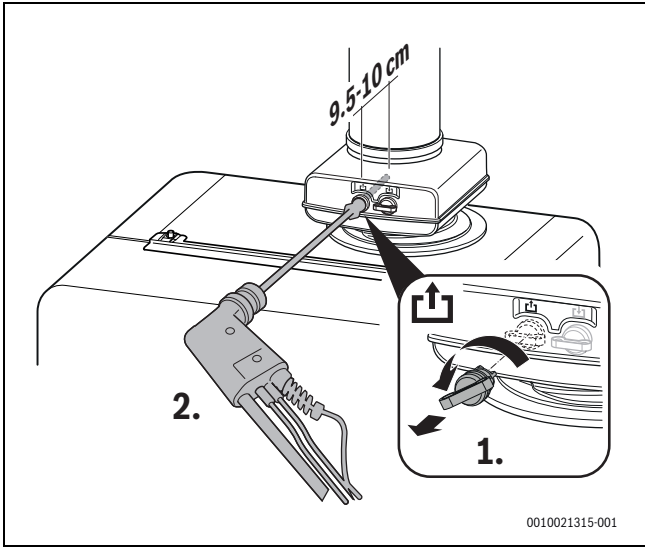
Bild 57 CO/CO 2 -Gehalt messen
