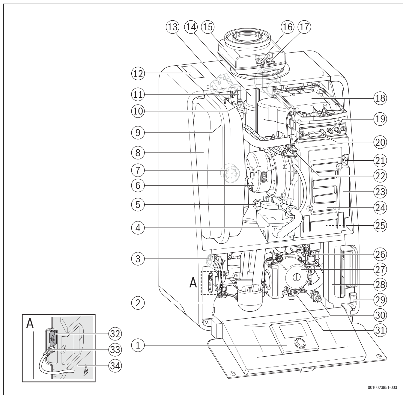
Bild 2 GC9001iW 20 E(B)
