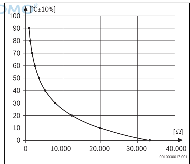
Bild 9 Widerstandskennlinie Temperaturfühler (ausgenommen die Außentemperaturfühler)
