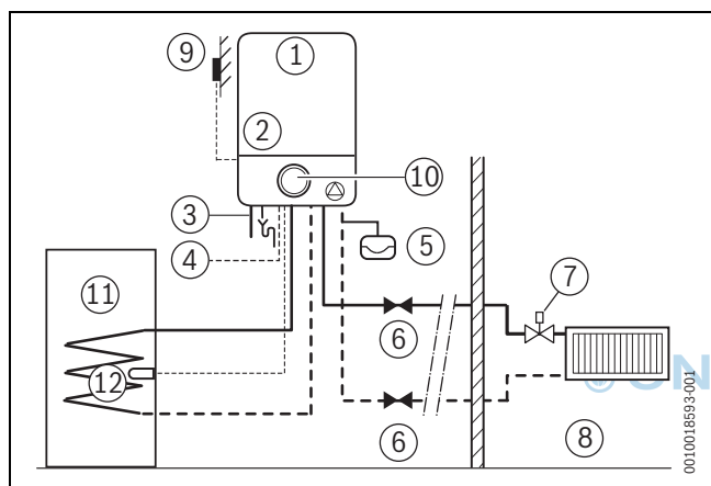
Bild 18 Anwendungsbeispiel mit außentemperaturgeführter Regelung und Warmwasserspeicher
