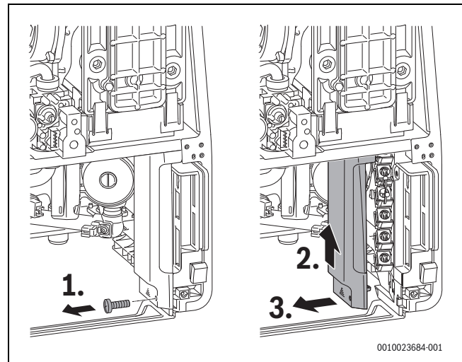
Bild 50 Abdeckung lösen
