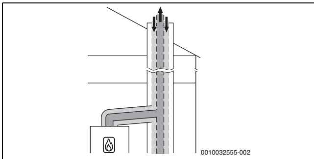
Bild 31 Konzentrische Luft-Abgas-Führung nach C 43x im Aufstellraum
