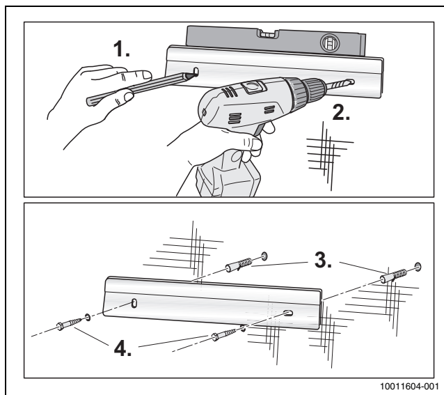
Bild 12 Aufhängeschiene montieren
