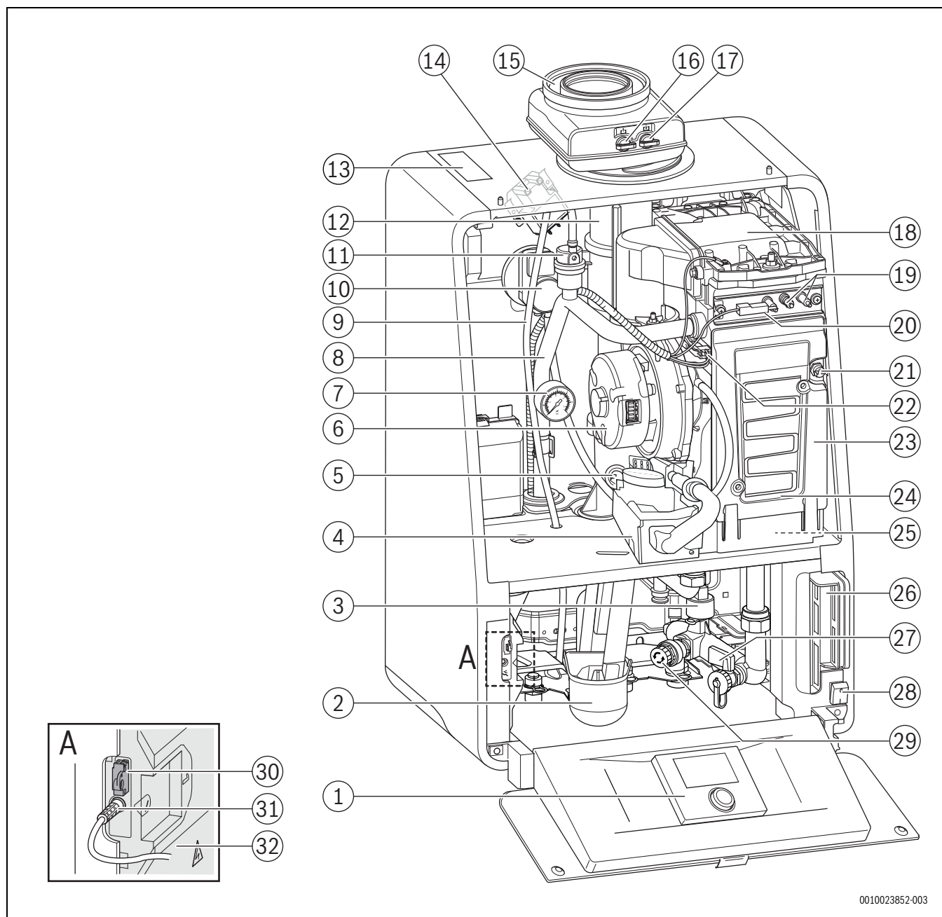
Bild 3 GC9001iW 20 H
