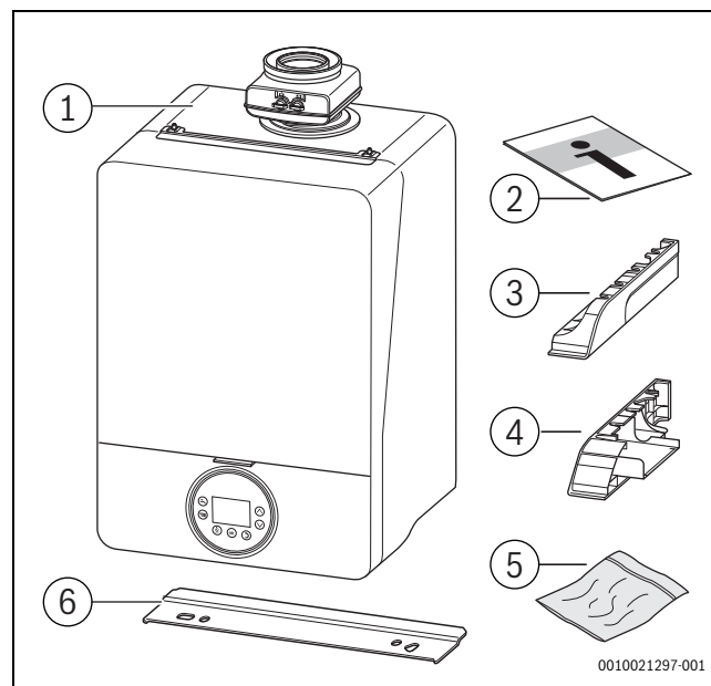
Bild 1 Lieferumfang
