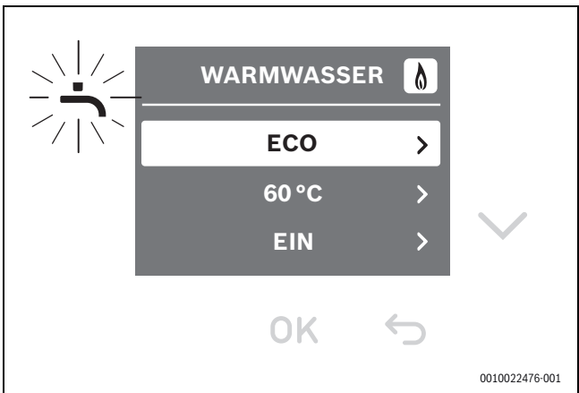
Bild 59 Menü Warmwassertemperatur
