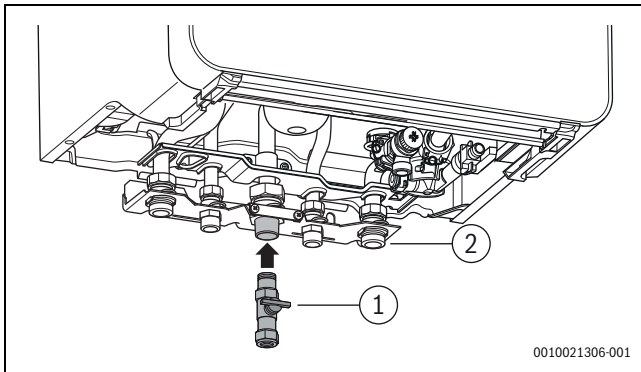
Bild 14 Gasanschluss herstellen
