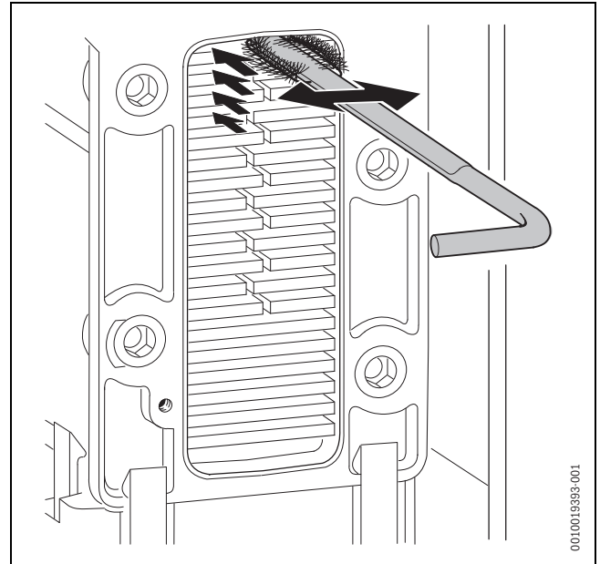
Bild 75 Wärmeblock mit Bürste reinigen
