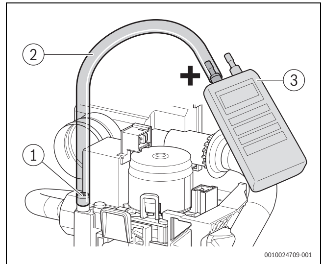
Bild 56 Gas-Anschlussdruck messen
