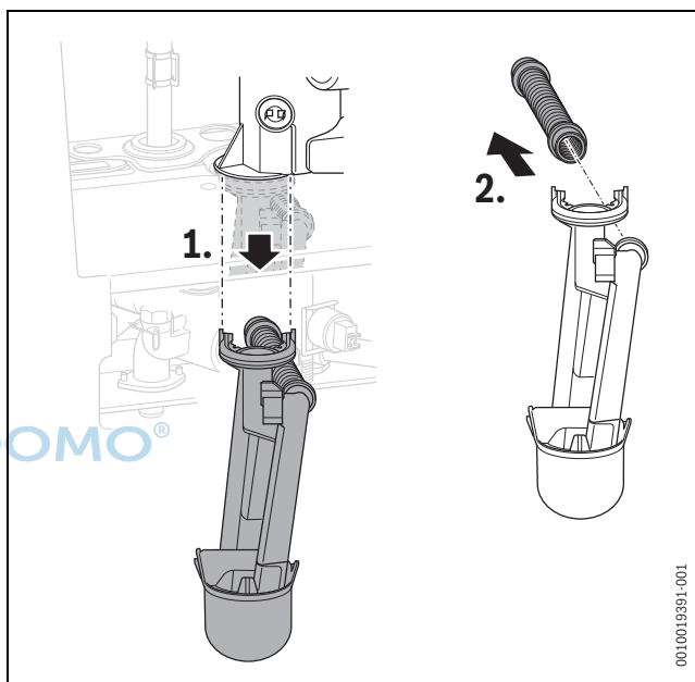
Bild 73 Kondensatsiphon
