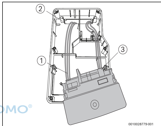
Bild 52 Funktionsmodul anschließen
