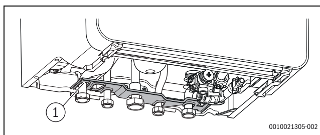
Bild 13 Entfernen Transporthalterung
