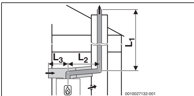
Bild 32 Starre Abgasführung nach C 53x im Schacht und Luft-Abgas-Führung mit separater Luftzufuhr und konzentrischer Abgasableitung im Aufstellraum
