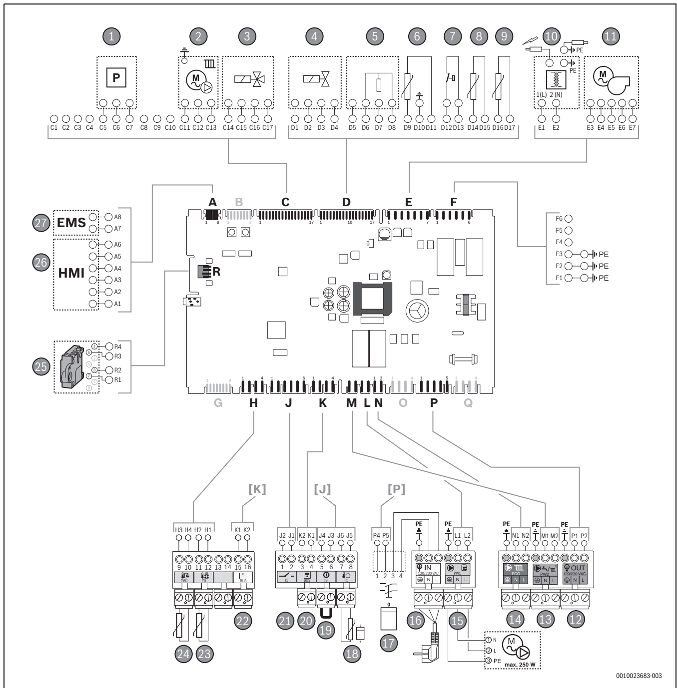
Bild 6 Anschlussplan
