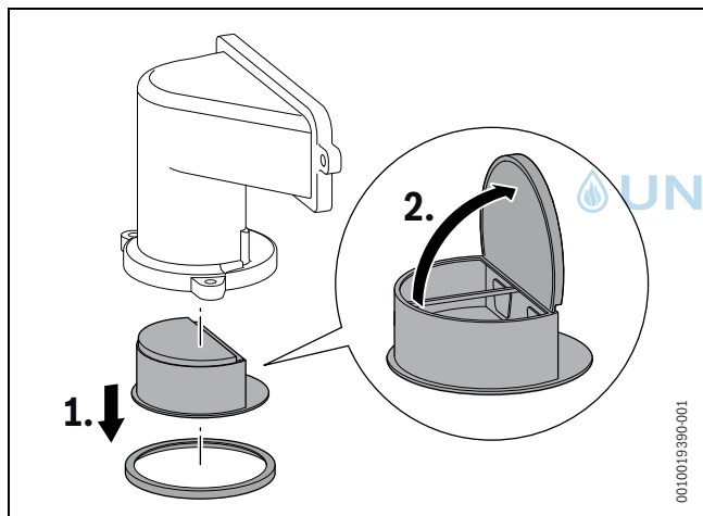
Bild 72 Rückschlagklappe in der Mischeinrichtung
