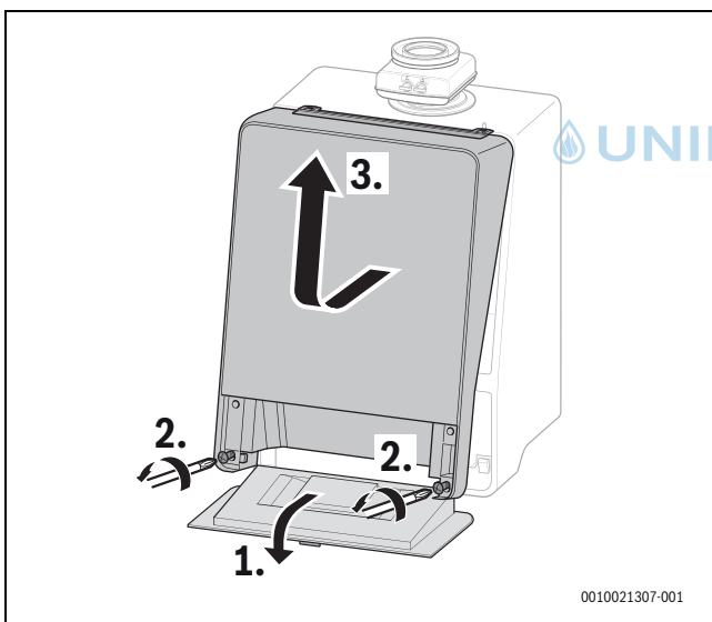
Bild 15 Verkleidung Gerät demontieren
