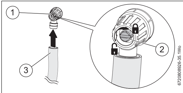
Bild 32 Entleerungsanschluss
