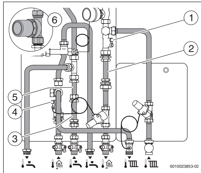
Bild 21 Adapterrohre ersetzen
