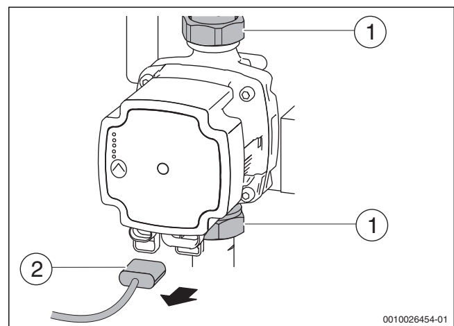
Bild 35 Heizungspumpe
