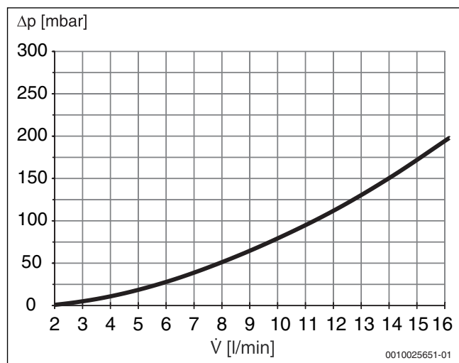
Bild 6 Druckverlust Trinkwasserseite
