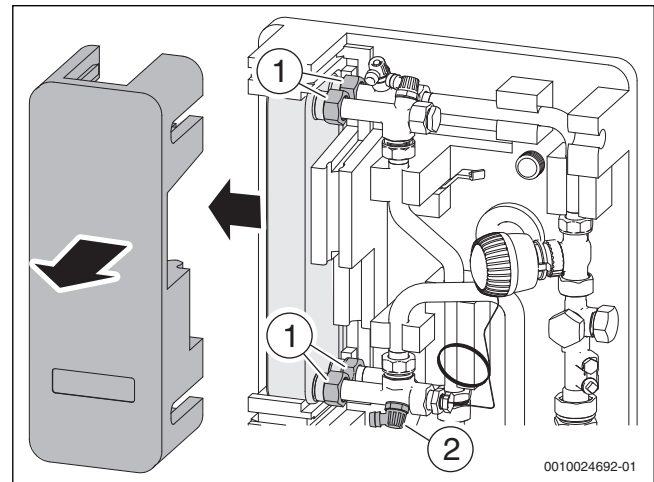
Bild 34 Wärmetauscher demontieren
