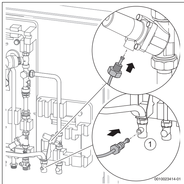
Bild 19 Kapillarleitung montieren
