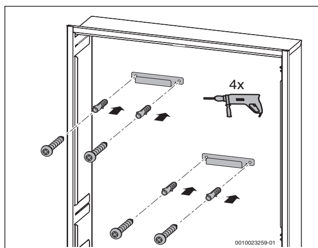
Bild 13 Beiliegende Wandhalter montieren
