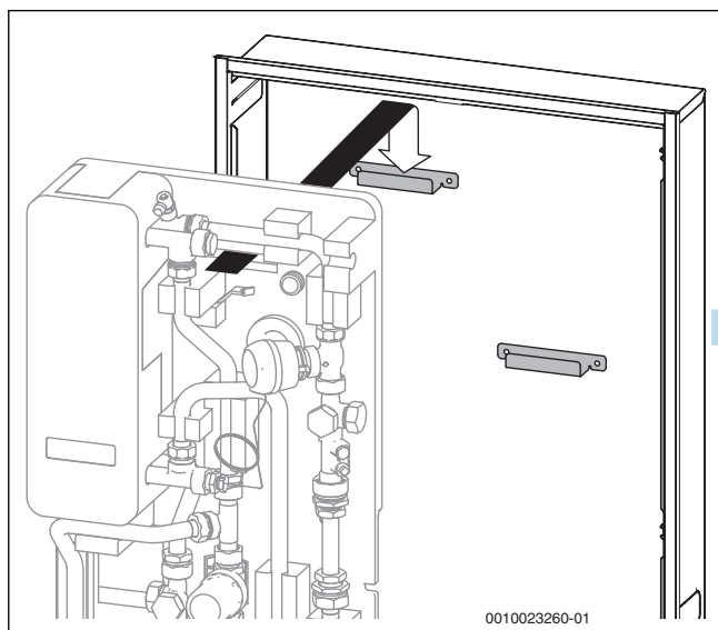
Bild 14 Grundmodul aufhängen
