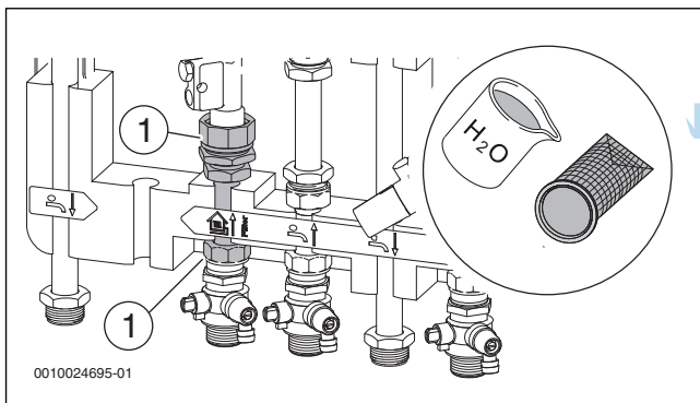
Bild 33 Filter reinigen
