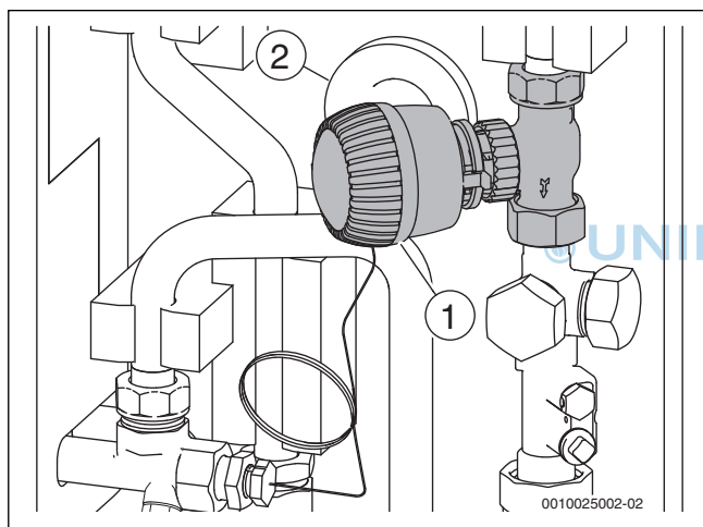
Bild 23 Warmwassertemperatur einstellen
