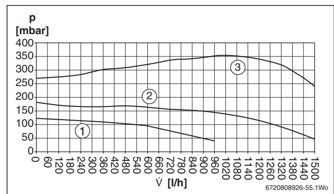
Bild 28 Restförderhöhe
