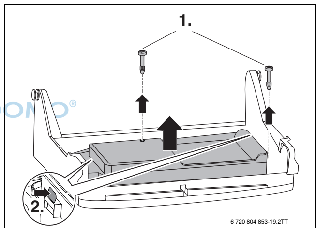
Bild 76 Abdeckung entfernen
