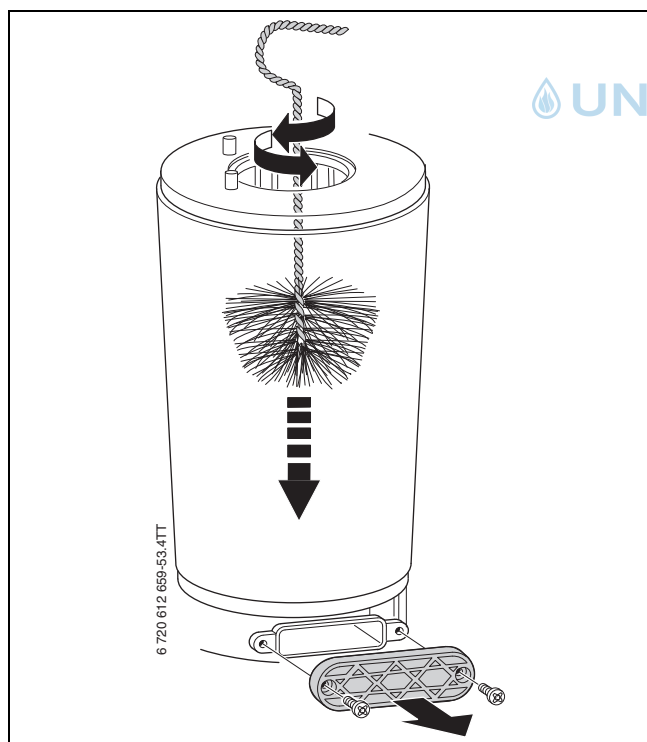
Bild 59 Wärmeblock reinigen
