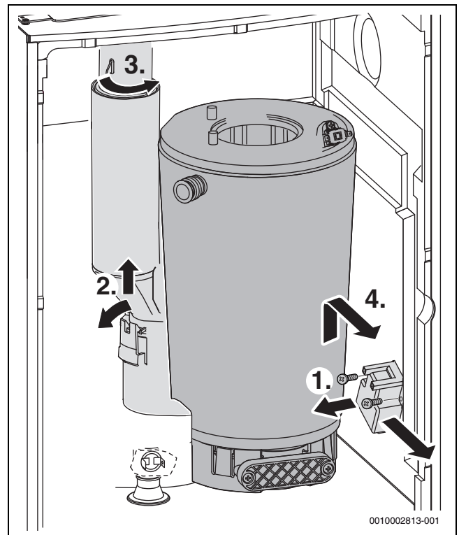
Bild 80 Wärmeblock ausbauen
