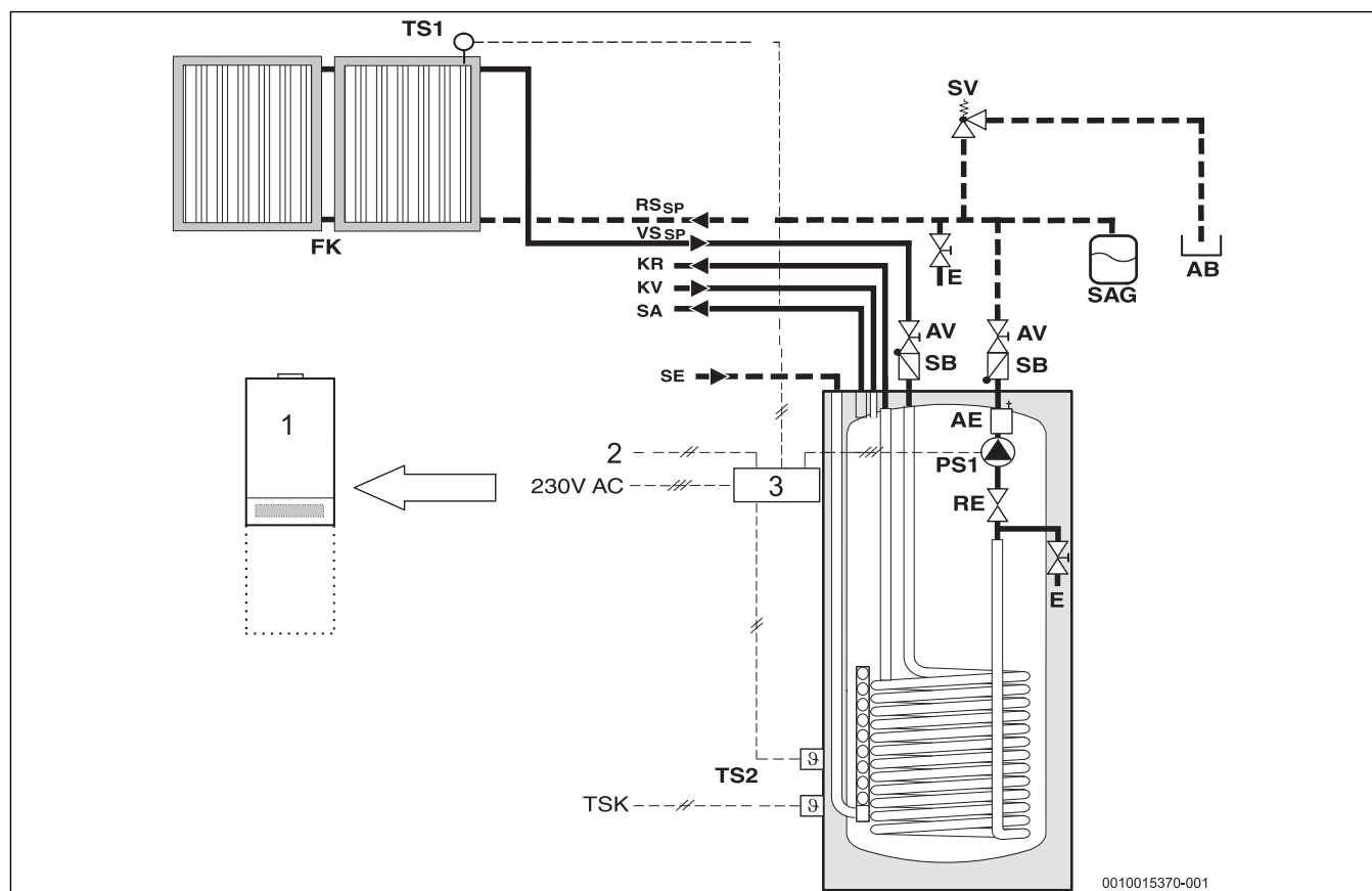
Bild 3 Trinkwasserseitiges Anschluss-Schema
