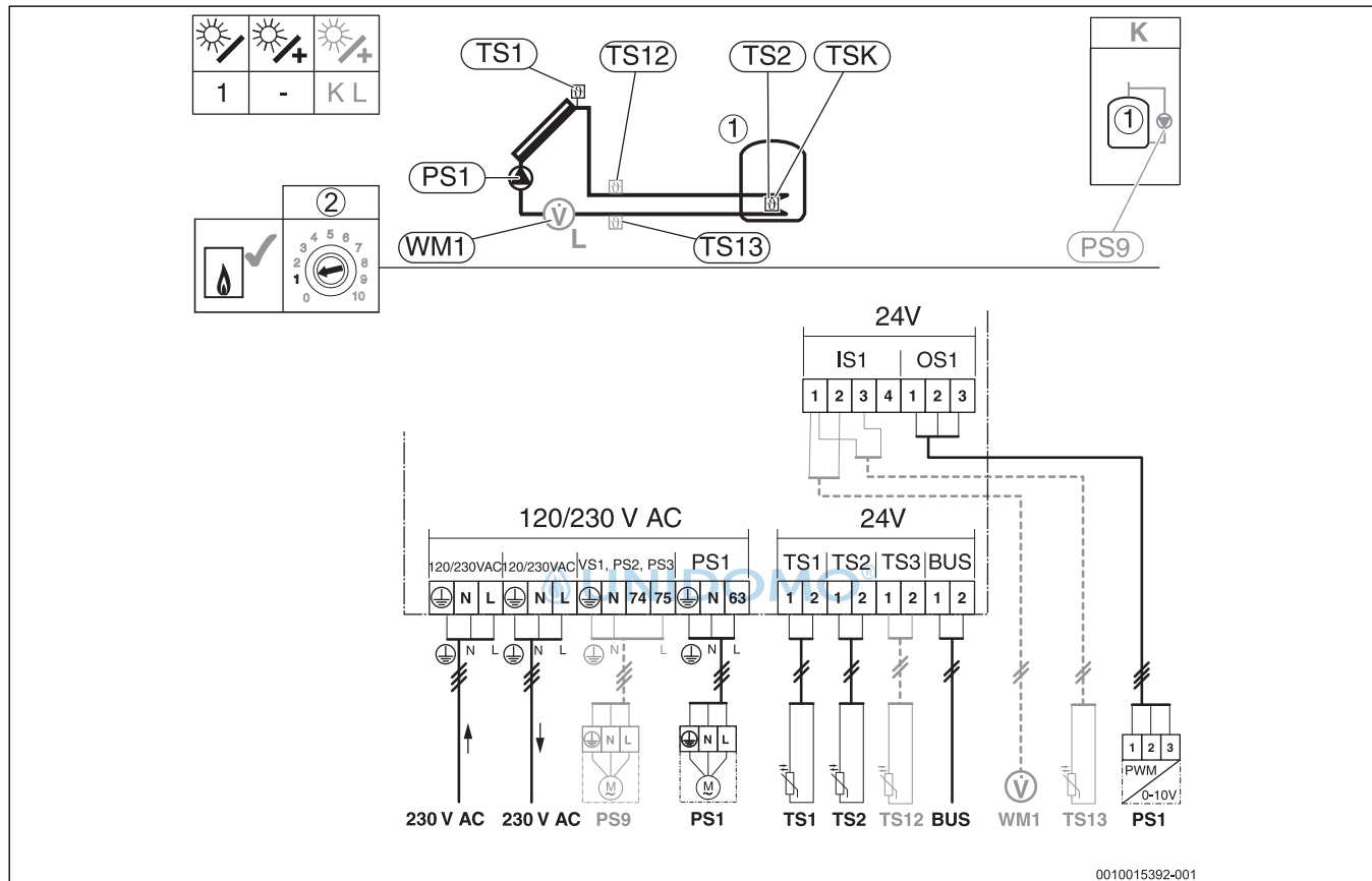
Bild 2 Elektrischer Anschluss
