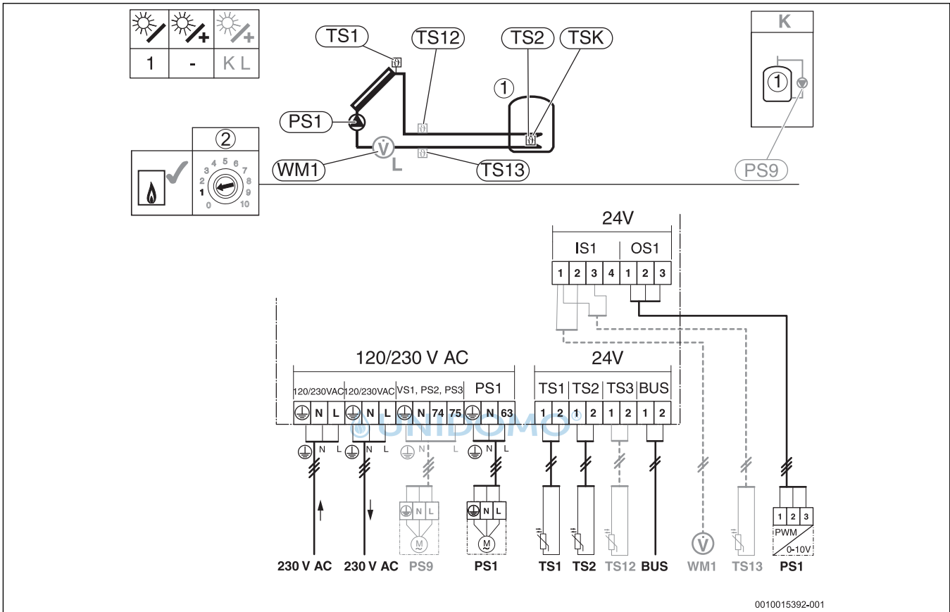
Fig. 2 Conexión eléctrica
