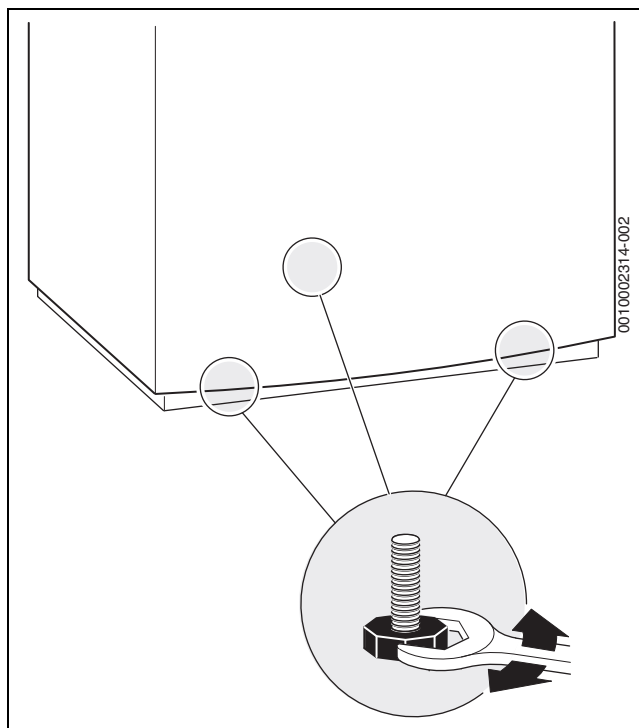
Bild 53 Speicher ausrichten
