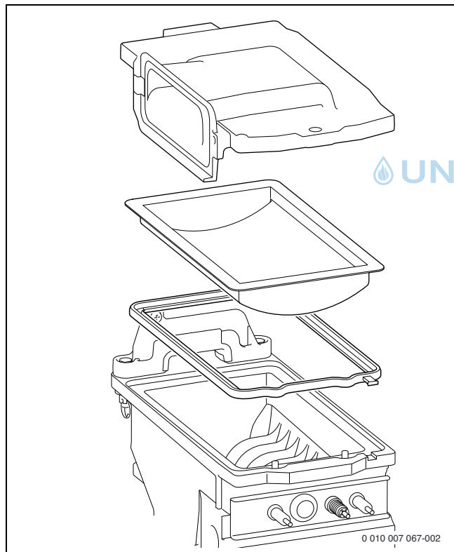
Bild 255 Brenner
