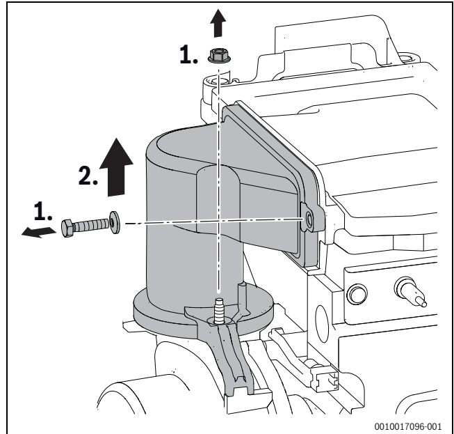
Bild 263 Mischeinrichtung ausbauen
