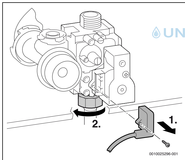
Bild 268 Stecker abziehen und Überwurfmutter lösen
