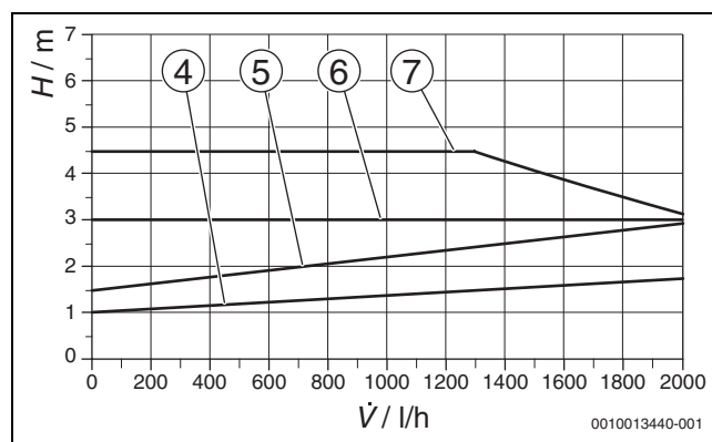
Bild 281 Pumpenkennlinien für Proportionaldruck und Konstantdruck
