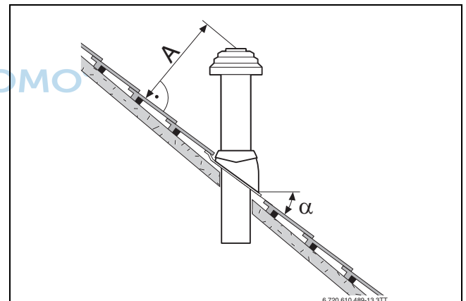
Bild 24 Abstandsmaße und Dachneigungen bei Schrägdach
