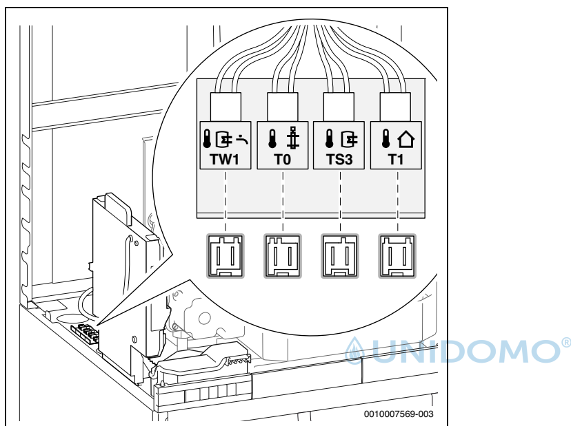
Bild 230 Stecker am Steuergerät
