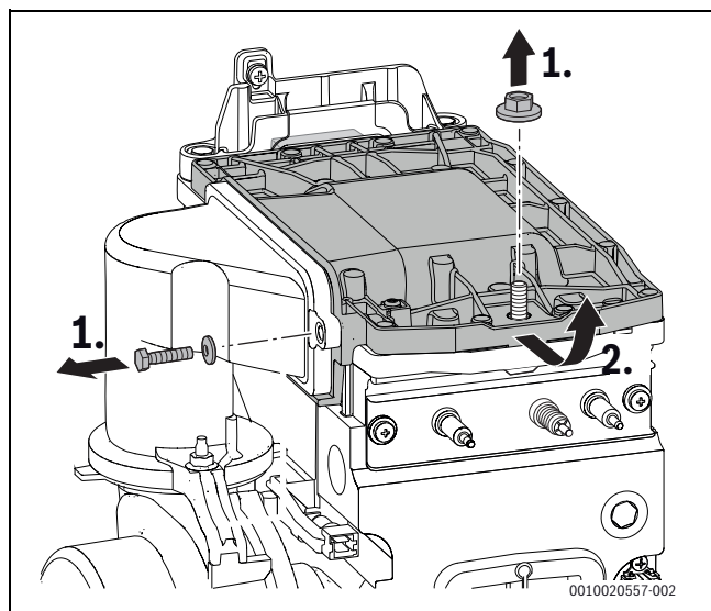
Bild 254 Brennerdeckel ausbauen
