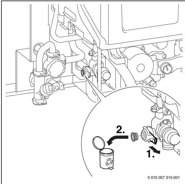
Bild 115 Stopfen entfernen
