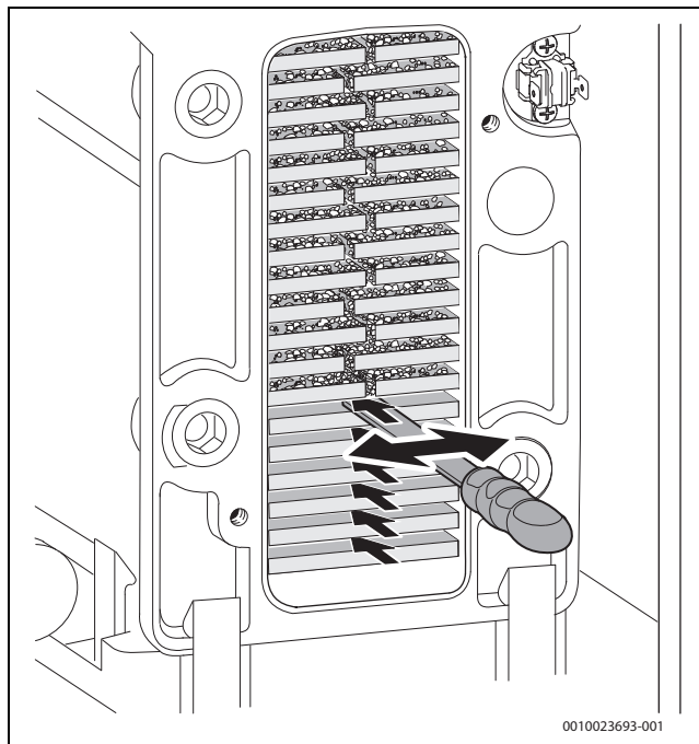
Bild 257 Reinigungsmesser
