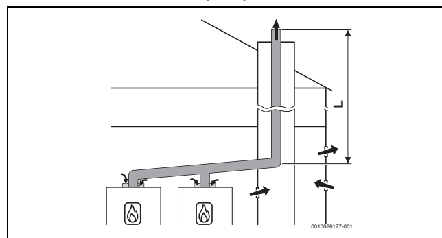
Bild 43 Kaskade mit 2 Geräten: Starre Abgasführung im Schacht nach B 23p /B 53p mit raumluftabhängiger Luftzufuhr am Gerät
