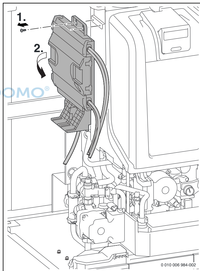
Bild 62 Steuergerät abnehmen
