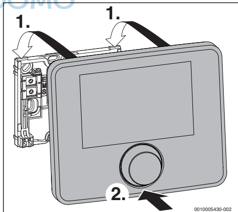
Bild 5 Bedieneinheit einhängen
