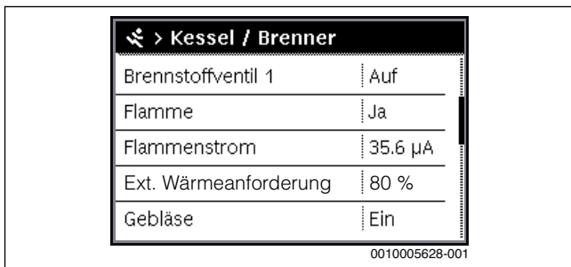
Bild 55 Ionisationsstrom (Flammenstrom) im Menü Monitoring
