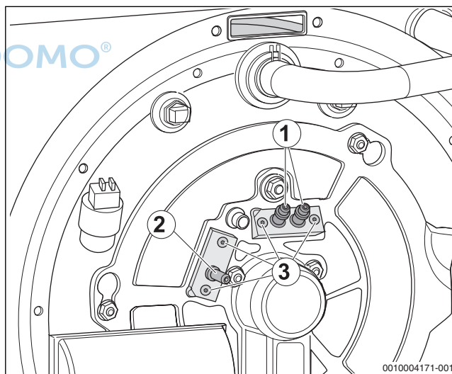
Bild 69 Elektrodenposition
