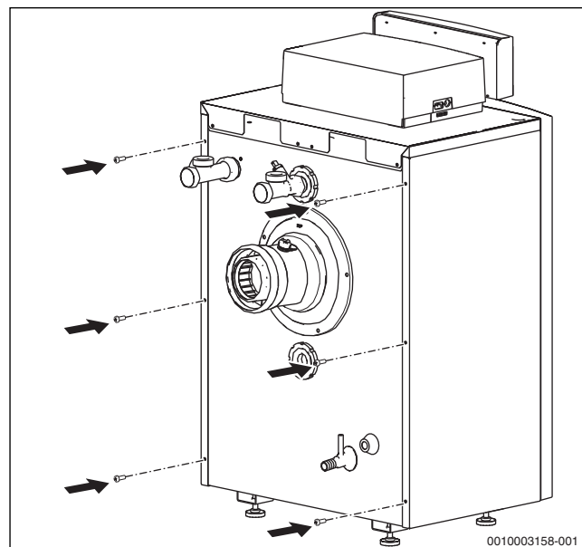
Bild 78 Seitenwände befestigen
