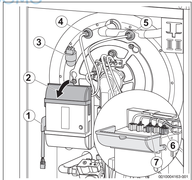
Bild 61 Steckverbinder lösen
