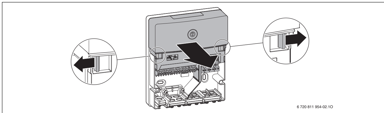
Bild 26 Funktionsmodul entfernen
