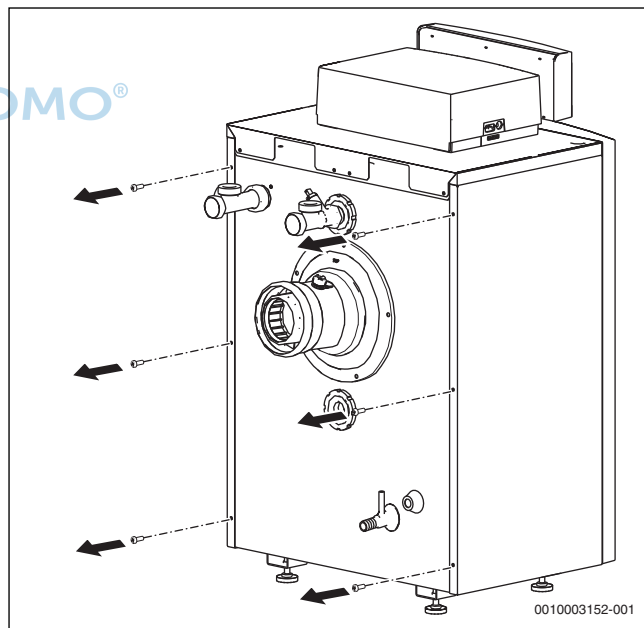
Bild 72 Befestigungsschrauben lösen
