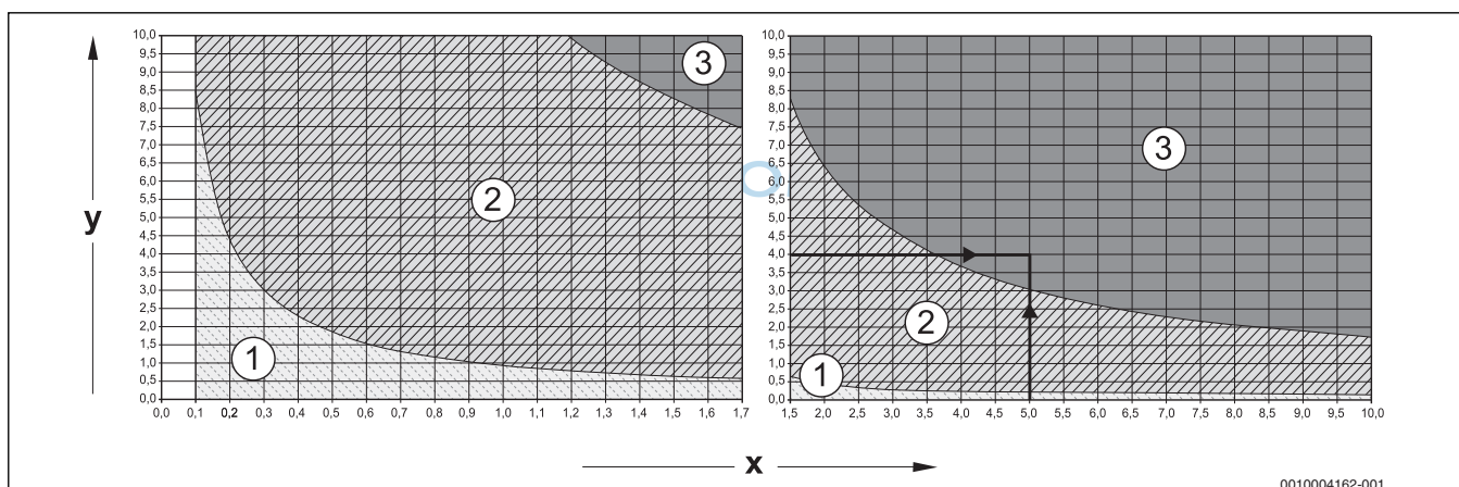
Bild 59 Zulässiger Druckabfall pro Minute bei der inneren Dichtheitsprüfung mit vorhandenem Gasdruck
