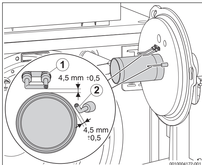
Bild 70 Abstände Elektroden
