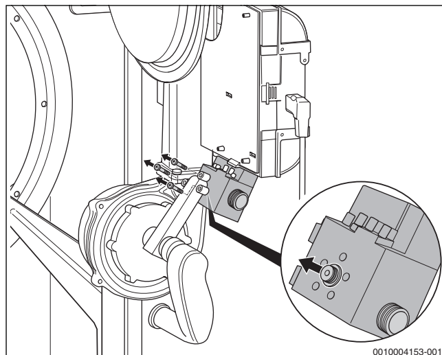
Bild 17 Gasarmatur
