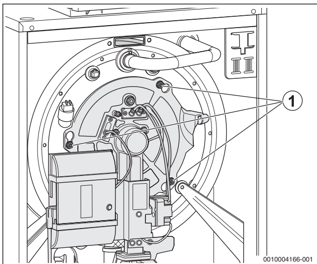
Bild 64 Befestigungsmuttern lösen
