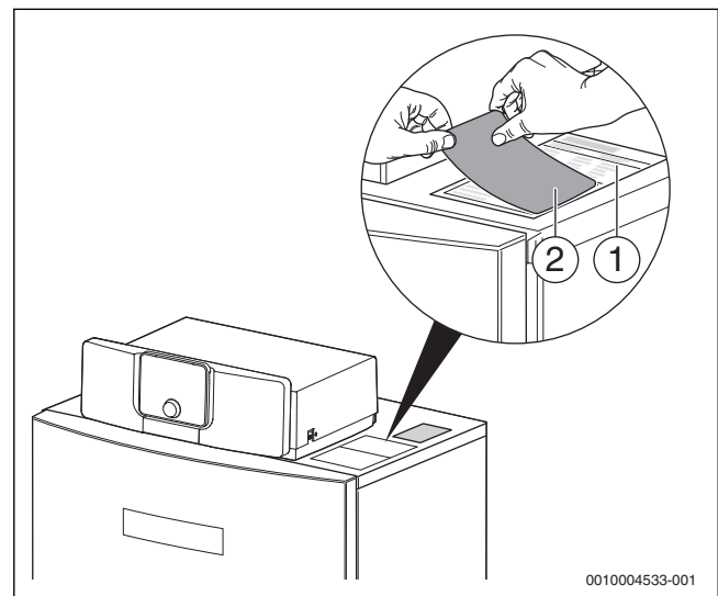
Bild 31 Typschild aktualisieren
