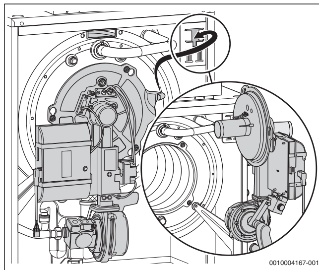
Bild 65 Brenner in Wartungsposition
