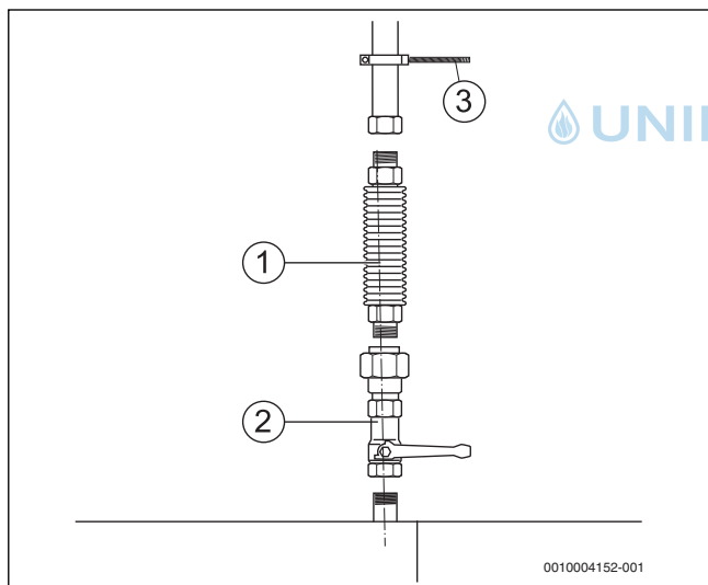
Bild 16 Gasanschluss herstellen
