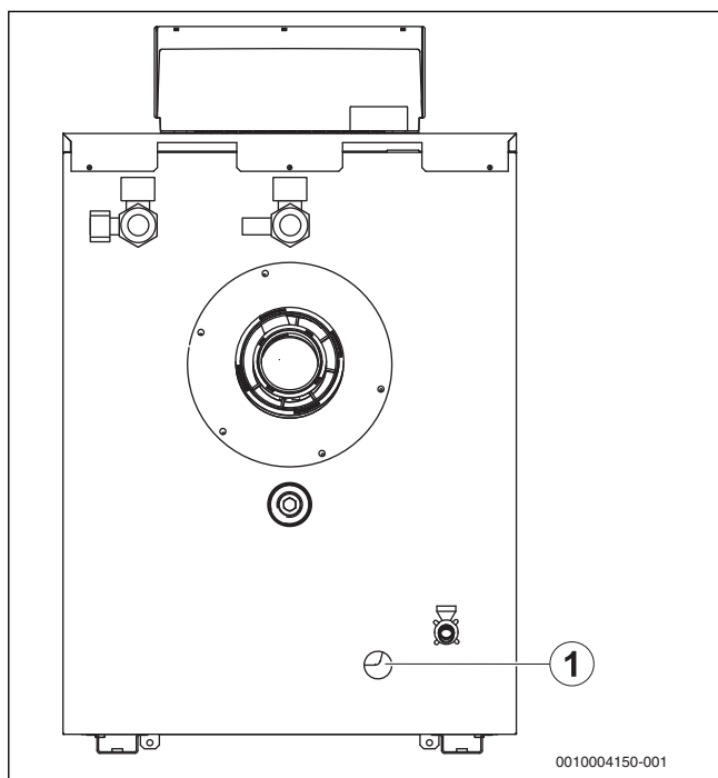
Bild 12 Kondensatschlauch montieren
