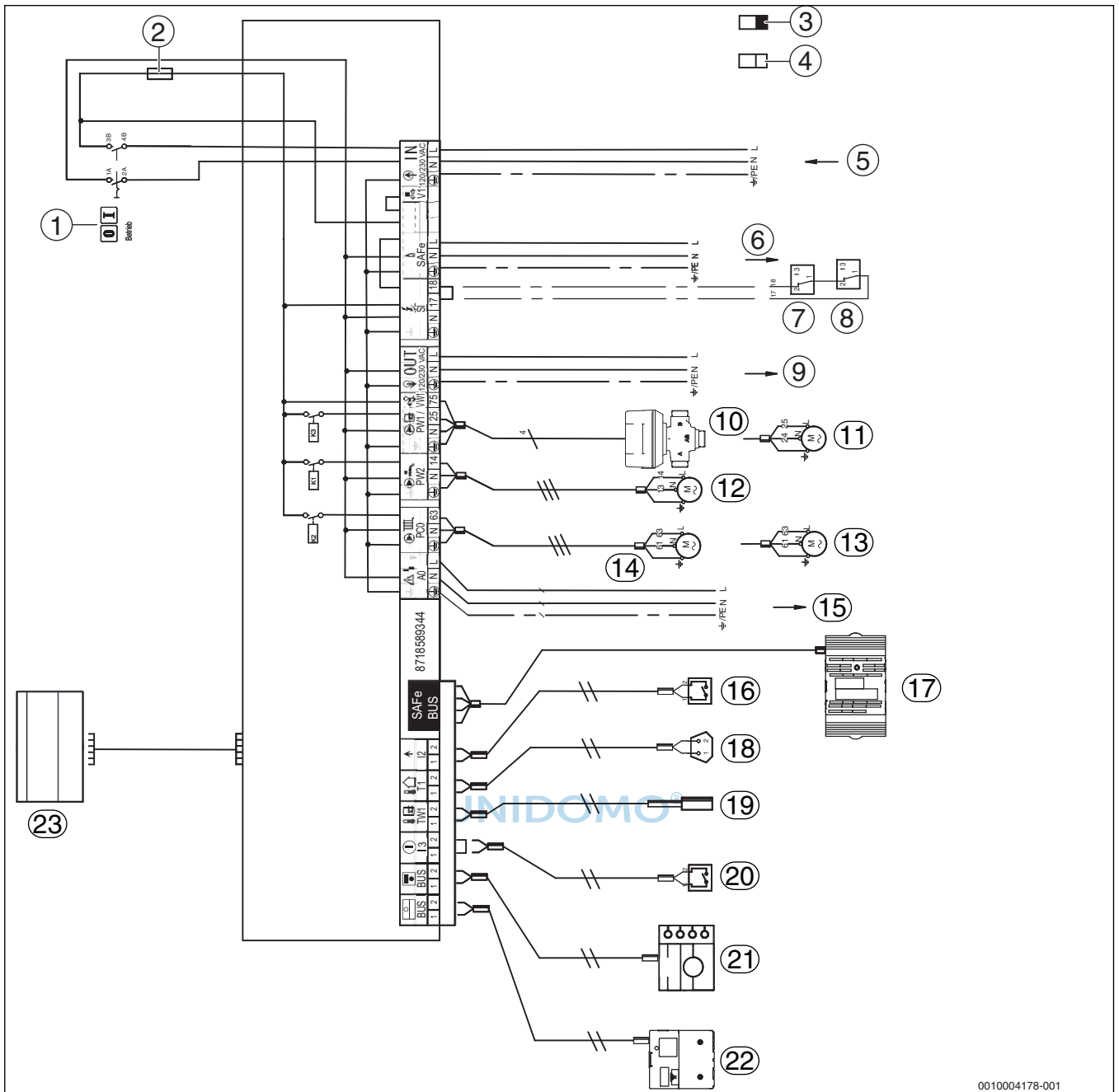
Bild 81 Anschlussplan Regelgerät MX25
