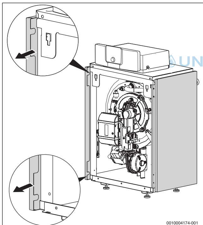
Bild 74 Seitenwände aus dem Rahmen schieben
