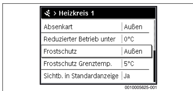
Bild 45 Frostschutz einstellen
