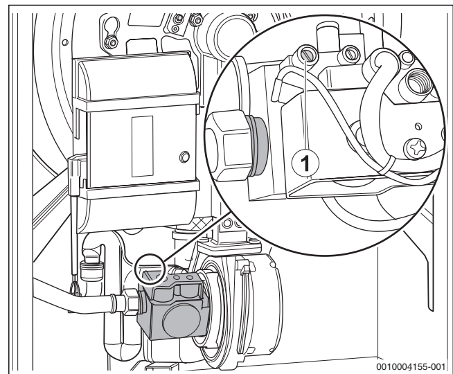
Bild 32 Gasleitung entlüften
