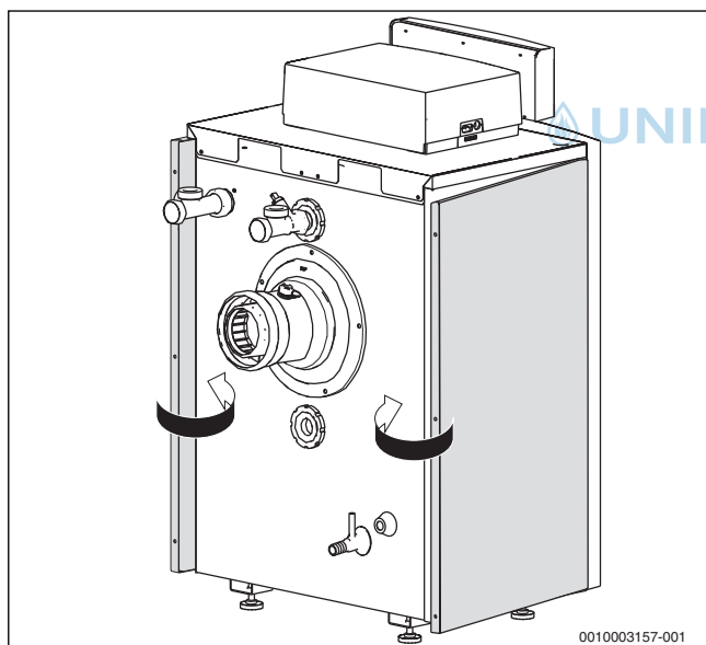
Bild 77 Seitenwände über die Kesselrückwand drücken
