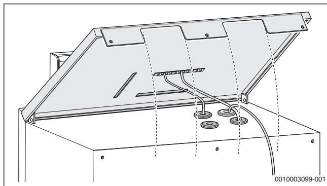
Bild 21 Haube anheben
