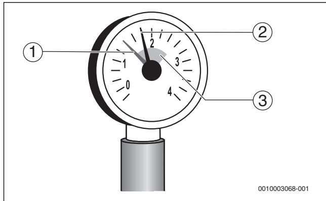
Bild 60 Manometer für geschlossene Anlagen
