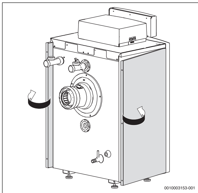
Bild 73 Seitenwände nach außen schwenken
