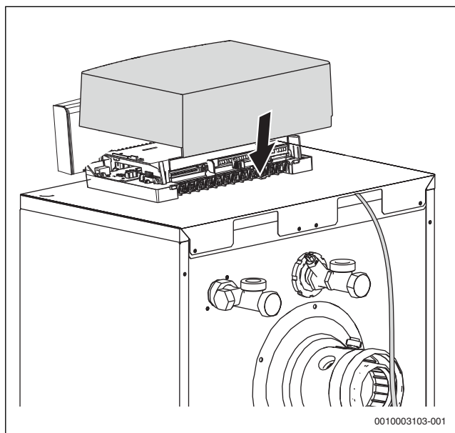
Bild 29 Abdeckhaube montieren
