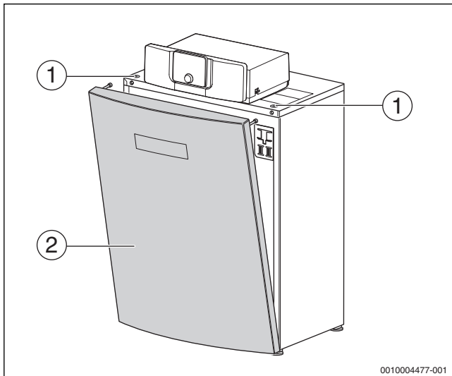
Bild 56 Kesselvorderwand montieren
