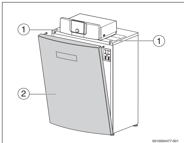
Bild 7 Kesselvorderwand demontieren
