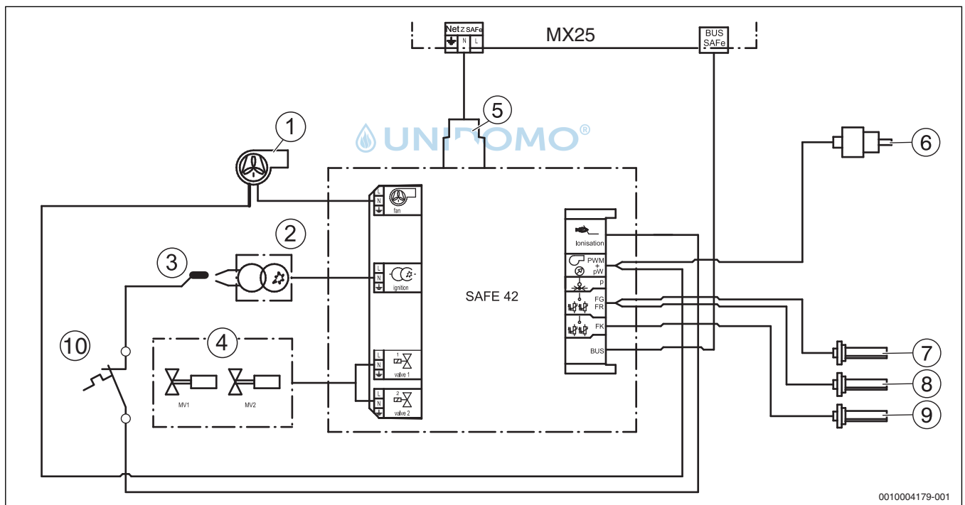
Bild 85 Anschlussplan Feuerungsautomat SAFe (15...40 kW; auch 50 kW bei manchen Modellen)
