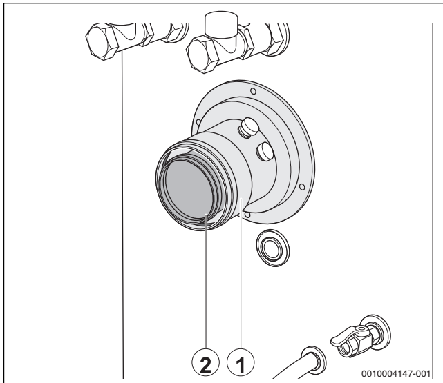
Bild 9 Abgasanschluss montieren
