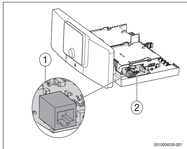
Bild 49 IP-Modul im Regelgerät
