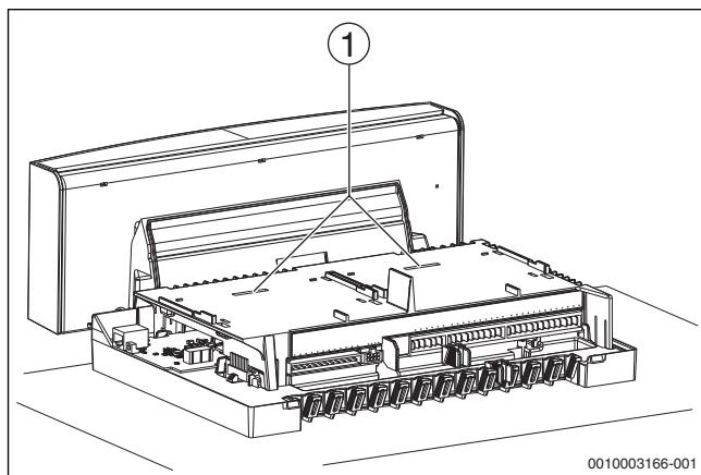
Bild 82 Ansicht ohne Abdeckhaube und ohne Module
