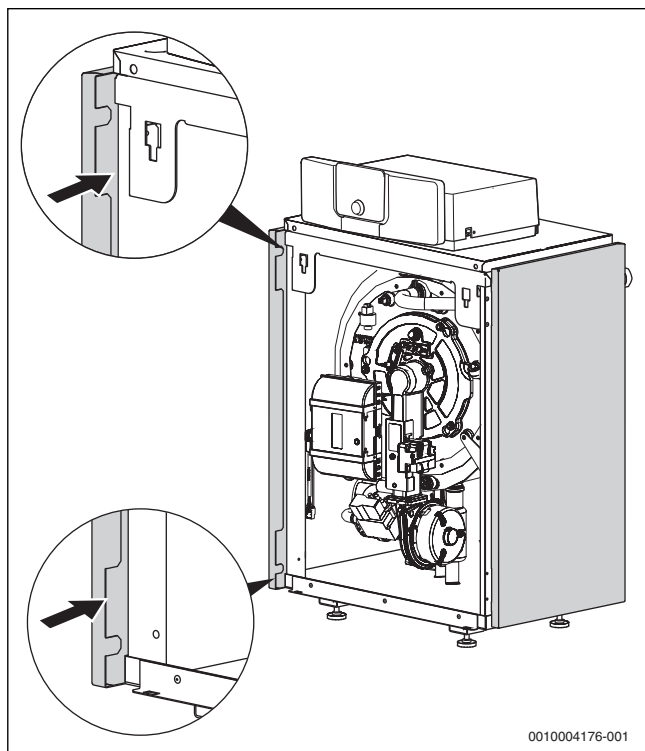
Bild 76 Seitenwände ansetzen und nach hinten schieben
