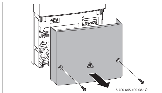
Bild 25 Gehäuse öffnen
