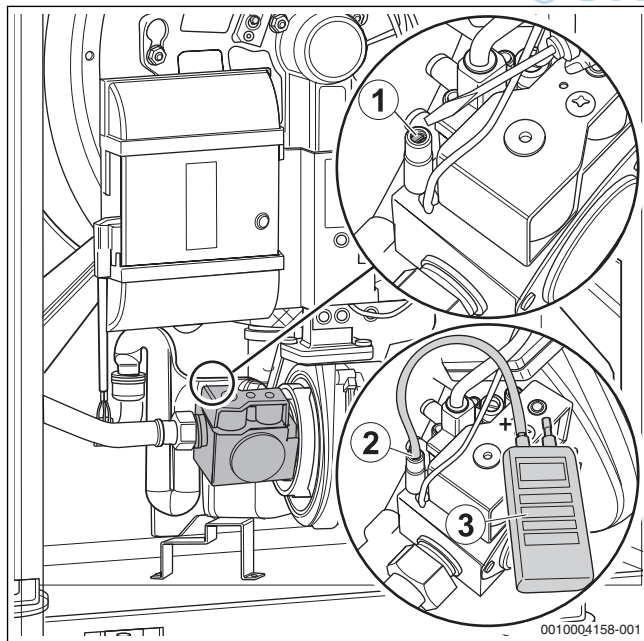
Bild 50 Gas-Anschlussdruck messen
