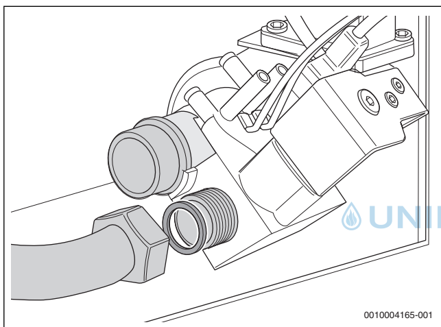
Bild 63 Anschlüsse an der Gasarmatur lösen
