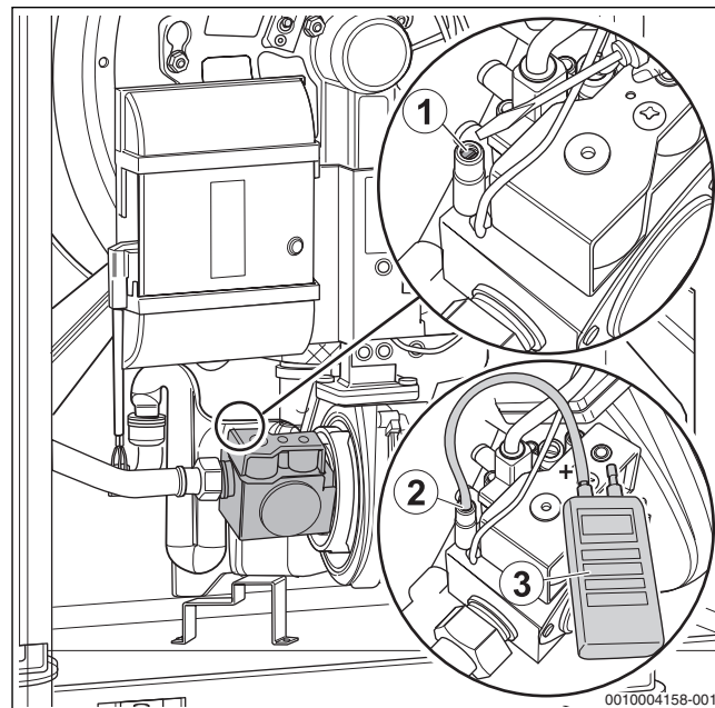
Bild 58 Gas-Anschlussdruck messen
