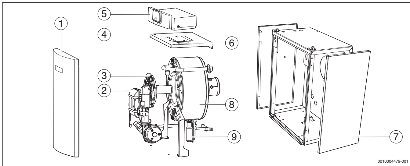
Bild 2 GC7000F 15...50 – Hauptbestandteile
