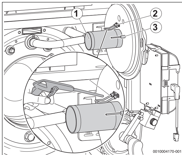
Bild 68 Brennerrohr mit Druckluft ausblasen
