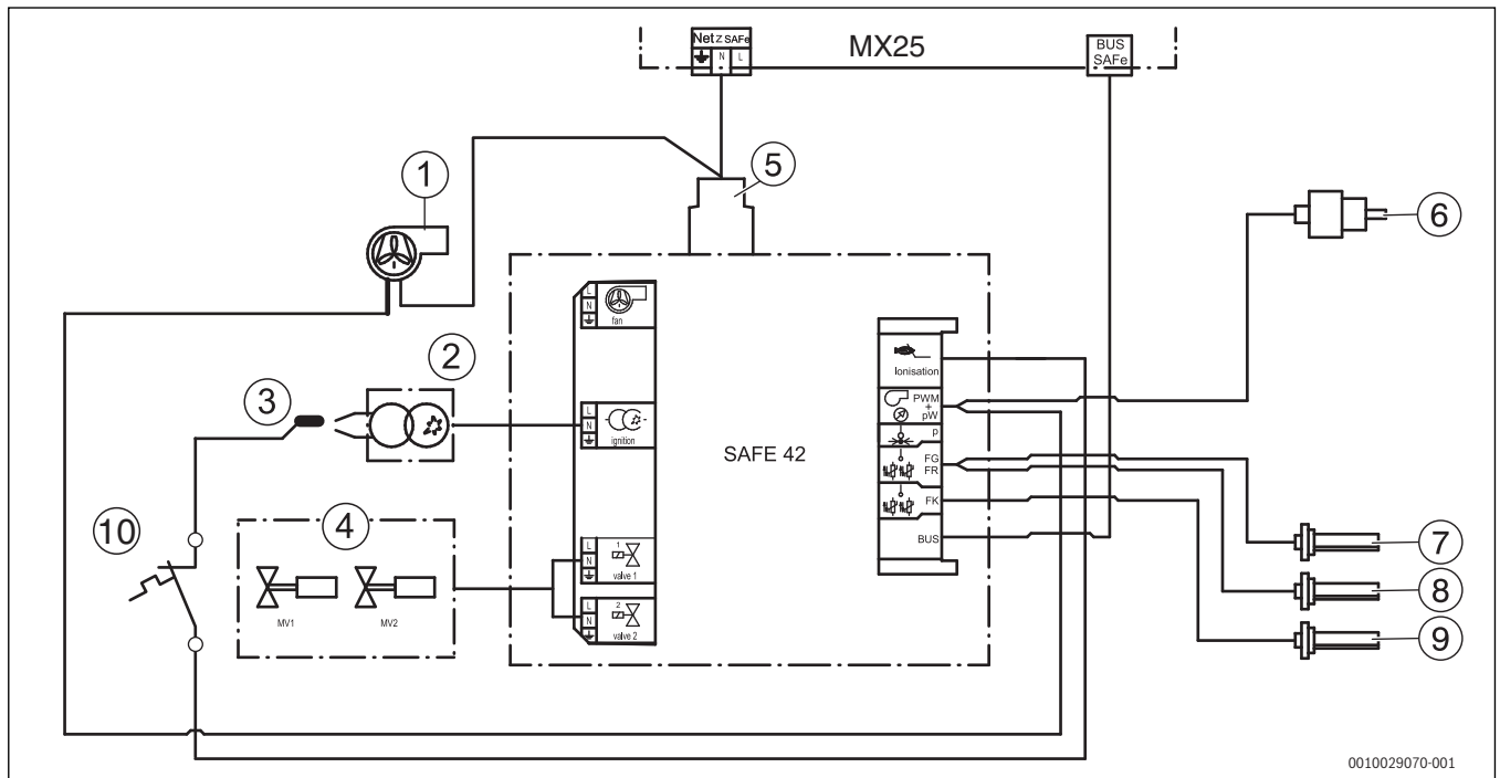
Bild 84 Anschlussplan Feuerungsautomat SAFe (50 kW; nicht bei allen Modellen)
