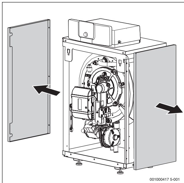
Bild 75 Seitenwände abnehmen
