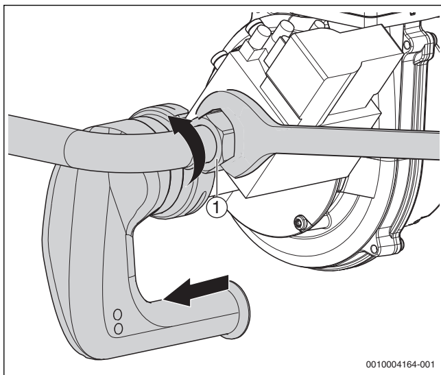
Bild 62 Anschlüsse an der Gasarmatur lösen (Bild beispielhaft 22 kW Kessel)
