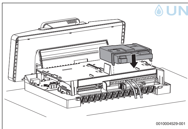
Bild 27 Funktionsmodule einstecken
