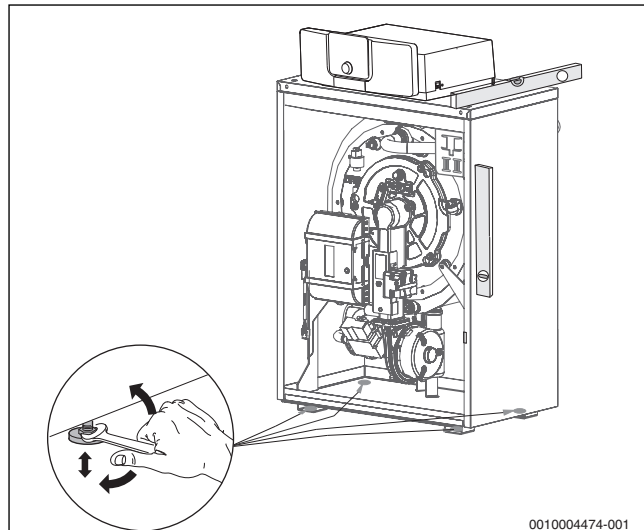
Bild 8 Heizkessel ausrichten
